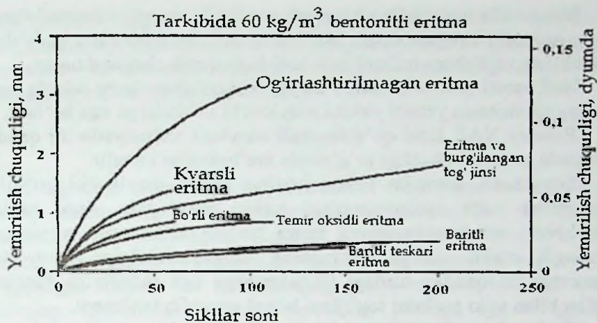
10.1-rasm. Mustahkamlash quvurlariga og'irlashtirilgan burg'ilash eritmalarini turini ta'sir etish grafiklari
