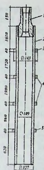
17.6-rasm. Diametri 168 mm li mustahkamlash tizmasini tekshirish uchun shablon: 1-uzatma; 2-korpus; 3-yuqori halqa; 4-oraliq halqa; 5-pastki halqa.
