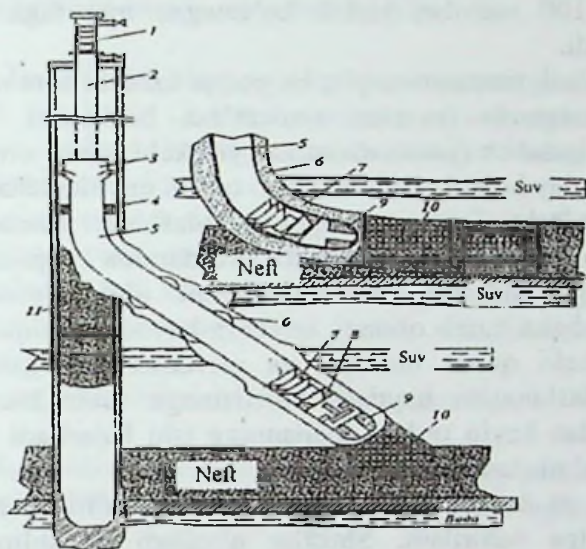
19.4- rasm. Yon stvolni o'rnatish sxemasi:
