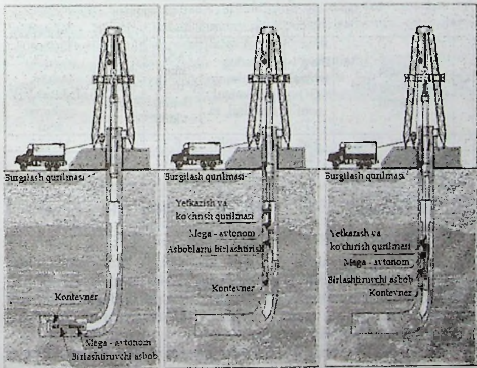
7.3-rasm. TBTT apparaturasi jamlanmasining tarxi
