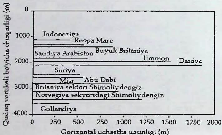
6.3-rasm. Gorizontalar quduqlarni burg'ilashni har xil mamlakatlarda kengayishi
