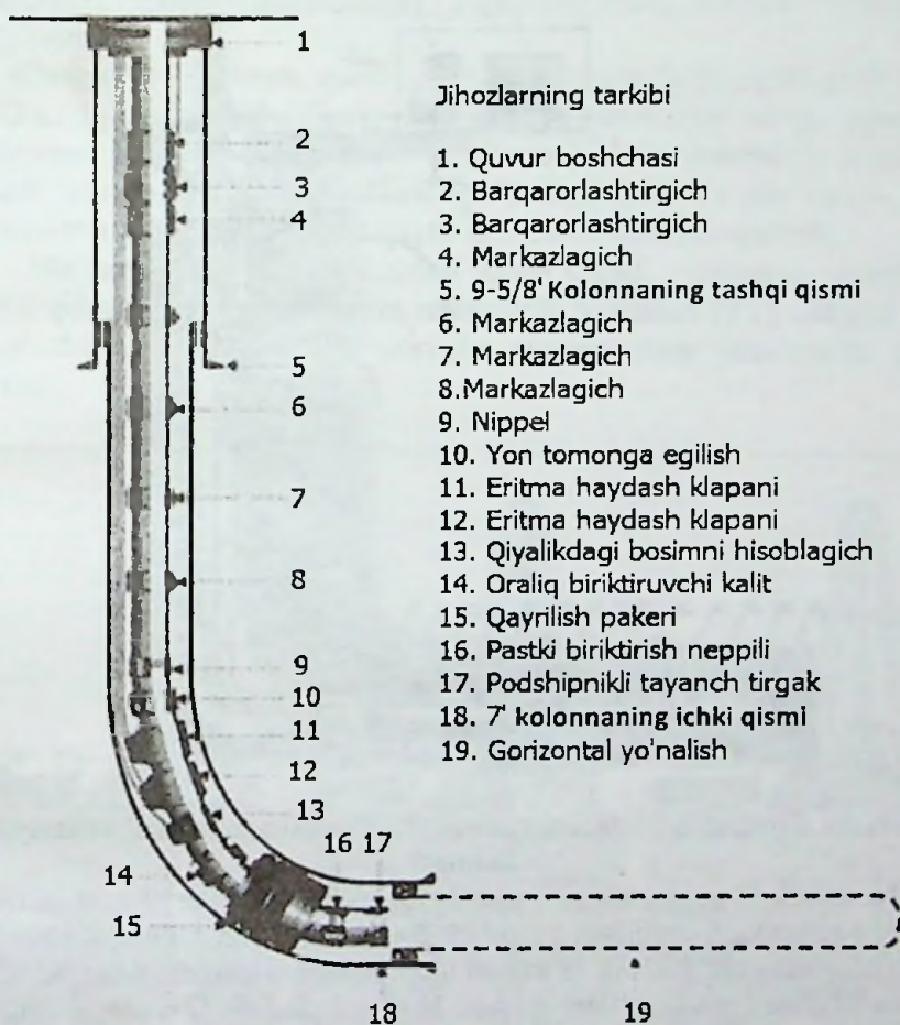
7.1-rasm. Gorizontaal quduqning umumiy ko'rinishi va ichki jihozlari
