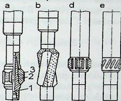
3.3-rasm. Turboburli burg'ilashda qo'llaniladigan barqarorlashtirgich qurilmalari:
