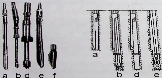
1.4-rasm. Pona shaklli og'dirgichlar
