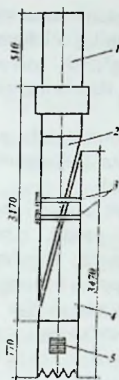
17.4-rasm. Klinli og'dirgichli jamlanma: 1-magnitli uzatma; 2-tushiriladigan klin; 3-qirquvchi boltlar; 4-og'diruvchi klin; 5-plashkalar.
