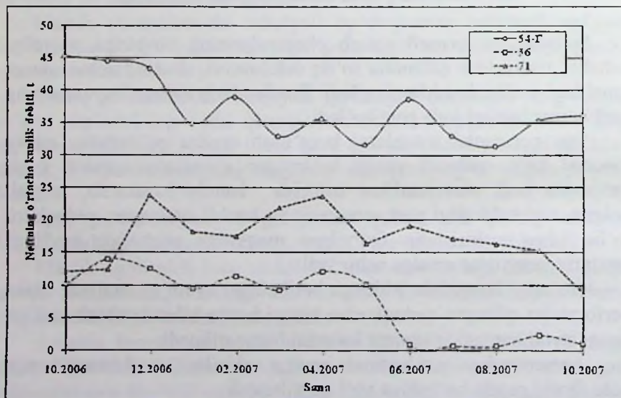
6.8-rasm. № 54-G gorizontal quduq va №56, №71 vertikal quduqlardan o'rtacha kunlik qazib olinadigan neftni taqqoslash grafigi
