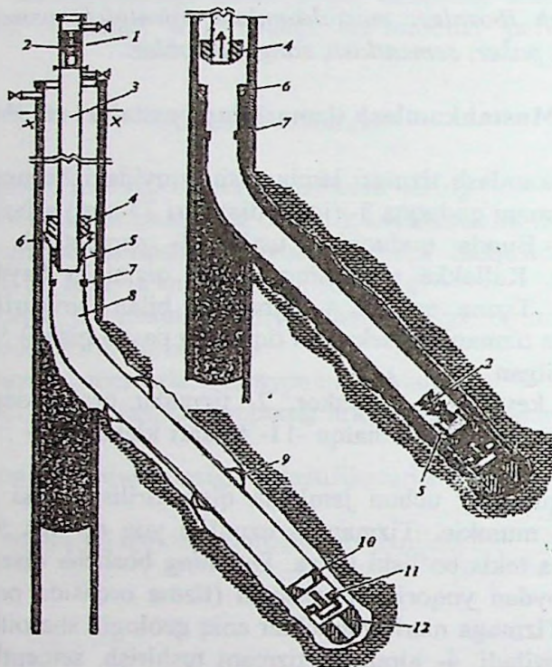
19.1-rasm. Yon stvolli quduqning jamlanmasi:
