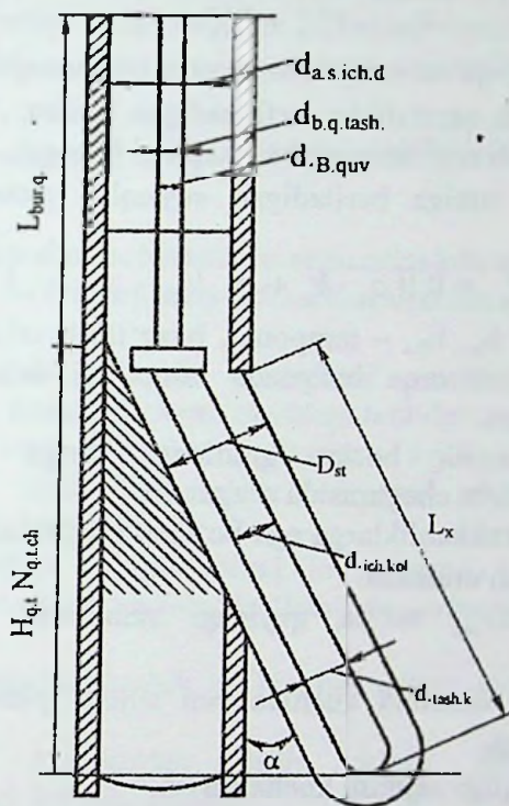
18.1-rasm. Qo‘shimcha stvolni quduq konstruksiyasini gidravlik hisoblash sxemasi
