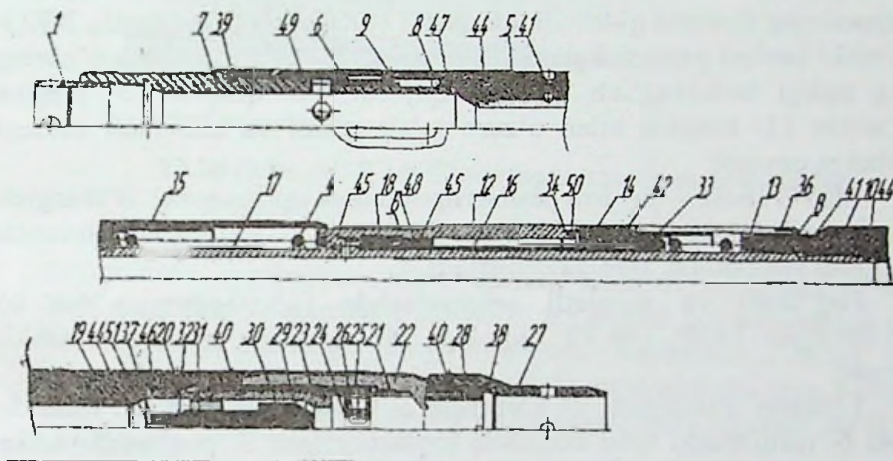
13.9-rasm. Ko'p funksional boshqaruvchi jihoz – KRR.146.050 o'tkazgich
