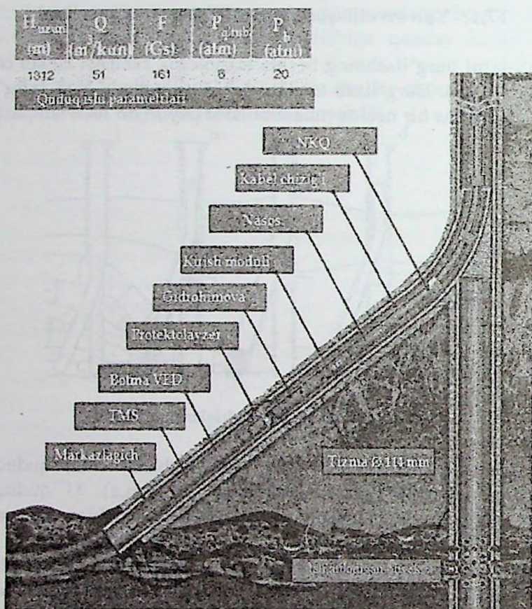
17.2-rasm. Yon stvol quduqlarda ichki jihozlarning joylashuvi
