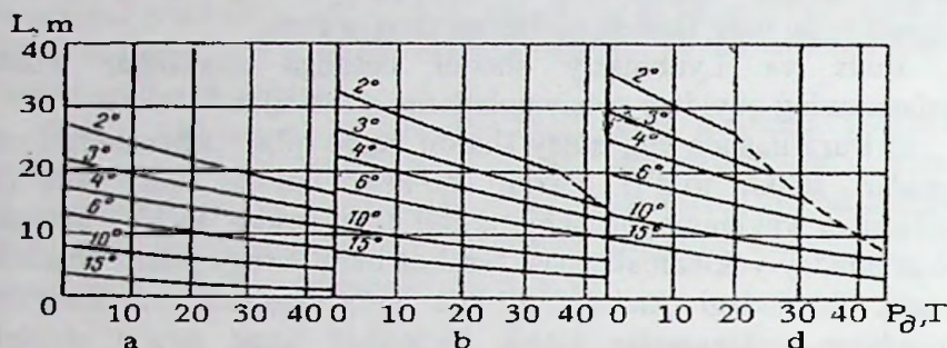
1.2-rasm. Markazlagichlarni eng qulay o'rnatish joy aniqlanadigan nomogramma:
