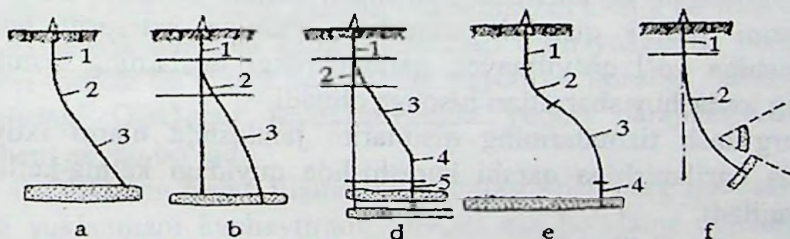
1.1-rasm. Qiya quduqlarning profili:
