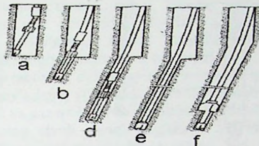
1.5-rasm. Sharnirli og'dirgichlar
