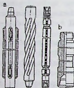
3.2-rasm. Barqarorlashtiruvchi qurilmalar: a – barqarorlashtirgichlar; b – maxovik.
