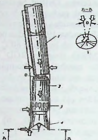
13.3-rasm. Muvozanatlangan burg'i ustiga o'rnatiladigan kengaytirgich:
