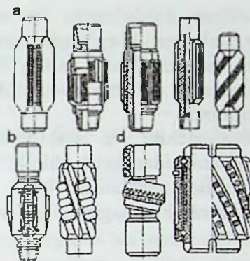
3.1-rasm. Kalibratorlar: a - parrakli; b - sharoshkali; d – sharikli.
