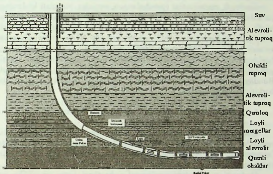
14.1-rasm. Quvurlarning orqa halqasini pakerlar va sementlash muftalari yordamida berkitish
