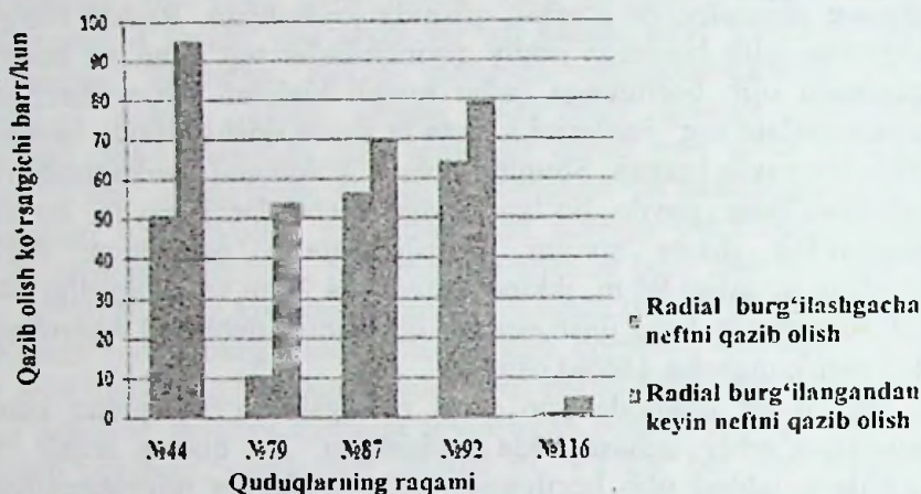
20.14-rasm. Radial burg'ilangan quduqlarning ko'rsatkichlarini taqqoslash diagrammasi
