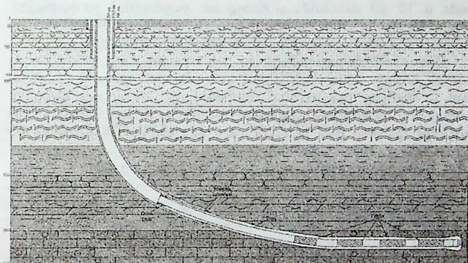
14.4-rasm. Gorizontal quduqlarni filtr yordamida tugallash sxemasi
