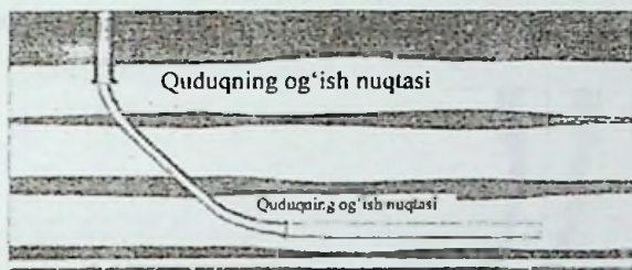
14.2-rasm. Gorizontall quduqni ochiq stvol bilan tugallash Teshilgan yoki qirqilgan «xvostovik»lar
