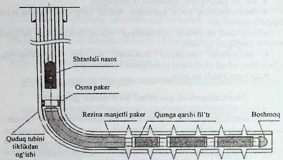
14.7-rasm. Gorizontal uchastkani teskari klapan bilan jihozlash
