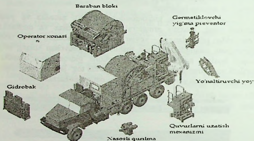
20.7 -rasm. Maxsus koltyubing jamlanmasining umumiy ko'rinishi
