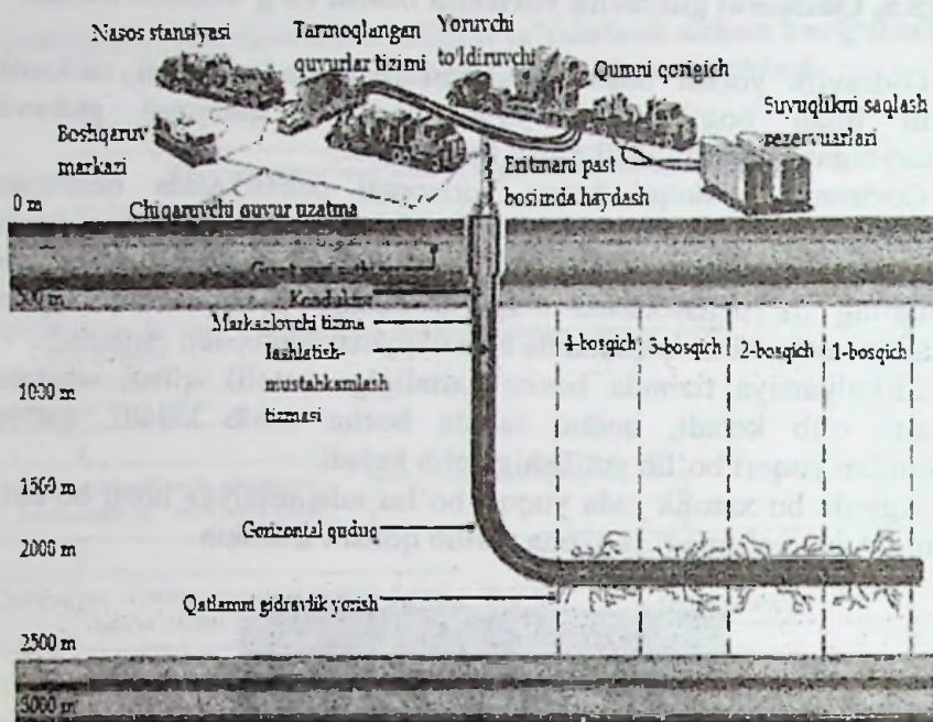
15.1-rasm. Gorizontaal uchastkani bosim ta'sirida yorishda qo'llaniladigan mashinalarni joylashuv holati
