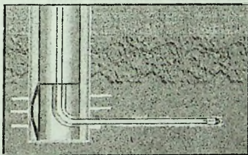
20.13-rasm. Deflektorli va gorizontaal yo'naltirilgan oqim yordamida perforatsiya qilishni amalga oshirish
