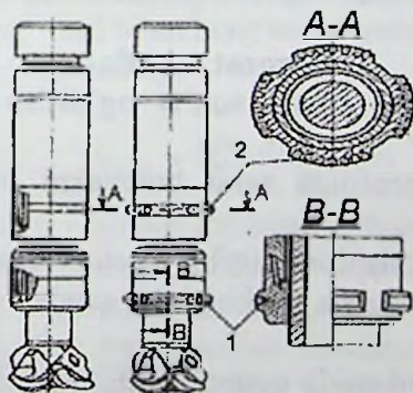
3.4-rasm. ZTSSH1-195 turboburlari uchun oraliq seksiyali va nippelli stabilizatorlar:
