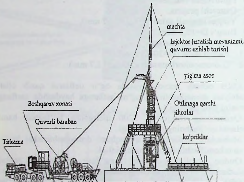
20.10-rasm. Kolyubing qurilmasining umumiy ko'rinishi
