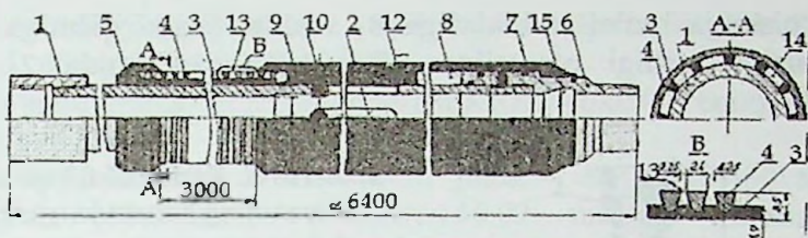
13.7-rasm. KRR.146.02 turidagi boshqariladigan quduq filtri:
