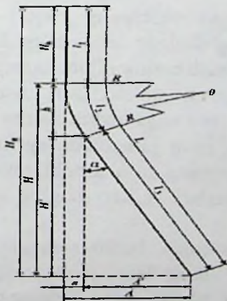
2.2-rasm. Tangensial tipdagi yo'naltirilgan quduqning vertikal proeksiyasi
