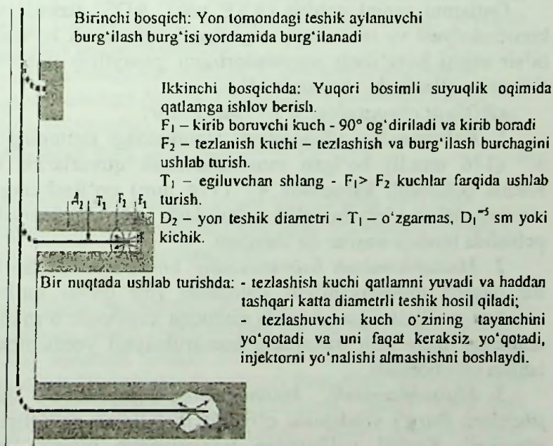
20.11-rasm. Radial burgʻilashni olib borish jarayonlari
