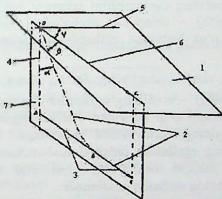
9.1-rasm. Quduqning fazoviy holatini aniqlovchi elementlar:
