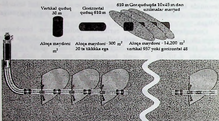
6.1-rasm. Gorizontal quduqning umumiy sxemasi tasvirlangan
