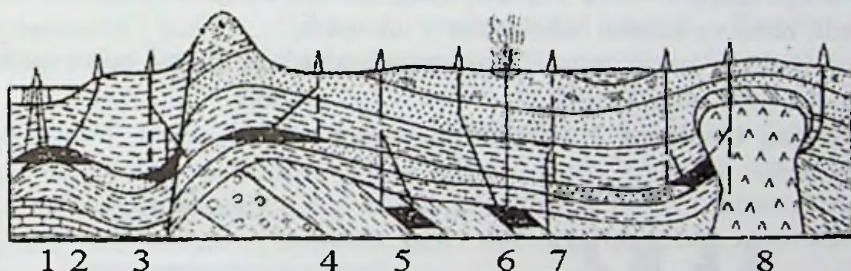
1.3-rasm. Qiya burg'ilashni ko'rinishlari:
