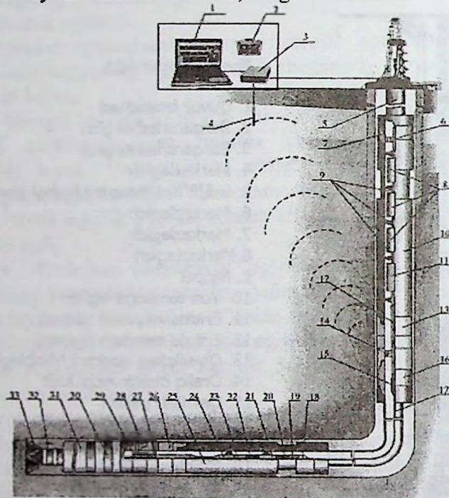
7.2-rasm. Elektroburi telemetrik tizim (ETT) va tugunlar jamlanmasining sxemasi:
