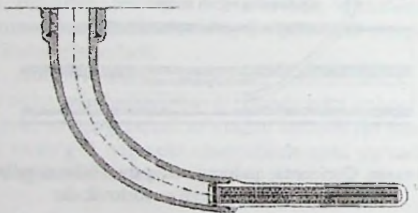
14.3-rasm. Teshilgan «xvostovik» bilan gorizontal quduqni tugallash
