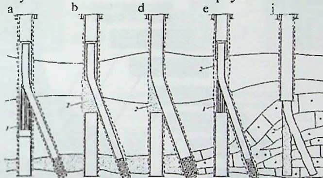
17.1-rasm. Yon stvolli quduqlarning profili
