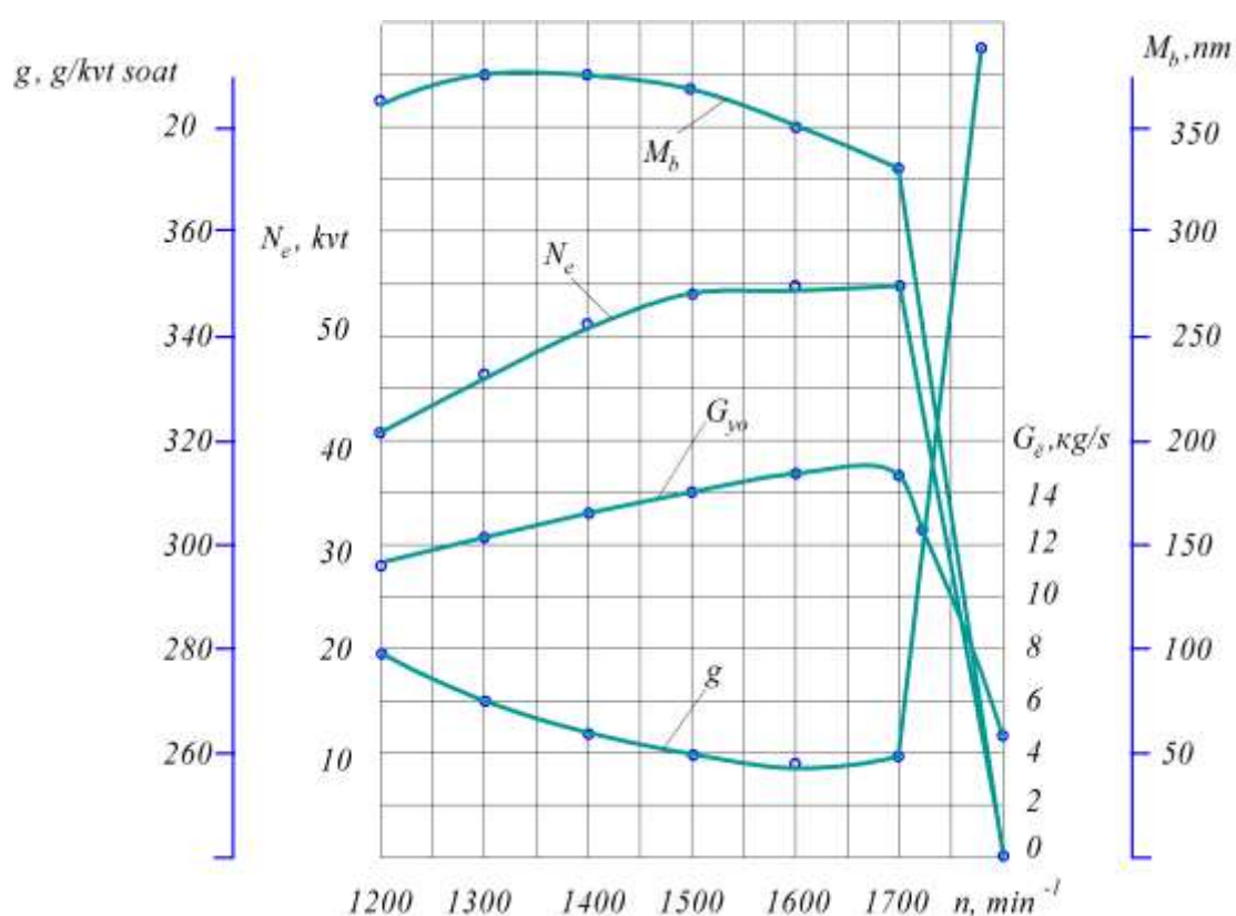
59-rasm. Dizel dvigateli tezlik xarakteristikasi grafigidan namuna
