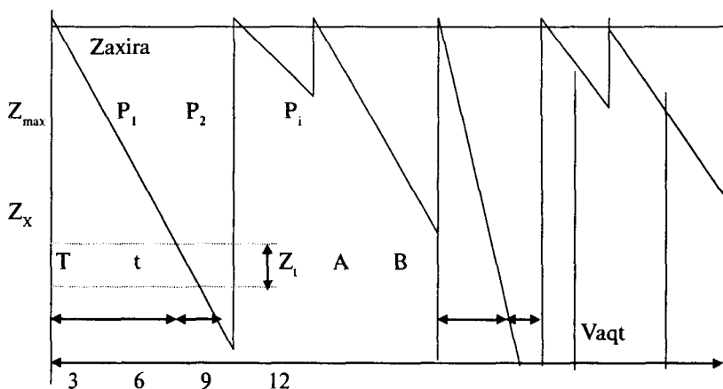
17-chizma. Zaxiralarni davr oralig'i zaxirasi holati ustidan nazorat qilish tizimining jadval modeli
