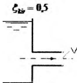
3.7.4-rasm. Suyuqlikning idishdan quvurga oqishi
