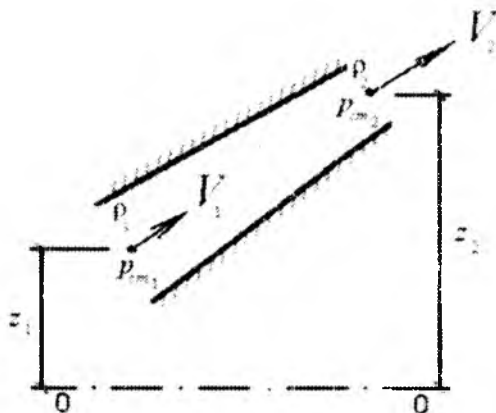
5.2.1-rasm. Gazlar uchun Bernulli tenglamasiga doir sxemasi.
