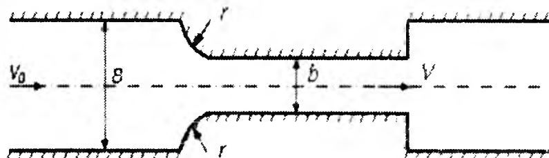
7.7.4-rasm. Zinasiz suv to'kgichning bir ko'rinishi
