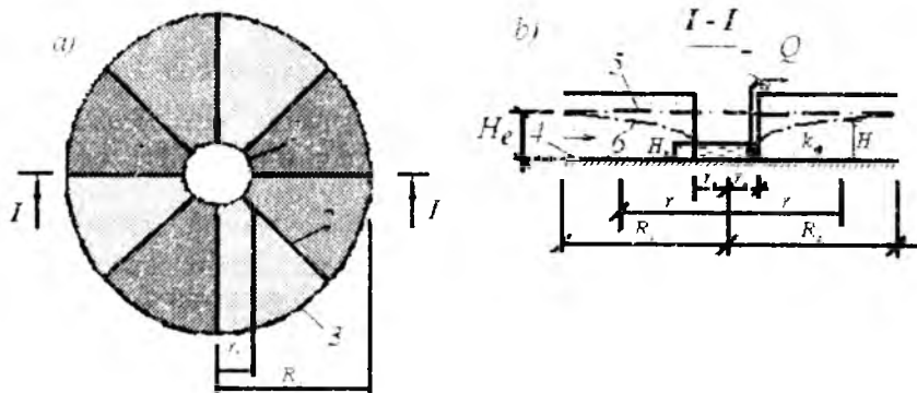
6.2.3. a, b-rasmlar. Tayyer chuqurga filtaratsiya. a-reja; b-ko'ndalang kesim: 1-chuqur, 2-filtaratsiya yo'nalishi, 3-chegara filtaratsiya maydoni; 4-suv bosimi, 5-issiq suvni tabiiy bosimi, 6-pasaytirilgan tabiiy bosimga aylanma harakat, 7-nasos.
