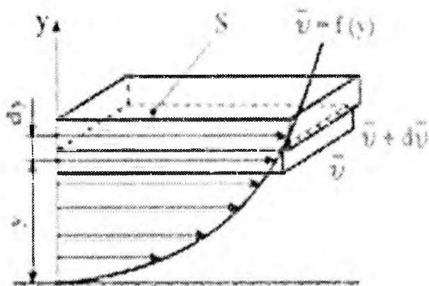
2.16.1-rasm. Qattiq devordagi suyuqlik yopishqoqligining epyurasi
