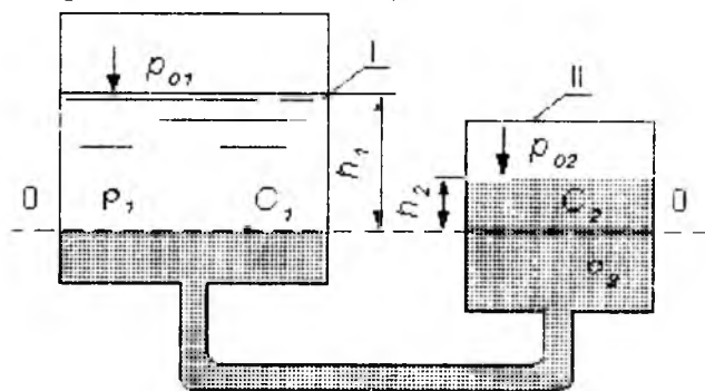
2.33.1-rasm. Tutashgan idishlar
