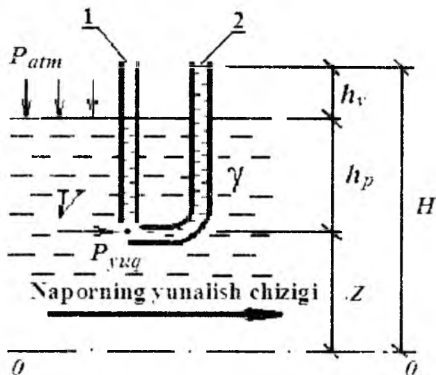
3.5.1-rasm. Gidrodinamik naporni tushintirishga doyr sxema: 1 – p'ezometr; 2-Pito naychasi.
