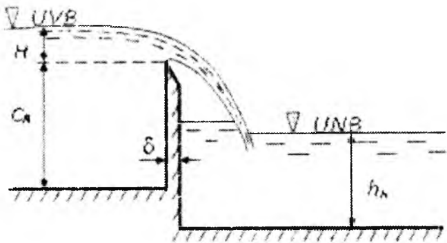
7.7.1-rasm. Yupqa devorli cho'ktirilmagan suvto'kgich
