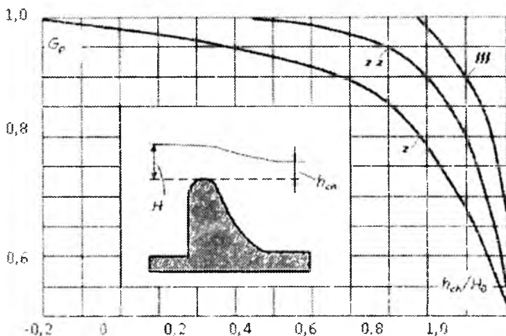
7.7.7-rasm. Amaliy profili suv to'kgichlarning cho'ktirish koeffitsiyenti \sigma_{ch} ni aniqlash grafigi
