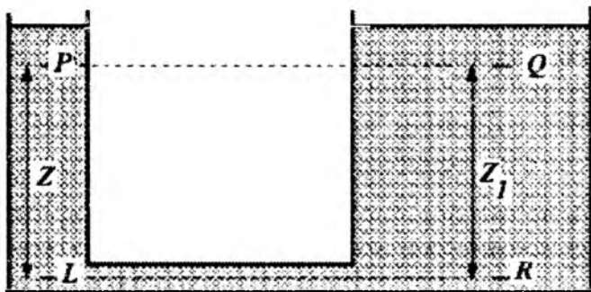
2.24.2-rasim. Ikkita turli ko'ndalang kesishuvli, quvur orqali bog'langan idishlar.
