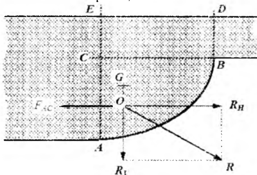
2.7.1-rasm. Cho'kkan egri sathdagi natijaviy kuch
