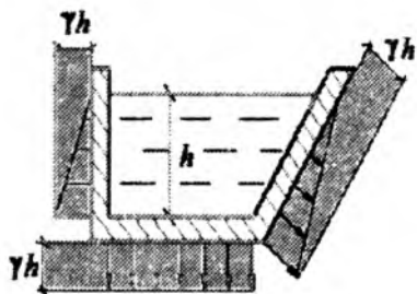
5.8.2-rasm. Yassi devoridagi suyuqlik ustini bosimining chizmasi.
