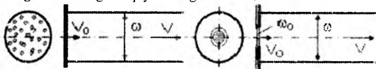
3.7.11-rasm. Shayba yoki chetlari o'tkir teshikli to'rlardan quvurga to'g'ri kirayotgan suyuqliklar
