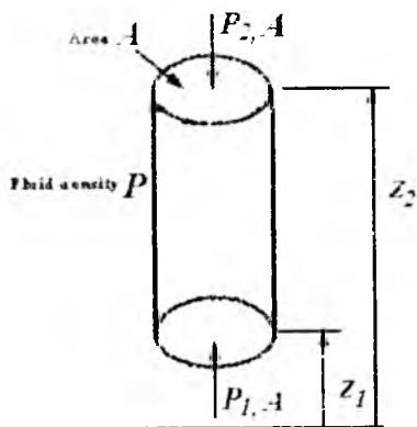
2.23.1-rasm. Og'irlik kuchi ta'siridagi suyuqlikda bosimning vertikal o'zgarishi
