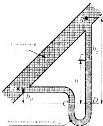
2.26.8-rasm. "U" –Trubkali manometr yordamida bosimlarning to'g'riiligini o'lchash
