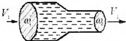
3.4.1-rasm. Oqim va oqimchalar tenglamasi uchun sxemasi.
