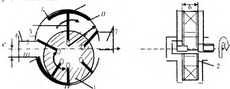
8.15.4-rasm. Plastinkali nasoslar.
