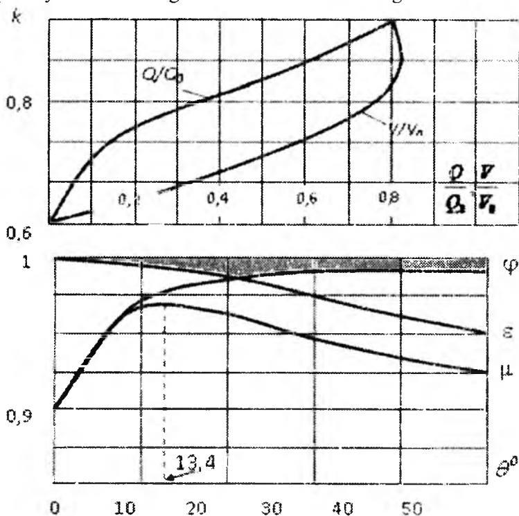
7.6.1-rasm. Tajribadan olingan bog'lanishlar
