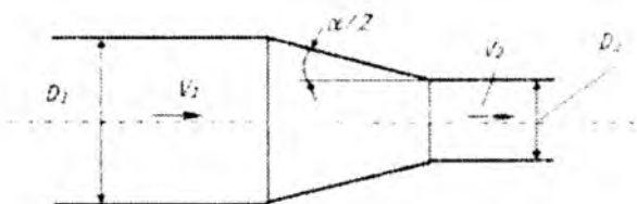
3.7.6-rasm. Konfuzorlar
