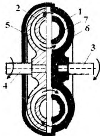
8.16.1-rasm. Gidrodinamik mufta yoki turbomufta nasos g'ildiragi
