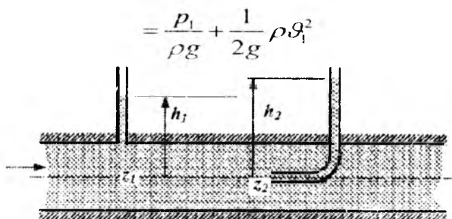
3.18.2-rasm. P'ezometr va Pito trubkasi
