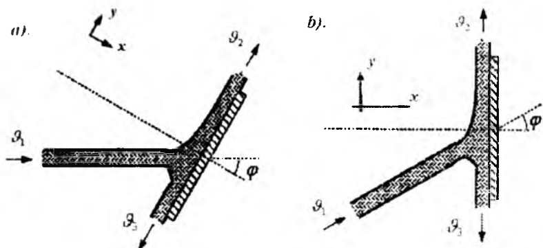
3.27.1-rasm. a – b. Qiya tekislikdagi reaktiv oqim \mathcal{Q}_3
