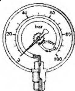
2.26.11. a-rasm. Purjinali manometr. 2.26.11. b-rasm. Membranaali manometr
