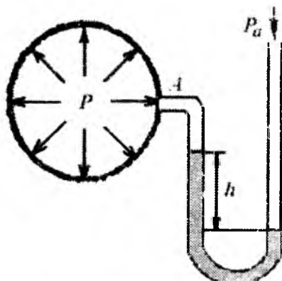
2.26.4-rasm. Vakuummetr
