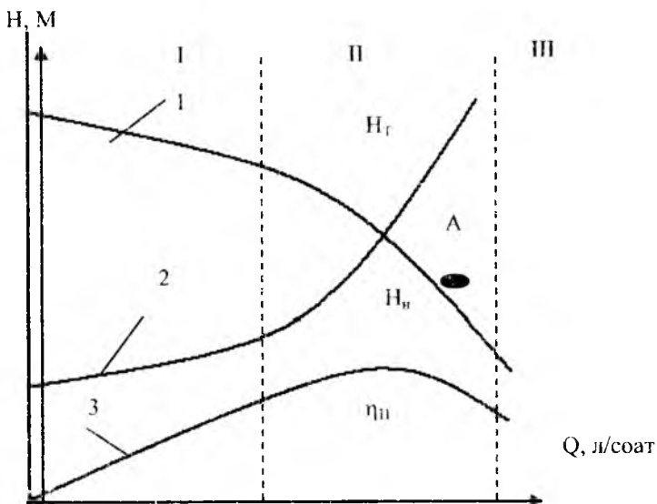
3 12.1-rasm Nasosning ishechi nuqtasini aniqlashga doir chizma
