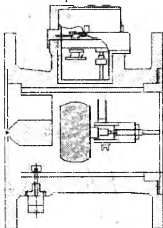
2.26.15-rasin. Spiralsimon parrakli suyuqlik hisoblagichi
