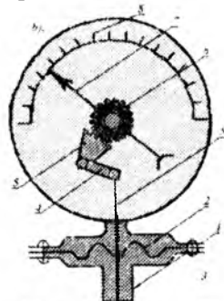
2.26.11. a-rasm. Purjinali manometr. 2.26.11. b-rasm. Membranaali manometr
