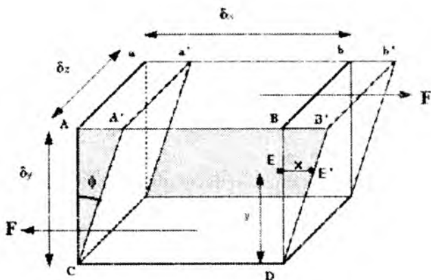
2.15.1-rasm. Ko'ndalang kuch ta'siridagi suyuqlik elementi.
