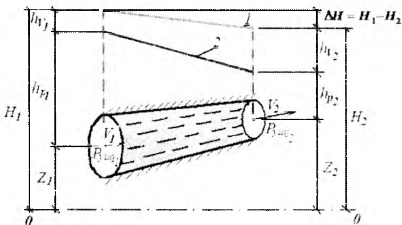
3.12.1-rasim. Bernulli tenglamasiga doir sxema:
