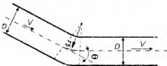
3.7.8-rasm. Quvurlarning tekis burilishi
