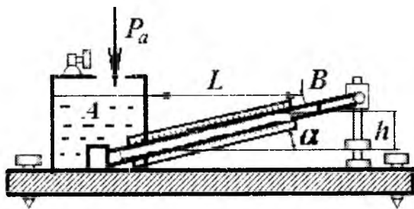
2.26.2-rasm. Mikromanometr
