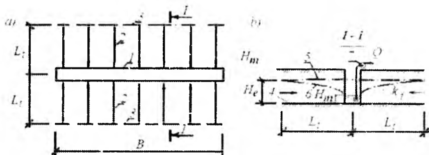
6.2.2. a, b-rasmlar. Chuqurga filtaratsiya. a-reja; b-kundalang kesimi: 1-yauqur, 2-filtaratsiya yunalishi, 3-chegara filtaratsiya maydoni; 4-suv bosimi, 5-issiq suvni tabiiy bosimi, 6-pasaytirilgan tabiiy bosim, 7-nasos.
