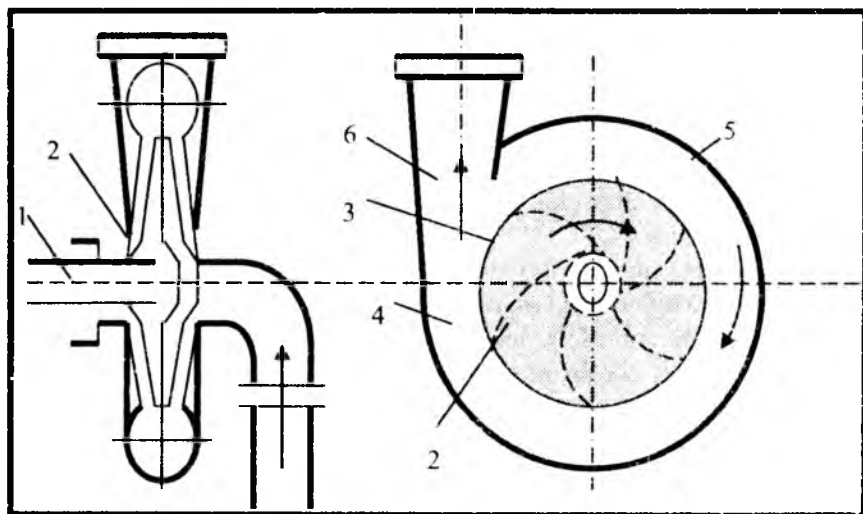
3.4.1-rasm . Markazdan qochma nasos sxemasi.
