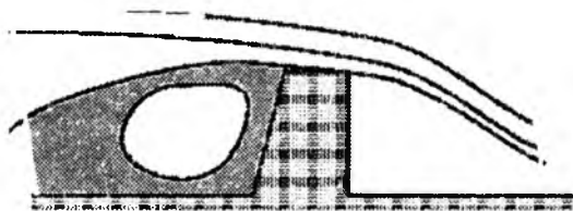
3.8.2-rasm. Suv chiqishi toʻsigʻi ustidan oʻtgan ikki oʻlchamli oqim
