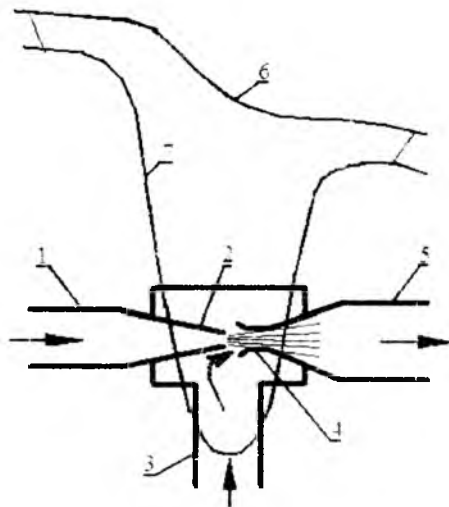
3.16.1-rasm. Oqimchali nasos. 1-suyuqlik haydovchi quvur; 2-saplo; 3-so'ruvchi quvur; 5-uzatuvchi quvur; 6-napor chizig'i; 7-p'ezometrilar chizig'i.
