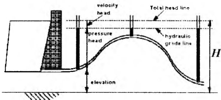
3.14.3-rasm. Suyuqlik o'tayotganda p'ezometr darajalari.
