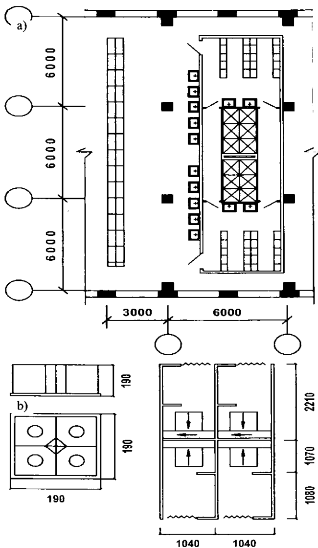
5.5-rasm. Dush xonasining yechimi va jihozlanishiga doir misol: a–zal tizimidagi gardierobda joylashtirish; b–bo'limlarga ajratilgan dush xonachalari.
