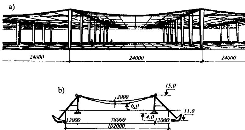
8.14-rasm. Osma konstruksiyalar: a–panelli osma yopmalar; b–panelli tortma tom yopmalar.
