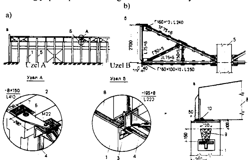
8.20-rasm. Karkas elementlariga tik bog'lamalarni mahkamlash:
