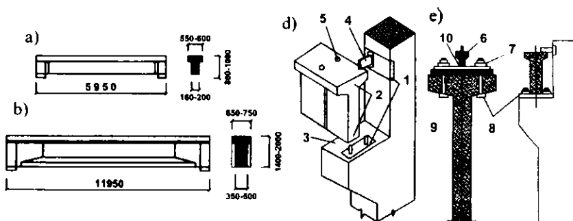
8.4-rasm. Temir-beton kran osti to'sinlari:
