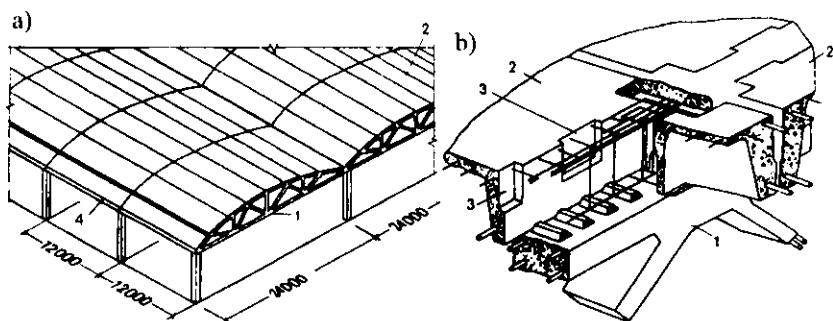
8.11-rasm. Yig'ma temir-betonli qisqa qobiq: a—umumiy ko'rinishi; b—tutashuv tuguni: 1—ferma-diagramma; 2—yopma plita; 3—beton pona; 4—yon element.
