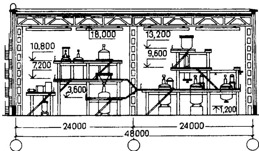
16.7-rasm. Bino ichiga yig'iluvchi-titiluvchi shiypon turidagi javonning qirqimda umumiy ko'rinishi
