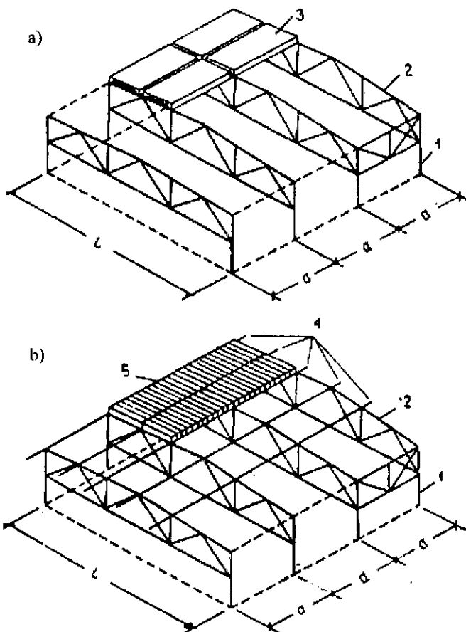
12.2-rasm. Yopmaning to'suvchi qismini konstruktiv sxemasi: a–sarrovtsiz; b–sarrovli: 1–ustun; 2–ferma; 3–yopma plita; 4–sarrov; 5–sarrovdagi o'rnatiladigan kichik o'lchamli plita.
