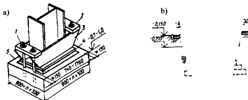
9.4-rasm. Quyma temir-beton poydevor va metalli ustun a–doimiy kesimli; b–ikki shoxli: 1–zulfinli bo' 2–zulfin taxtasi; 3–traversa; 4–tayanch plita; 5–seme 6–ustunning betonlanadigan qismi.
