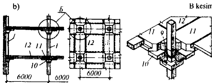
10.3-rasm. Ko'p qavatli sanoat binolari orayopmalarining konstruksiyalari: a—to'sinli orayopma, b—to'sinsiz orayopma: 1—ustun; 2—to'sin; 3—yopma plita; 4—markazlashtiruvchi o'ratma; 5—o'ratma detallar; 6—ustun boshi (ogolovnik); 7—chiqib turuvchi armaturalar; 8—element; 9—birinchi galdagi quyma; 10—kapitel; 11—ustun usti plitasi; 12—oraliq panellari.
