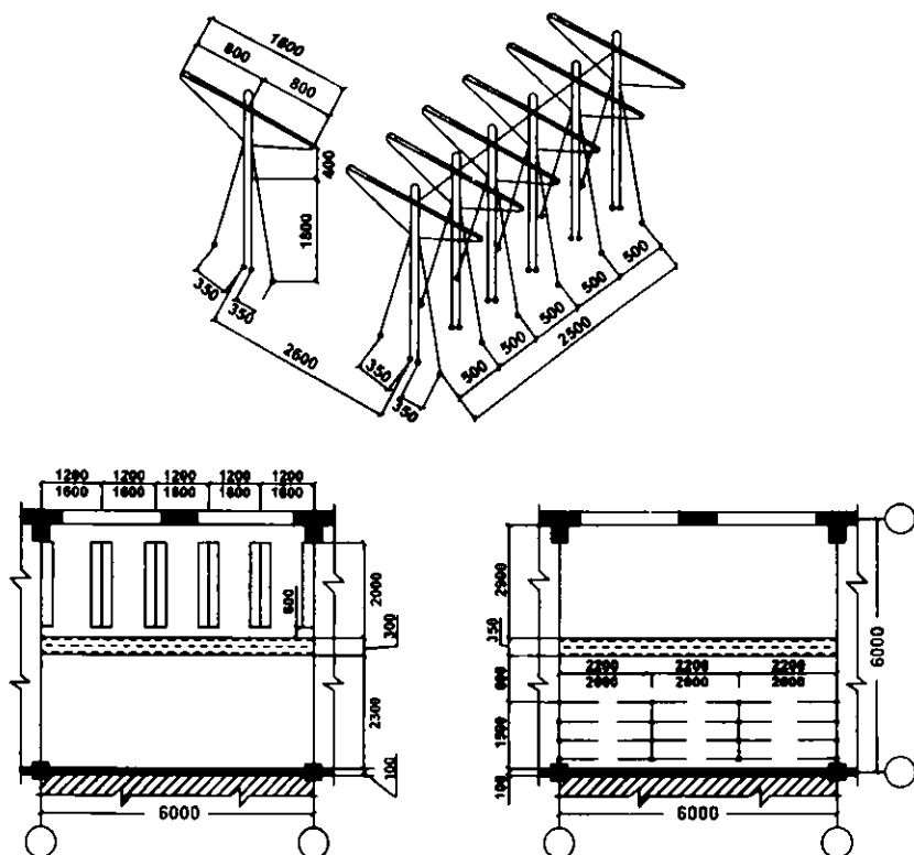
5.4-rasm. Ochiq ilgaklar bilan jihozlangan garderooblar sxemasi.
