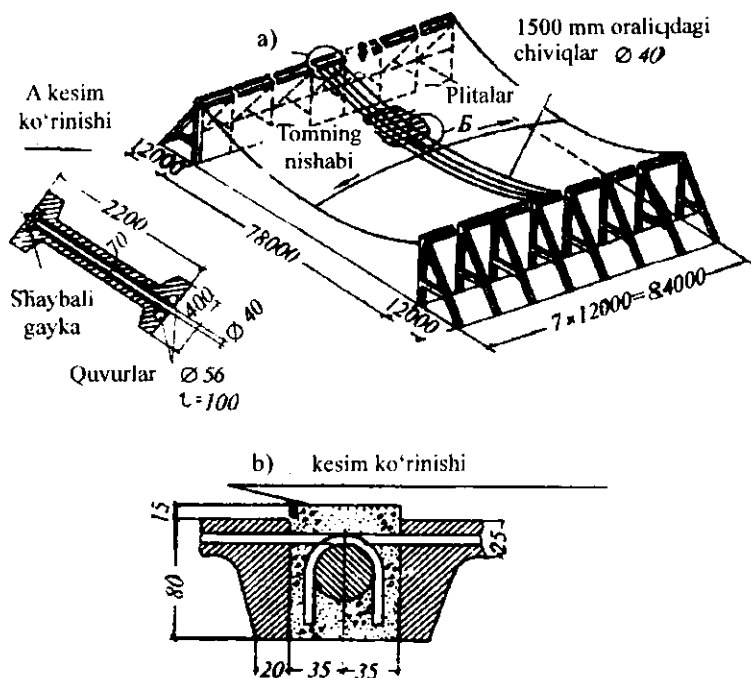
8.15-rasm. Egiluvchan vantali osma temir-beton qobiqlar.
