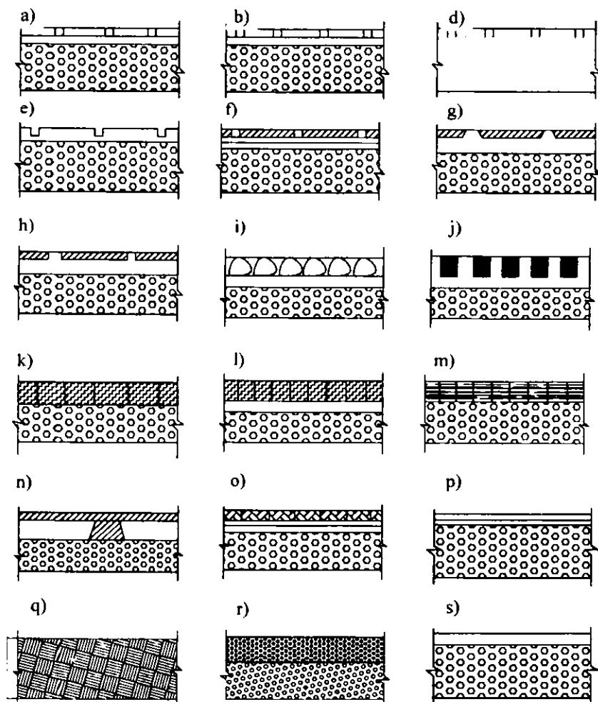
15.1-rasm. Pollarning konstruksiyasi:
