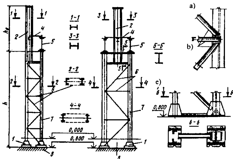
9.3-rasm. Panjarali ustunning sxemasi:
