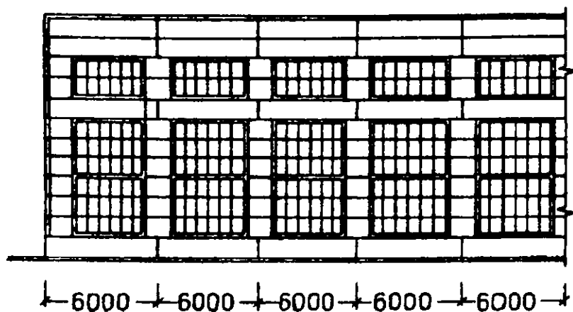
11.10-rasm. Bino devorlarini panellarga kesish sxemasi.
