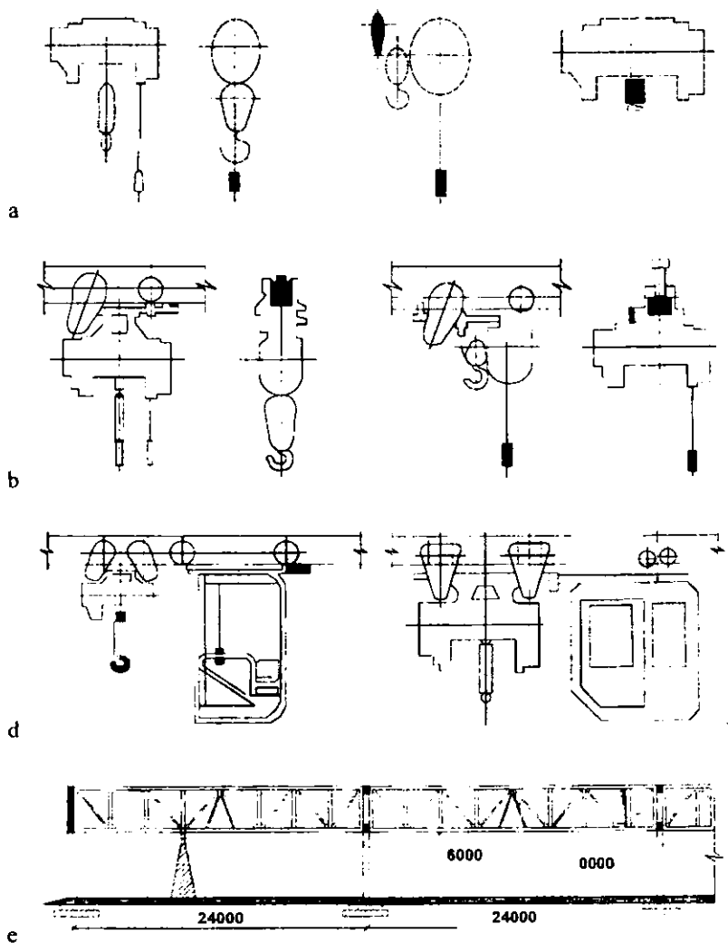
1.3-rasm. Elektr chig'irlar. a—osma ko'chmas; b—o'ziyurar; d—ildirilgan bo'limli; e—harakat bo'limi.
