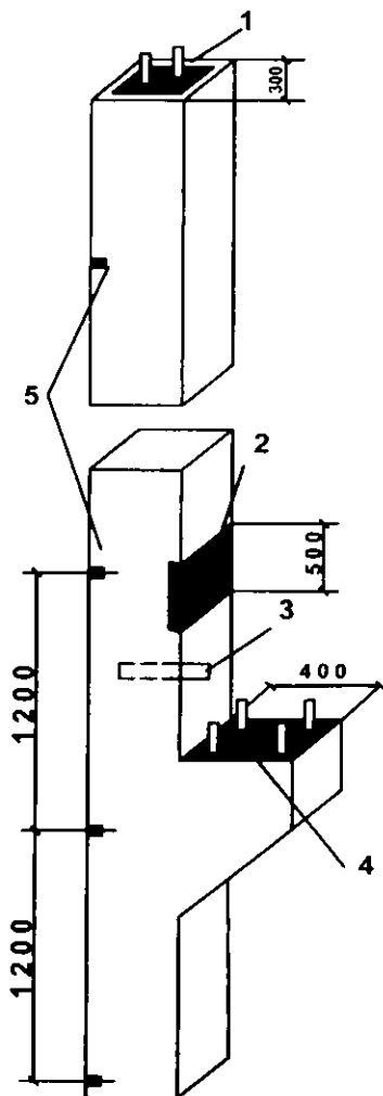
8.2-rasm. Yig'ma temir-beton ustunda po'latli detallarni joylashuvi:
