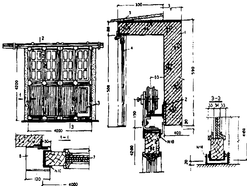
16.4-rasm. Siljivchi darvozalar konstruksiyasi:
