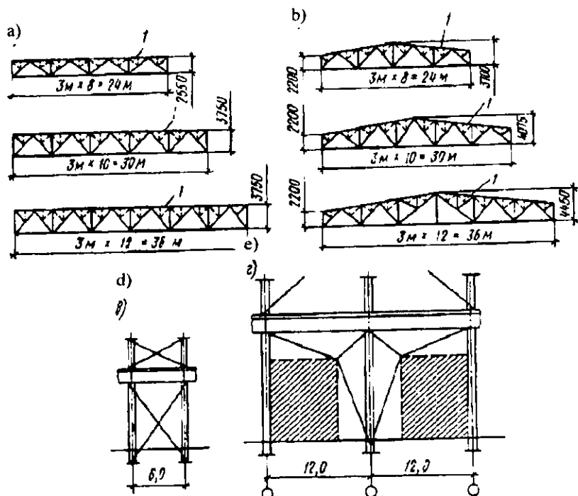
9.7-rasm. Yopmalar fermalarining birxillashtirilgan turlari: a—parallel tasmali ferma; b—ikki nishabli ferma; d—ustunlar orasida o'rnatilgan tik xoch bog'lamalar; e—shunday, portalli.
