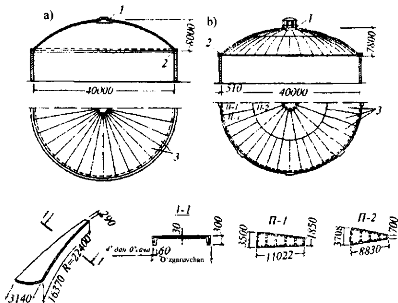
8.13-rasm. Yig'ma temir-betonli gumbaz:
