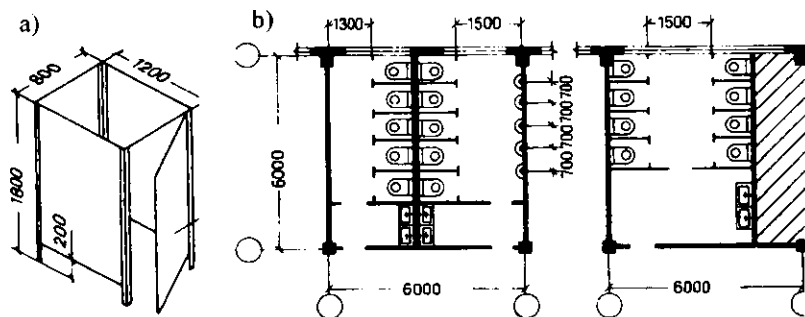
5.8-rasm. Sanitariya tuguni. a—kabina o'Ichamlari, b—rejaviy yechim.
