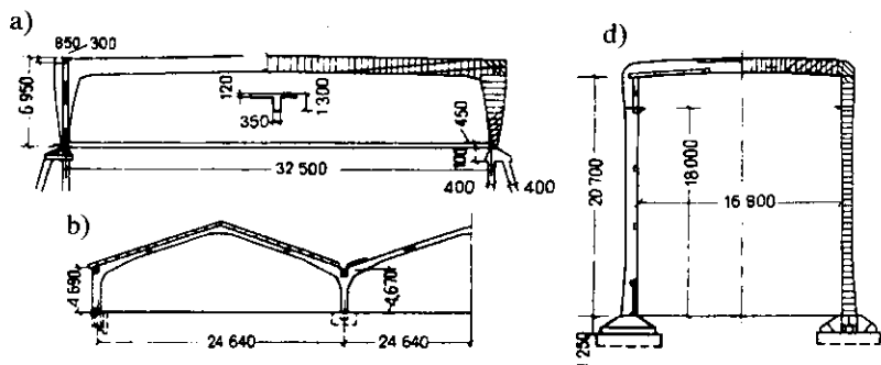
8.9-rasm. Temir-beton ramalar: a, d–bir oraliqli quyma; b–ko'p oraliqli yig'ma.
