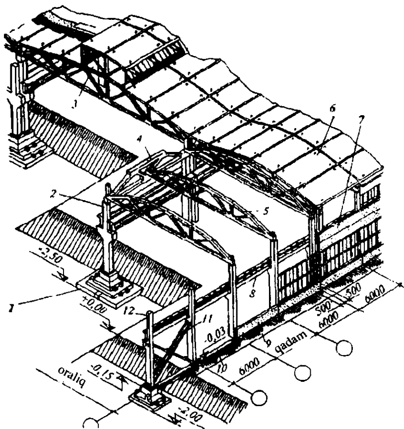
7.1-rasm. Temir-beton karkasli bir qavatli sanoat binosining konstruksiyasi: 1 -ustun osti poydevori; 2-o'rta ustun; 3-fonus; 4-chordoq to'sini osti fermasi; 5-yopma fermasi; 6-yopma plitasi; 7-devor paneli; 8-kran osti to'sini; 9-tashqi devor atrofi to'shamasi; 10-poydevor to'sini; 11-tik bog'lama; 12-chetki ustun.
