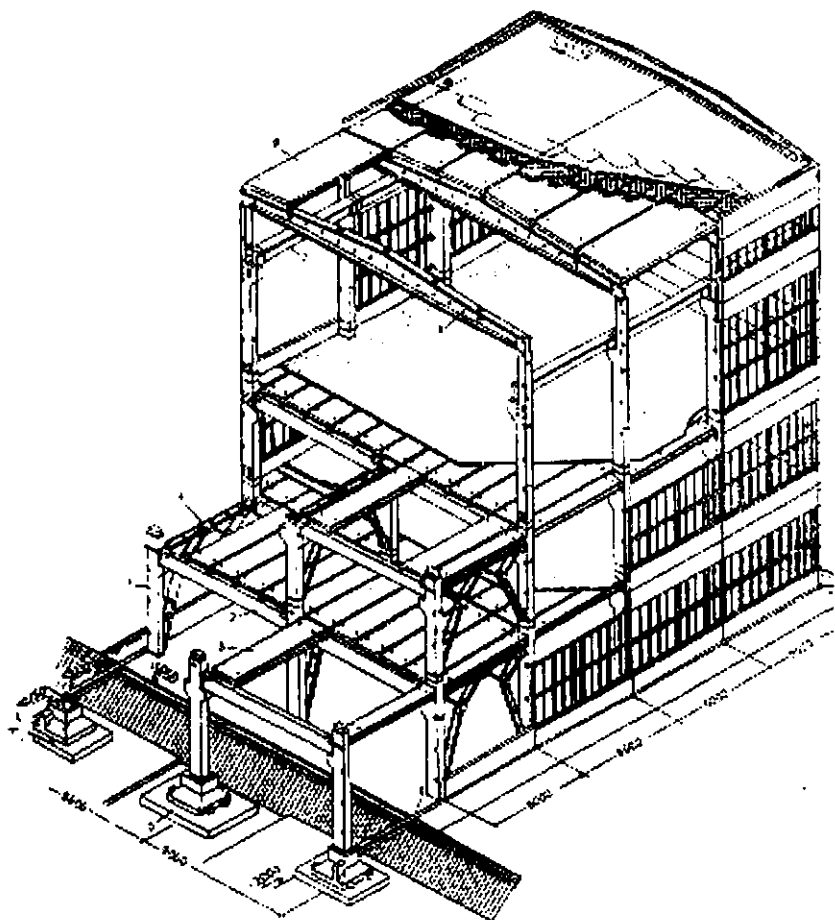
10.1-rasm. Yopmalari to'sinli konstruksiyada bajarilgan ko'p qavatli sanoat binosining yig'ma temir-beton karkasi:
