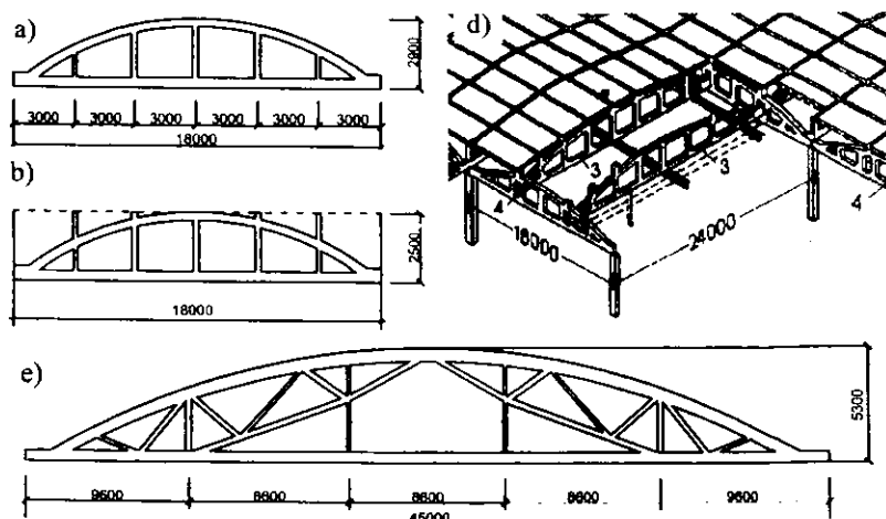
8.7-rasm. Yig'ma temir-beton fermalar: a—nishabli yopmasi bo'lgan binolar uchun; b—yassi tomli binolar uchun; d—yopmaning umumiy ko'rinishi; e—ikkita yarim fermadan iborat ravoq; 1—qo'shimcha ustuncha; 2—yopma plita; 3—chordoqli ferma; 4—chordoq osti fermasi.
