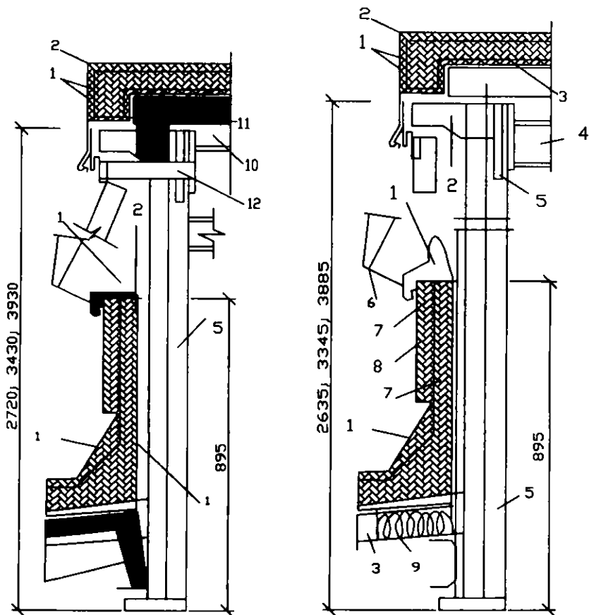
13.4- rasm. To'g'ri to'rtburchakli yorug'lik-aeratsiya fonarining detallari: a- va b-po'lat kesim (profil) va temir-beton to'shamalardan tayyorlangan tomda: 1-ruxlangan krovli po'lati; 2-shveller; 3-profillangan to'shama; 4-fonus karkasi; 5-fonus paneli; 6-tavaqa; 7-yog'och g'o'lacha; 8-to'lqinli po'lat tunuka; 9-yong'inga qarshi to'siq; 10-temir-betonli plita; 11-karnizli panel; 12-mahkamlovchi zulfín.
