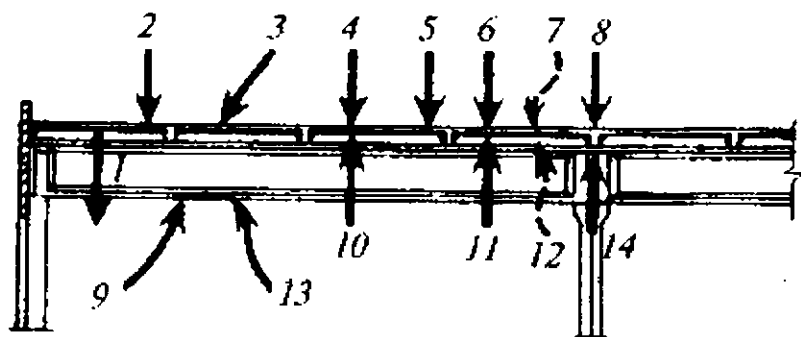
12.1-rasm. Yopmaga tashqi ta'sirlar:
