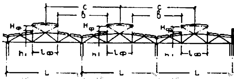
13.2-rasm. Fonar va bino o'lchamlari orasidagi o'zaro bog'liqlikka doir
