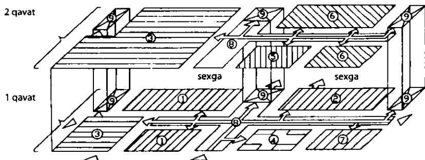
5. 1-rasm. Sexga tutash qurilgan yordamchi binoning funksional bo'limlarga bo'lish sxemasi: 1—erkaklar maishiy xonalari; 2—ayollar maishiy xonalari; 3—oshxona; 4—meditsina punkti; 5—muhandis-texnik xodimlar xonalari; 6—konstruktorlik byurosi, o'quv mashg'ulotlari va jamoat tashkilotlari xonalari; 7—madaniy xizmat xonalari; 8—garderoblar; 9—zinalar.
