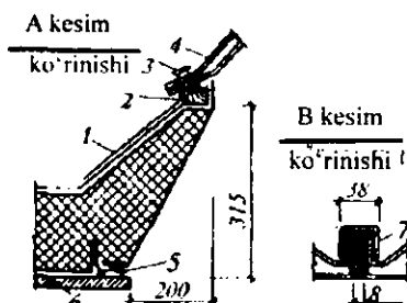
13.5-rasm. Gumbaz (zenatli) li fonartar:
