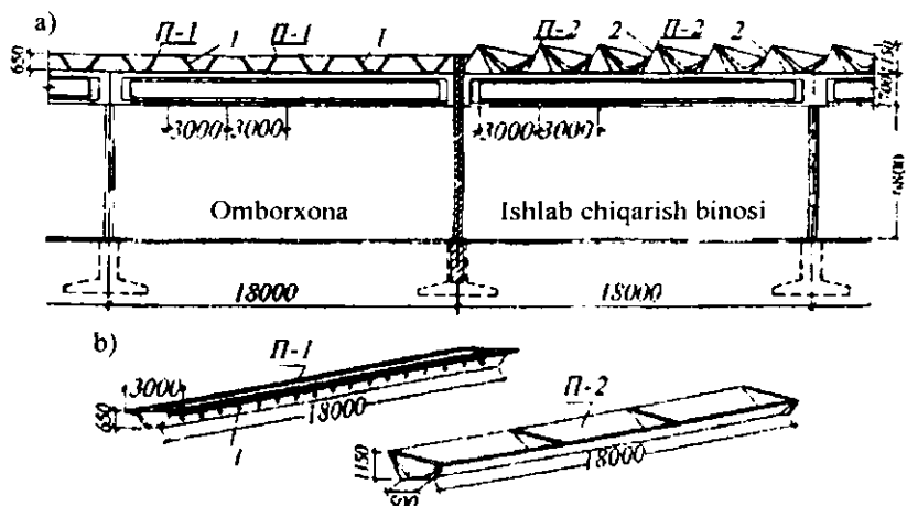
8.12-rasm. Buklangan yopmalar: a—ko'ndalang qirg'im; b—yig'ma elementlar; П-1—buklama elementi; 1—aylana deraza; П-2—buklama element; 2—qiya shishalangan.
