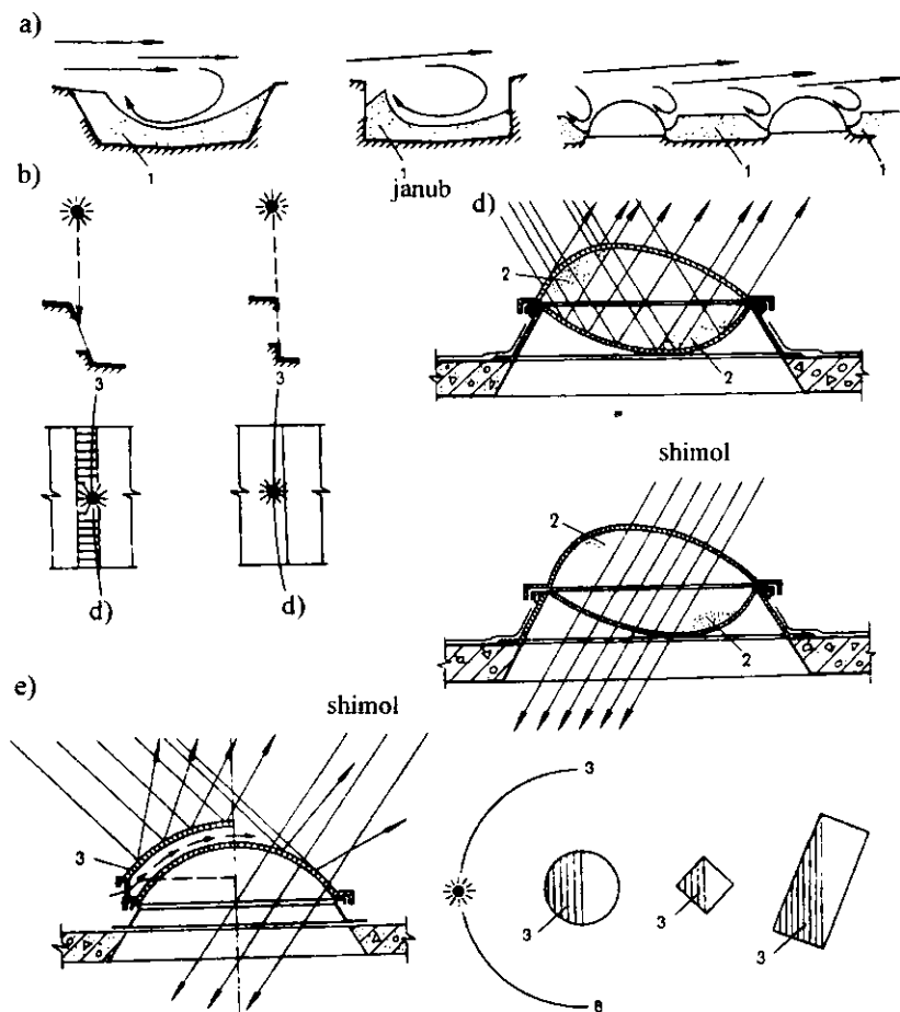
13.3-rasm. Binolarning yorug'lik fonarlariga doir:
