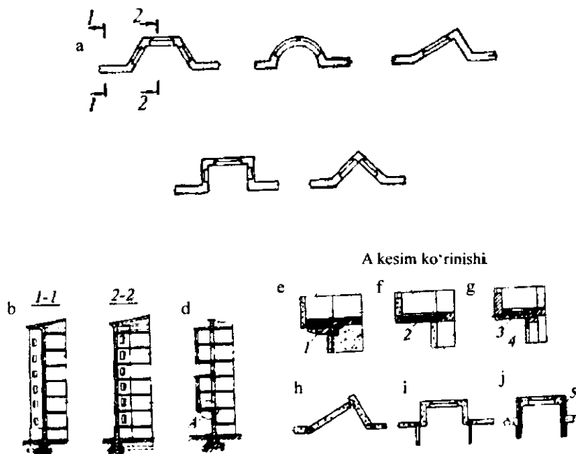
15.3-rasm. Erkerlar: a—erkerning rejadagi shakllari; b—yuk ko'taruvchi devorli; d—osma; e—panelli binoda ichki devor konsollariga tayanadigan osma; f—g'ishtli binoda ichki devor konsollariga tayanadigan osma; g—keramzitbeton plitaga tayanadigan osma; h—panelli; i—hajmiy elementli erker; j—hajmiy blokli binolarda erkerni ko'rnatish; 1—ichki panel devorning temir-beton konsoli; 2—orayopma konsoli; 3—erkerning keramzit-beton plita konsoli; 4—deraza bo'shlig'ining to'sig'i; 5—issiq qatlamli panel
