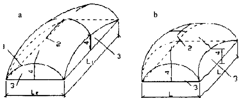
26.4-rasm. Ikkilamchi musbat qiyshilikka ega bo'lgan qobiqlarning chizmalari: a-rejada to'g'ri burchak; b-rejada kvadrat shaklda (to'rt yelkanli toq); 1-hosil qiluvchi egri chiziq; 2-yo'naltiruvchi egri chiziq; 3-diafragma; 4-ko'tarilish o'qi
