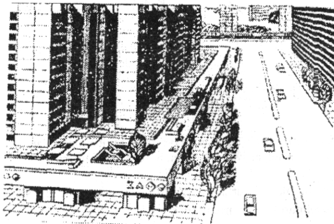
8.3- rasm . Magistral yo‘l yoqasida shovqinga qarshi mo‘ljallangan turar-joy binosini joylashtirish
