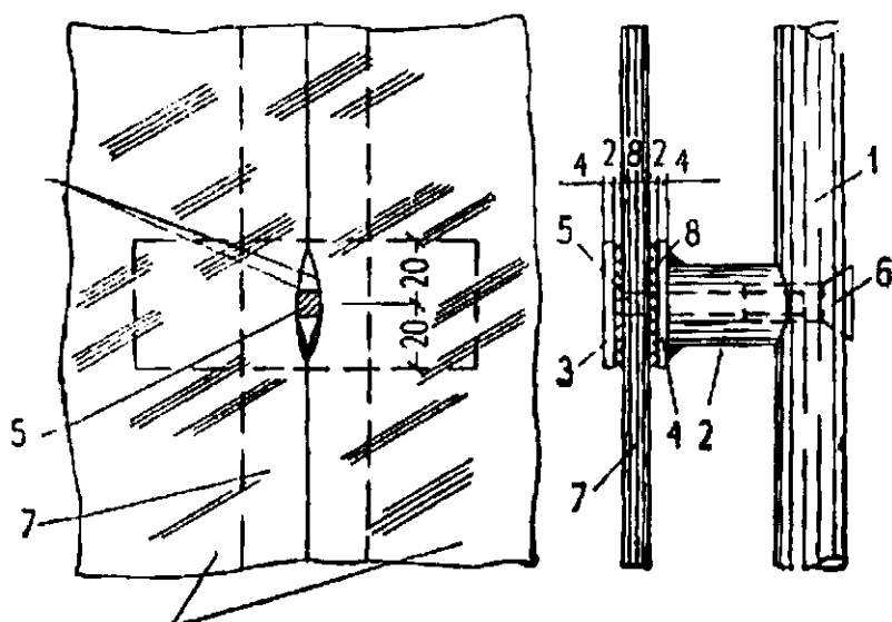
30.7-rasm. Vitrina oylarini profilsiz birlashtirishga misol 1—ustun; 2—mufta; 3—qisqichlar; 4—nakladka; 5—mix; 6—rezbalı mufta; 7- sillıqlangan oyna (b=8mm); 8—rezinalı prokladka
