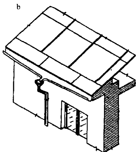
17.12-rasm. Tomlardan suvlarni qochirish uchun tarnoqlar: a—devorga yopishgan holda; b—osma
