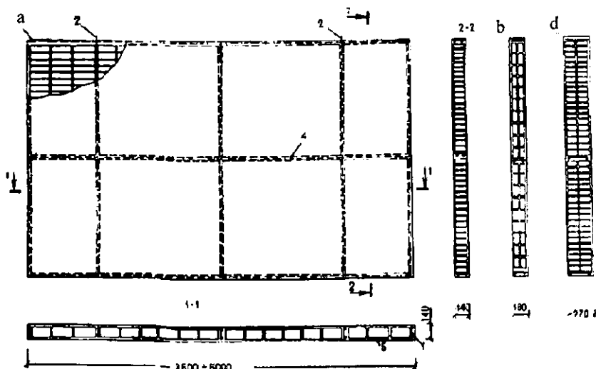
18.3-rasm. Ichki devorlar uchun g'isht panellar:
