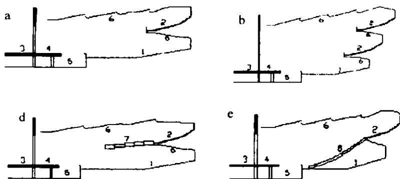
21.8-rasm. Teatrlar zallarining qirgimdagi sxemalari: a–amfiteatrli va balkonli; b–bal- konlari ikki yarusli; d–yon tomondan zina shaklidagi balkonlar; e–amfiteatr shaklidagi balkonlar; 1–amfiteatr; 2–balkon; 3–sahna; 4–avansahna; 5–orkestr; 6–osma shift; 7–yon balkon; 8–amfiteatr shaklidagi yon balkon
