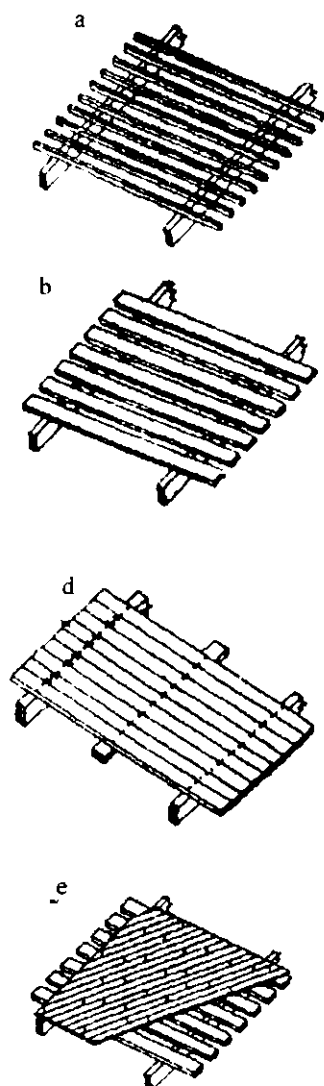
17.7-rasm. Tayyorlangan yog'och panjaralar: a-brusoklardan; b-taxtalardan; d-yaxlit; e-ikki qatlamli yaxlit
