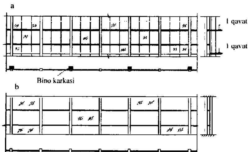
30.1-rasm. Vitrajlarining sxemalari: a-qavat tom konstruksiyalariga birlashtirilgan; b-tom va sokol konstruksiyalariga birlashtirilgan
