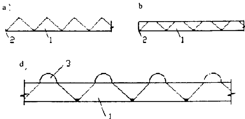
26.3-rasm. Burma konstruksiyalarning chizmalari:
