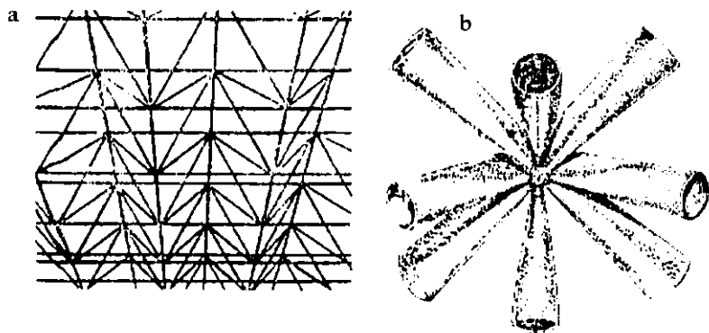
25.8-rasm. Trubkali sterjenlardan tashkil topgan kesishgan konstruksiylar: a–umumiy ko'rinish; b–tugun
