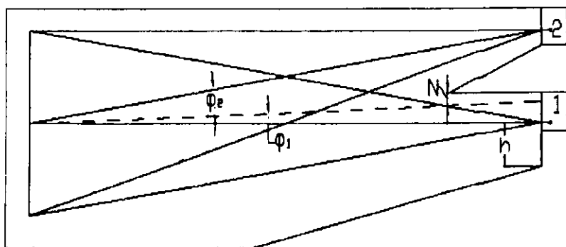
22.11-rasm. Kinoproyeksion xonalarning joylashtirish sxemalari 1–balkon ostida; \varphi_1 –30° dan ko'p emas; 2–balkon ostida; \varphi_2 –60° dan ko'p emas; N–balkon osti chizigidan nurgacha bo'lgan masofa 0,5 m dan kam bo'lmاسligi kerak; h–1,9 m dan kam bo'lmاسligi kerak
