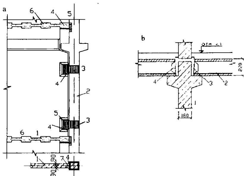
24.5-rasm. Bog'lovchi devor: a—bog'lovchi devorlarning ustunlar bilan birlashtirilishi; b—tom konstruksiyasi; 1—bog'lovchi devorlar; 2—ustun va yopma konstruksiyasi; 3—beton bilan to'ldirish; 4—tom konstruksiyalari bo'shliqlarini to'ldirish; 5—payvandlash; 6—quyma beton (shponka); 7—armaturani diafragmadan chiqarish
