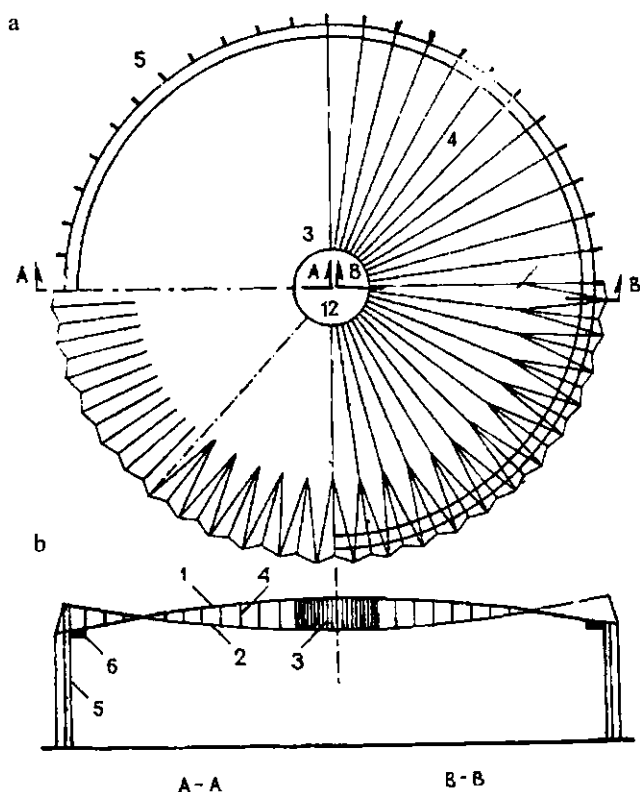
28.10-rasm. Sport saroyi ikki belbog'li osma tomining reja sxemasi va qirqimi: a—reja; b—qirqim; 1—yuqoridagi tros­lar; 2—pastki tros­lar; 3 markaziy halqa; 4—itaruvchi ustunchalar; 5—ustunlar; 6—tashqi kontur halqasi
