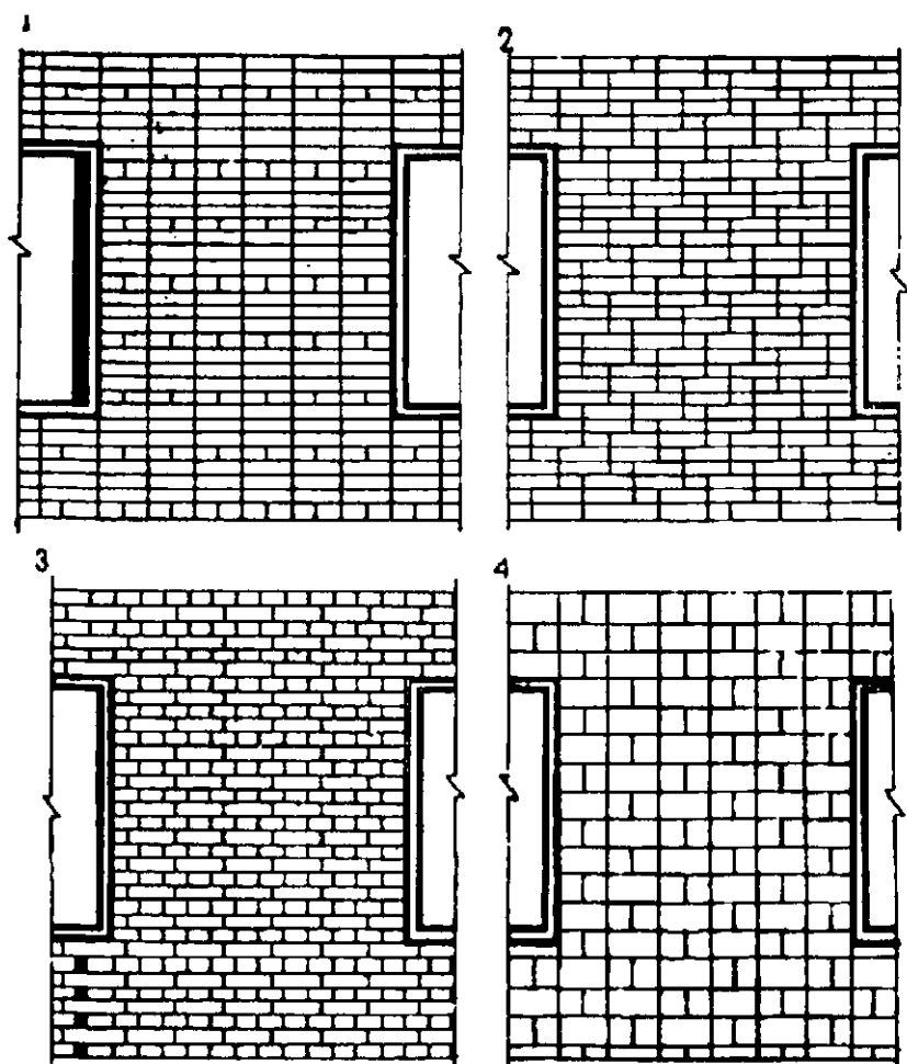
13.7-rasm. Fasad devorlarining dekorativ qoplashga misollar: 1–3- g'ishtli qoplama; 4–sopol blokli qoplama
