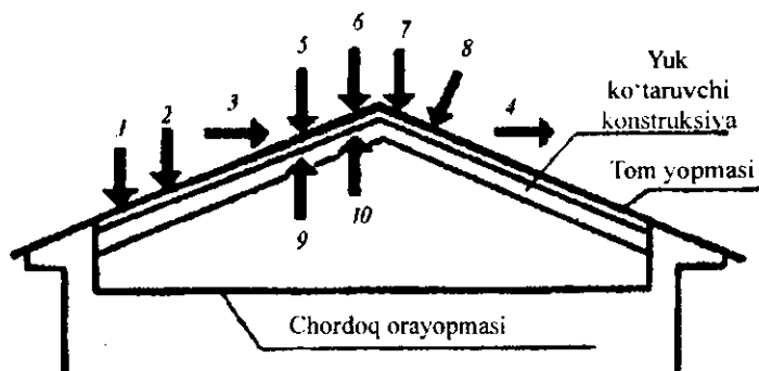
16.1-rasm. Tomga ta'sir qiluvchi tashqi faktorlar:
