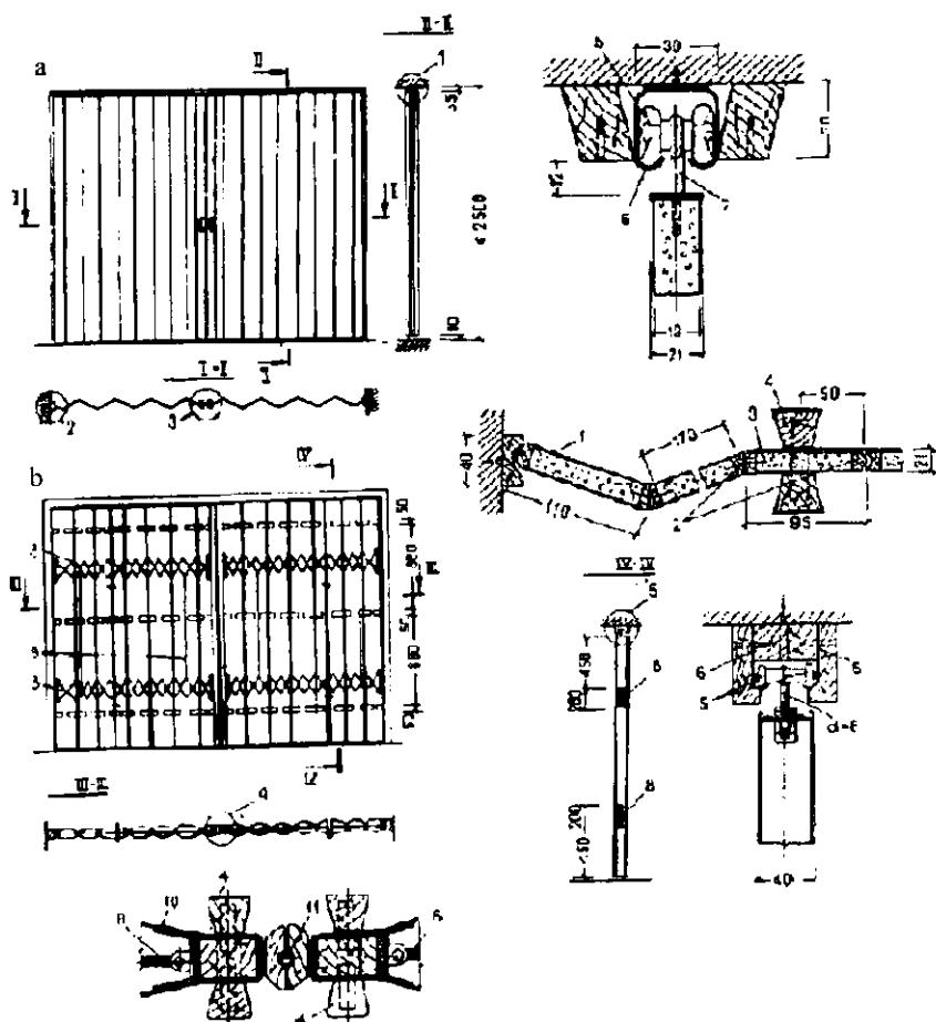
18.5-rasm. Suriluvchi pardevorlar:
