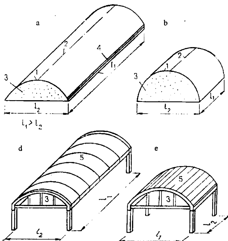
26.1-rasm. Silindrik temir-beton qobiqlar:
