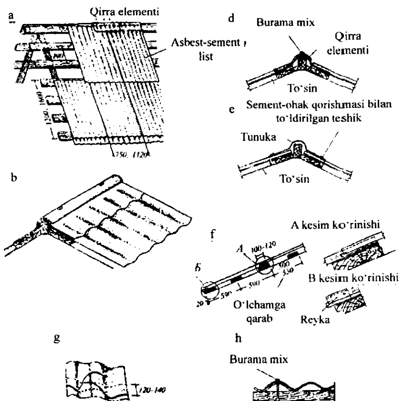
17.10-rasm. To'liqinsimon asbestosement listlardan yopilgan chordoqli tom: a–umumiy ko'rinish; b, d, e–qirraning yopmasi; f–birikmalar; g–varaqlarni bir-biriga minish sxemasi; h–panjaraga qotirish
