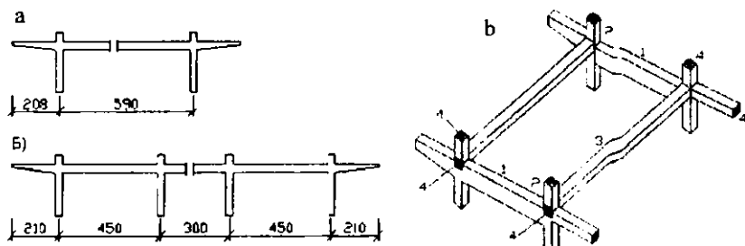
24.10-rasm. Xojli elementlardan boʻlgan ramali karkasning chizmasi: a–ikki konsolli elementlardan; b–konsolli N shaklli elementlardan; d–N shaklli elementli karkas fragmenti; 1–rigel; 2–ustun; 3–bogʻlovchi balka; 4–rigel bilan bogʻlash uchun ulanish elementi.
