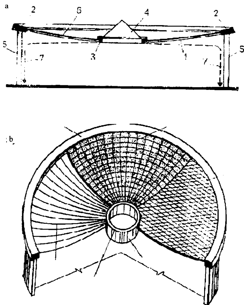
28.7-rasm. Bir belbog'li osma tom sxemasi: a–qirqim; b–aksonometriya; 1–po'lat troslar; 2–temir-beton tayanch halqa kontur; 3–markaziy po'lat tayanch halqa; 4–fonar (yorug'lik yoki aeratsion); 5–ustunlar; 6–himoya konstruksiyasi; 7–ichki tashkillashtirilgan suv qochirish quvuri.
