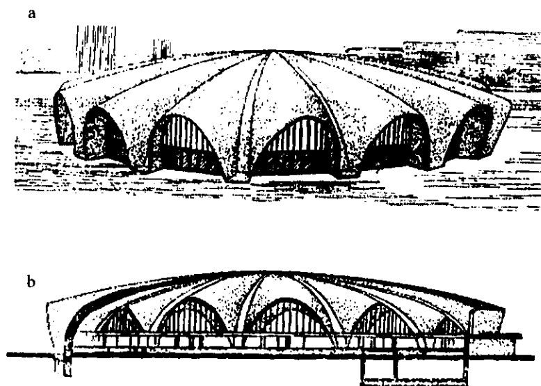
27.9-rasm. Bozor ustidagi to'liqinli gumbaz: a-umumiy ko'rinishi; b-qirqimi
