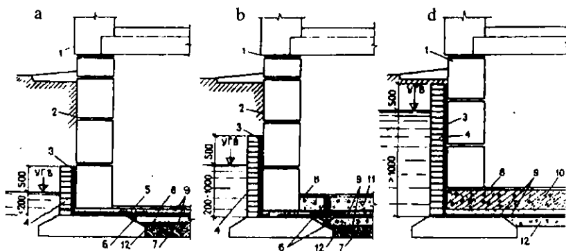
12.4-rasm. Poydevorlar gidroizolyatsiyasi:
