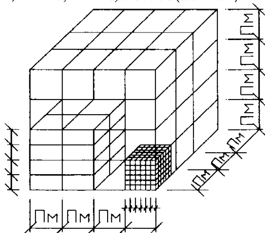
2.1- rasm. Modul tekisliklarining samoviy sistemasi:
