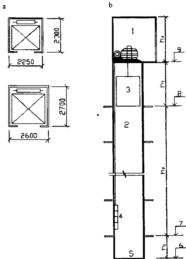
22.13-rasm. Lift shaxtalari va kabinolari:
