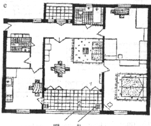
7.7-rasm. Xonadonlar planirovkalariga doir misollar: d—galereya tipidagi uydagi xonadon; e—uch xonali devorlari transformatsiya bo'ladigan kvartira
