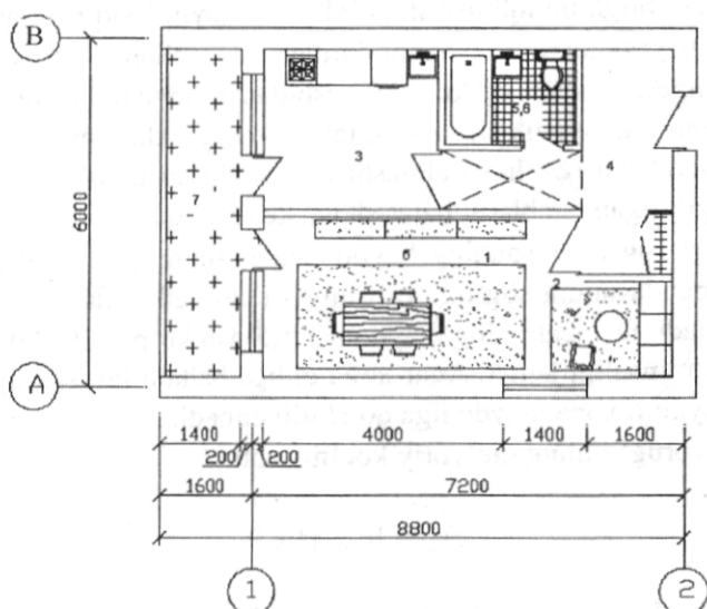
6.11 - rasm. Kvartirani zonalarga (guruhlariga) bo'lish sxemasi:
