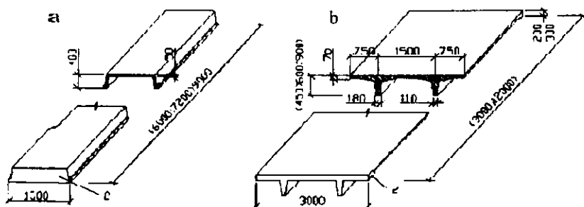
24.8-rasm. Plitalarning ko'rinishlari: A - qovurg'ali plita; B - plita T-T; 1- uzunligi bo'yicha qovurg'a; 2-yon qovurg'a.
