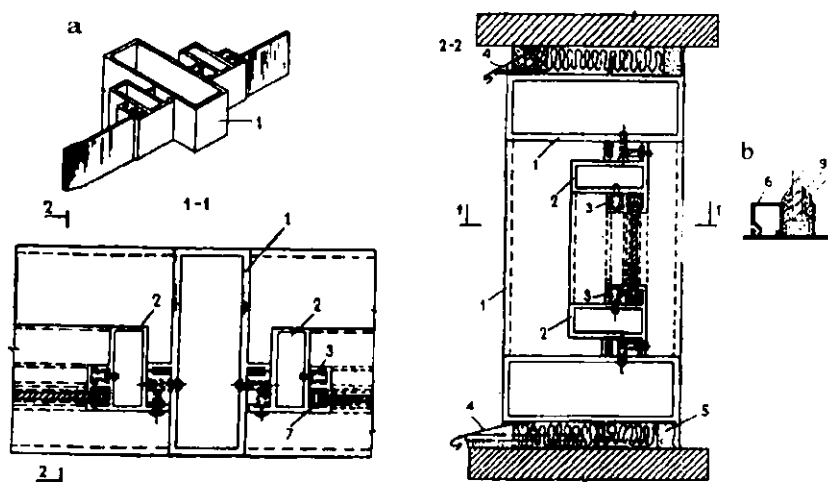
14.3-rasm. Vitrajning konstruksiyasi: a—aluminiy aralashmalaridan tayyorlangan yuk ko'taruvchining konstruksiyalari va tabaqalari; b—shishani qotirish elementi: 1—impost; 2—tabaqa; 3—prujinali shtapik; 4—metalldan yasalgan suvqochirgich; 5—qorishma; 6—qistirgichli shtapik; 7—rezina qistirgich; 8—PRV-1 arkali rezina; 9—germetik.
