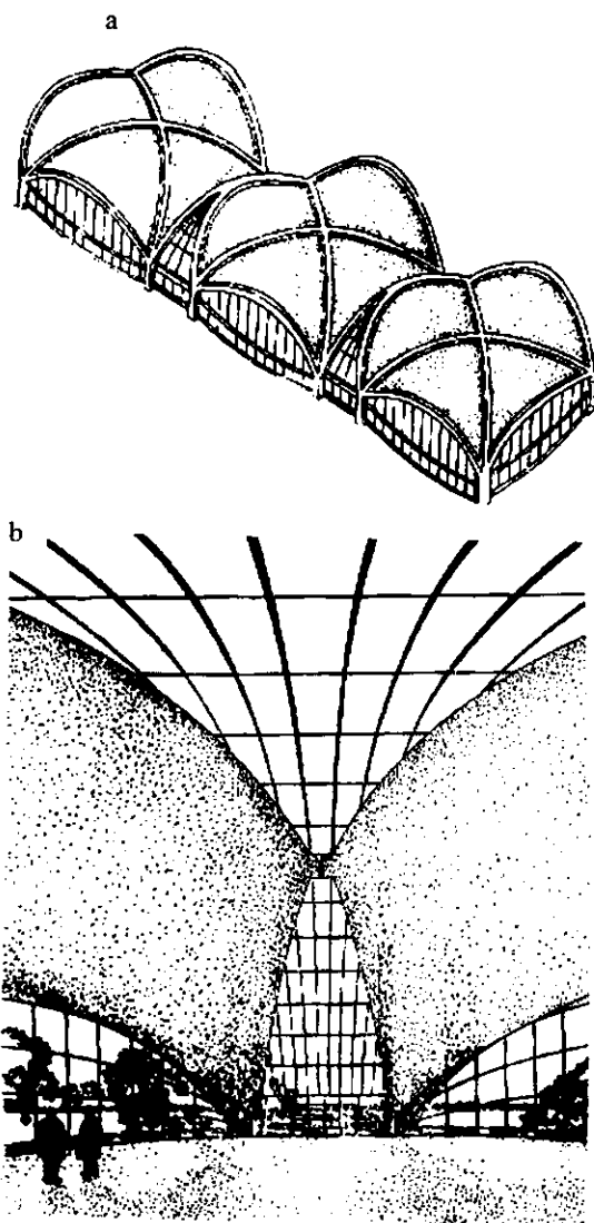
26.8-rasm. San-Luizdagi aerovokzal. Xojli qobiqlar: a–aksonometriya; b–interer
