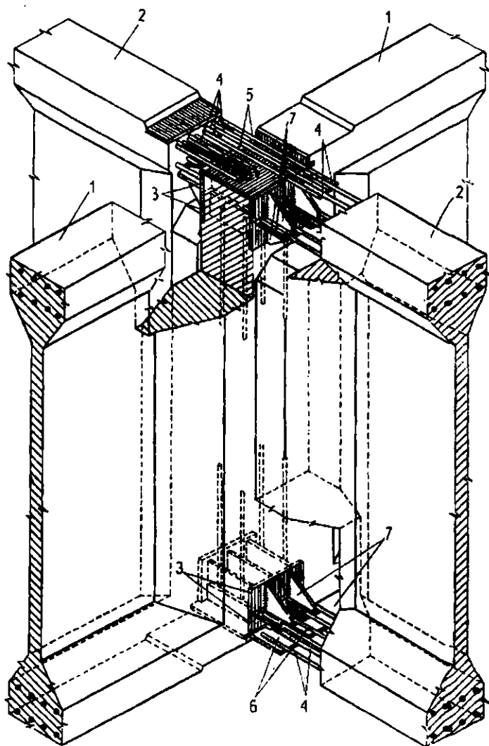
25.9-rasm. Kesishgan temir-beton balkalarning ulanishi: 1-butun balka; 2-ulanuvchi; 3-butun balkaning ulanish detali; 4-ulanuvchi balkalarning armaturalari; 5, 6, 7-birlashtiruvchi sterjenlar, nakladkalar va kosinkalar
