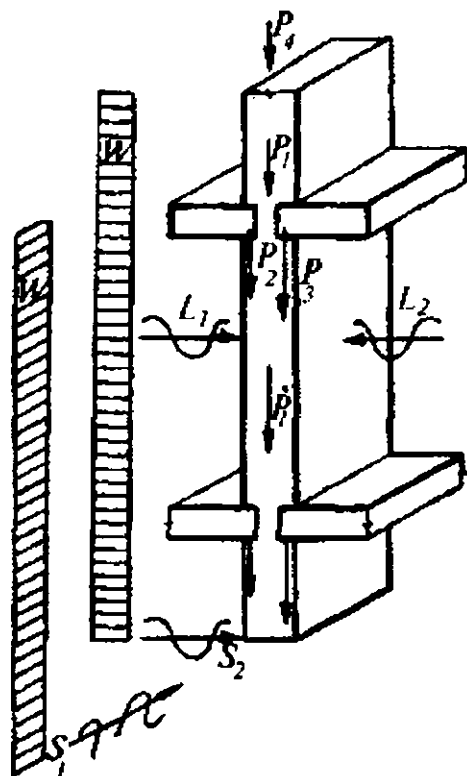
18.1-rasm. Ichki devor konstruksiyalariga tushadigan yuklar va ta'sirlar: R_1 —ichki devor massasi; R_2 , R_3 —orayopmalardan tushadigan vertikal yuklar; R_4 —tom yopmalaridan tushadigan vertikal yuklar; W —shamol bosimi; L_1 , L_2 —havo shovqini; S_1 , S_2 —zilzilaviy ta'sirlar
