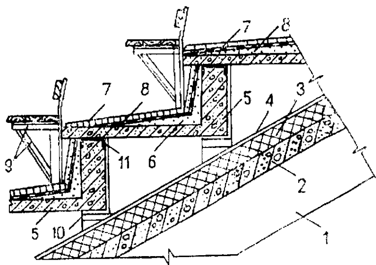
29.5-rasm. Zina konstruksiyasining detallari.
