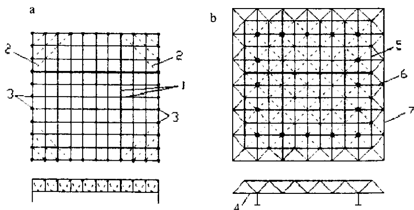
25.7-rasm. Tomlarning kesishgan konstruktiv tizimlari chizmasi:
