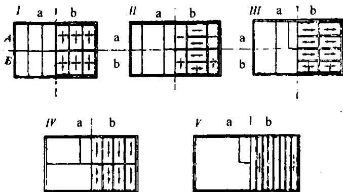
10.5-rasm. Karkassiz binolarning konstruktiv sxemalari. I kesishgan-devorli; II va III ko'ndalang-devorli; IV va V bo'ylama-devorli; a-yuk ko'tarmaydigan yoki o'z-o'zini ko'taradigan bo'ylama devorli variantlar; b-shuni o'zi, faqat yuk ko'taruvchi devorlar bilan; d-devorlar rejasi; e-tom rejasi
