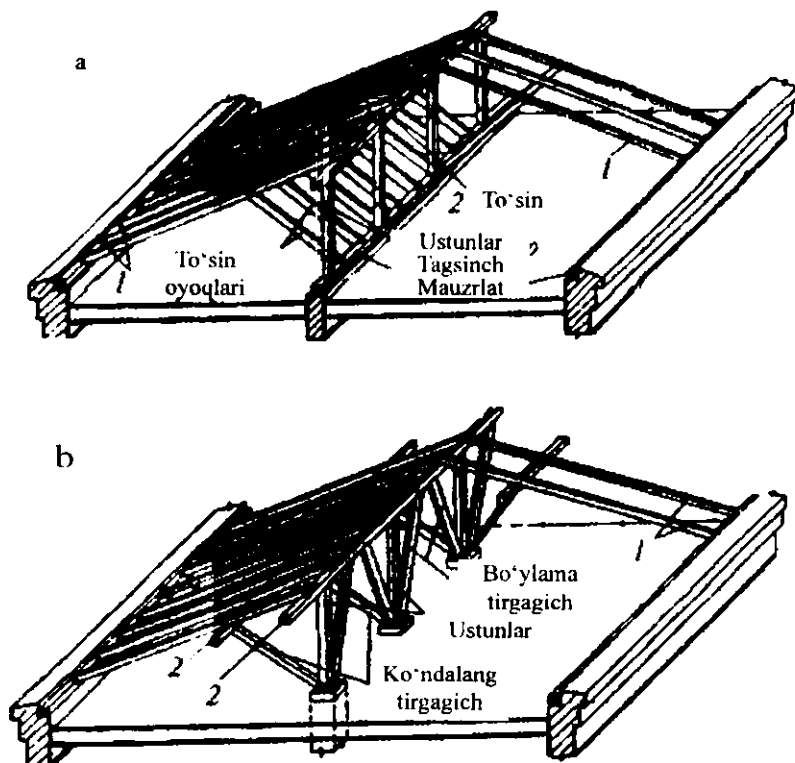
17.1- rasm. Qiya tayanuvchi chordoq to'sinlari: a-bo'ylama ichki devorga tayanish; b-xuddi shunday, ustunlarga
