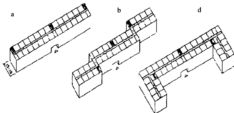
22.1-rasm. O'rta koridorli jamoat binolarining hajm-rejaviy yechimlari: a—to'g'ri to'rtburchakli, b—zinasion; d—П shaklidagi
