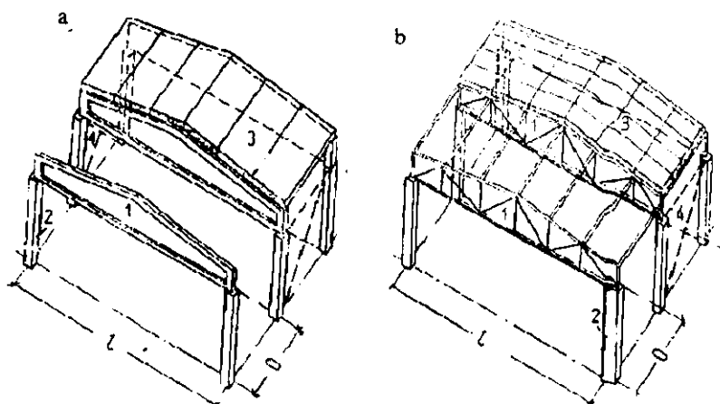
25.1-rasm. Yassi ko'tarma konstruksiyali zal xonarining tom sxemalari:
