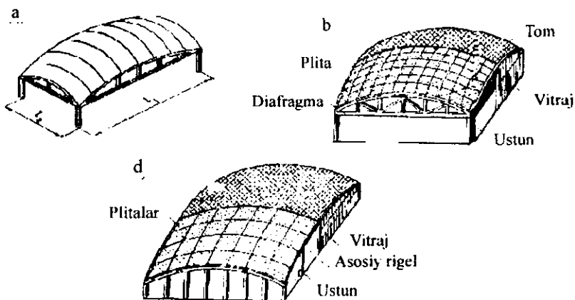
26.5-rasm. Ikkilamchi musbat egrilikka ega bo'lgan yig'ma qobiq: a-fermalar ko'rinishidagi diafragmalar bilan hamda egri chiziqli yig'ma elementlar bilan; b-konturli egri chiziqlar chiziqli rigellar bilan
