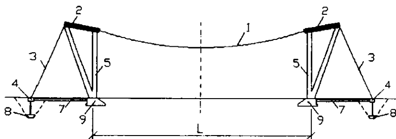
28.2-rasm. Tortmali osma tom sxemasi:
