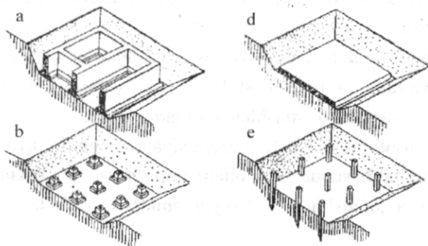
12.3-rasm. Poydevorlar konstruktiv sxemalari:
