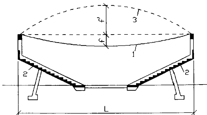
28.1- rasm. Tomlarni taqqoslash sxemasi: 1–osma tom; 2–temir-beton konsol ramasi; 3–qobiq
