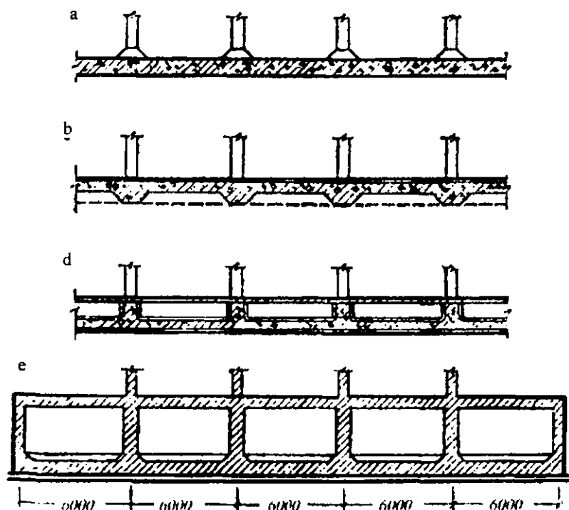
12.8-rasm. Yaxlit poydevor plitalari:
