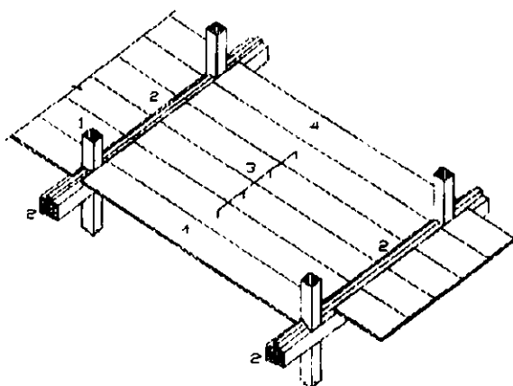
24.9-rasm. Tom konstruksiyalarini joylashtirish sxemasi: 1-ustun; 2-rigel; 3-panel; 4-panel-bog'lovchi element
