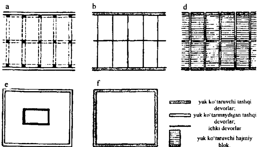
10.2-rasm. Asosiy konstruktiv sistemalar:
