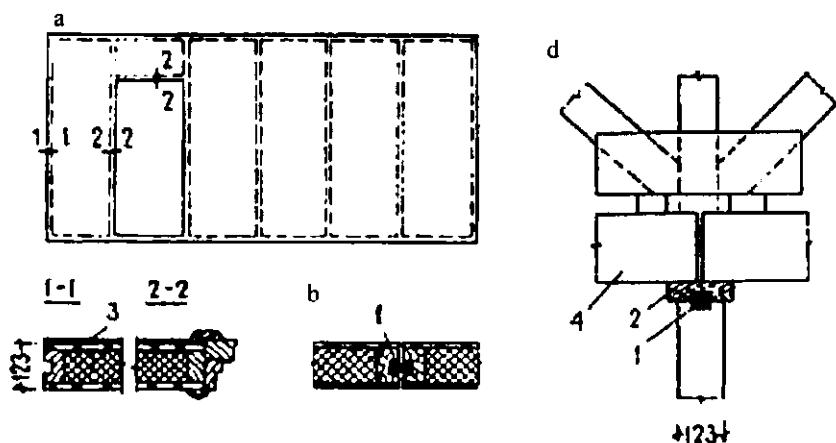
18.2-rasm. Yog'och panellardan bajarilgan pardevorlar: a—panel fasadi; b—oddiy vertikal birikish; d—chordoq tomi paneli bilan gorizontal birikish; 1—birikish reykasi; 2—gorizontal ulama; 3—namligi baland xona tomonidan suv o'tkazmaydigan qo'shimcha qatlam; 4—chordoq orayopma paneli
