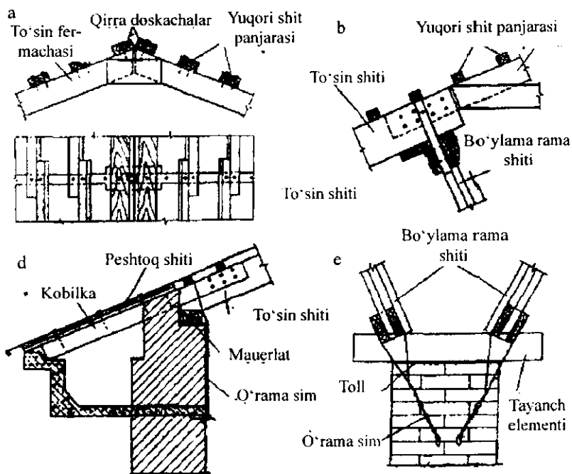
i7.4-rasm. Yig'ma chordoq to'sinlarining detallari: a—qirra birikmasi; b—to'sin shaklining to'sin shitiga tayanishi; d—peshtoq shiti; e—o'rta tayanch birikmasi
