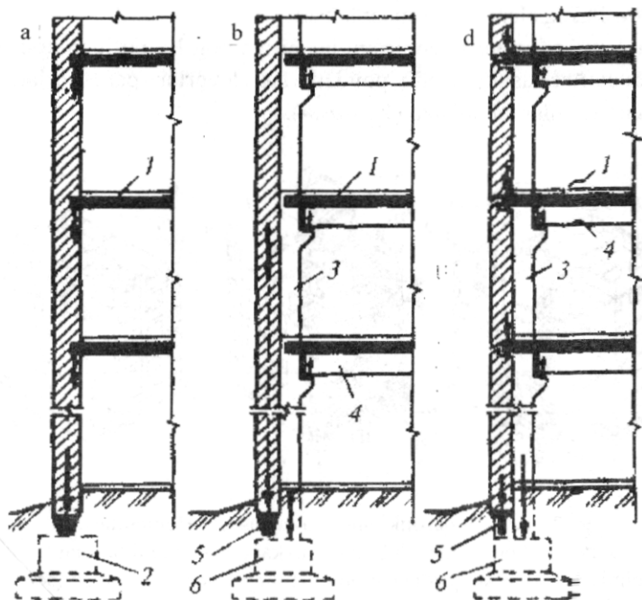
9.3-rasm. Tashqi devor turlari:
