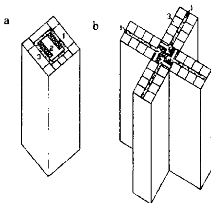
22.4-rasm. Baland qavatli jamoat binolarining hajm-rejaviy yechimlari: a–kvadrat shaklida; b–xo'j shaklida; 1–koridor; 2–vertikal kommunikatsiyalar; 3–asosiy xonalar
