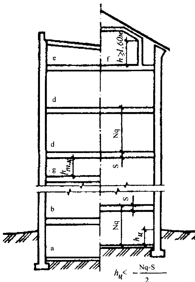
9.1-rasm. Bino qavatlarining joylashuvi: a—yerto'la; b—poypesh qavati; d—yer yuzasida joylashgan qavat; e—chordiq qavati; f—mansarda; g—texnik qavat
