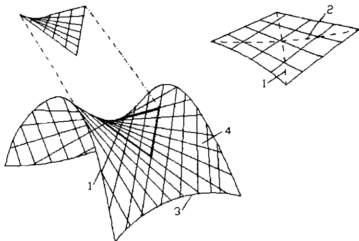
26.9-rasm. Egar shaklidagi gipar sxemasi:
