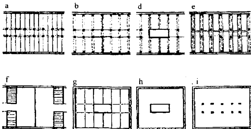
10.3-rasm. Aralash konstruktiv sistemalar:
