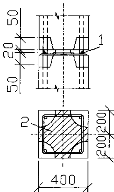
24.3-rasm. Temir-beton ustunlarning «quruq bogʻlanish» usuli:
