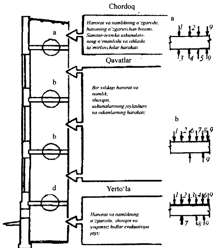
19.1-rasm. Orayopmalarga yuklardan tushuvchi va tashqi muhit ta'sirlari
