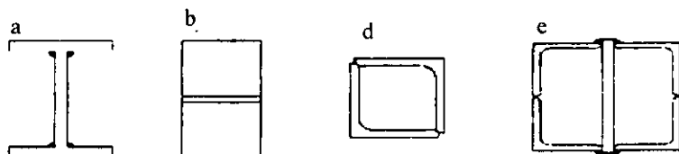
24.4-rasm. Po'lat karkaslar ustunlari: a, b—tasmali po'latdan; d, e—burchakliklardan
