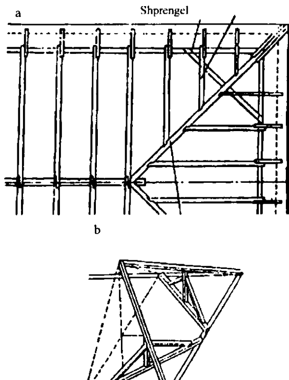
17.6-rasm. «Valma» tipidagi chordoq to'sinining konstruksiyasi: a—reja; b—umumiy ko'rinish
