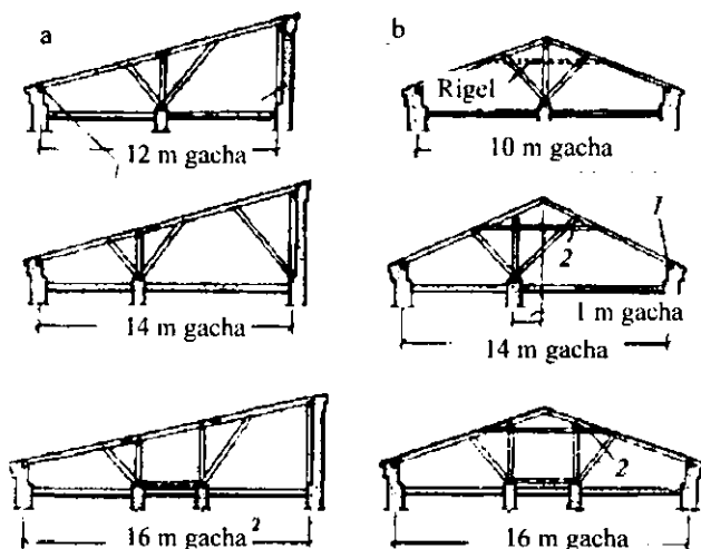
16.3-rasm. Yog'ochli qiya tayanuvchi – stropila to'sinlarning sxemalari:
