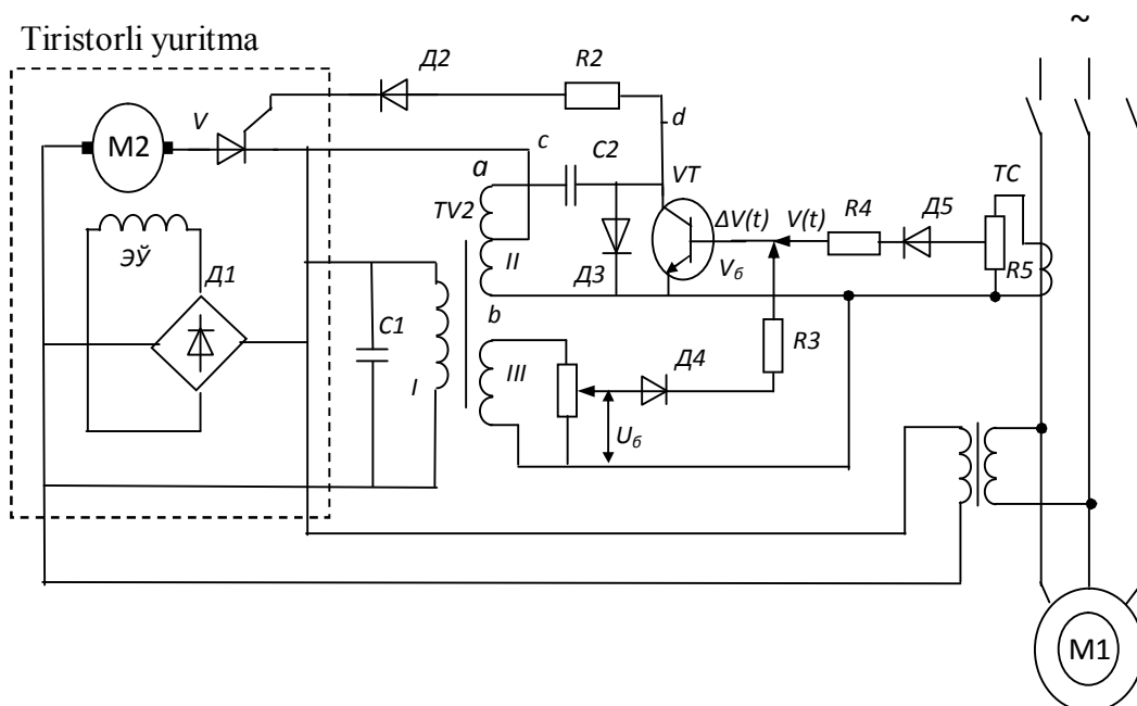
4.2- rasm. Paxta yoki chigit valigi zichligining yuklanish «og'ishi» bo'yicha ARTning elektr sxemasi.
