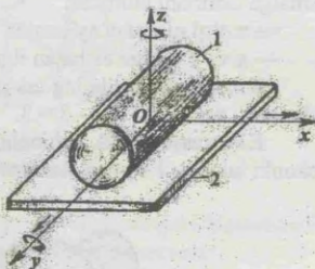
1.17-rasm. Silindr-tekislik kinematik juftligi.
