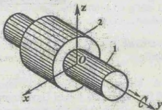
1.19-rasm. Silindr kinematik juftligi.
