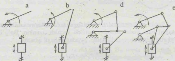
1.15-rasm. Qaytma-ilgarilanma harakatlanuvchi mexanizm.
