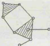
3-tartibli IV sinf Assur guruhlari
