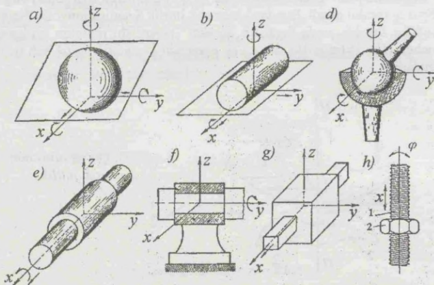
1.2-rasm. Kinematik juftliklarning turli sinflari.
