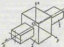
1.20-rasm. Ilgarilama kinematik juftlik.
