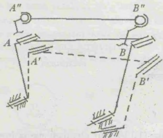
1.12-rasm. To'rt sharnirli mexanizm.
