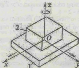
1.18-rasm. Tekislik kinematik juftligi.
