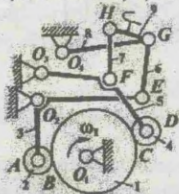
1.21-rasm. To'quv mashinasining strukturaviy sxemasi.
