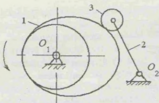
1.13-rasm. Kulachokli mexanizm.
