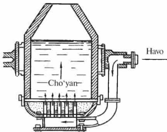
14.3- rasm. Cho'yandan po'lat quyib olinadigan konverter.
