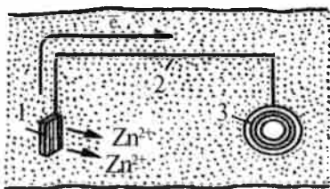
12.7- rasm. Yerosti metall quvurlarining protektorli muhofaza sxemasi:
