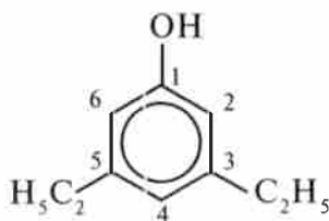
3,5- dietilfenol
