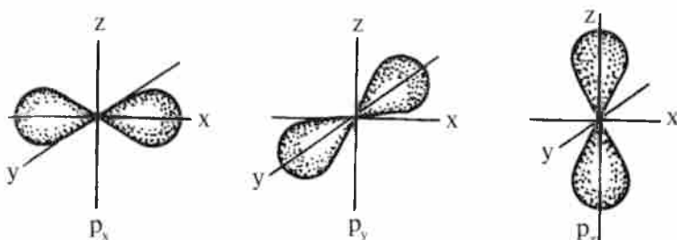
2.5- rasm. p - elektron orbitallarning shakli va joylashishi.
