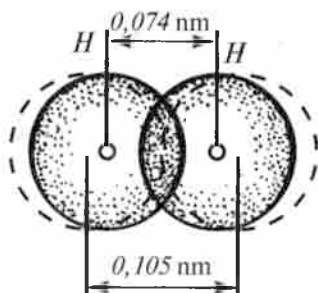
3.1- rasm. Vodorod molekulari hosil bo‘lishida elektron orbitallarning bir-birini qoplash sxemasi.
