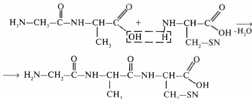
Tripeptid (glitsil-alanil-sistein)
