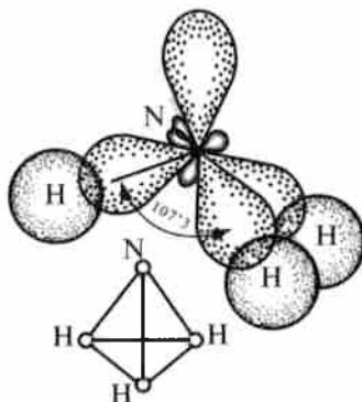
3.4-rasm. \text{NH}_3 molekulasida kimyoviy bog‘lanishlarning hosil bo‘lish sxemasi.
