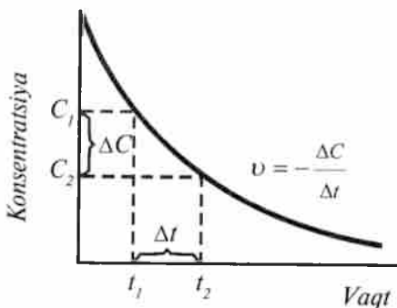
4.1.-rasm. Reaksiya kirishayotgan modda konsentratsiyasining vaqt o'tishi bilan o'zgarishi.
