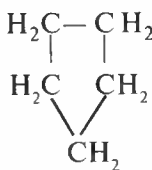
siklopentan
