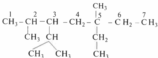
2,5-dimetil-5-etil-3-izopropilgeptan
