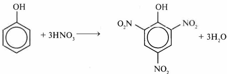
2, 4, 6 - trinitrofenol
