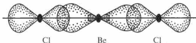
3.7- rasm. \text{BeCl}_2 ning chiziqsimon molekulası.
