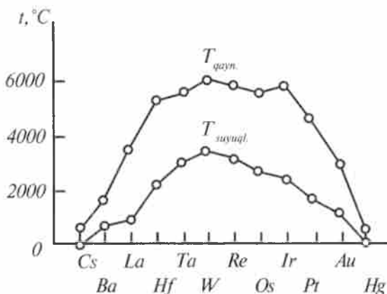
12.2- rasm. VI davr metallarining suyuqlanish va qaynash temperaturalari egri chiziqlari.
