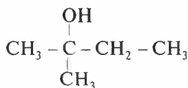
2-metilbutanol-2
