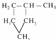
metilsiklopentan
