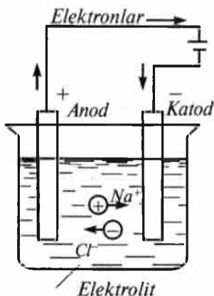
7.2- rasm. \text{NaCl} suyuqlanmasini elektroliz qilish sxemasi.
