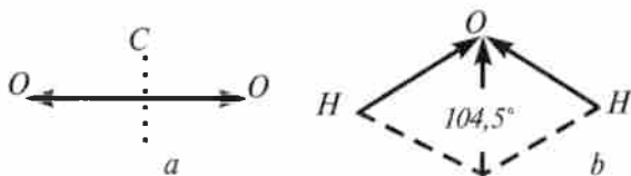
3.13-rasm. \text{CO}_2 (a) va suv (b) molekularida bogʻlanishlar dipol elektr momentlarini geometrik qoʻshish.
