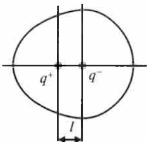
3.12-rasm. Dipol elektr momenti o'zgaras bo'lgan qutbli molekula.
