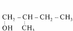
2-metilbutanol-1
