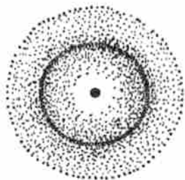
2.2-rasm. Vodorodning zichligi notekis bo'lgan elektron buluti.
