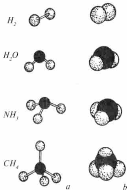
3.19-rasm. Molekularlarning modellari:
