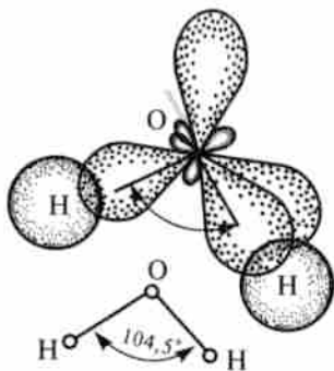
3.3-rasm. \text{H}_2\text{O} molekulasida kimyoviy bog‘lanishlarning hosil bo‘lish sxemasi.
