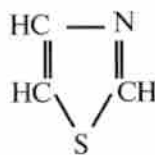
tiazol
