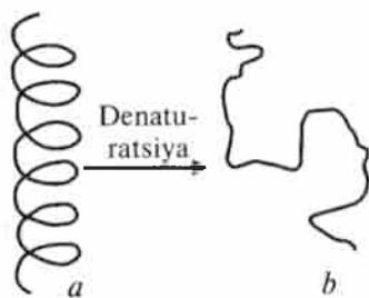
18.1-rasm. Denaturatsiyada oqsil molekulasi konfiguratsiyasining o'zgarishi:
