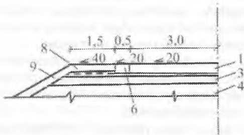
4.1-rasm. I - IV toifali avtomobil yo'llari uchun sementbeton qoplamali yo'l to'shasining namunaviy ko'ndalang kesimlari sxemasi 7
