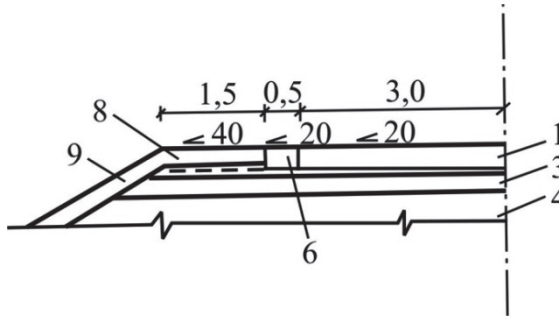
4.1-расм. I–IV тоифали автомобил йўллари учун цементбетон қопламали йўл тўшамасининг намунавий кўндаланг кесимлари схемаси 7 :
