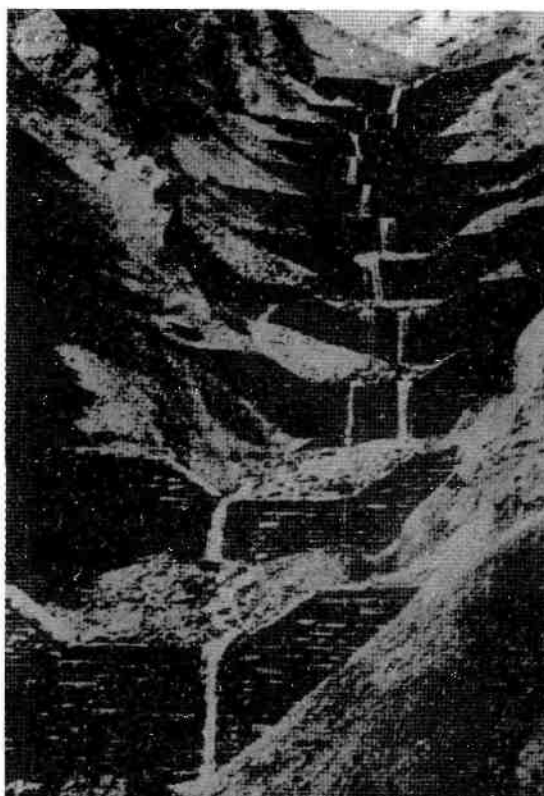
Рис. 6.7. Противоселевые барражи. Бреттервандбах близ Матрия, Восточный Тироль, Австрия
