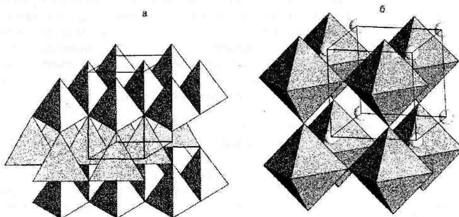
Рис. 2.22. Кристаллические решетки: а — вюрцита ( \text{ZnS} ) и б — перовскита ( \text{CaTiO}_3 )
