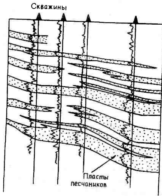
Рис. 3.6. Электрокаротажные кривые в скважинах, помогающие выявить пласты песчаников в толще пород, обладающих относительно высоким сопротивлением. На кривых хорошо видны «пики», соответствующие песчаникам
