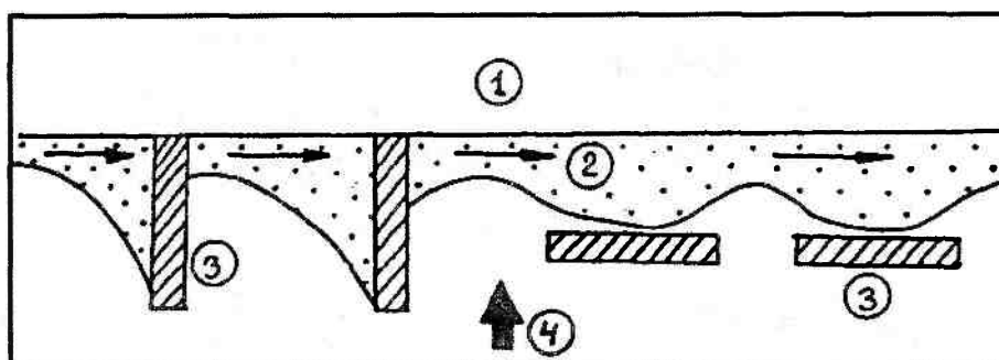
Рис. 14.36. Защита пляжа от размывания волнами. 1 — берег, 2 — пляж, 3 — бетонные блоки, 4 — направление действия волн. Стрелки указывают направление перемещения материала на пляже
