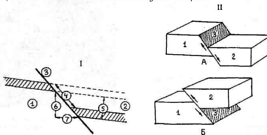
Рис. 17.23. I — Элементы сброса. Блоки (крылья): 1 — поднятый (лежащий), 2 — опущенный (висячий), 3 — сместитель, 4 — амплитуда по сместителю, 5 — стратиграфическая амплитуда, 6 — вертикальная амплитуда, 7 — горизонтальная амплитуда. II — блок-диаграммы: А — сброса, Б — взброса. Крылья: 1 — лежащее; 2 — висящее; 3 — сместитель
