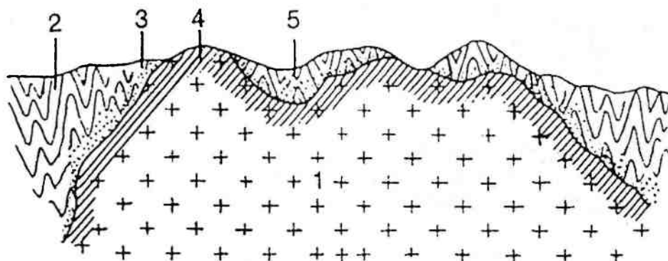
Рис. 15.5. Характер контактов в интрузивном массиве гранитов. 1 — собственно интрузивный массив гранитов, 2 — вмещающие породы; 3 — зона экзоконтакта (изменение вмещающих пород); 4 — зона эндоконтакта (изменение гранитов); 5 — провесы кровли
