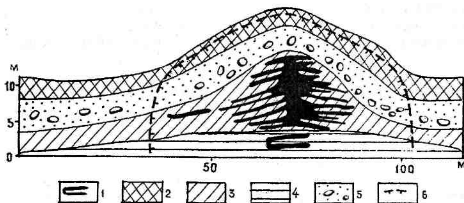
Рис. 13.15. Разрез бугра пучения в долине р. Хантайки (по Г. С. Константиновой, 1963). 1 — шилы льда мощностью до 20–25 см; 2 — торф; 3 — суглинок; 4 — глина, 5 — песок; 6 — верхняя поверхность вечной мерзлоты
