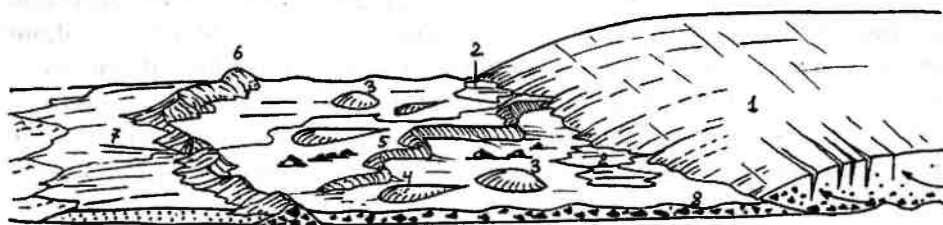
Рис. 12.16. Перигляциальная область покровного ледника: 1 — ледник; 2 — приледниковые озера; 3 — камы; 4 — друмлины; 5 — озы; 6 — конечно-моренный вал; 7 — зандровая равнина; 8 — донная морена
