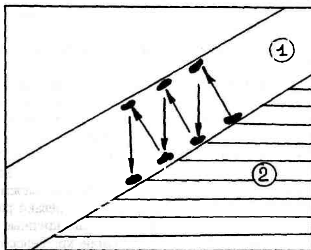
Рис. 13.16. Схема перемещения частиц и обломков в деятельном слое на склоне — процесс солифлюкции. 1 — деятельный слой; 2 — многолетнемерзлые породы
