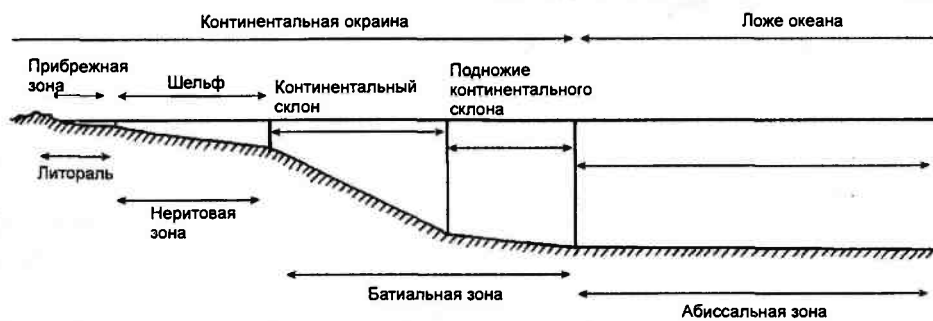
Рис. 14.40. Области в океанах, отличающиеся разными условиями осадконакопления
