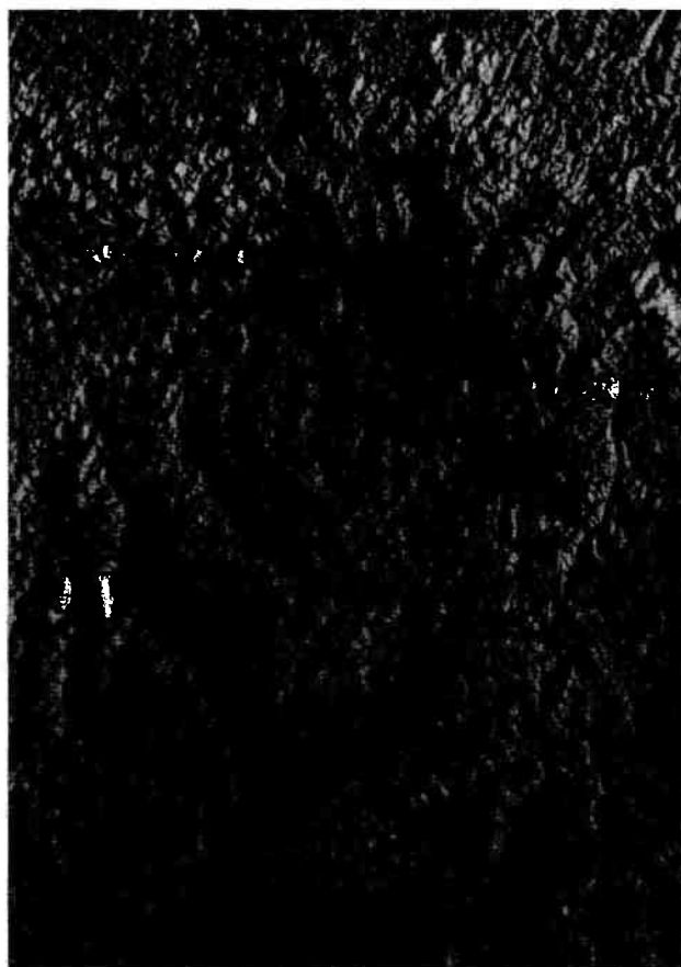
Рис. 16.7. Попигайская астроблема на севере Анабарского массива (Восточная Сибирь). Диаметр около 90 км, время образования — 35 млн лет назад, ранний олигоцен
