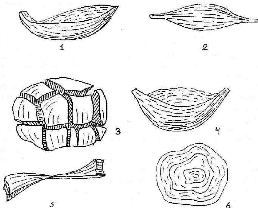
Рис. 15.21. Типы вулканических бомб: 1 — веретеновидная, односторонняя; 2 — веретеновидная; 3 — типа хлебной корки; 4 — двухполюсная веретенообразная; 5 — ленточная; 6 — типа коровьей лепешки
