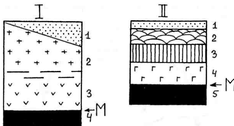
Рис. 2.27. Схемы строения земной коры. I — континентальная кора, слои: 1 — осадочный, 2 — гранитно-метаморфический, 3 — гранулитно-базитовый, 4 — перидотиты верхней мантии. II — океаническая кора, слои: 1 — осадочный, 2 — базальтовых подушечных лав, 3 — комплекса параллельных даек, 4 — габбро, 5 — перидотиты верхней мантии. М — граница Мохоровичича
