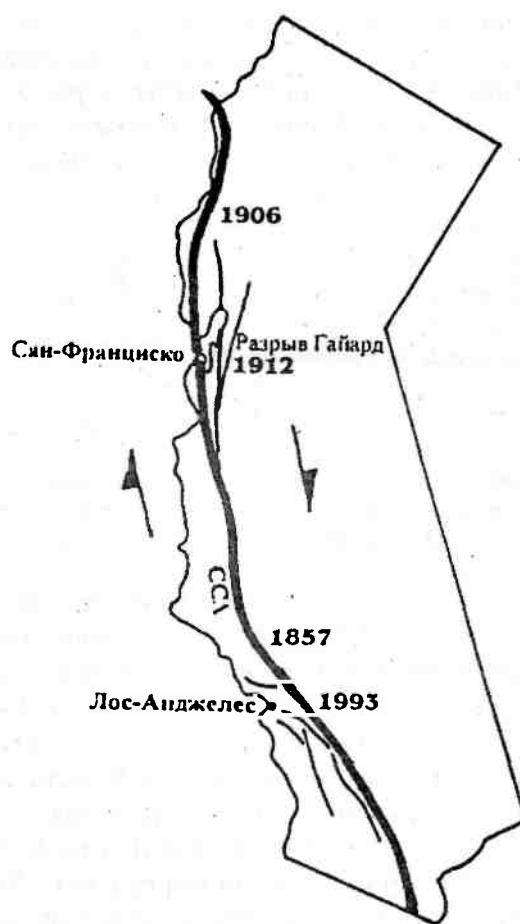
Рис. 17.29. Сдвиг Сан-Андреас в Калифорнии (США). Города Сан-Франциско и Лос-Анджелес находятся в опасной сейсмической зоне
