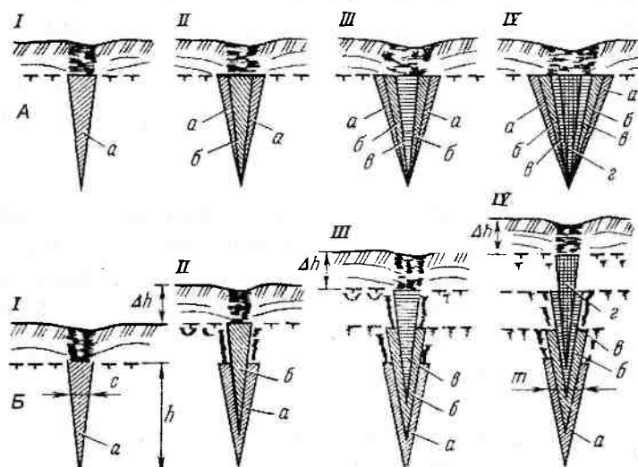
Рис. 13.3. Схема эпигенетического (А) и сингенетического (Б) роста повторно-жильных льдов (по Б. А. Достовалову): I–IV — последовательные стадии роста жил, a – z — ежегодно образующиеся элементарные ледяные жилки, \Delta h — мощность накапливающегося за год слоя при сингенезе, h и c — высота и ширина элементарной жилки, m — общая ширина клина
