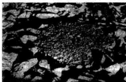
Рис. 13.12. Сортированные каменные многоугольники. Северная Земля (фото В. Г. Чигира)
