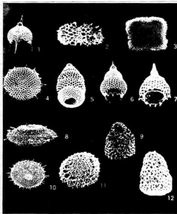
Рис. 14.55. Связь распространения некоторых современных радиолярий с водными массами (по Дж. П. Кеннегу, 1987). Тропические (1–3): 1 — Pterocanium praetextum , \times 245 ; 2 — Ommatartus tetrathalaniae , \times 307 ; 3 — Spongaster tetras , \times 249 . Субтропические (4–7): 4 — Phacodiscid , \times 249 ; 5 — Sticocyrtis sp., \times 297 ; 6 — Lamprocyclas maritima (холодноватый), \times 248 ; 7 — Lamprocyclas maritima (тепловодный), \times 297 . Полярные — субполярные (8–11): 8 — Spongotrochus glacialis , \times 269 ; 9 — Antarctissa strelkovi , \times 265 ; 10 — Spongotrochus glacialis , \times 242 ; 11 — Lithelius nautiloides , \times 344 ; 12 — Antarctissa denticulata , \times 292 .
