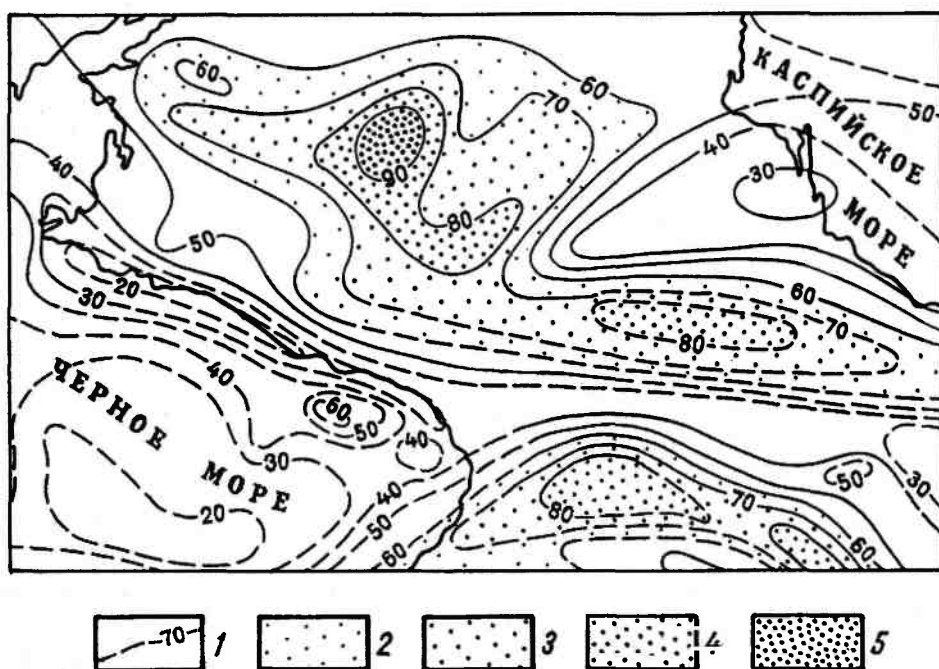
Рис. 2.18. Схема теплового потока Кавказа (по В. Чермаку и Е. Харгиту): 1 — изолинии теплового потока в \text{мВт}/\text{м}^2 ; 2–5 — разные величины теплового потока
