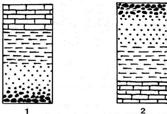
Рис. 14.62. Залегание отложений: 1 — трансгрессивное, 2 — регрессивное
