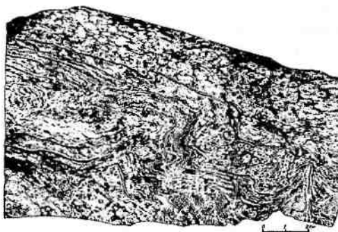
Рис. 2.25. Флюидальная текстура (текстура течения) в риолитовой лаве
