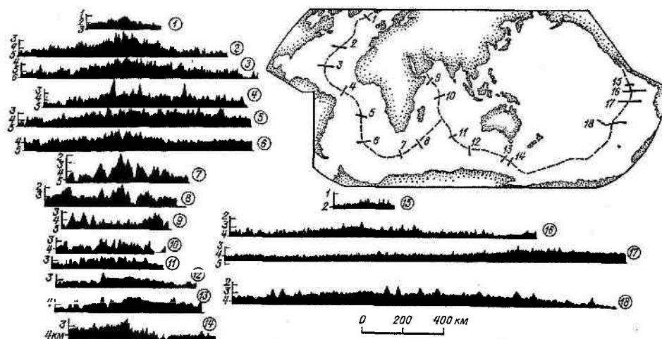
Рис. 14.19. Обзорные профили рельефа срединно-океанических хребтов Мирового океана
