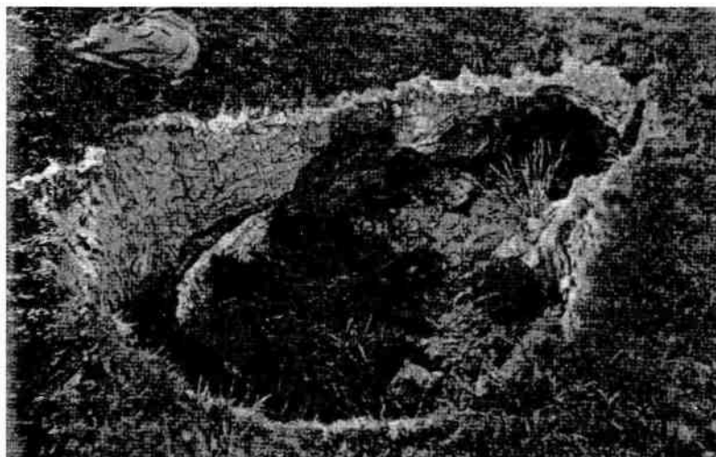
Рис. 8.5. Суффозионная воронка в низовьях р. Пахры (фото З. Виноградова)
