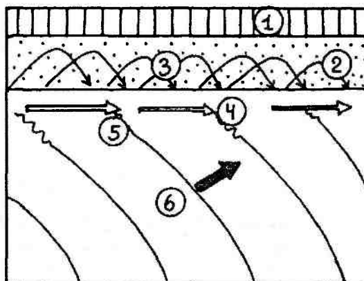
Рис. 14.33. Перенос песка вдоль пляжа и перемещение взвешенного материала в воде вдоль берега в зоне прибоя. 1 — берег; 2 — пляж; 3 — перемещение песка вдоль пляжа; 4 — перенос в воде взвешенного песка; 5 — зона прибоя; 6 — волны
