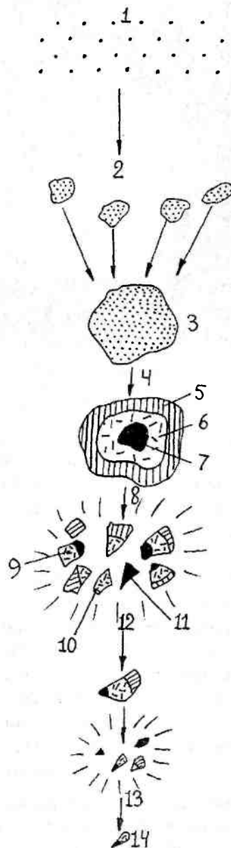
Рис. 1.14. Образование метеоритов. 1 — газопылевое облако; 2 — аккреция в тела размером в несколько метров (планетезимали); 3 — аккреция планетезималей в тела размером 10–200 км; 4 — плавление и дифференциация; 5 — базальты; 6 — силикаты; 7 — железо; 8 — дробление при ударе. Обломки: 9 — железоканменные; 10 — канменные; 11 — канзные; 12 — канзный метеорит; 13 — дробление; 14 — каннее канный метеорит
