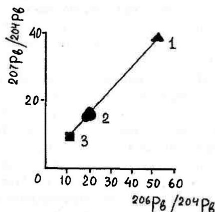
Рис. 3.12. Определение возраста Земли с помощью изотопных хронометров (по Ю. А. Шуколюкову, 2000). 1 — каменные метеориты; 2 — средний изотопный состав свинца Земли; 3 — железные метеориты
