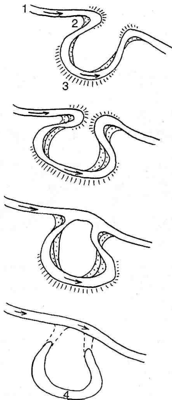
Рис. 6.13. Развитие меандры и перехват реки с образованием старицы. На отмеле берегу накапливается аллювий, а обрывистый берег все время подмывается: 1 — река; 2 — отмельный берег; 3 — приглубый берег; 4 — старица
