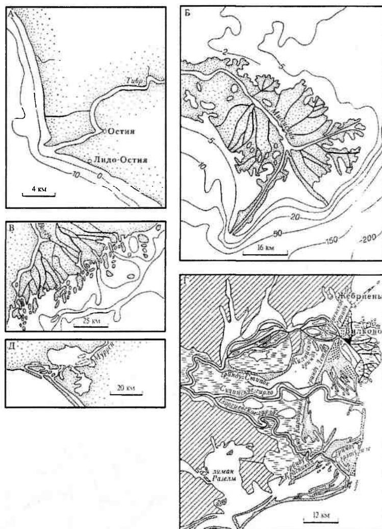
Рис. 6.23. Различные типы дельт. А — р. Тибр, Италия; Б — р. Миссисипи, США; В — р. Волга, Россия; Г — р. Дунай, Румыния; Д — р. Муррей, США
