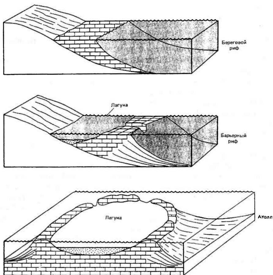
Рис. 14.51. Блок-диаграммы трех главных типов современных рифов
