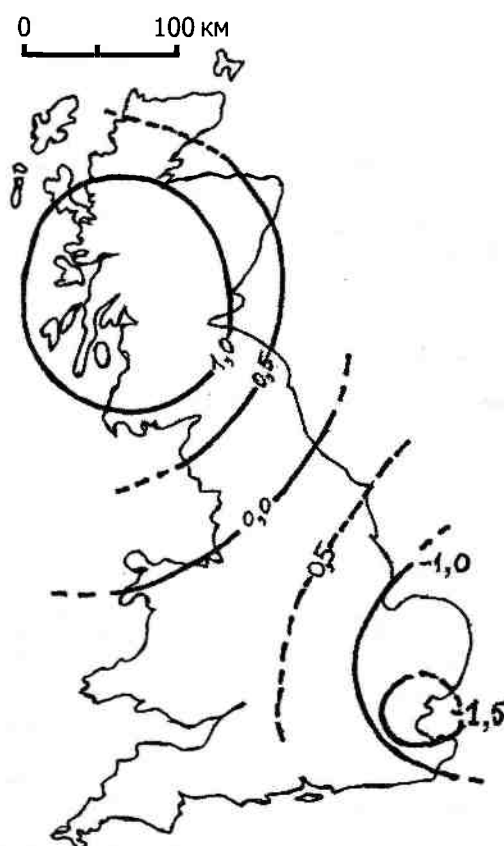
Рис. 17.3. Современные тектонические движения земной коры Великобритании в километрах. Северная часть страны поднимается после освобождения от ледникового покрова, а юго-восточная — испытывает опускание
