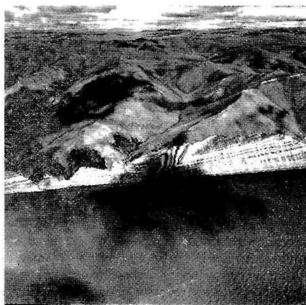
Рис. 17.19. Одиночная складка в горизонтально залегающих меловых отложениях в низовьях р. Лены, Восточная Сибирь
