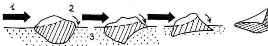
Рис. 11.2. Образование драйкантеров (вентифактов): 1 — ветер; 2 — переворачивание камня; 3 — перемещающийся песок обтачивает и полирует поверхность камня
