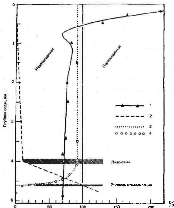
Рис. 14.57. Параметры, влияющие на распространение карбоната кальция в осадках экваториальной области Тихого океана с увеличением глубины. 1 — насыщение кальцитом (%); 2 — (скорость растворения/скорость поступления) \times 100 ; 3 — содержание \text{CaCO}_3 в осадках рассчитанное; 4 — содержание \text{CaCO}_3 в осадках наблюдаемое (по Tj H. Van Andel et al, 1975)
