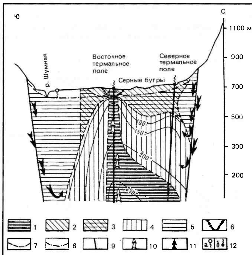
Рис. 15.47. Гидрогеологическая и гидрохимическая модель гидротермальной системы кальдеры Узон (по Карпову). 1 — зона растворов сульфатно-хлоридно-натриевого состава; 2 — зона сульфатных вод; 3 — зона растворов сульфатно-хлоридно-бикарбонатного состава; 4 — зона хлоридно-сульфатных растворов; 5 — пресные инфильтрационные воды; 6 — зона ртутно-сурьмяно-мышьякового оруденения; 7 — граница зоны разных гидрохимических типов вод; 8 — уровень грунтовых вод; 9 — разломы; 10 — пути миграции глубинных флюидов; 11 — пути инфильтрации вадозовых вод; 12 — источники: а — газифицирующие «холодные» углекислые; б — термальные
