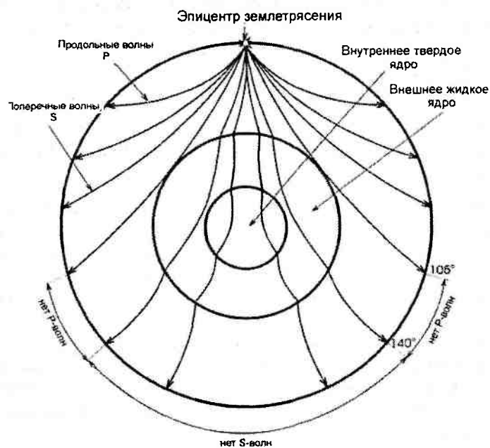
Рис. 2.4 Прохождение продольных (P) и поперечных (S) волн через Землю. Поперечные волны не проходят через жидкое внешнее ядро, а у продольных волн есть «зона тени» в 35^\circ , т. к. в жидком ядре волны преломляются
