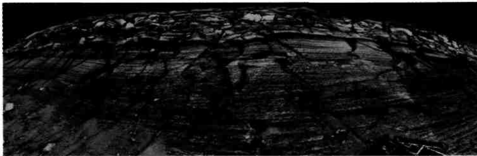
Рис. 4. Слоистые породы на Марсе — результат осаждения в водной среде. Место посадки космического аппарата «Оппортьюнити» (NASA)
