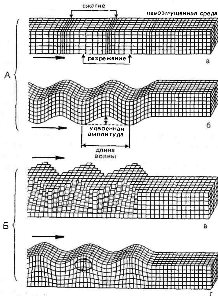
Рис. 2.2. Типы сейсмических волн. А — объемные волны: а — продольные, б — поперечные. Б — поверхностные волны: в — Лява, г — Рэлея. Стрелками показано направление движения волны
