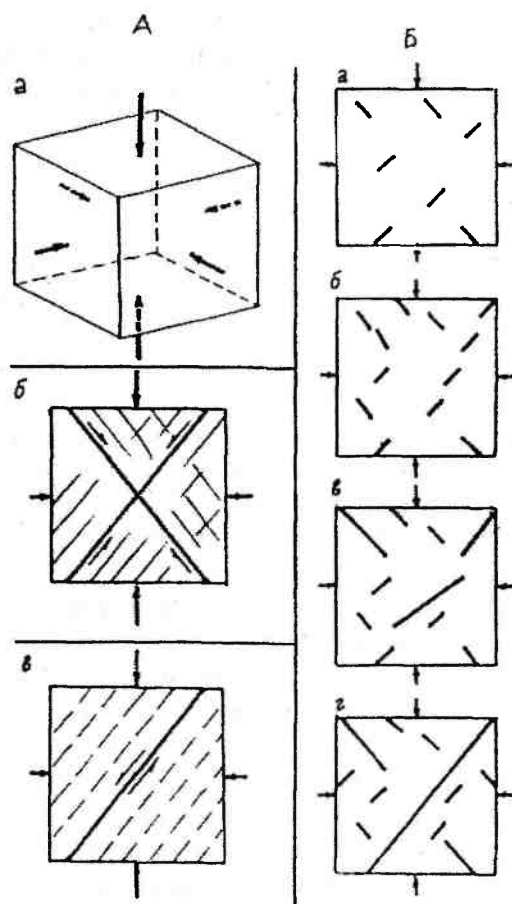
Рис. 21.3. Нелинейный геодинамический процесс — разрушение нагруженного блока горной породы. Механизм разрушения: А — механическая модель (а — схема нагружения квазисплошного блока; б, в — теоретические схемы скалывания: а — перекрестного, б — параллельного). Б — модель разрушения реального блока (а — зарождение рассеянных «микротрещин», б — взаимодействие и группирование «микротрещин», зарождение «мезотрещин» на конкурирующих сечениях и направлениях, в — послебифуркационная подготовка сквозного разрыва на некотором определенном макросечении, г — макроскалывание)
