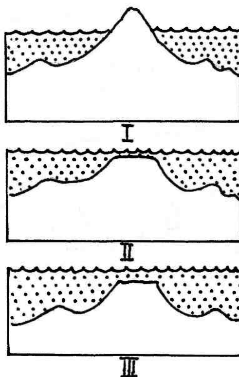
Рис. 14.24. Образование гайота. I — вулканический остров; II — срезание морской абразией вершины острова; III — опускание океанского дна
