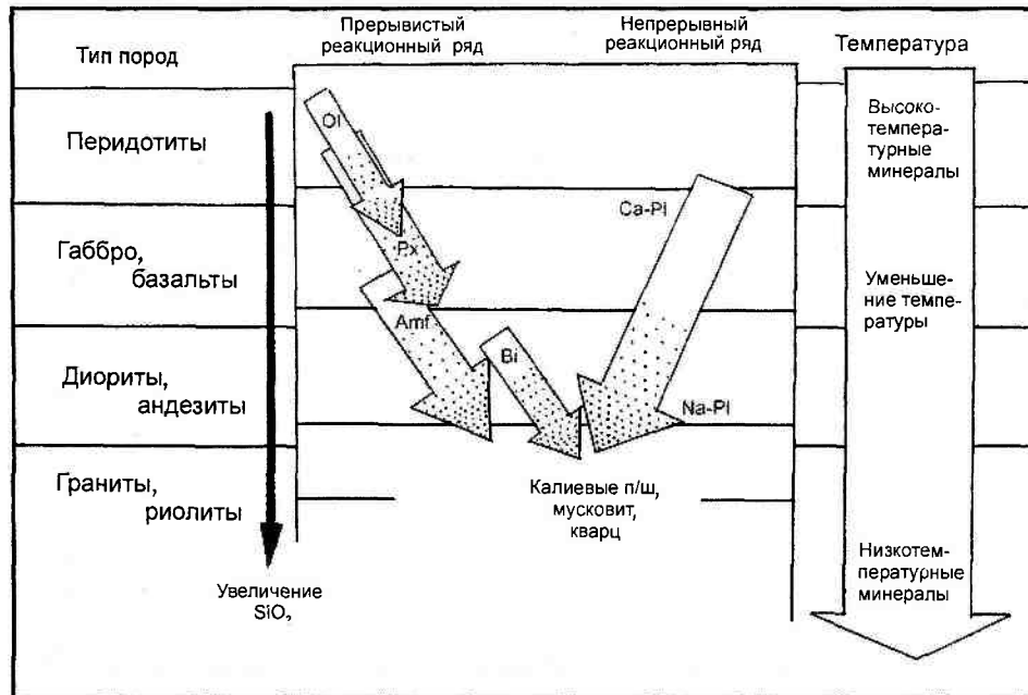
Рис. 15.3. Реакционный ряд Боуэна
