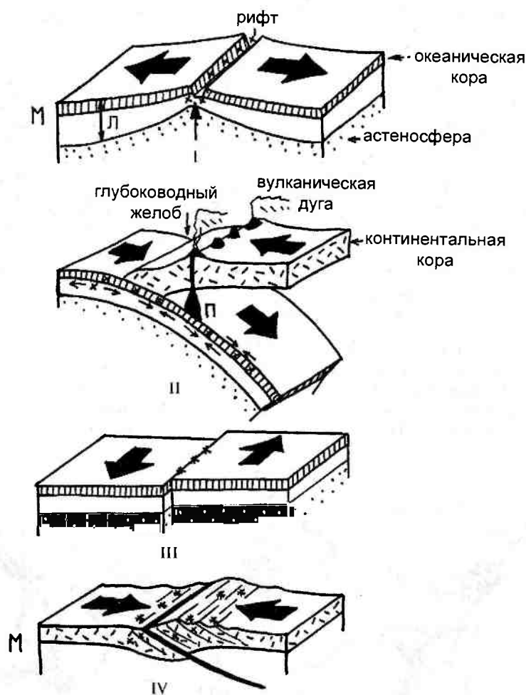
Рис. 3.15. Типы границ литосферных плит.
