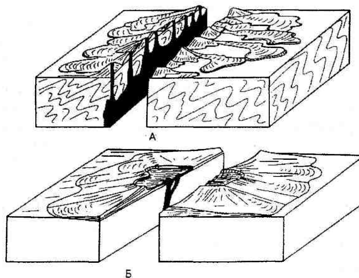
Рис. 15.42. Вулканы трещинного (А) и щитового центрального (Б) типов
