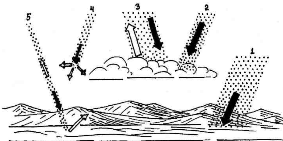
Рис. 4.2. Солнечная радиация, поступающая на Землю. 1 — 47 % поглощается горными породами, почвой и водой на земной поверхности; 2 — 19 % поглощается атмосферой и облаками; 3 — 23 % отражается облаками; 4 — 8 % рассеивается атмосферой; 5 — 3 % отражается грунтами
