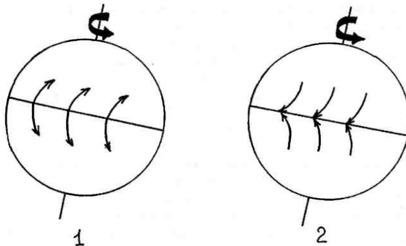
Рис. 14.11. Эффект ускорения Кориолиса.
