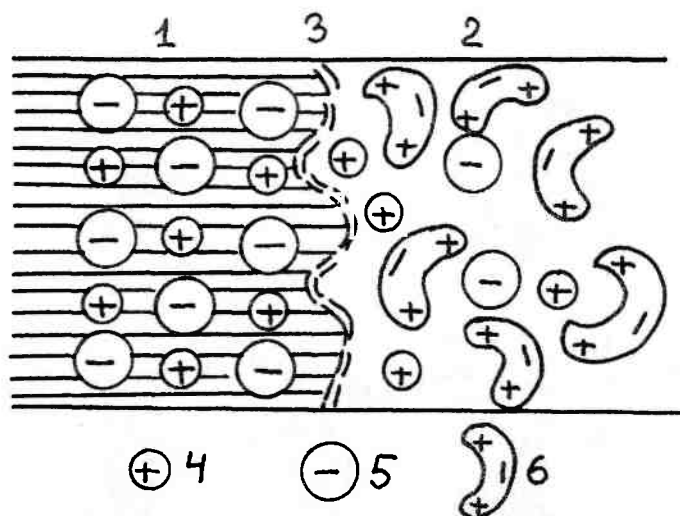
Рис. 5.5. Схема взаимодействия воды с поверхностью минерала. Молекулы воды способны отрывать ионы от минерала. 1 — минерал; 2 — раствор; 3 — поверхность минерала; 4 — катион; 5 — анион; 6 — молекула воды
