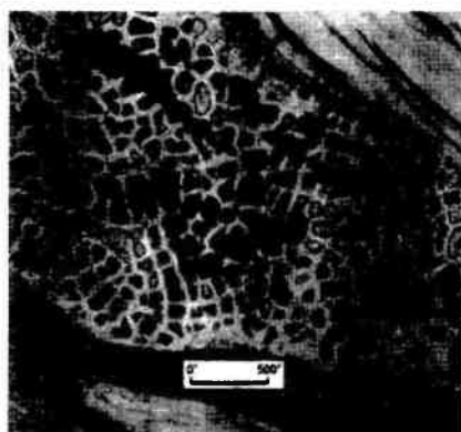
Рис. 13.11. Полигональные поля
