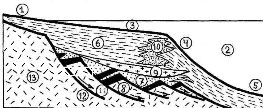
Рис. 14.25. Пассивная континентальная окраина: 1 — суша, 2 — океан, 3 — шельф, 4 — континентальный склон, 5 — континентальное поднятие, 6 — морские осадки, 7 — континентальные осадки, 8 — базальты, 9 — каменная соль, 10 — рифтовый массив, 11 — направление смещения блоков, 12 — листрические сбросы, 13 — континентальная кора
