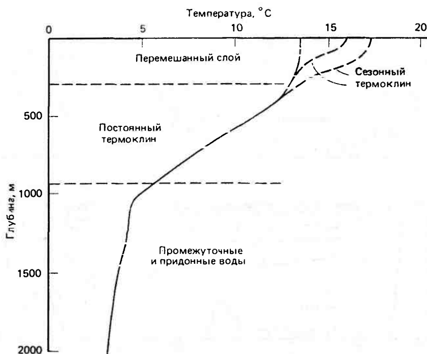
Рис. 14.2. Постоянный термоклин. В верхнем перемешанном слое толщиной несколько сот метров может развиваться сезонный термоклин (по В. W. Pipkin et al, 1977)
