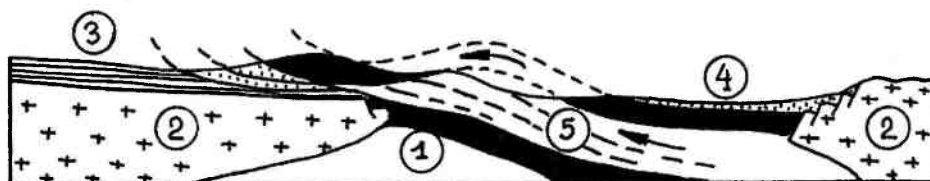
Рис. 3.23. Начальное образование покрова Семайл на востоке Аравийского полуострова (по Р. Дж. Колмену): 1 — океаническая кора (офиолиты), 2 — континентальная кора, 3 — платформенный чехол, 4 — глубоководные осадки, 5 — покров
