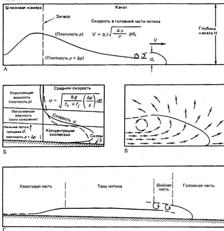
Рис. 14.44. Гидравлика турбидных потоков по лабораторным экспериментам в лотках. А. Волна турбидного потока, наблюдавшаяся в горизонтальном канале после спуска суспензии из шлюзовой камеры в одном его конце. Скорость головной части потока V зависит от толщины головной части ( d_2 ), разности плотностей суспензии в турбидном потоке и воды над ним ( \Delta\rho ), плотности воды \rho и ускорения силы тяжести g . Б. Стационарный однородный турбидный поток вниз по склону g . Средняя скорость потока u зависит от толщины потока d , разности плотностей, сил трения на границе с дном ( f_0 ) и с вышележащей водой ( f_i ). В. Характер движений внутри и вокруг головной части турбидного потока. Г. Схема расчленения турбидного потока на головную часть, тело и хвостовую часть (по G. V. Middleton, M. A. Hampton, 1976)
