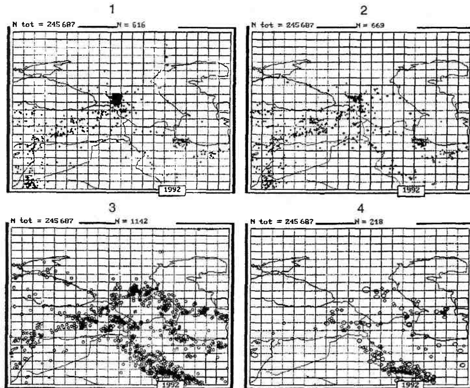
Рис. 18.10. Распределение эпицентров землетрясений в Кавказском регионе. Глубина (км): 1 — 0–10; 2 — 10–25; 3 — 25–50; 4 — глубже 50
