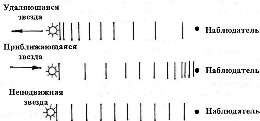
Рис. 1.1. Эффект Доплера. При удалении объекта от наблюдателя спектральные линии смещаются в сторону красного цвета («красные смещения»)
