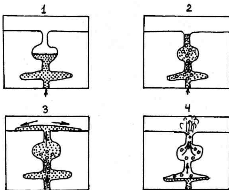
Рис. 15.48. Схема действия гейзера. 1 — снизу поступает горячая вода; 2 — уровень воды повышается, пузырьки собираются в узком месте; 3 — пузырьки выталкивают воду вверх, и она начинает переливаться через край жерла; 4 — уменьшение давления превращает воду в пар, и он выбрасывается вверх вместе с водой. Гейзер фонтанирует
