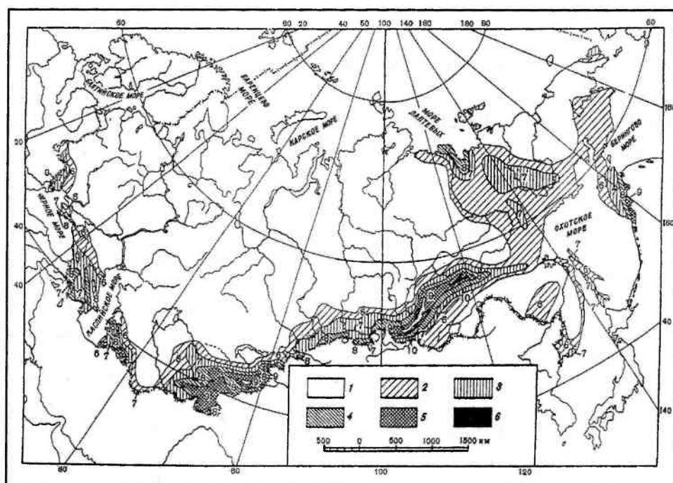
Рис. 18.11. Сейсмическое районирование территории бывшего СССР. 1–6 — районы с различной балльностью, показанной цифрами. Белый цвет — балльность от 0 до 5
