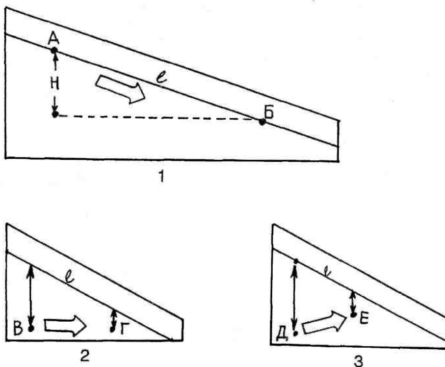
Рис. 7.5. Движение грунтовых вод в зависимости от уровня вод и давления. 1. Точки А и Б имеют одинаковое давление, но А выше Б и вода движется от А к Б (толстая стрелка). 2. Точка В имеет более высокое давление, чем точка Г, и вода движется от В к Г. 3. Точка Д имеет более высокое давление, чем точка Е, вода движется от Д к Е. e — уровень грунтовых вод
