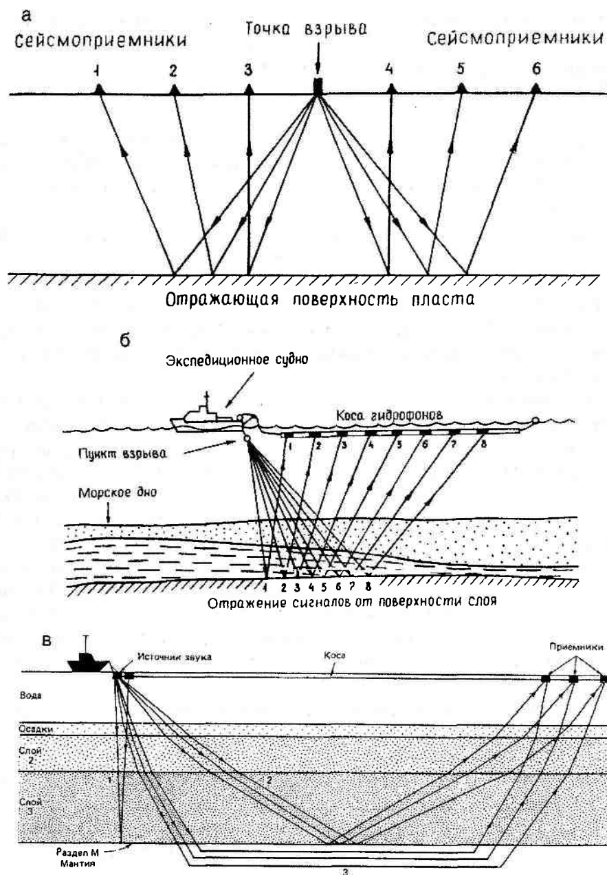
Рис. 2.3. Схема отражения сейсмических волн а) от поверхности пласта горных пород; б) метод работы НСП (непрерывное сейсмическое профилирование); в) прохождение отраженных и преломленных волн через слои земной коры от источника до приемника: 1 — вертикальное отражение, 2 — широкоугольные отражения, 3 — преломленные волны
