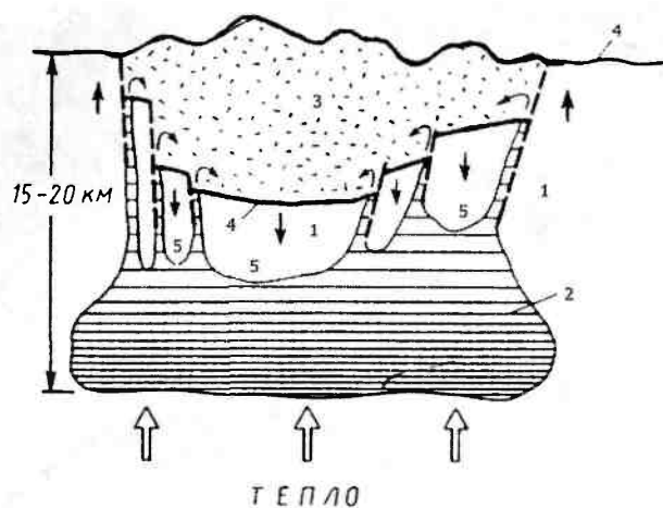
Рис. 15.33. Образование вулканотектонической впадины (вне масштаба):
