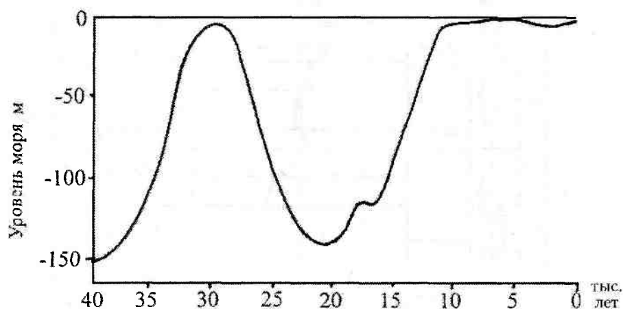
Рис. 14.39. Изменение уровня моря за последние 40 тыс. лет (по Дж. Д. Хэнсому, 1988)
