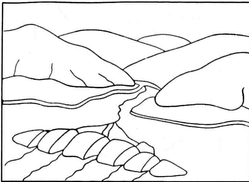
Рис. 6.28. Антецедентные долины рукавов р. Гирдыманчая, прорезающие растущую Карамарьянскую антиклиналь у сел. Падар (по В. А. Гроссгейму)
