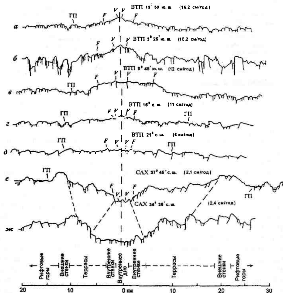
Рис. 14.20. Характерные профили рельефа рифтовой зоны срединно-океанических хребтов с различными скоростями спрединга. Неовулканическая зона ограничена символами V, а зона трещиноватости — F, отметки ГП определяют зону границы плиты.
