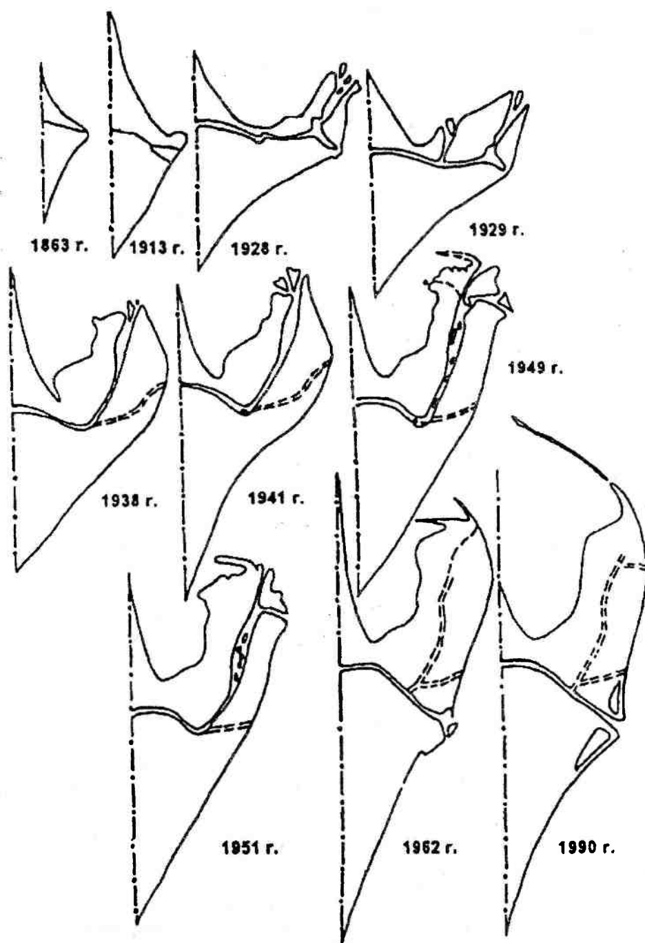
Рис. 6.22. Схема эволюции дельты р. Сулака в XIX и XX вв.
