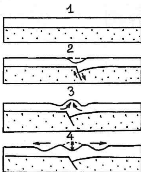
Рис. 18.13. Образование цунами. 1 — до землетрясения, светлое — вода, точки — океаническое дно; 2 — землетрясение вследствие сброса на дне, на поверхности океана возникает впадина; 3 — на месте впадины образуется купол воды; 4 — купол распадается на круговые волны
