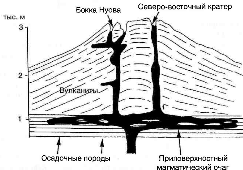
Рис. 15.51. Структурная модель вулкана Этна (Сицилия), по сейсмическим данным. Близповерхностный магматический очаг располагается непосредственно под вулканом на контакте с субстратом
