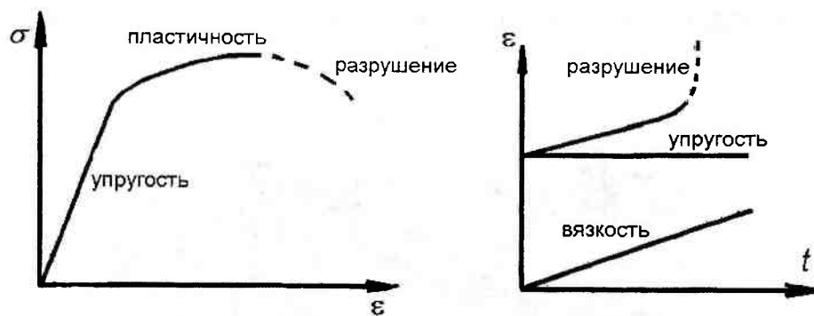
Рис. 17.4. Виды деформаций: \sigma — напряжение, \varepsilon — деформация, t — время
