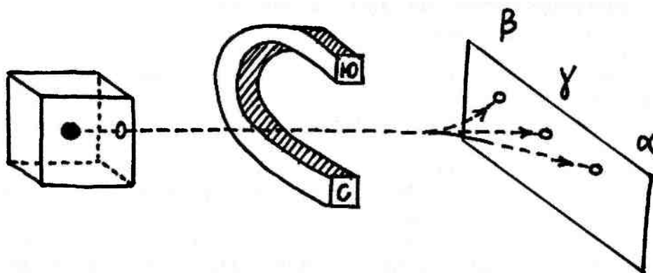
Рис. 3.7. Три типа радиации, выявленные Э. Резерфордом. В свинцовой коробке находится радиоактивное вещество. Радиация состоит из трех типов: альфа ( \alpha ), гамма ( \gamma ) и бета ( \beta ), что фиксируется на фотографической пластинке.
