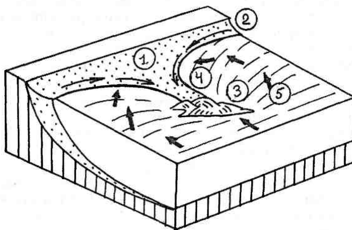
Рис. 14.35. Формирование томболо — перемычки между берегом и островом. 1 — пляж; 2 — перемещение песка на пляже; 3 — остров; 4 — томболо; 5 — волны
