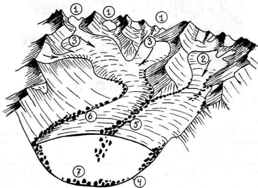
Рис. 12.13. Схема питания и строения горного ледника. 1 — кары; 2 — цирки; 3 — области питания ледника; 4 — ледниковая корытообразная долина — трог. Морены: 5 — срединная, 6 — боковая, 7 — донная
