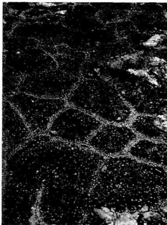
Рис. 13.6. Полигональные структуры — каменные многоугольники
