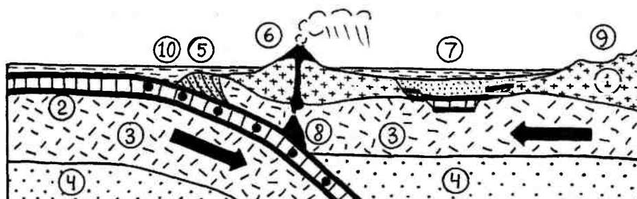
Рис. 14.28. Активная континентальная окраина: 1 — континентальная кора, 2 — океаническая кора, 3 — литосфера, 4 — астеносфера, 5 — аккреционный клин, 6 — островная дуга, 7 — окраинное море, 8 — первичный магматический очаг, 9 — суша континента, 10 — глубоководный желоб
