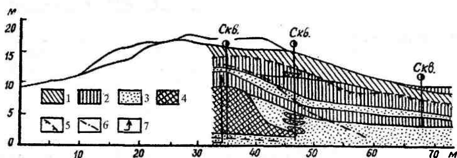
Рис. 13.14. Разрез булгунняха. Лено-Амгинское междуречье. Центральная Якутия (по П. А. Соловьеву): 1 — супеси, 2 — суглинки, 3 — пески, 4 — лед, 5 — верхняя граница мерзлых пород, 6 — граница ядра с выделением линзочки чистого льда, 7 — напор водоносного горизонта
