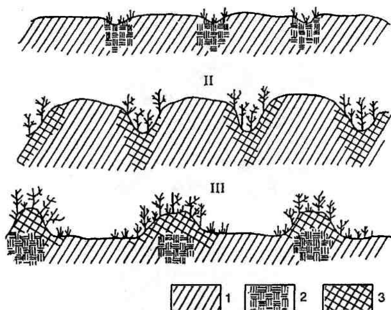
Рис. 13.10. Основные морфологические типы пятен-медальонов: I — плоские или слабо выпуклые, II — выпуклые на пьедесталах-кочках, III — плоские или вогнутые. 1 — суглинок или супесь, 2 — гумусированный грунт, 3 — торф
