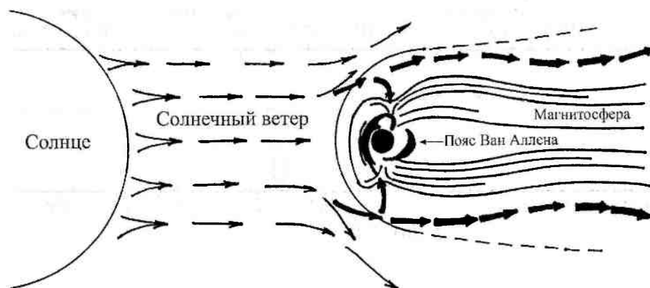
Рис. 1.5. Солнечный ветер
