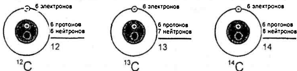
Рис. 3.10. Строение атомов углерода
