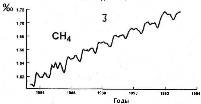
Рис. 12.21. Изменения некоторых параметров приземной атмосферы. 1 — температура; 2 — содержание углекислого газа; 3 — содержание метана. По разным источникам
