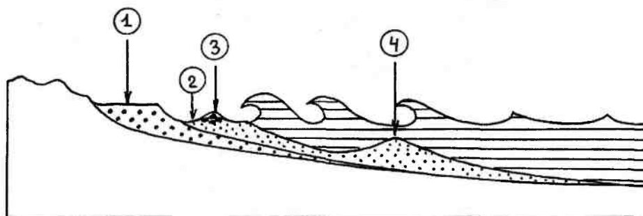
Рис. 14.31. Строение пляжа: 1 — верхний пляж; 2 — нижний пляж; 3 — береговой вал; 4 — подводный бар. Летом пляж расширяется, зимой сокращается
