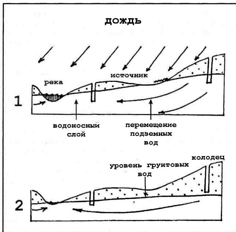
Рис. 7.7. Положение уровня грунтовых вод в дождливый (1) и засушливый (2) сезоны. В сухой сезон понижается уровень реки (межень) и некоторые колодцы пересыхают
