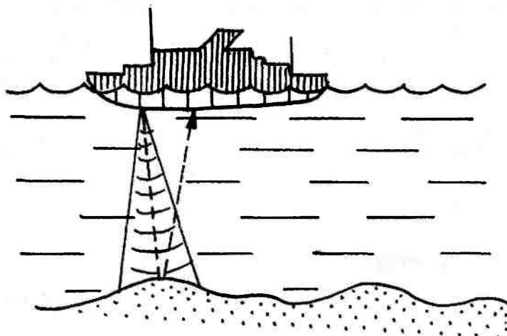
Рис. 14.17. Принцип действия эхолота. Звуковой сигнал отражается от дна и принимается на корабле. Зная скорость звука в воде и разделив время прохождения звукового сигнала на 2, получаем глубину океана
