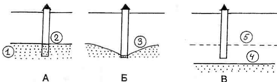
Рис. 7.6. Образование депрессионной воронки в уровне грунтовых вод при усиленном отборе воды из скважины. 1 — водоносный горизонт; 2 — уровень воды в скважине; 3 — депрессионная воронка; 4 — новый уровень грунтовых вод; 5 — прежний уровень грунтовых вод (до отбора)
