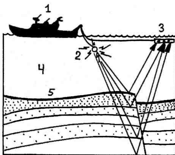
Рис. 3.4. Непрерывное сейсмическое профилирование. 1 — корабль; 2 — источник звуковых волн; 3 — приемник отраженных сигналов; 4 — вода; 5 — морское дно. Стрелками показано отражение звуковых волн от различных слоев горных пород на морском дне
