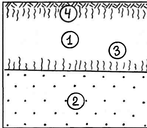
Рис. 7.2. Распределение воды выше зоны грунтовых вод. 1 — зона аэрации, 2 — зона полного насыщения (водоносный горизонт), 3 — капиллярно-подтянутая вода, 4 — капиллярно-подвешенная вода
