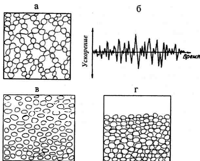
Рис. 18.12. Разжижение грунта при землетрясении (по Е. А. Вознесенскому).
