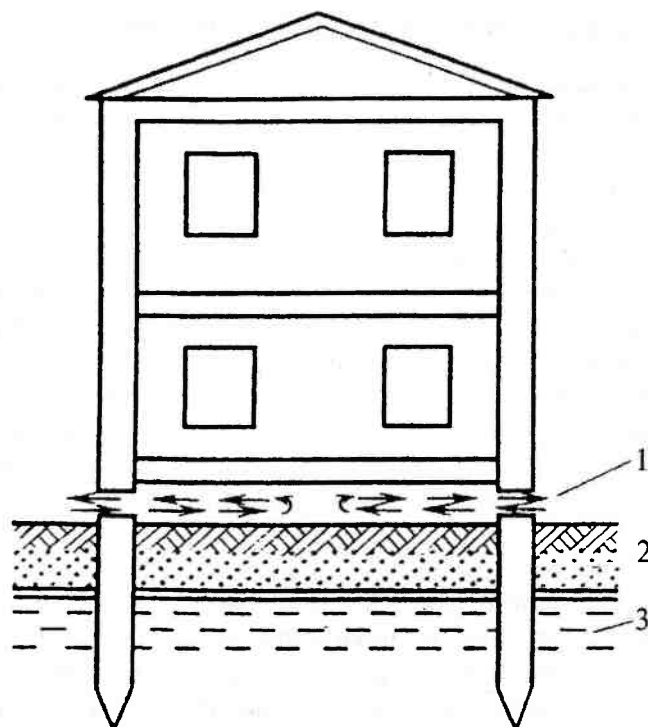
Рис. 13.20. Строительство в криолитозоне. Дома стоят на бетонных сваях, забитых в многолетнемерзлые породы ниже деятельного слоя: 1 — отверстия для циркуляции воздуха; 2 — деятельный слой; 3 — многолетнемерзлые породы
