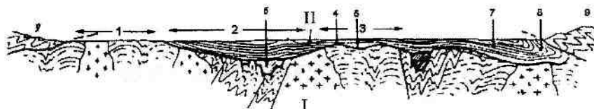
Рис. 19.1. Схема строения платформы: I — фундамент; II — чехол: 1 — щит, 2 — синеклиза, 3 — антеклиза, 4 — свод, 5 — впадина, 6 — авлакоген, краевой прогиб (7 — внешняя зона, 8 — внутренняя зона), 9 — складчатое сооружение
