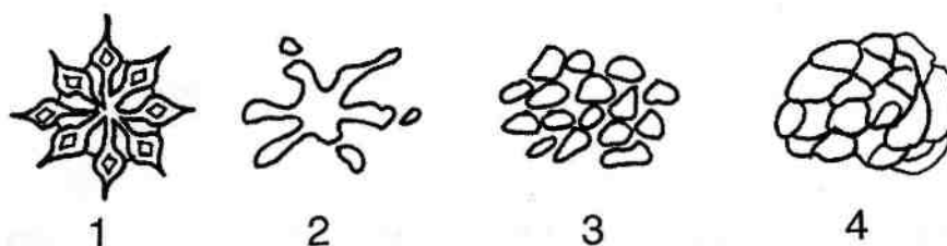
Рис. 12.1. Превращение снега в лед: 1 — снежинка; 2 — под воздействием сублимации (возгонки) выделяется тепло и снежинка оплавляется; 3 — оплавленные комочки образуют фирн; 4 — фирновые зерна соединяются, сплавляются вместе, превращаясь в лед
