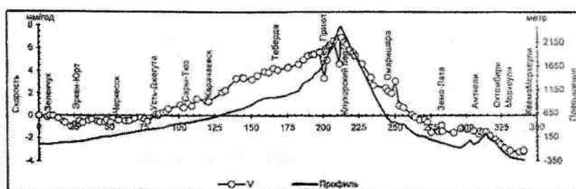
Рис. 17.2. Результаты повторного нивелирования через Большой Кавказ (по Д. А. Лилиенбергу)
