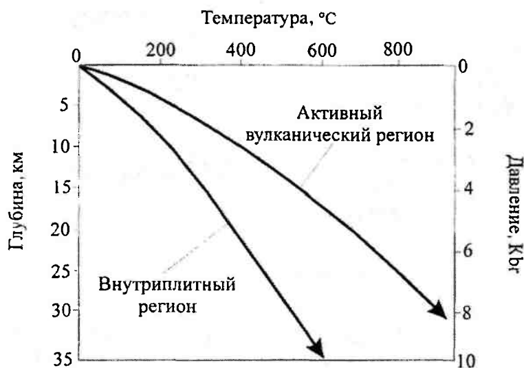
Рис. 2.19. Геотермический градиент в различных геологических регионах
