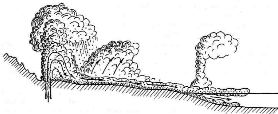
Рис. 15.24. Извержение пеплового потока, распространяющегося на большие расстояния при минимальном уклоне местности. Достигнув моря, некоторое время поток движется по его поверхности и по дну. Благодаря высокой температуре происходят фреатические взрывы. Из пеплового потока образуются игнимбриты — спекшиеся пеплы
