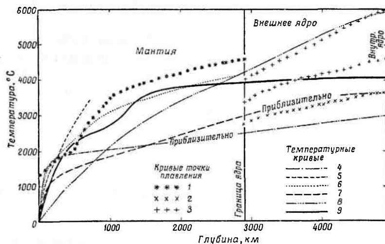
Рис. 2.17. Оценки температур внутри Земли разными авторами (по Б. Гутенбергу, 1963). Все кривые содержат неопределенные предположения. 1 — Аффен (по Гутенбергу, 1956); 2 — Симон (по Гутенбергу, 1954); 3 — Галвари (по Дю Буа, 1957); 4 — Гутенберг (1951); 5 — Джеффрис (1952); 6 — Джекобс (1956); 7 — Ферхуген (1958); 8 — Гилварри (1957); 9 — Любимова (1958)
