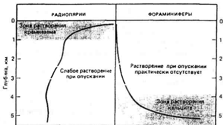
Рис. 14.56. Сравнение профилей растворения радиолярий и планктонных фораминифер, составленное по результатам натурных экспериментов. Основная масса радиолярий и диатомовых растворяется в поверхностных водах. Напротив, растворение известковых микрофоссилий происходит главным образом на дне океана, на глубине более 3,5 км (по W. H. Berger, 1975)
