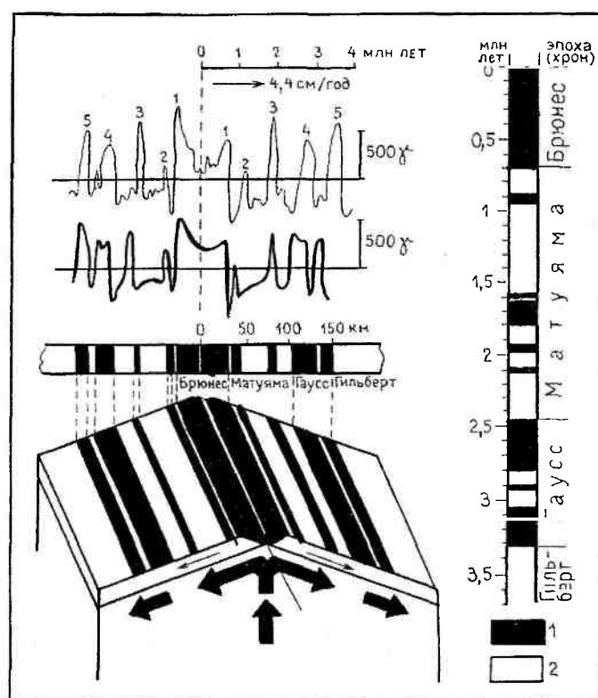
Рис. 3.19. Симметричная система линейных магнитных аномалий (в гамах) на пересечении Восточно-Тихоокеанского поднятия ( 51^\circ ю. ш.). Верхний профиль — по данным аэромагнитной съемки, нижний рассчитан по магнитохронологической шкале (дана справа) исходя из гипотезы Вайна — Мэтьюза о записи геомагнитных инверсий в процессе двустороннего спрединга (см. блок-диаграмму внизу). По Ф. Вайну (1966) и А. Коксу (1969), с изменениями. 1 — прямая полярность, 2 — обратная полярность
