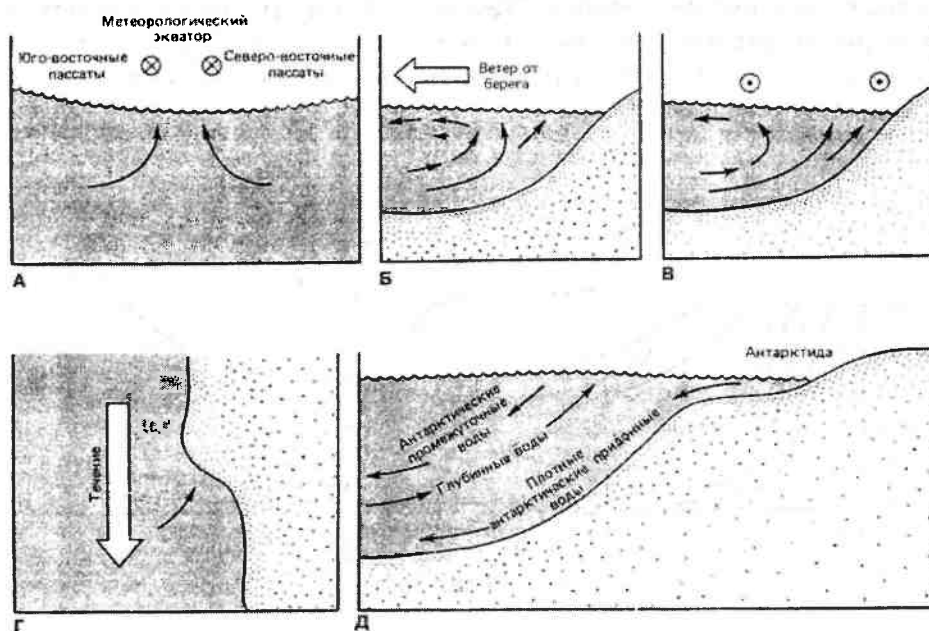
Рис. 14.12. Процессы апвеллинга (описание в тексте). Точка в кружке — ветер, дующий в сторону читателя; крест в кружке — ветер, дующий от читателя. А — апвеллинг в открытом океане, обусловленный действием силы Кориолиса; Б — апвеллинг, вызванный ветром; В — перенос вод под действием силы Кориолиса; Г — апвеллинг, вызываемый конфигурацией берега; Д — апвеллинг, обусловленный разницей в плотности вод (по В. W. Pirkin et al, 1977)
