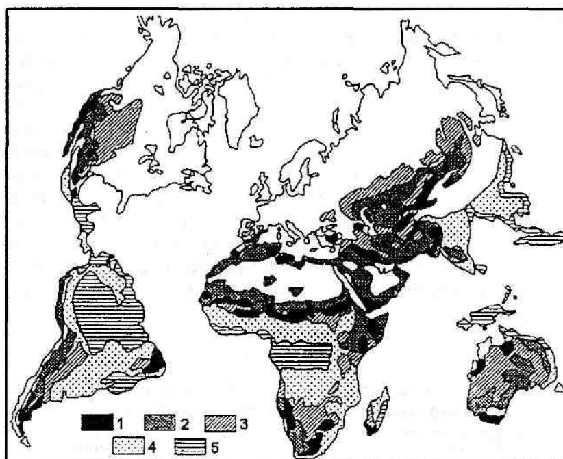
Рис. 20.1. Регионы мира со значительными негативными экологическими нарушениями (по С. П. Горшкову, 1987).
