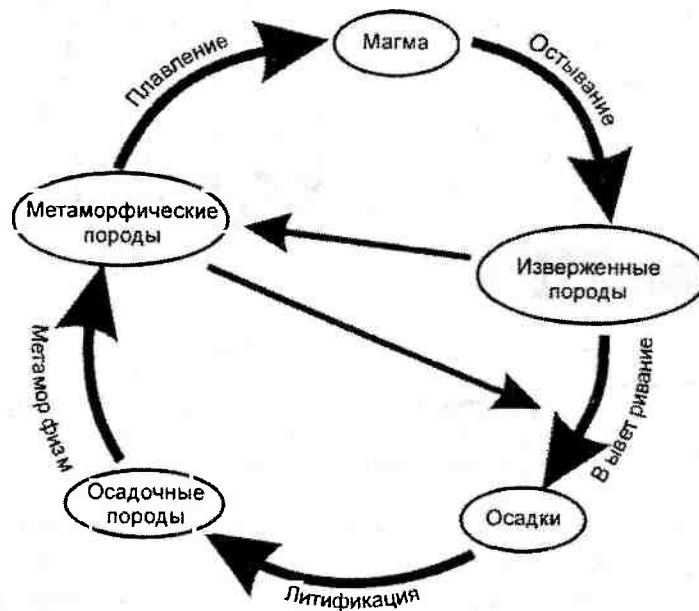
Рис. 2.26. Круговорот горных пород
