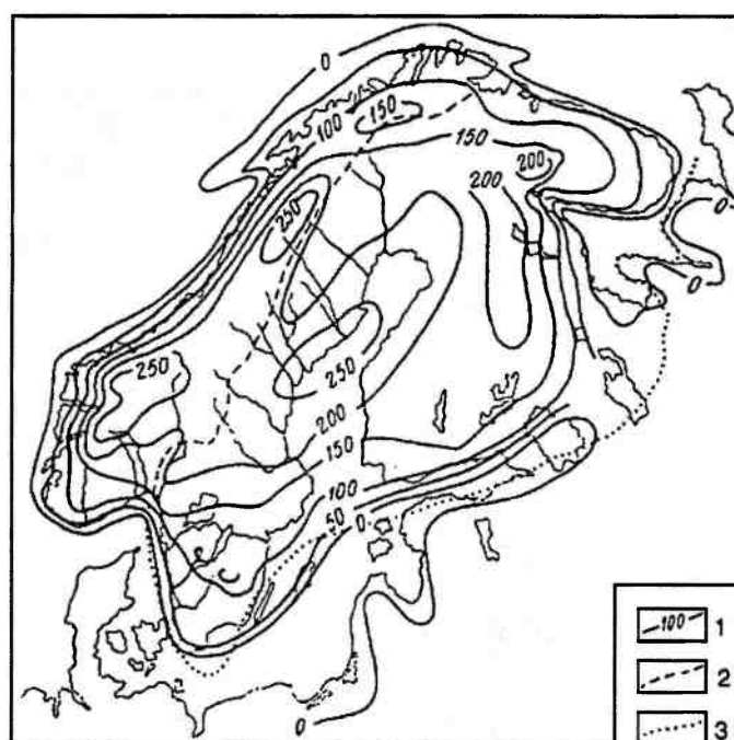
Рис. 2.12. Гляциоизостатическое поднятие Балтийского щита после исчезновения последних ледников 8–7 тыс. лет назад (по Н. И. Николаеву): 1 — изогипсы в метрах, 2 — граница каледонид Норвегии, 3 — граница Балтийского щита
