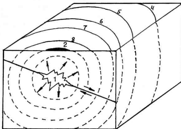
Рис. 18.1. Очаг землетрясения и распространения сотрясений в объеме породы. 1 — область очага, или гипоцентр, 2 — проекция гипоцентра на поверхность Земли — эпицентр. Линии изосейст на поверхности — линии равных сотрясений в баллах
