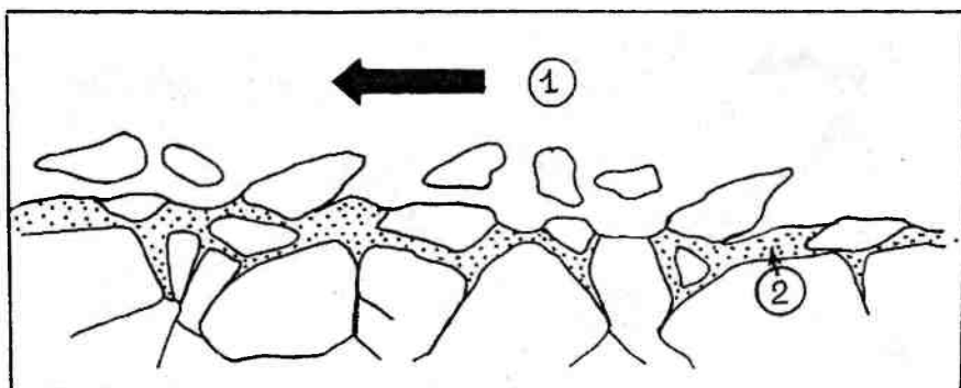
Рис. 12.12. Схема образования донной морены. Нижняя часть льда пластична с температурой, близкой к 0 °С. Вода, проникая по трещинам, замерзая, откалывает глыбы пород, которые вовлекаются в движение льда. 1 — направление движения льда, 2 — вода в трещинах пород ложа ледника
