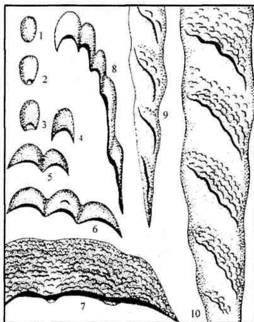
Рис. 11.4. Схема развития основных форм рельефа оголенных песков (по Б. А. Федоровичу): 1 — барханная лепешка (щитовидная дюна); 2 — эмбриональный бархан; 3 — молодой бархан; 4 — полулунный бархан; 5 — парный бархан; 6 — барханная цепь; 7 — крупная комплексная барханная цепь; 8 — групповой бархан, переходящий в продольную ветру барханную грядку; 9 — барханная продольная гряда с диагональными ребрами; 10 — крупная продольная гряда с комплексными диагональными ребрами
