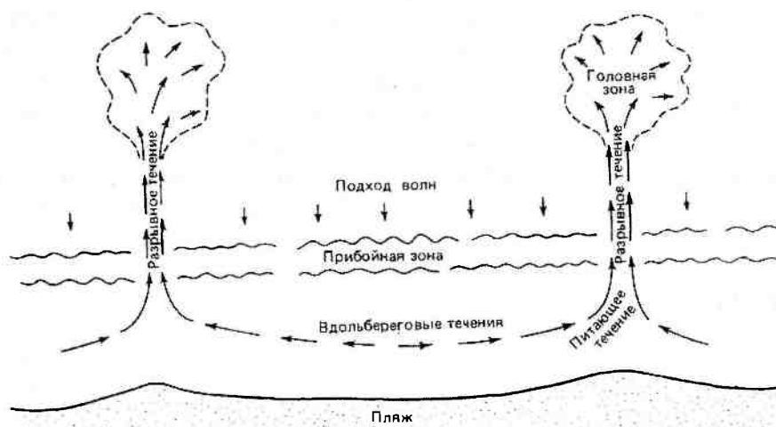
Рис. 14.32. Образование разрывного течения (сулоя) при наличии вдольбереговых течений
