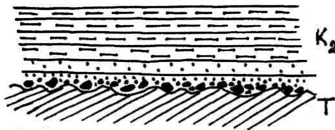
Рис. 14.63. Пример углового несогласия. Отложения верхнего мела с несогласием залегают на деформированных отложениях триаса. Отсутствуют отложения юрской системы и нижнего отдела меловой системы. Базальный горизонт состоит из обломков пород триасовой системы
