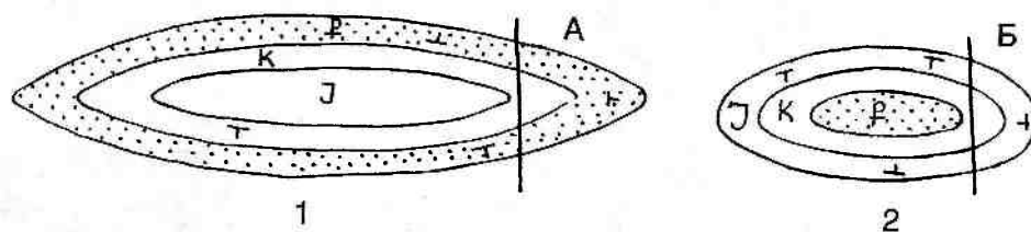
Рис. 17.20. Складки в плане. 1 — линейная антиклинальная складка, 2 — брахискладка синклиная. А — периклиналь — замыкание антиклинальной складки. Б — центриклиналь — замыкание синклиальной складки
