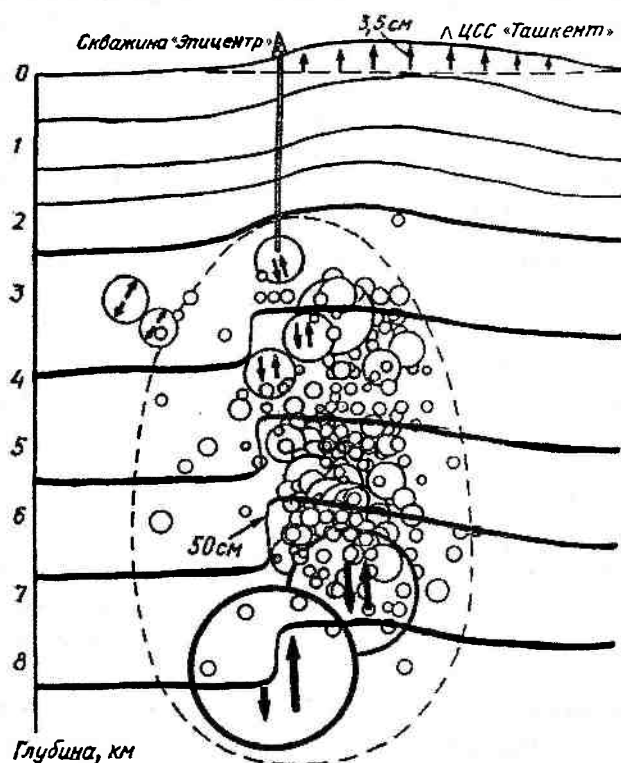
Рис. 18.6. Очаговая область ташкентского землетрясения 1966 г. под городом. Большие круги — место главного толчка, более мелкие — афтершоки. Стрелки — направление подвижек. У поверхности стрелки — величина вспучивания, по данным повторного нивелирования
