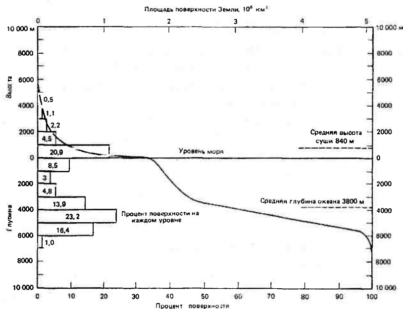
Рис. 14.18. Распределение площадей по высотным уровням. Гипсографическая кривая поверхности Земли, построенная по гистограмме частоты встречаемости (слева), показывает долю (в %) поверхности, лежащей выше или ниже любого уровня (по W. A. Anikuchine, R. W. Sternberg, 1973)
