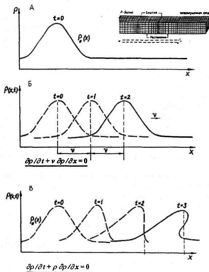
Рис. 21.2. Динамическая линейность и нелинейность: А — единичное возмущение поля плотности (по оси x — расстояние, по оси P — плотность); Б, В — перемещение продольной волны: Б — линейное, В — нелинейное (по С. П. Курдюмову, Г. Г. Малинецкому, с изменениями)
