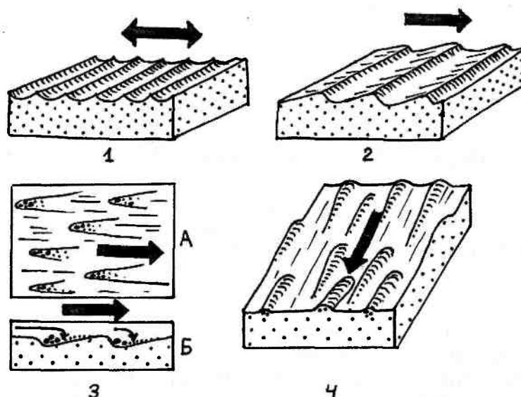
Рис. 14.37. Знаки ряби и образование иероглифов. 1 — осциляционное движение воды, знаки ряби симметричные; 2 — однонаправленное быстрое движение воды, знаки ряби асимметричные; 3–4 — образование иероглифов. Формирование углублений за счет вращения более крупных обломков или песчинок: А — план, Б — поперечный разрез; 4 — иероглифы в перевернутом пласте песчаника, подошва пласта — сверху. Черные стрелки указывают направление движения воды
