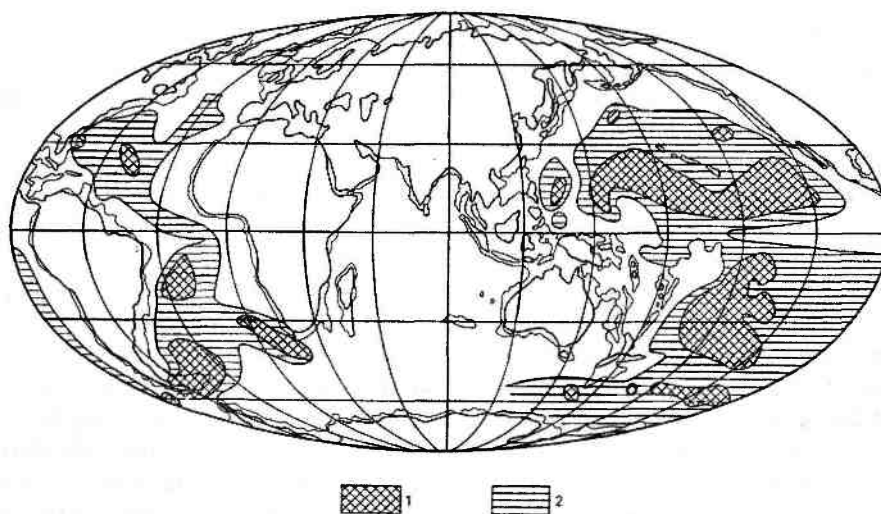
Рис. 14.59. Распространение железомарганцевых конкреций в Тихом и Атлантическом океанах: 1 — плотное покрытие дна конкрециями, местами более 905; 2 — конкреции встречаются часто, хотя распределены неравномерно (по Дж. П. Кеннету, 1987)
