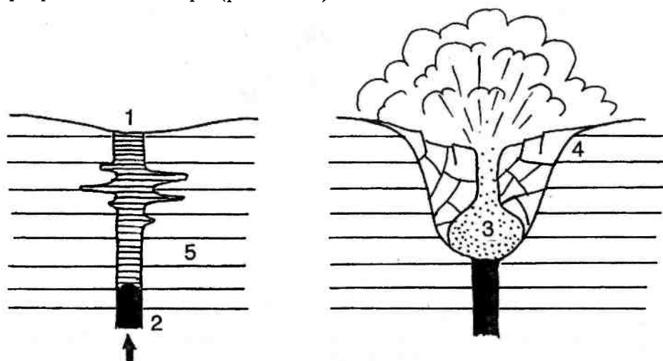
Рис. 15.44. Образование маара. 1 — вода; 2 — магма; 3 — взрыв вскипевшей воды, образование воронки и раздробление пород; 4 — воронка; 5 — коренные породы
