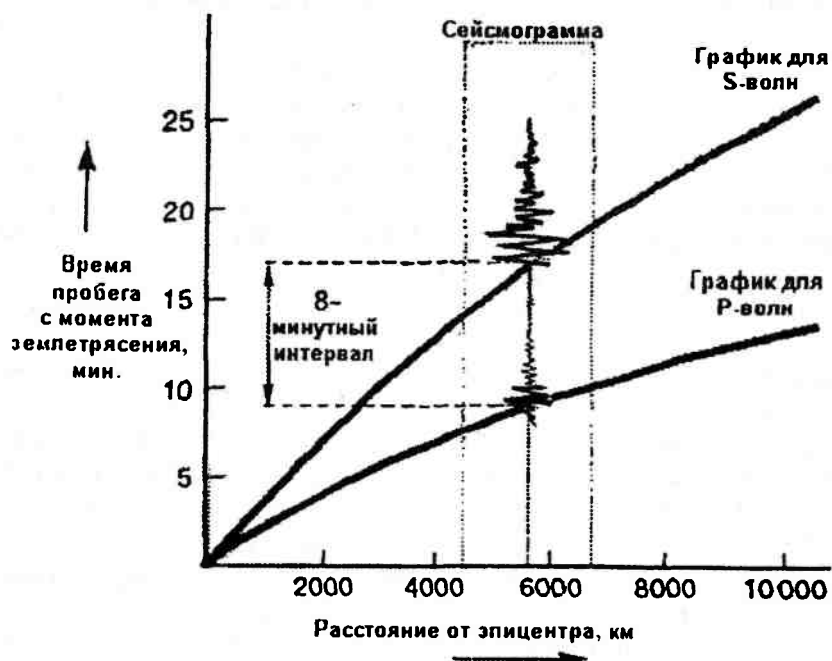
Рис. 18.3. Время пробега сейсмических волн от эпицентра землетрясения, используемое для определения расстояния от эпицентра до точки регистрации землетрясения
