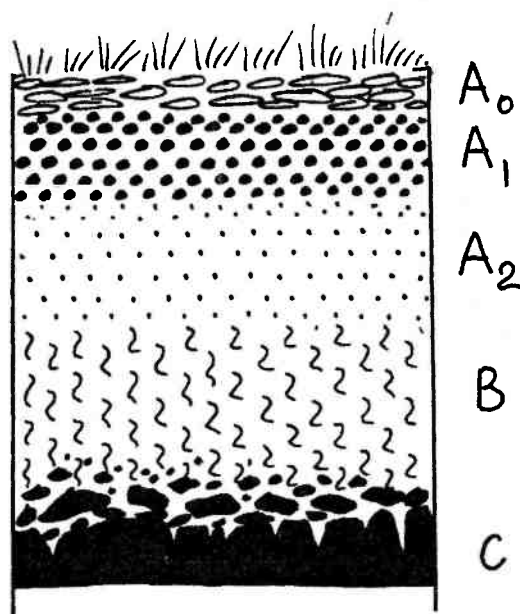
Рис. 5.7. Нормальный почвенный профиль. Горизонты:
