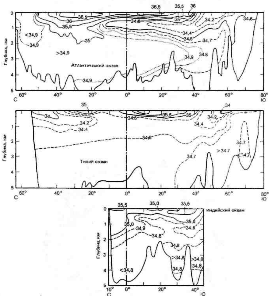
Рис. 14.6. Изменение солености по вертикали в трех океанских бассейнах (по G. Dietrich, 1963)
