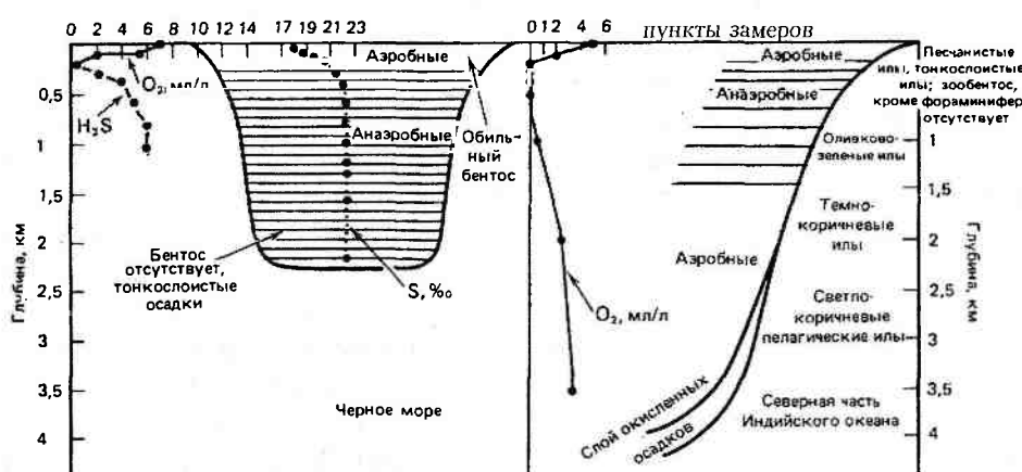
Рис. 14.58. Схема аэробных-анаэробных водных масс и их влияние на распространение осадков в Черном море и в северной части Индийского океана (J. Thiede, Tj. H. Van Andel, 1977)
