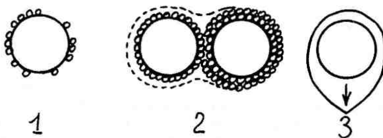
Рис. 7.1. Типы воды: 1 — прочносвязанная, 2 — рыхлосвязанная, 3 — гравитационная
