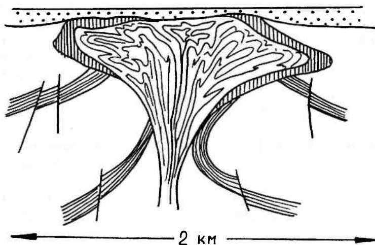
Рис. 17.15. Строение соляного купола, ядро которого очень сильно дислоцировано, а по краям — оторочка гипса (вертикальная штриховка)
