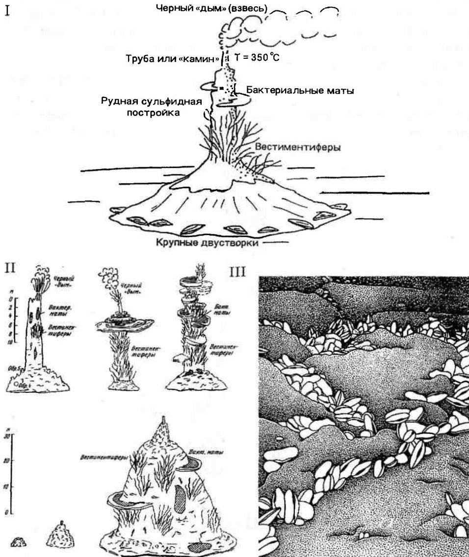
Рис. 14.48. Строение «черного курильщика» — современной «фабрики руды» на дне океана (I). Разные типы «курильщиков» (по А. П. Лисицыну и др., 1990) (II). (III) Галапагосский рифт. Цепочки крупных двустворок Caliptogenos вблизи трещин у «черных курильщиков», из которых просачивается разбавленный гидротермальный раствор (по данным Л. Лобье)
