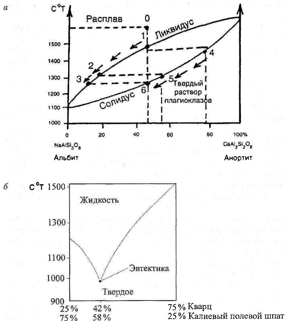
Рис. 15.2. а — диаграмма плавкости для твердых растворов плагиоклазового ряда (по Н. Боуэну). Давление P = 1 атм. Состав выделившихся из расплава кристаллов определяется на оси. Точки 1, 2, 3, 4, 5 и 6 обозначают разные стадии кристаллизации расплава; б — эвтектика — плавление двух минералов при минимальной температуре
