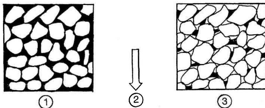
Рис. 7.4. Влагоемкость и водоотдача. 1 — полная влагоемкость, все поры заполнены водой; 2 — водоотдача, гравитационная вода стекла; 3 — максимальная молекулярная влагоемкость: вода удерживается силами молекулярного сцепления. Разница между объемами воды в 1 и 3 называется водоотдачей
