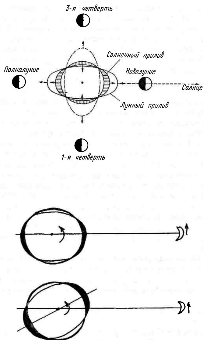
Рис. 14.14. Образование приливов в океанах на Земле. Положение приливных выступов при отсутствии (вверху) и наличии (внизу) трения
