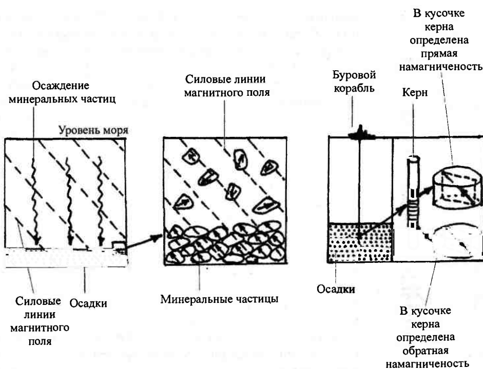
Рис. 2.16. Схематические рисунки, показывающие приобретение осадочными породами остаточной намагниченности и определение ее в кернах буровой скважины
