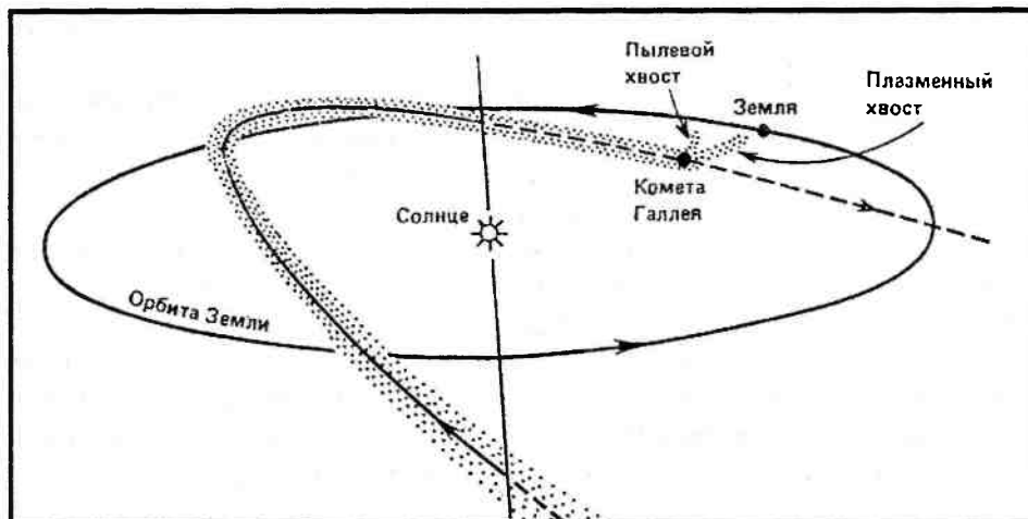
Рис. 1.12. Положение кометы Галлея при сближении ее с Землей в марте 1986 г. Схема образования у нее плазменного хвоста (направлен от Солнца), пылевого хвоста (мельчайших частичек пыли) и пылевого шлейфа (более крупных частиц железосиликатной пыли, рассеивающихся вдоль кометной орбиты)
