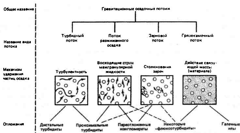
Рис. 14.43. Классификация подводных гравитационных потоков (по G. V. Middleton, M. A. Hampton, 1976)
