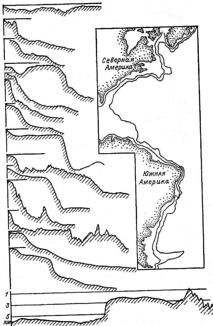
Рис. 14.26. Профили рельефа атлантических континентальных окраин Северной и Южной Америк (В. М. Литвин, 1987)
