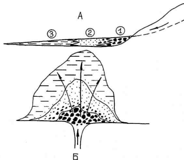
Рис. 6.9. Пролувиальный конус выноса. А — продольный профиль: 1 — наиболее грубые отложения — валунные, 2 — песчанистый материал, 3 — глинисто-песчаный. Б — план. Стрелки — направления движения масс
