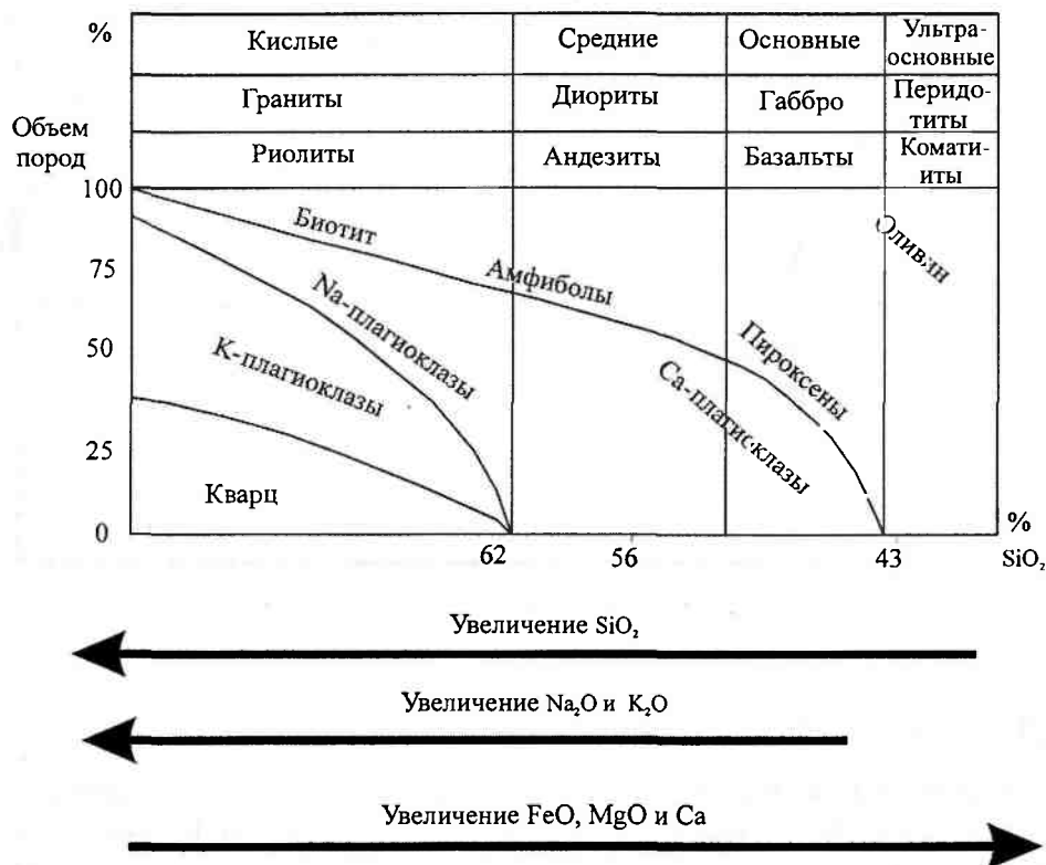
Рис. 15.4. Классификация наиболее распространенных интрузивных пород. Приведены вулканические породы, аналоги интрузивных
