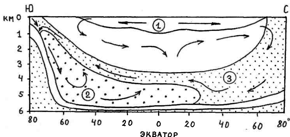
Рис. 14.13. Распределение течений воды в продольном разрезе Атлантического океана. Холодные арктические и антарктические воды располагаются в глубоких частях океана. 1 — теплая вода; холодные воды: 2 — антарктические, 3 — арктические
