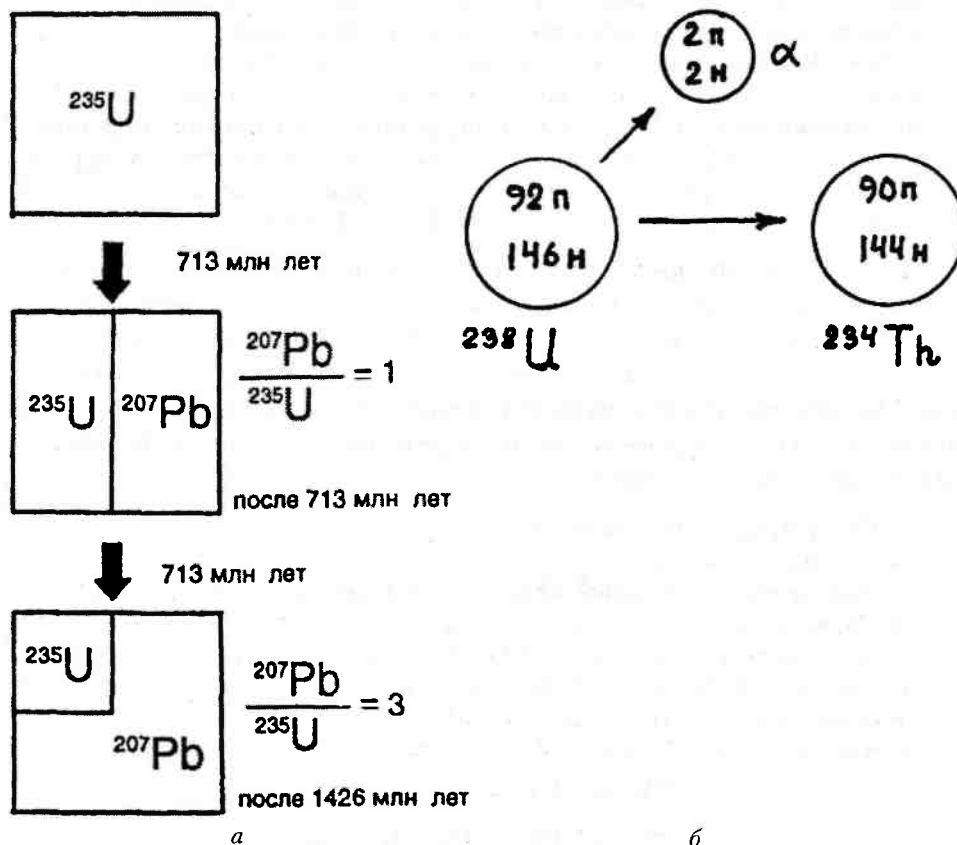
Рис. 3.8. Радиоактивный распад а — урана 235 и б — урана 238
