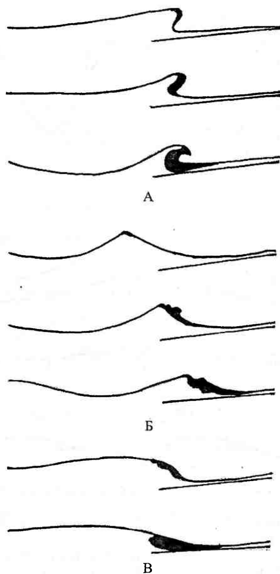
Рис. 14.16. Различные типы обрушения гребня волны: А — ныряющий, Б — стекающий, В — выступающий. Забурунивание показано черным цветом
