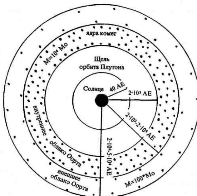
Рис. 1.8. Строение Солнечной системы. АЕ — одна астрономическая единица (150 млн км)
