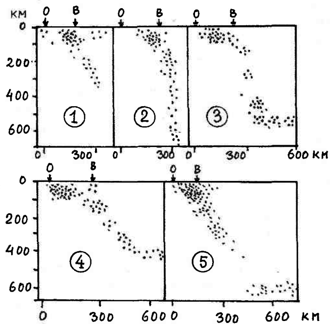
Рис. 18.8. Зоны Беньофа. Гипоцентр с 1954 по 1969 гг.: 1 — Алеутская дуга, 2 — Северо-Марианская дуга, 3 — Южная Илзу-Бонинская дуга, 4 — Северная Илзу-Бонинская дуга, 5 — Ново-Гейбридская дуга, 0 — ось желоба, В — вулканы
