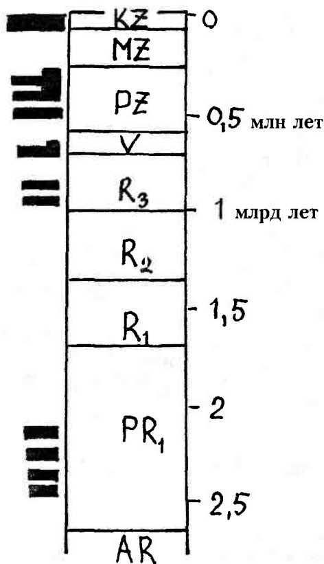
Рис. 12.20. Основные криогенные (ледниковые) эпохи в истории Земли (черные)
