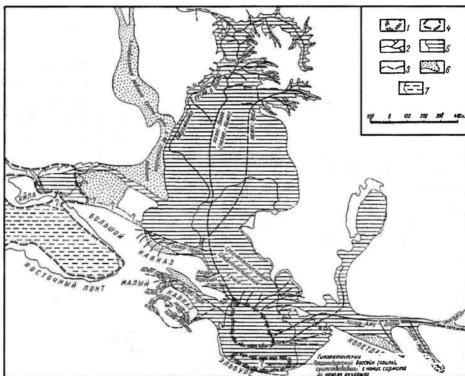
Рис. 6.25. Палеогеографическая схема Каспийского и Черноморского бассейнов для среднего и начала позднего плиоцена (акчагыл) (по Е. Е. Минановскому).
