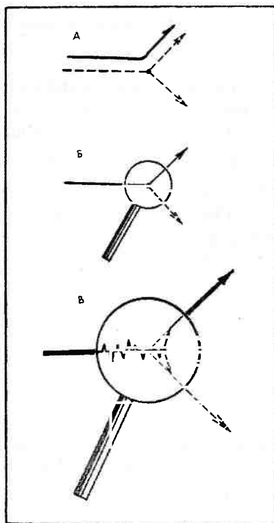
Рис. 21.4. Точка бифуркации и ее окрестности (А); последовательное увеличение детальности изучения (Б, В) выявляет предбифуркационные флуктуации траектории, но сама точка бифуркации остается точкой с непредсказуемым выбором в ней одной из исходящих траекторий
