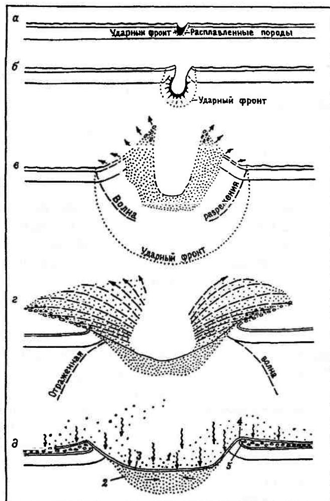
Рис. 16.6. Стадии образования взрывного (метеоритного) кратера (по Л. Н. Хряниной, 1987): а–в — I стадия — ударное сжатие, растекание метеорита в грунте; г — II стадия — экскавация и выброс грунта отраженной волной; д — III стадия — деформация или заполнение (1 — воронка, 2 — истинное дно, 3 — видимое дно, 4 — вал брекчии, 5 — лежащая синклиналь цокольного вала)
