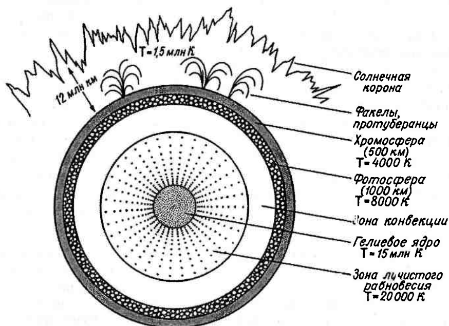
Рис. 1.4. Внутренняя структура Солнца
