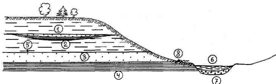
Рис. 7.3. Схема залегания грунтовых вод: 1 — верховодка (водоносный временный горизонт), 2 — локальный водоупор, 3 — водоносный горизонт, 4 — водоупорный горизонт, 5 — зеркало грунтовых вод, 6 — река, 7 — аллювий, 8 — родник
