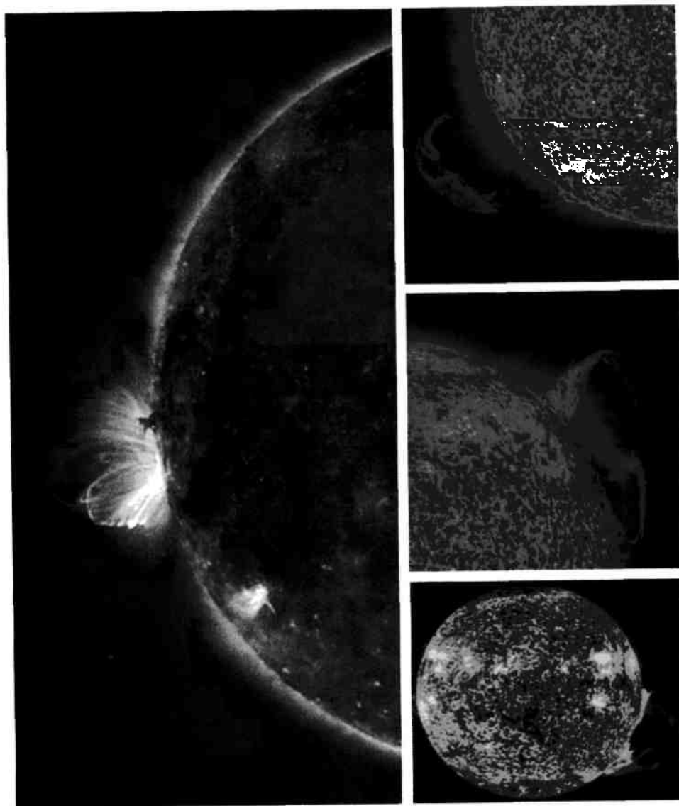
Рис. 1. Петли и протуберанцы над поверхностью Солнца. Проект SOHO
