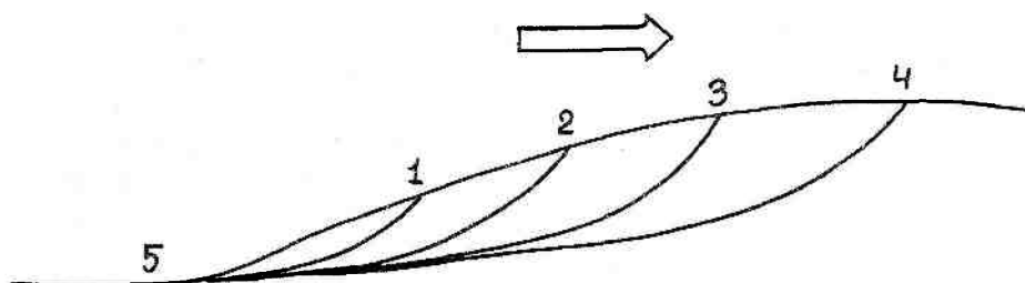
Рис. 6.3. Пятящаяся эрозия оврага. Стрелкой указано направление роста оврага. Стадии роста отмечены цифрами. 5 — базис эрозии оврага
