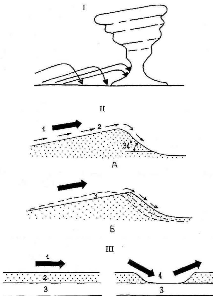
Рис. 11.1. Разрушение и аккумуляция сыпучего материала при эоловых процессах. I — корразия. Песчинки, перемещающиеся ветром путем сальтации (прыжками), обтачивают выступы горных пород. II.A — образование бархана. 1 — ветер; 2 — песок; 34^\circ — угол естественного откоса сыпучих тел — подветренный склон; Б — перемещение бархана — пунктир; 3 — зона ветровой эрозии песка. III — образование котловин выдувания: 1 — ветер; 2 — песок; 3 — увлажненный грунт; 4 — котловино выдувание
