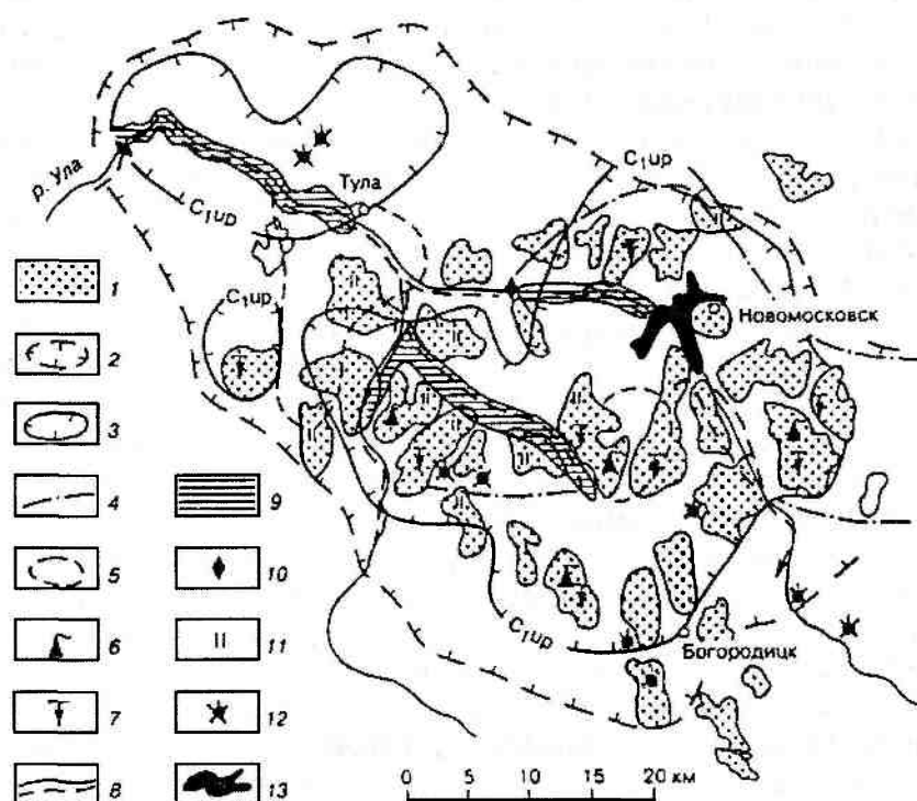
Рис. 20.2. Схема техногенной измененности территории Центрального Москбасса (по материалам ПЛОГСа геологического факультета МГУ). 1 — площади деформированных земель (мульды оседания, провалы, трещины, уступы); 2 — граница областей речных бассейнов с изменившейся структурой водного баланса; 3–5 — границы (на 1979 г.) депрессионных воронок водоносных горизонтов (3 — упинского, 4 — яснополянского); 6 — горячие терриконы; 7, 8 — участки техногенного загрязнения грунтовых и поверхностных вод соответственно; 9 — участки рек с инверсией подземного стока; 10 — изменение речного стока (более 50 %) под влиянием сточных вод; 11 — техногенное заболачивание; 12 — техногенная активизация карстово-суффозионных процессов; 13 — Шатское водохранилище
