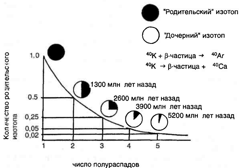
Рис. 3.9. Распад радиоактивного изотопа ^{40}\text{K} имеет два пути, превращаясь в ^{40}\text{Ar} или в ^{40}\text{Ca}
