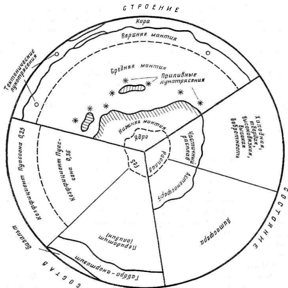
Рис. 1.16. Строение, состояние и состав лунных недр (по А. Т. Базилевскому и др., 1981)
