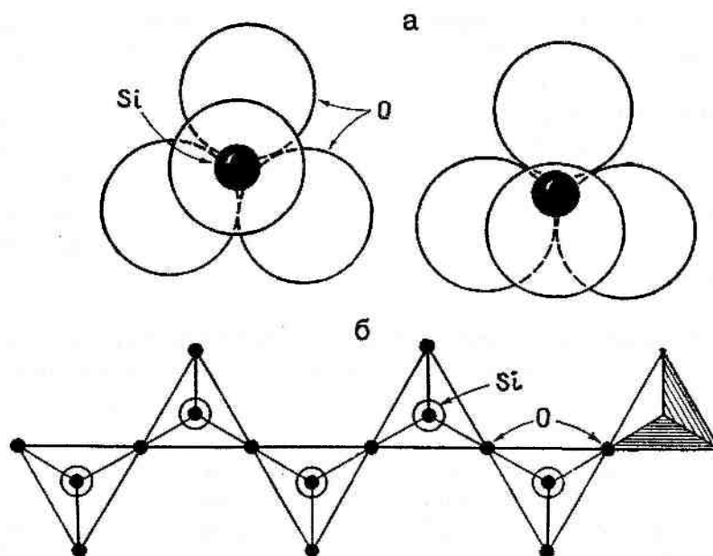
Рис. 2.21. Структура кремнекислородного тетраэдра: а — одиночный; б — соединенные в цепочку
