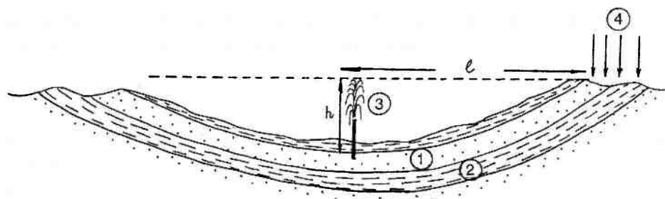
Рис. 7.8. Артезианские напорные воды: 1 — водоносный горизонт, 2 — водоупорный горизонт, 3 — фонтанирующая скважина, 4 — осадки, h/l — напорный градиент
