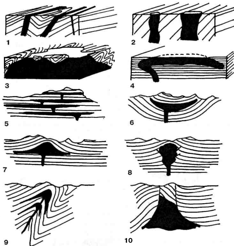
Рис. 15.7. Формы интрузивных тел. 1 — дайки, 2 — штоки, 3 — батолит, 4 — гарполит, 5 — многоярусные силлы, 6 — лополит, 7 — лакколлит, 8 — магматический диапир, 9 — факолит, 10 — бисмалит
