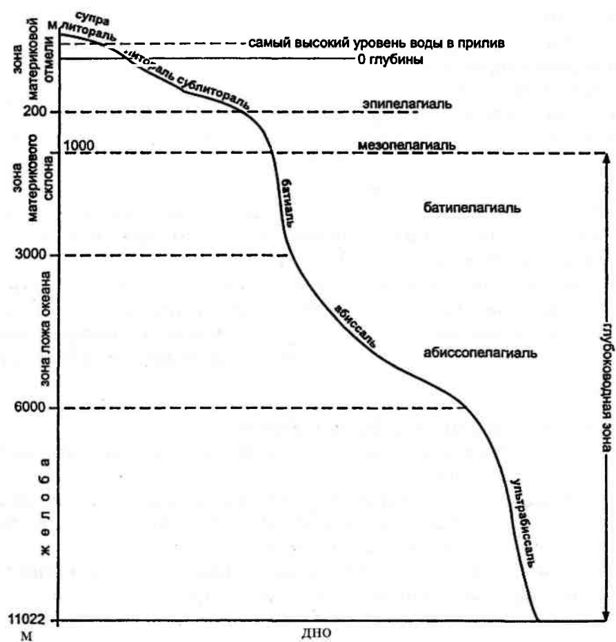
Рис. 14.41. Схема вертикальной зональности Мирового океана
