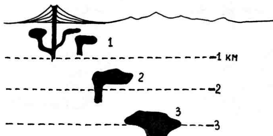
Рис. 15.6. Подразделение интрузивов по глубине формирования. 1 — субвулканические (близповерхностные), до 1 км, 2 — гипабиссальные (среднеглубинные), 1–2 км, 3 — абиссальные (глубинные), глубже 2–2,5 км
