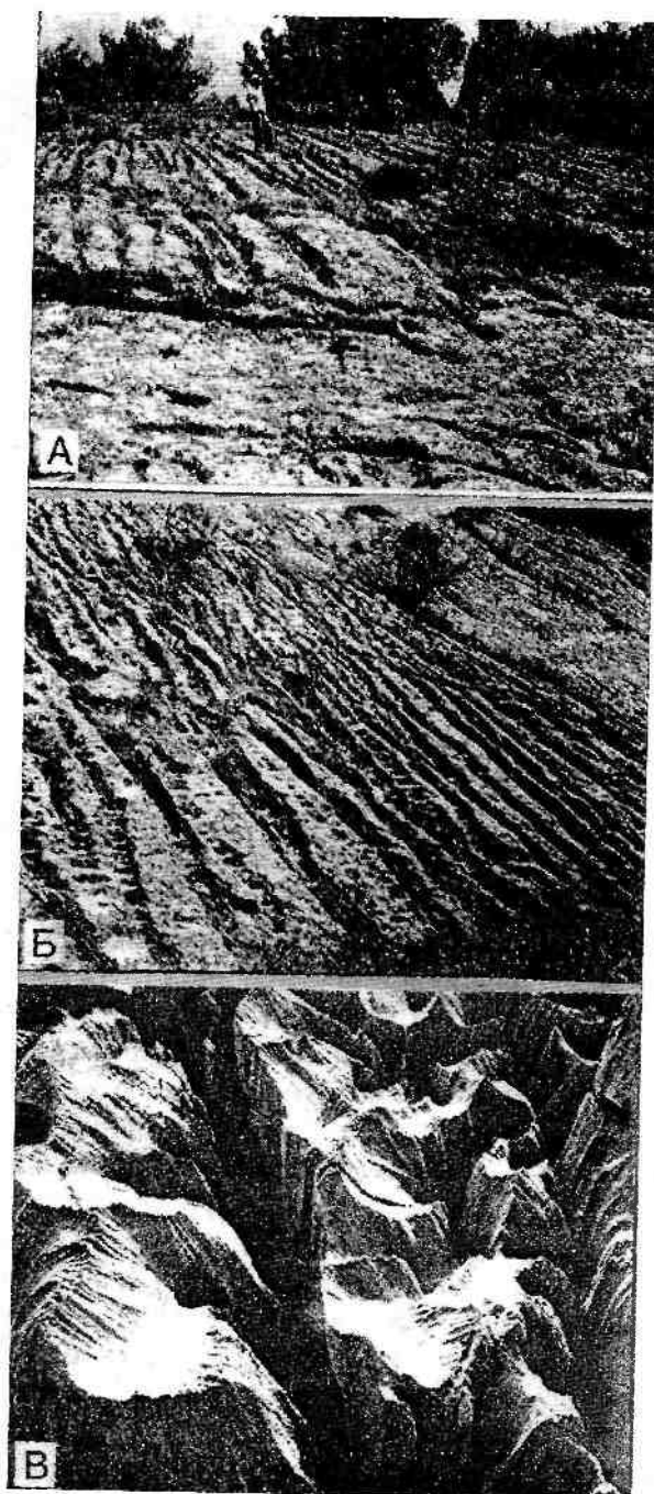
Рис. 8.2. А — карры в ущелье Кульсу (по Н. А. Гвоздецкому); Б — развитие карров и каррового ландшафта (по Бондарчуку); В — деталь каррового поля
