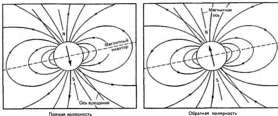
Рис. 2.14. Силовые линии дипольного магнитного поля Земли. Слева — нормальная полярность, справа — обратная
