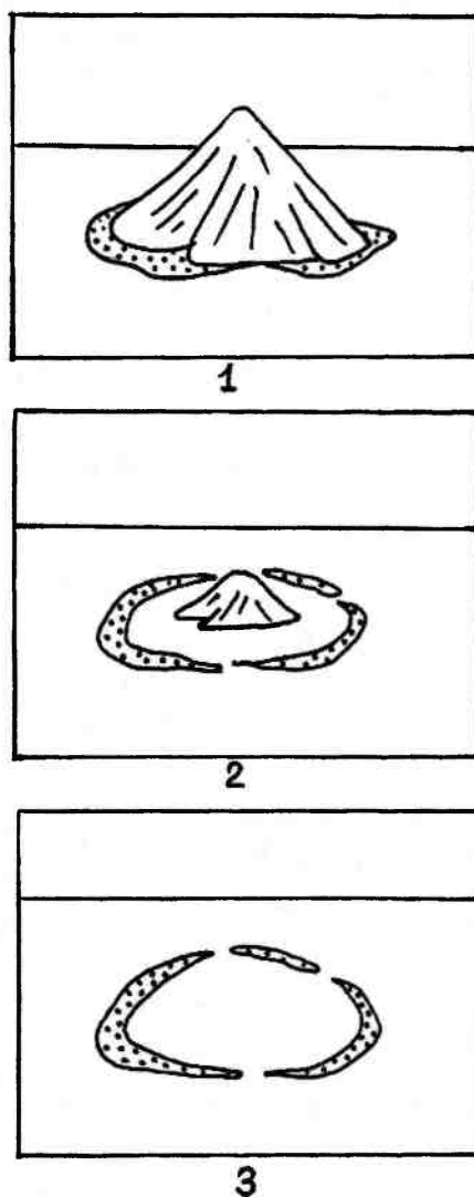
Рис. 14.53. Формирование атолла. 1 — вулкан, окруженный кольцевым рифом; 2 — погружение вулкана и образование кольцевого рифа; 3 — на месте опустившегося вулкана образовалась лагуна
