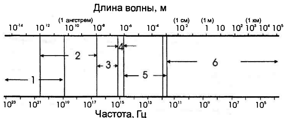
Рис. 1.6. Электромагнитный спектр: 1 — гамма-лучи; 2 — рентгеновские лучи; 3 — ультрафиолетовые лучи; 4 — видимый свет; 5 — инфракрасные лучи; 6 — радиоволны. Скорость электромагнитных волн в вакууме — 299,793 км/с
