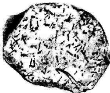
Рис. 3.11. Кристалл апатита с треками спонтанного деления урана, увеличенными путем химического травления. Возраст остывания данного кристалла — 60–70 млн лет назад. Фото любезно предоставлено профессором Дж. И. Гарвером (Юнион Колледж, Скенектади, США)
