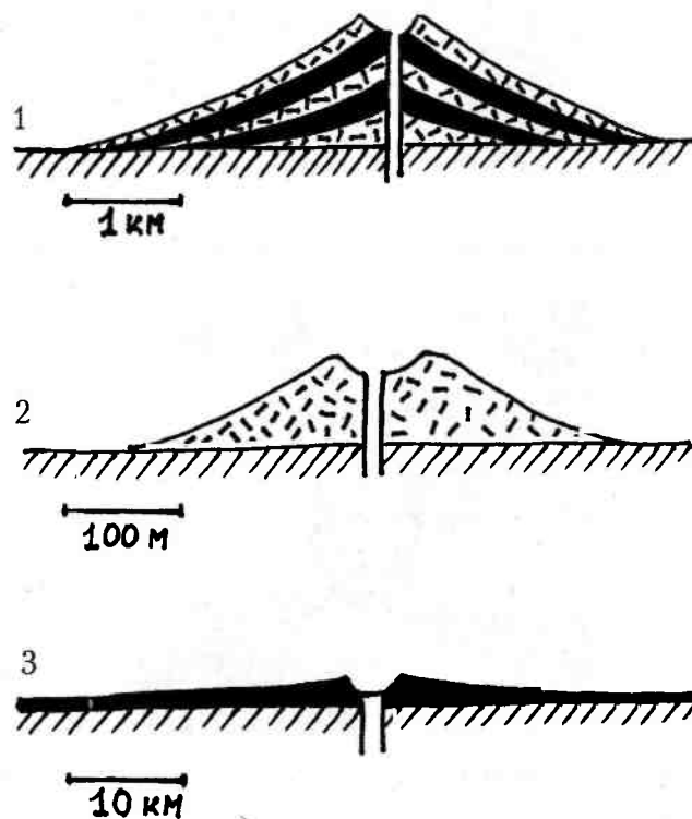
Рис. 15.26. Типы вулканов: 1 — стратовулкан (слоистый полигенный вулкан), чередование лав (черное) и туфов (штрихи); 2 — шлаковый вулкан (моногенный); 3 — щитовой лавовый вулкан
