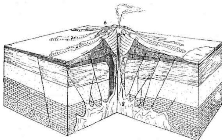
Рис. 15.29. Схема строения стратовулкана. 1, 2, 3 — разные вулканические толщи, образующие конус вулкана; 4 — молодой вулканический конус, выросший после взрывного извержения и образования кальдеры; 5 — широкое жерло, образовавшееся во время взрыва; 6 — край кальдеры; 7 — молодые лавовые потоки; 8 — близповерхностный магматический очаг; 9 — молодой вулканический канал, заканчивающийся кратером
