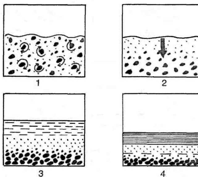
Рис. 14.45. Образование градационной слоистости во флишевых отложениях.
