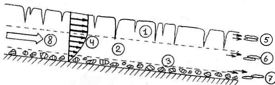
Рис. 12.5. Продольный разрез части горного ледника: 1 — зона хрупкого льда; 2 — зона пластичного льда; 3 — зона вмороженных в лед валунов; 4 — кривая скоростей движения льда; 5 — зерна льда, движущиеся вместе; 6 — верхние зерна опережают нижние; 7 — верхние зерна еще сильнее опережают нижние; 8 — направление движения льда
