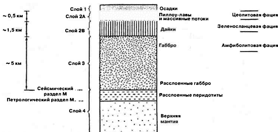
Рис. 2.28. Строение океанической земной коры
