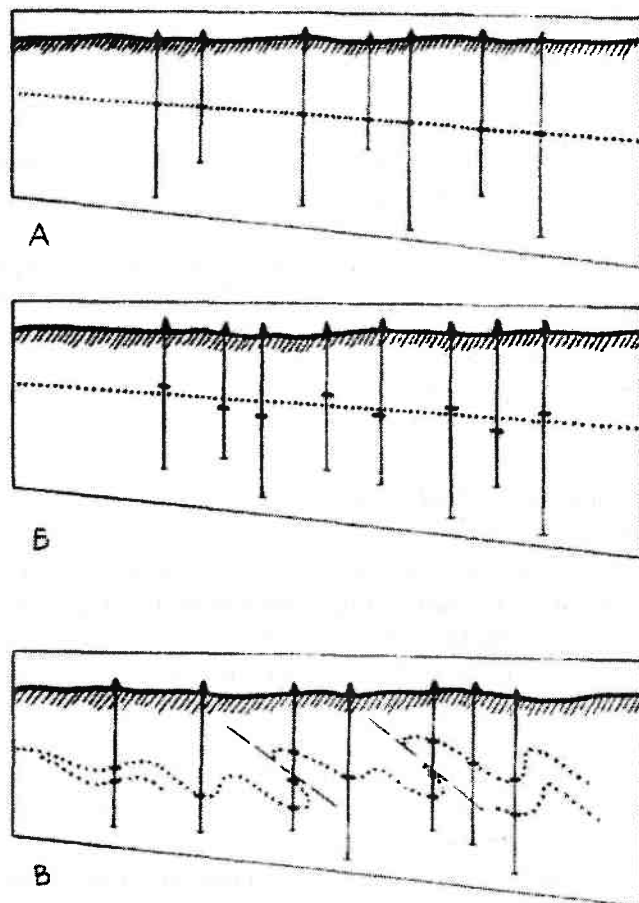
Рис. 21.1. Геометрическая линейность и нелинейность. Зависимость глубины залегания геологической границы от расстояния до некоторой начальной точки:
