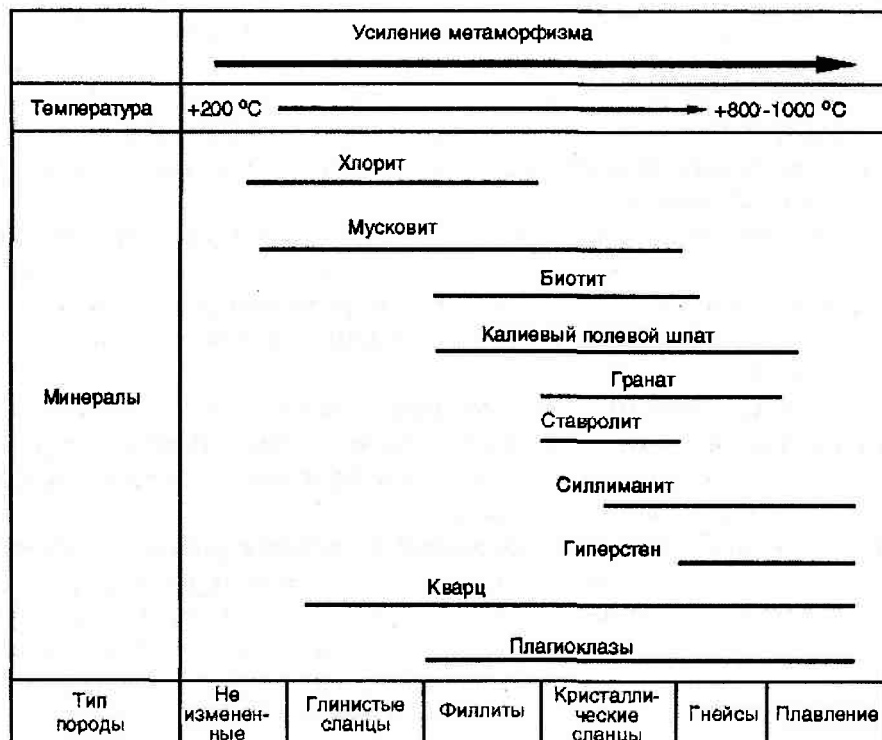
Рис. 16.4. Новообразование минералов при прогрессивном метаморфизме
