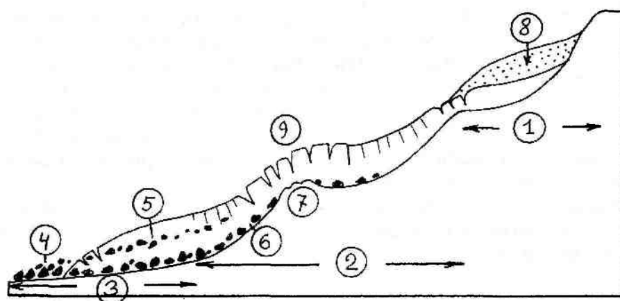
Рис. 12.2. Схема строения горного ледника. 1 — область аккумуляции; 2 — область движения; 3 — область разгрузки. Морены: 4 — конечная; 5 — срединная; 6 — донная; 7 — ригель; 8 — снег; 9 — кривасы (трещины)
