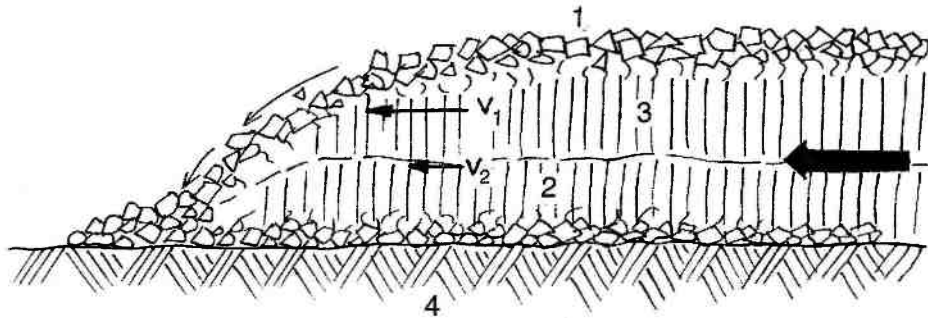
Рис. 15.15. Строение лавового потока среднего состава в продольном разрезе. Черная стрелка обозначает направление движения лавового потока. Тонкие стрелки — обвал глыб с фронта потока. 1 — верхняя лавобрекчия — аа-лавы, 2 — нижняя лавобрекчия, 3 — столбчатая отдельность, 4 — субстрат
