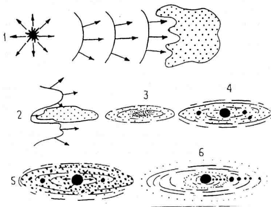
Рис. 1.15. Формирование Солнечной системы.
