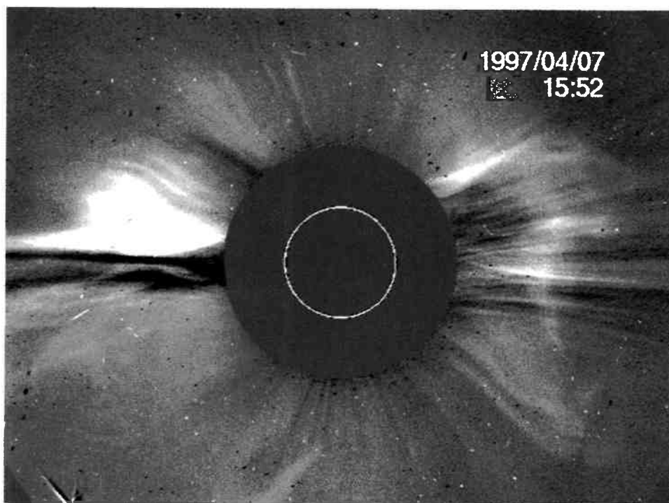
Рис. 2. Солнечная корона (диск Солнца закрыт). Видны выбросы солнечной плазмы. (Проект SOHO)
