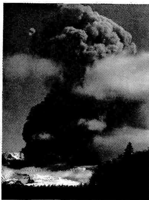
Рис. 15.41. Грандиозное эксплозивное извержение вулкана Шивелуч в апреле 1991 г. (Камчатка). Высота пепловых туч — 9–10 км (фото Н. П. Смелова)
