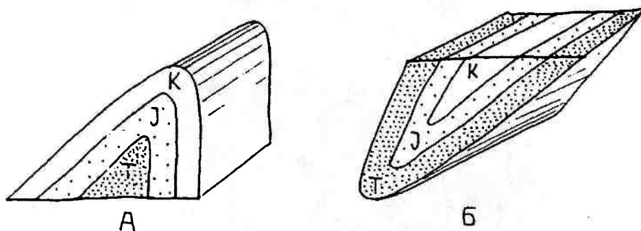
Рис. 17.9. Антиклинальная (А) и синклинали (Б) складки.
