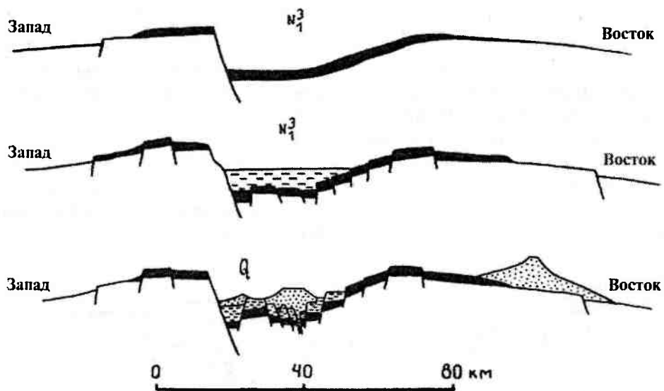
Рис. 17.26. Схематические профили, показывающие развитие Кенийского сложного грабена (Восточная Африка) с позднего миоцена до современности. Черные точки и штрихи — вулканические покровы разного возраста
