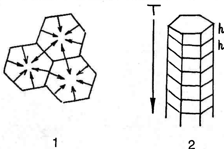
Рис. 15.18. Образование столбчатой отдельности. 1 — план. Сначала «выживают» центры охлаждения, и к ним направлено сжатие; 2 — разрез. По мере падения температуры ( T ) термонапряжение превышает предел прочности породы и возникает трещина на величину h . И далее процесс продолжается непрерывно, но скачками
