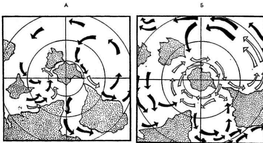
Рис. 14.10. Образование Циркум-Антарктического холодного течения благодаря перемещению литосферных плит. Белые стрелки обозначают холодные воды, черные — более теплые. А — 60 млн лет назад; Б — в наши дни
