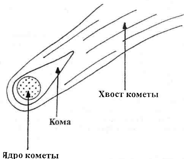
Рис. 1.11. Схема строения кометы. Хвост кометы всегда направлен в сторону от Солнца
