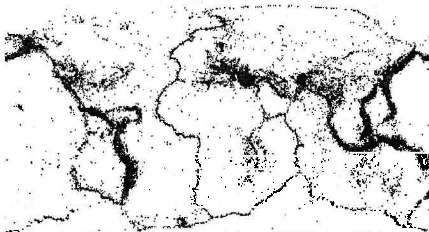
Рис. 3.14. Эпицентры землетрясений за последние 15 лет (без контуров материков)
