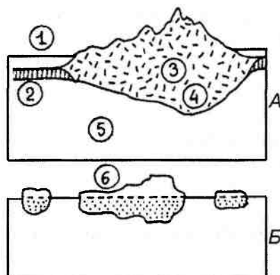
Рис. 2.10. А — «корень» гор. Чем выше горы, тем «корень» гор глубже проникает в верхнюю мантию: 1 — океан, 2 — океаническая кора, 3 — континентальная кора, 4 — «корень» гор, 5 — верхняя мантия. Б — айсберги (6), плавающие в морской воде. Над поверхностью воды возвышается 1/3 ледяной глыбы
