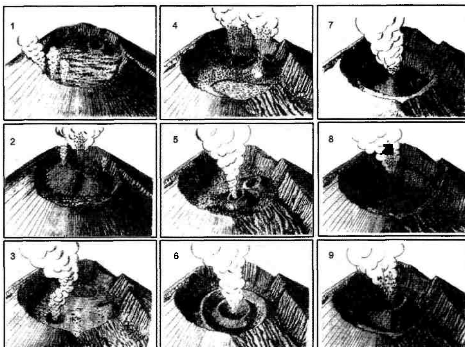
Рис. 15.30. Стадии изменения кратера Ключевского вулкана с 1936 по 1966 г. (по Н. Т. Кирсанову и А. М. Рожкову)
