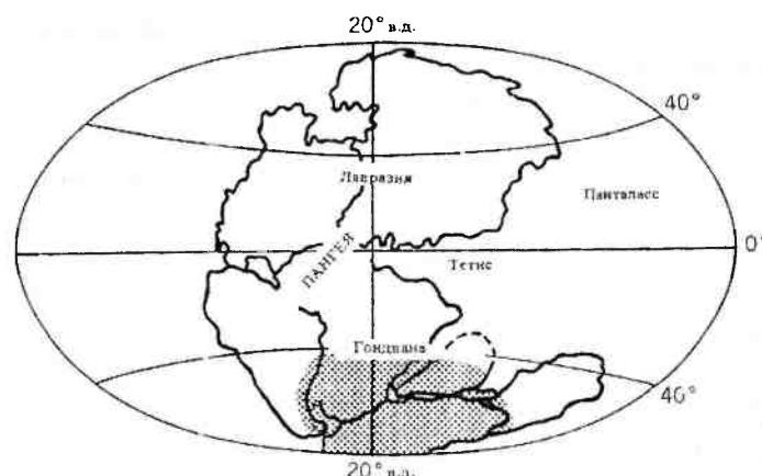
Рис. 3.25. Вегенеровская реконструкция суперконтинента Пангея около 2 млн лет назад. Панталасс («все моря») превратился в Тихий океан, а Средиземное море является остатком древнего океана Тетис. Заштрихованный участок обозначает полярные ледники, которые, как полагают, в пермское время двигались через Южную Гондвану, что объясняет существование различных форм ледникового рельефа в Южной Америке, Африке, Индии и Австралии
