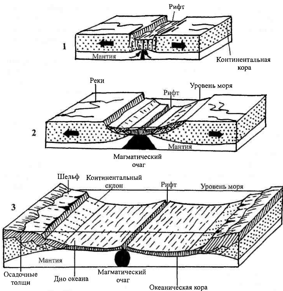
Рис. 3.16. Формирование океанической коры в результате процесса спрединга при расколе континента. 1 — начало раскола, образование рифта, внедрение даек; 2 — дальнейшее развитие рифта, образование океанической коры путем излияния базальтов из магматического близповерхностного очага (черный); 3 — разрастание океанического дна, образование пассивных континентальных окраин, формирование шельфа и континентального склона, дальнейшее функционирование рифта как места поступления базальтовых лав
