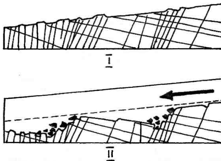
Рис. 12.10. Формирование ригелей (уступов) в днище троговой долины. I — скальное днище долины до оледенения с участками повышенной трещиноватости. II — днище долины в момент оледенения (движение ледника — черная стрелка). Трещиноватые зоны сильнее разрушаются ледниковой экзарацией
