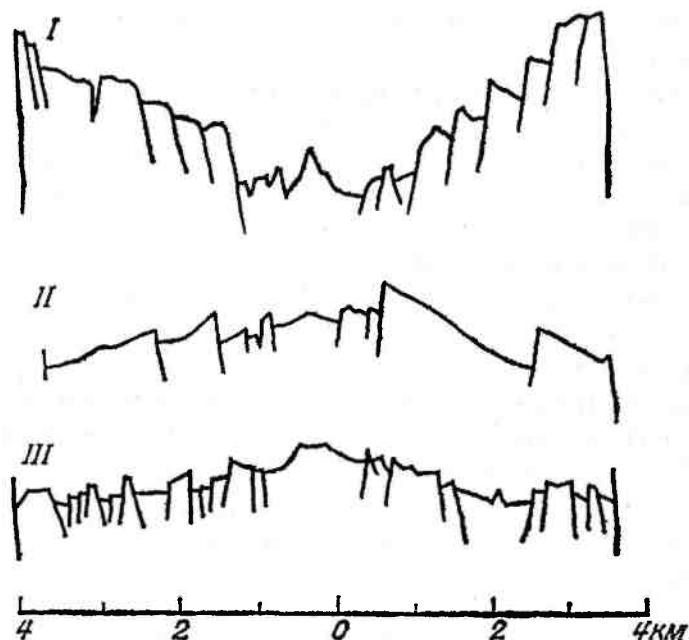
Рис. 14.22. Типичные профили осевой части рифтовой зоны. I — Атлантический хребет на 37^\circ с. ш. (скорость раздвижения 2 см/год); II — Галапагосский рифт на 86^\circ з. д. (7 см/год); III — Восточно-Тихоокеанское поднятие на 3^\circ 30' ю. ш. (15 см/год) (В. М. Литвин, 1987)
