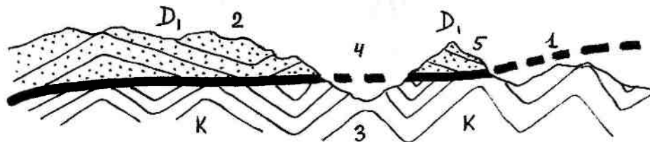
Рис. 17.28. Тектонический покров. 1 — поверхность разрыва; 2 — аллохтон (тело покрыва); 3 — автохтон; 4 — тектоническое окно; 5 — тектонический останец. D 1 — нижний девон. К — мел
