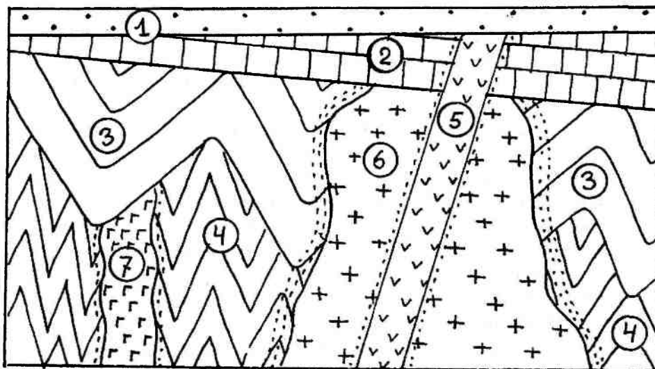
Рис. 3.1. Соотношение разновозрастных отложений и пересекающих их интрузивных тел. Цифры 1, 2, 3, 4 показывают последовательность формирования осадочных пород, толщи которых разделены угловыми несогласиями. Дайка 5 — самая молодая и внедрилась до образования толщи 1. Гранитная интрузия внедрилась до формирования толщ 2, после формирования толщ 3 и 4. Дайка 7 — самая древняя и прорывает только толщу 4
