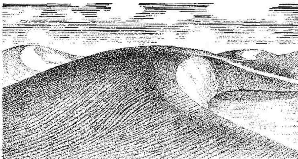
Рис. 11.3. Барханы
