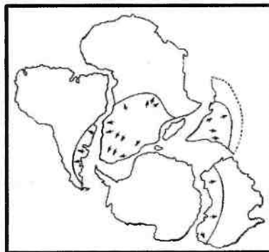
Рис. 3.24. Размещение ледниковых отложений позднего палеозоя. А — современная картина. Б — поздний палеозой, когда положение материков было другим и оледенение охватило большие участки спаянных вместе континентов в высоких широтах
