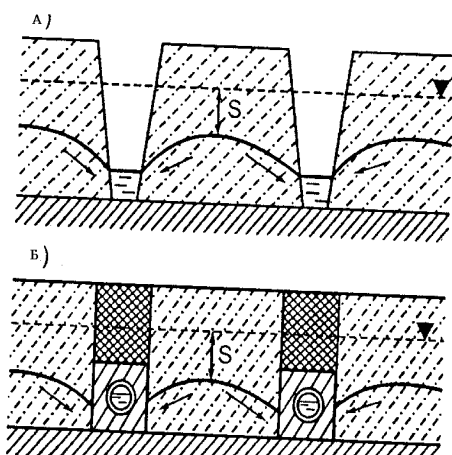
22.4.3-rasm. Zovurlargayer ostisuviniqibkelishi jarayoni (V.P.Ananev,bo'yicha). A-ochiqzovur; B-yopiqzovur)
