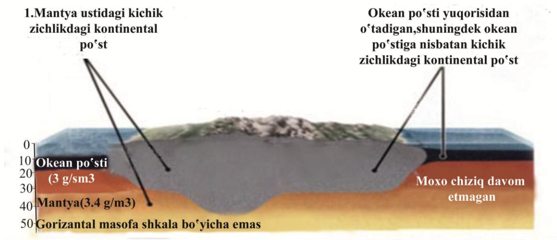
2.6-rasm Yer po'stining chegaralari.
