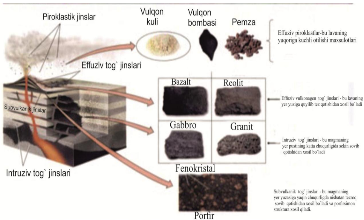
3.13-rasm. Piroklastik jinslarning hosil bo'lish jarayoni.
