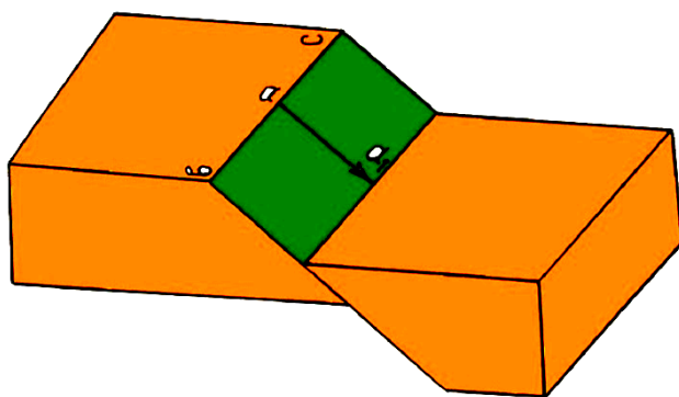
12.13-rasm. Uzilma strukturaning ko'rinishi.
