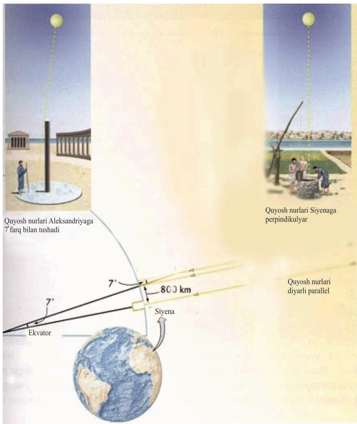
2.3–rasm. Eratosfenning Yer kattaligini oʻlchash usuli. (Understanding Earth., J. Grotzinger, T. H. Jordan, F. Press, R. Siever.)
