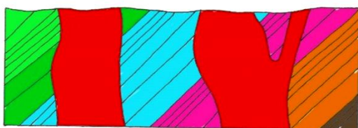
3.17-rasm. Shtoklar.
