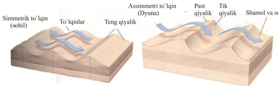
4.7-rasm. Qatlam yuzasidagi simmetrik va assimetrik to'liqin ryablari.
