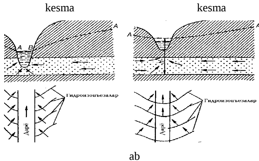
18.1-rasm. Bosimli suvlarni yer usti suv havzalari bilan ozaro aloqasi. a –bosimli suvlar oqimining daryo suvlari oqimi bo‘yicha ta’minlanishi; b –daryo suvlari oqimining bosimli suvlari oqimiga ta’minlanishi; AA–peizometrikyuza
