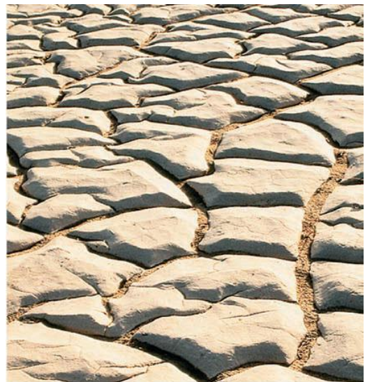
4.10- rasm. Qatlam koʻpburchakli qurish darzliklari.
