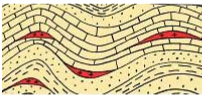
3.25-rasm. Fakolitlar.
