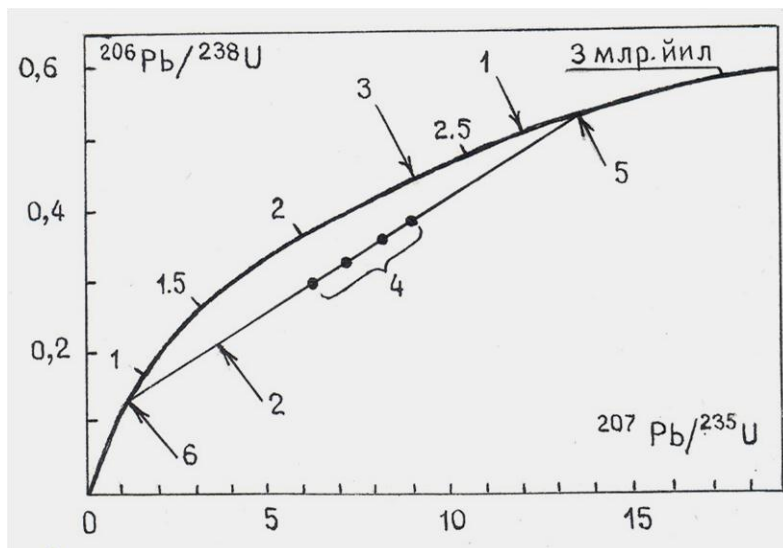
6.11-rasm. Konkordiyali izoxron diagramma: 1 - konkordiya; 2 - diskordiya; 3 - mineral yoshining konkordantli (muvofig) qiymati; 4 - diskordantli eksperimental ma'lumotlar; 5 - mineralning hosil bo'lgan vaqti; 6 - keyinroq sodir bo'lgan geologik hodisaning kechgan vaqti.
