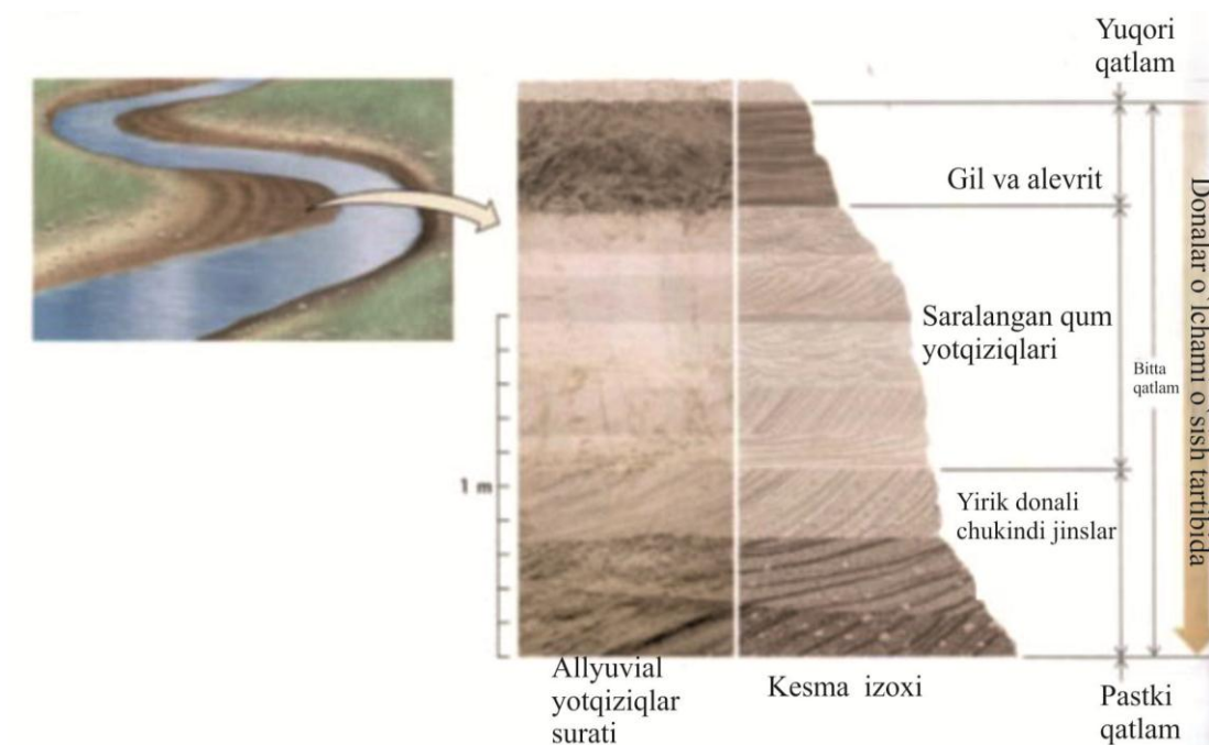
4.8-rasm. Gorizontal va qiyshiq qat-qatlik.
