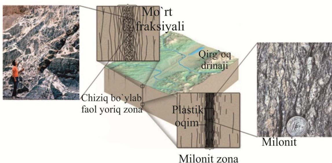
5.10-rasm. Dinamometamorfizm
