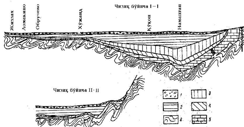
18.2-rasm. Farg'ona artezian havzasining strukturaviy geologik kesmasi (A.N.Sultonxo'jayev bo'yicha). Suvli tog' jinsiqatlamlari: 1—to'rtlamchi davr (Q); 2—quyi (Sox) to'rtlamchi ( Q_1 ) va baktriysvitasijinslari ( N_2 ); 3—massagetsvitasijinslari ( N_1 ); 4—paleogendavriyinslari (R); 5—birdavriyinslari (K); 6—paleozoydavriyinslari (Pz).
