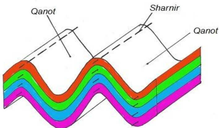
12.7-rasm. Burmalarning sharniri va qanotlari.
