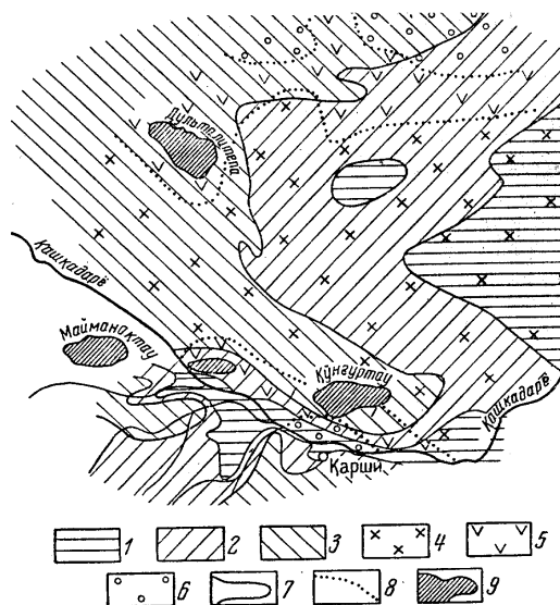
23.8-rasm. Amudaryo artezian xavzasi yer osti suvlarining minerallashish darajasini chuqurlik bo'yicha o'zgarish sxemasi (R.Ya.Boyko, G.G.Starostinalar bo'yicha)
