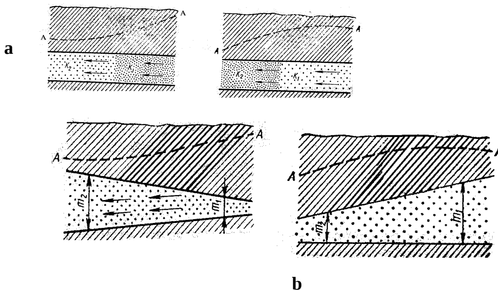
18.3.2-rasm. Bosimli suvlar p 'ezometrik yuzasi shaklini ( A-A ) tog' jins qatlamlari qalinligiga ( m ) va suv o'tkazuvchanlik xususiyatlariga ( K_p ) bog'liq xolda o'zgarishini ko'rsatuvchi sxema (G.V.Bogomolovdan). a-bosimli suvlar p 'ezometrik yuzasi shaklini tog' jinslarining suv o'tkazuvchanlik xususiyatini oshishi ( K_1 ) va kamayishi ( K_2 ) bilan o'zgarishi; b-suvli qatlamlar p 'ezometrik yuzasi shaklini, suv qatlamlar qalinligini ( m_1 ) oshishi va kamayishi ( m_2 ) bilan o'zgarishi
