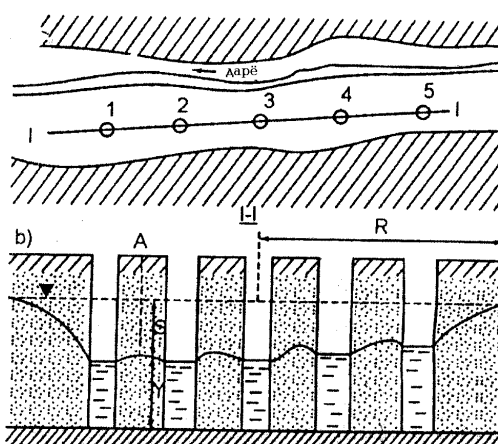
22.4.2-rasm. Daryovodiyisibo'ylab, bir yo'nqalishda joylashtirilgan suv chiqarish quduqlarinihg o'zaro ta'sir etish sxemasi.
