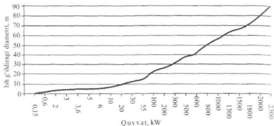
48-rasm. Shamol qurilmasi ish g'ildiragining diametri bilan uning quvvati orasidagi bog'lanish grafigi.
