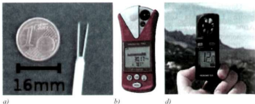
52-rasm. Issiqlik (a), ko'p funktsiyali sonli (b) va cho'ntak (d) anemometrlari.
