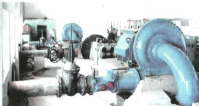
42-rasm. Gorizontaal radial-o'qiy turbinalar o'rnatilgan kichik GES binosining ko'rinishi.
