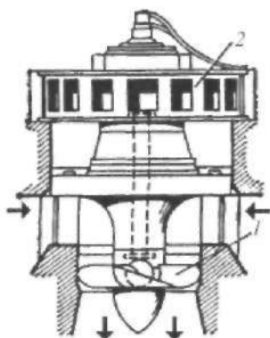
21-rasm. Gidroagregat:
