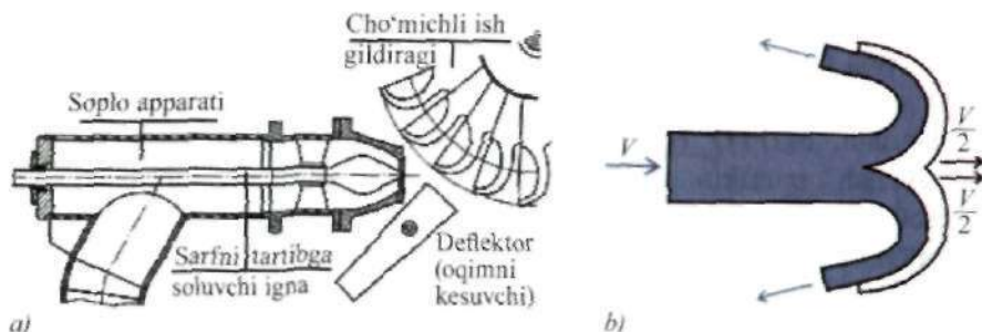
43-rasm. Cho'michli turbinaning yo'naltiruvchi moslamasi (a) hamda cho'michga suvning urilishi va tezlikning bo'linishi (b) sxemasi.
