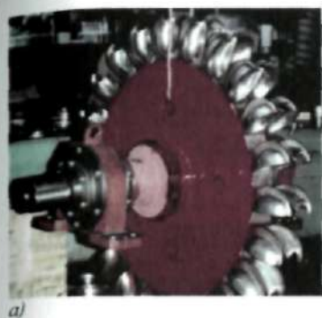
44-rasm. Osilgan (a) va yotqizilgan (b) cho'michli ish g'ildiraklari.
