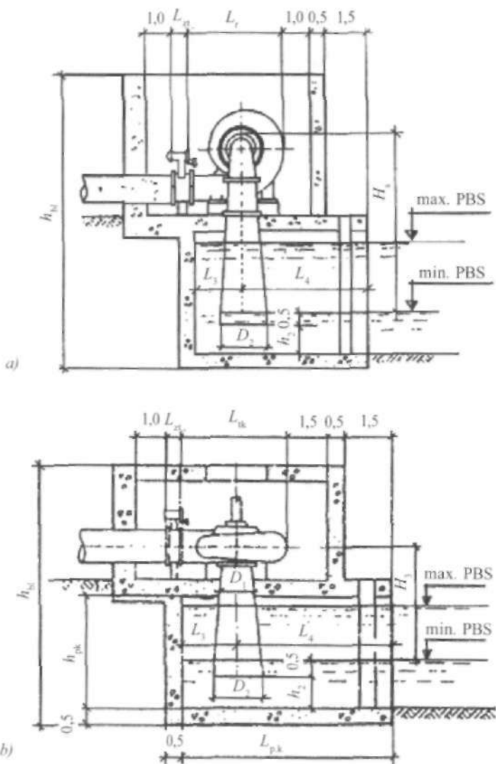
41-rasm. Gorizontial va vertikal o'rnatilgan radial-o'qiy turbinalar:
