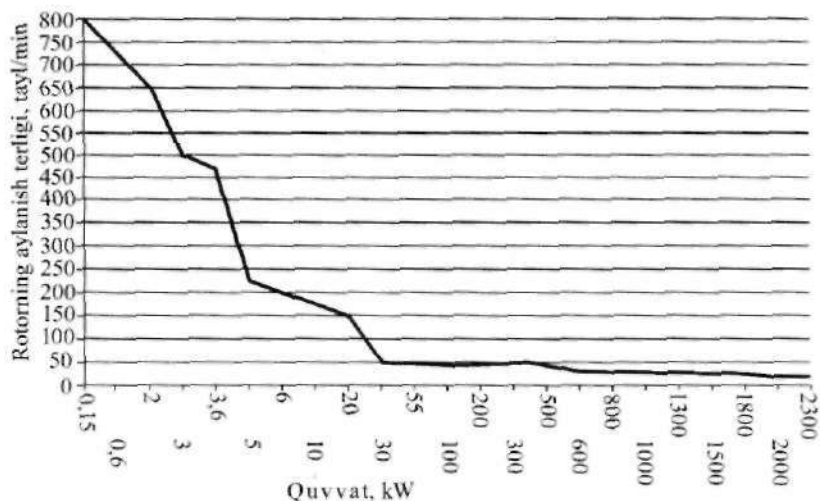
54-rasm. Shamol qurilmasi ish g'ildiragi (rotori)ning aylanish tezligi bilan uning quvvati orasidagi bog'lanish grafigi.
