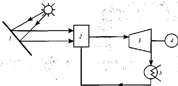
65-rasm. Quyosh energiyasini elektr energiyasiga aylantirish sxemasi: 1 – geliostatlar; 2 – qozon; 3 – turbina; 4 – generator; 5 – kondensator (bug'ni suvga aylantiruvchi qurilma).
