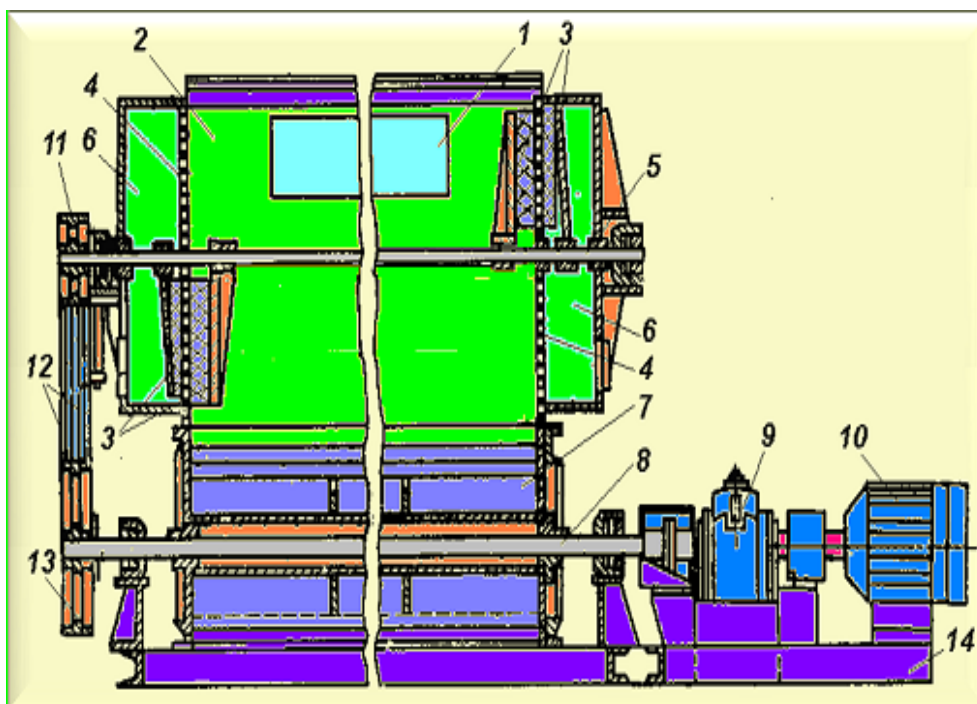
22-rasm. CC-15A separatorning bo'ylama kesim ko'rinishi
