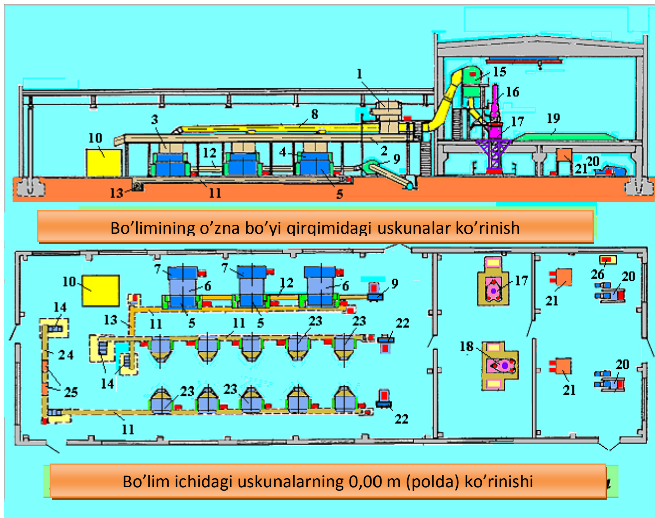
4-rasm . Bir qatorli arrali jinlar o'rnatilgan bosh binoda asosiy texnologik uskunalarning joylashish sxemasi
