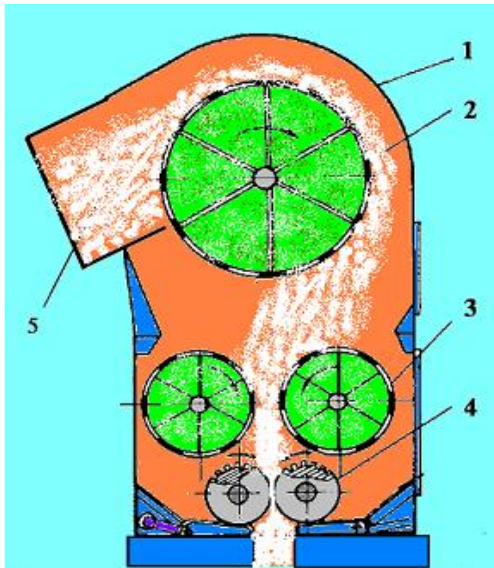
73-rasm. 5KB kondensorning texnologik jarayon sxemasi 1-korpus; 2-katta to'rli baraban; 3-to'rli kichik baraban; 4-qirrali valiklar; 5-tozalangan tola kiradigan quvur.
