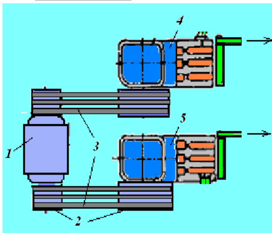
85 -rasm. ΓA-347 va ΓA-364 gidravlik nasoslarni elektr motoriga ulash sxemasi
