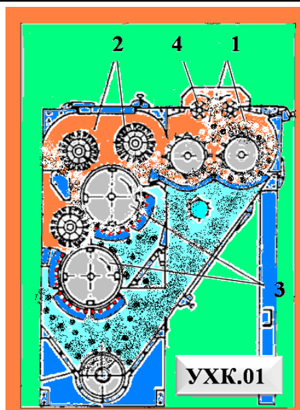
43-rasm. YXK agregti YXK.01 va. YXK.03 seksiyasilarining ko'ndalang qirqim ko'rinishi
