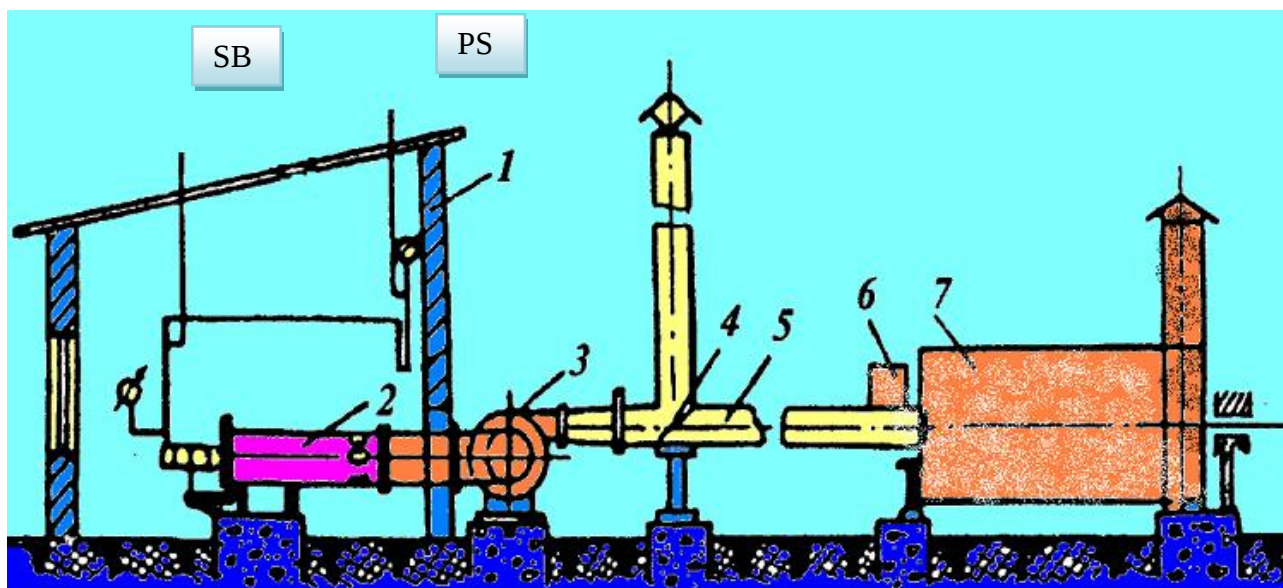
26-rasm. TG-1,5 issiqlik generatori bilan ta'minlangan chigitli paxtani quritish jarayoni sxemasi.
