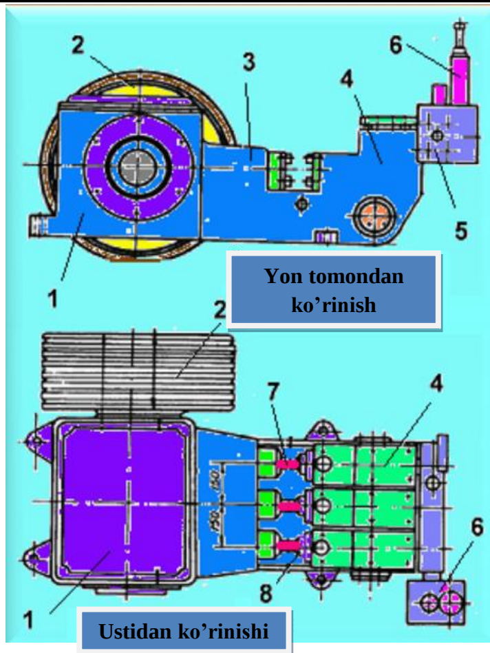
84-rasm. Uchta plunjerli ΓA-347 va ΓA- 364 gidravlik nasoslar
