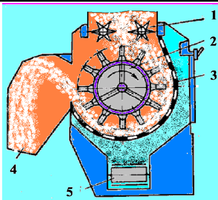
44-rasm. ПД - ta'minlagichning ko'ndalang qirgim sxemasi
