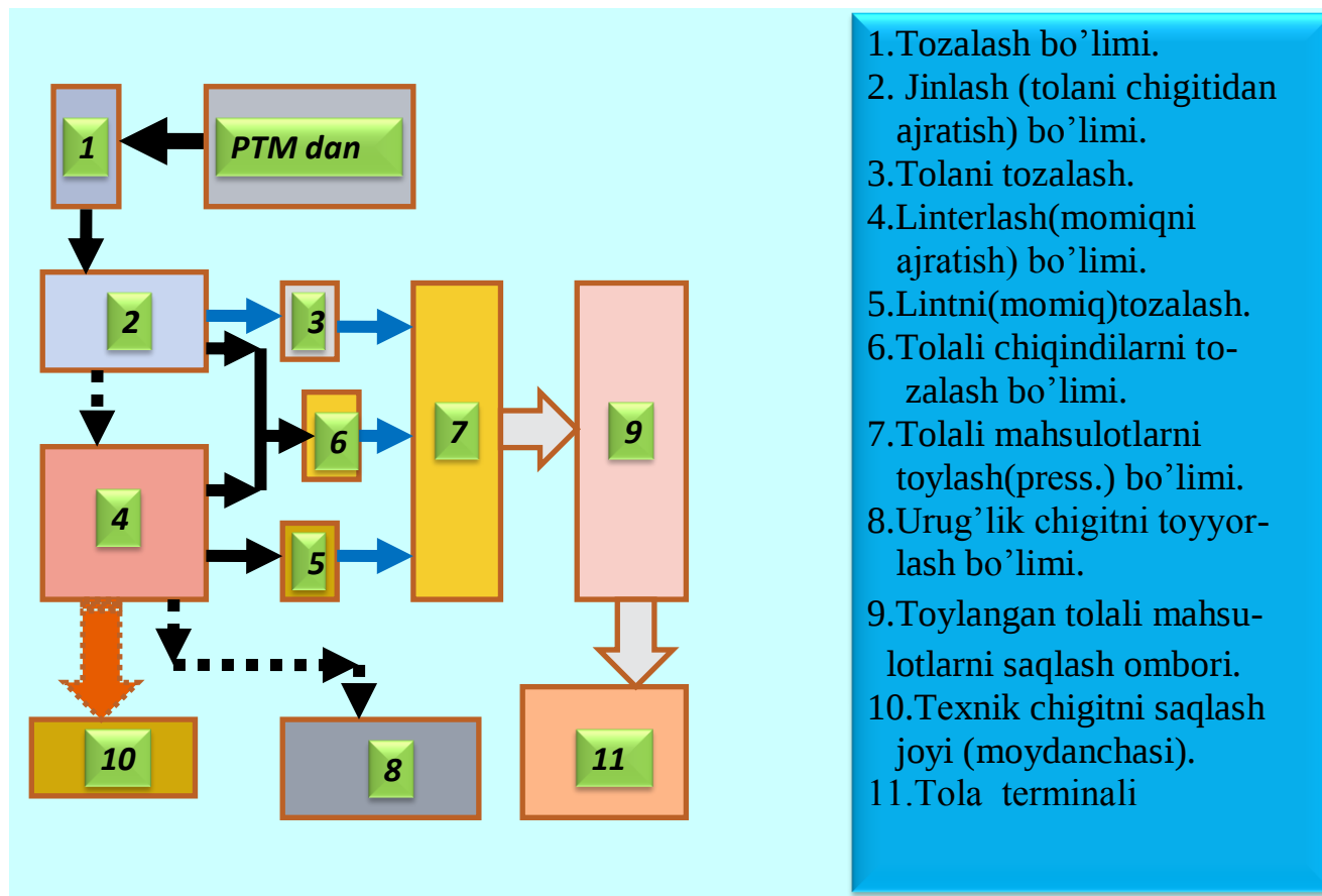
11-rasm. Paxta tozalash korxonasining umumiy texnologik jarayon
