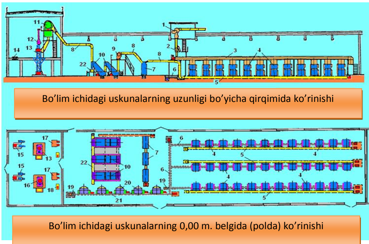
5-rasm. Paxta tozalash korxonasining bosh binosida 4 qatorda 10 tadan valikli jin o'rnatilgan texnologik jarayon sxemasi.
