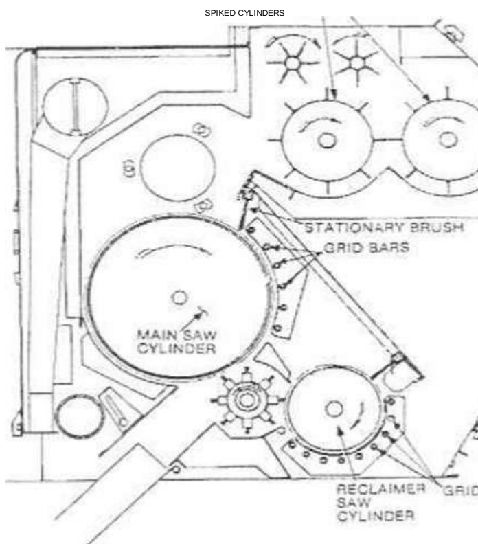
53-расм. Жин таъминлагичи
