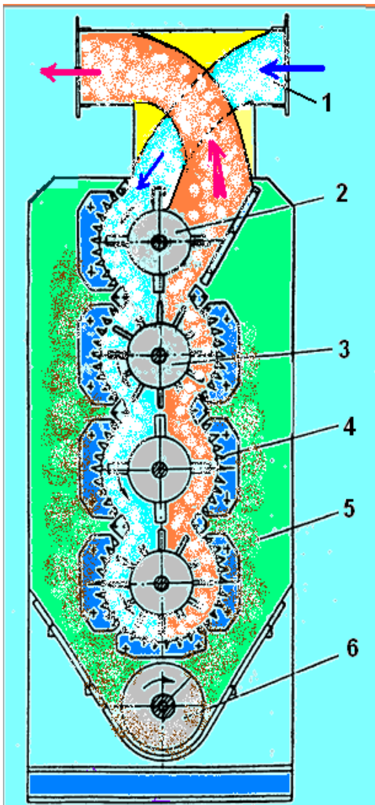
76-rasm. BTM rusumli tola tozalagich ko'ndalang qirqimi 1- tola kirish quvuri; 2- pichoqli barabanlar; 3- qoziqli barabanlar; 4-kolocnikli panjara; 5- ifloslik kamerasi; 6- ifloslik shnegi.
