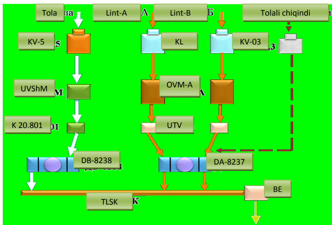
82-rasm. Presslash sexining texnologik jarayon sxemasi
