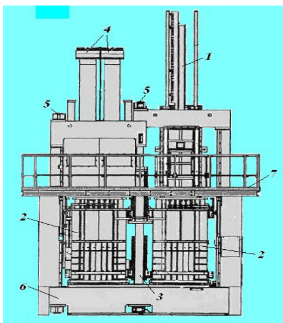
86-rasm. To'liq avtomatlashtirilgan toylovchi pastki eshikli press uskunasi. (Firma: M / s Bajaj Steyel Industriyes Ltd)
