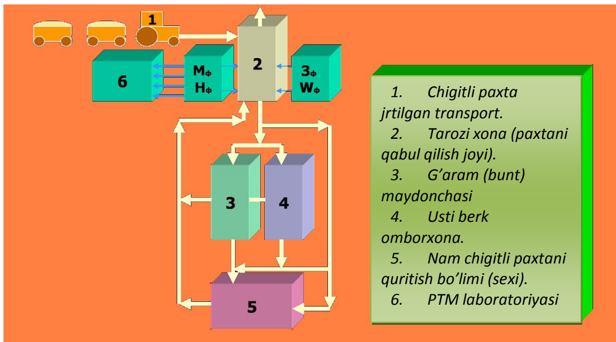
10-rasm. Namunaviy (tipovoy) paxta tayyorlash punktining umumiy texnologik jarayon sxemasi
