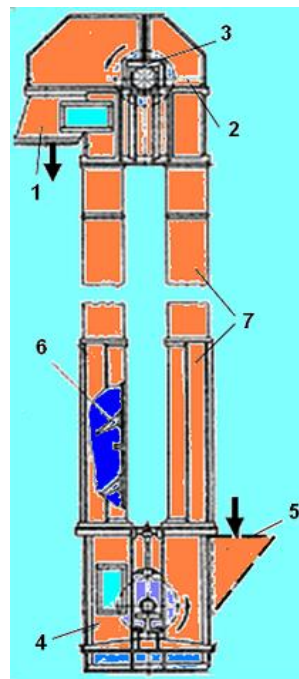
21-rasm. EC-15 rusumli chigit elevatori. 1.Chigit chiqadigan nov; 2- boshlang'ich qismi; 3- Yetaklovchi baraban; 4- boshmoq; 5 - cho'mich; 6- quvur;
