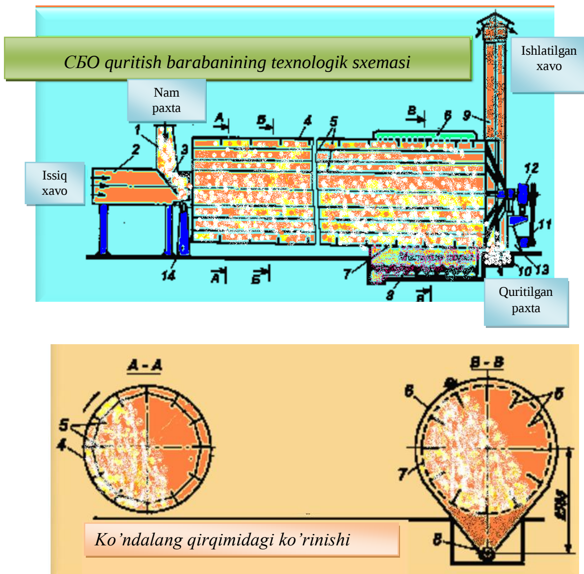
28- rasm. CBO markali barabanli quritgich sxemasi.
