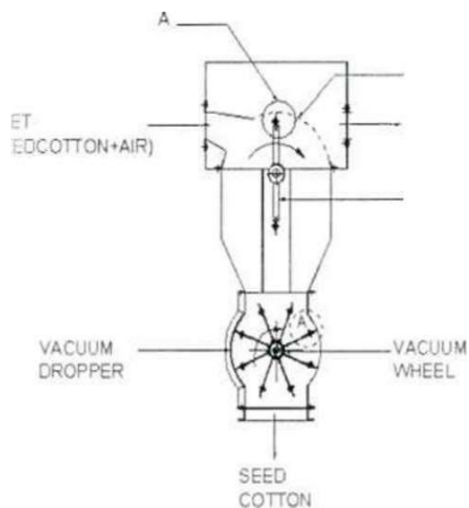
24-rasm. Havo separatori va vakuum klapaning ko'ndalang qirqim sxemasi
