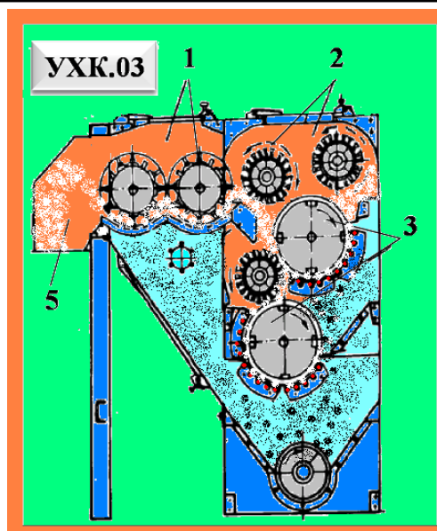
43-rasm. YXK agregti YXK.01 va. YXK.03 seksiyasilarining ko'ndalang qirqim ko'rinishi
