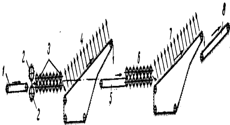
91-Rasm. Kalta tola ajratadigan KIIK-2 mashinasi
