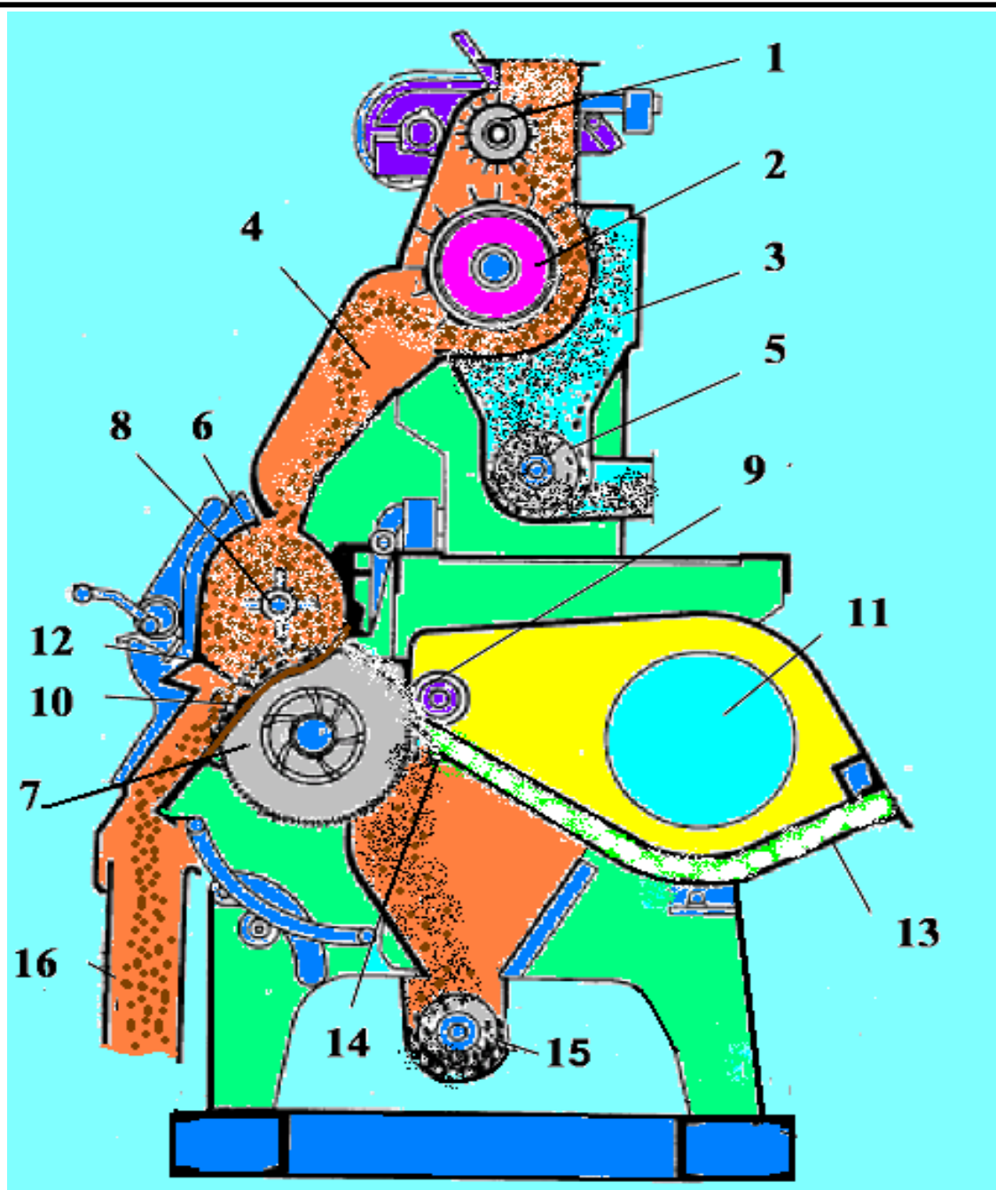
71-rasm.5/III - rusumli linterning texnologik jarayon sxemasi
