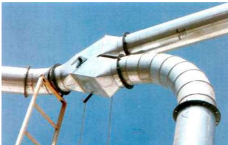
9-rasm. CHigʻanoqlari maxsus figurali havo yuradigan va soʻradigan quvurlar oqimi
