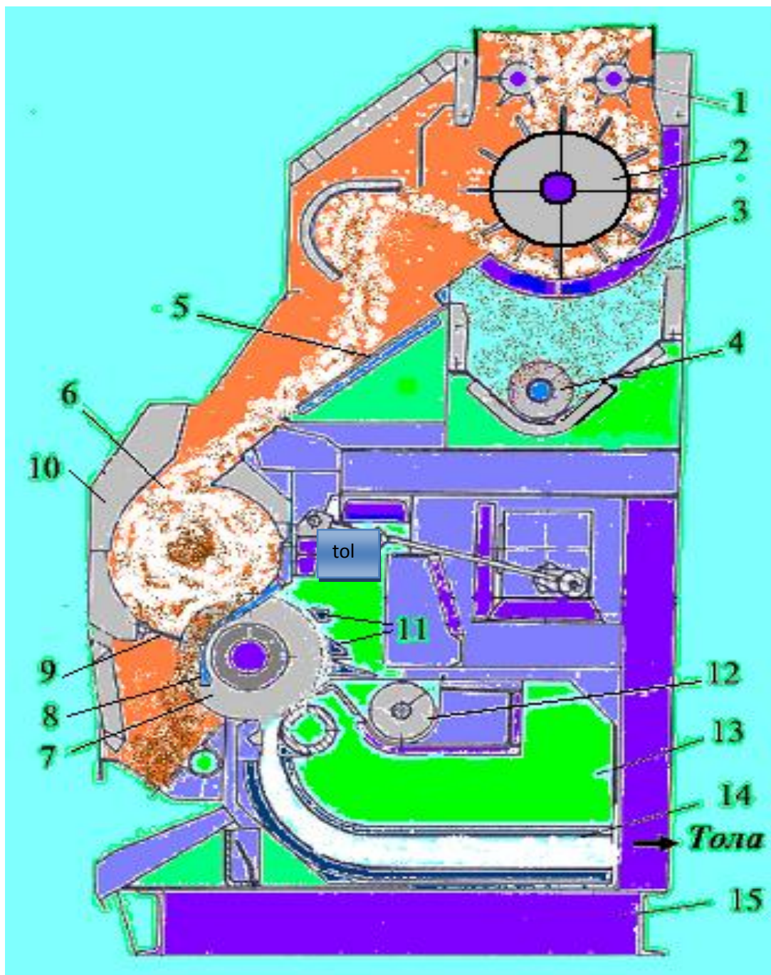
49 - rasm. 5ДП-130 arrali jinning ta'minlagichi bilan ko'ndalang qirqimi sxemasi
