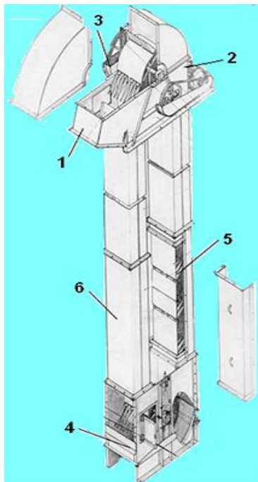
20-rasm. EC-14 rusumli chigit elevatori. 1.Chigit chiqadigan nov; 2- boshlang'ich qismi; 3- Yetaklovchi baraban; 4- boshmoq; 5. Chigit uzatish novi; 6- cho'mich; 7- quvur;
