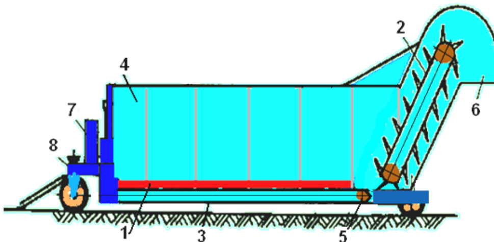
18-rasm. XIII qabul qilish - uzatish qurilmasining sxemasi
