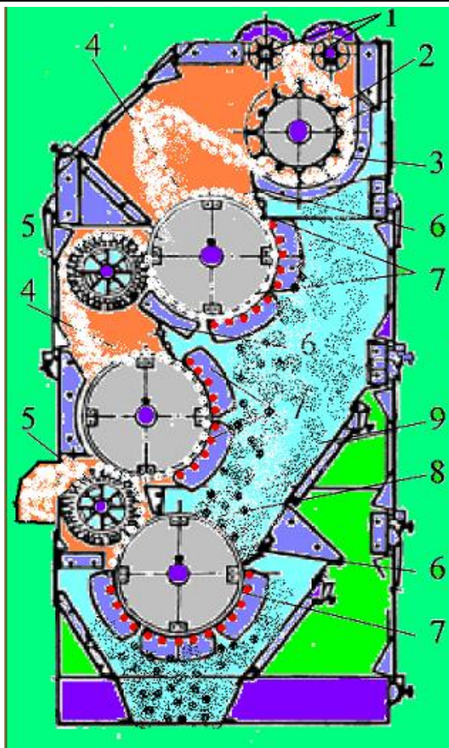
Rasm 42. 4X-3M2 rusumli paxtani yirik iflosliklardan tozalagichning ko'ndalang qirqimi va umumiy ko'rinishi
