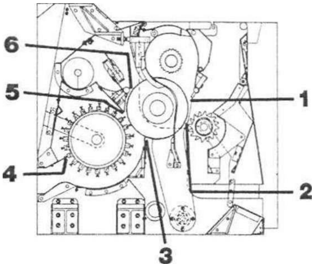
57-rasm. Arrali jinning nastroykasi.
