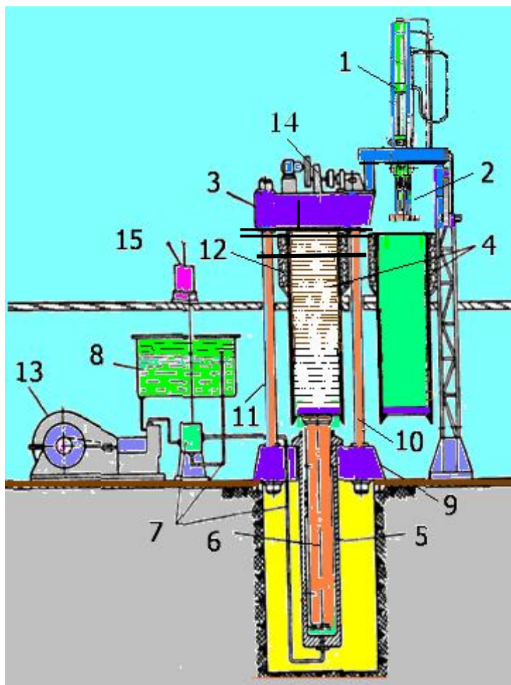
79-rasm. K20.801 gidravlik shibbalagichning umumiy ko'rinishi.
