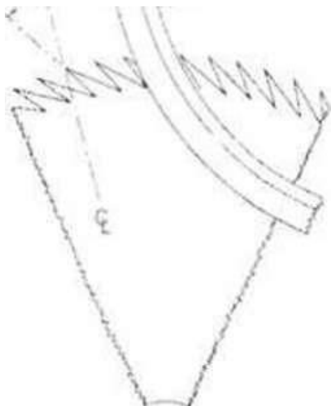
55-rasm. Arrali disk bilan qobirg'ani o'zaro joylashish sxemasi
