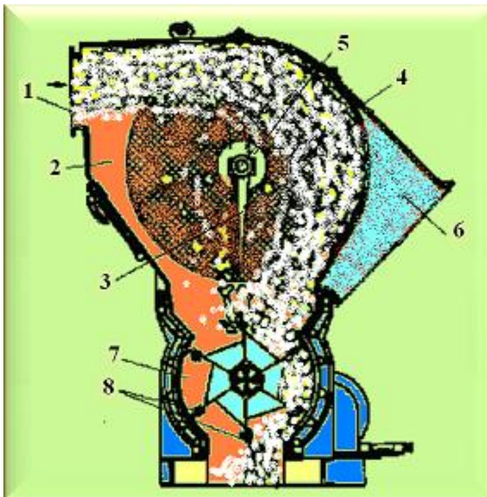
23-rasm. CC-15A separatorining ko'ndalang kesim ko'rinishi
