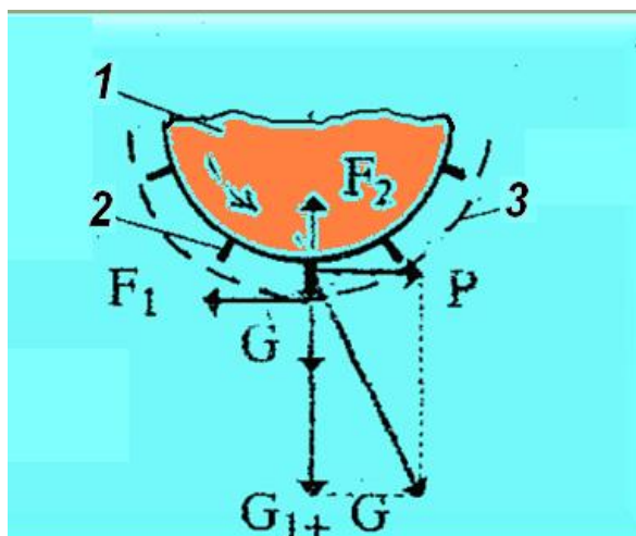
31-rasm. Baraban qozig'ning paxta bo'lakchasiga ta'sir qilish sxemasi
