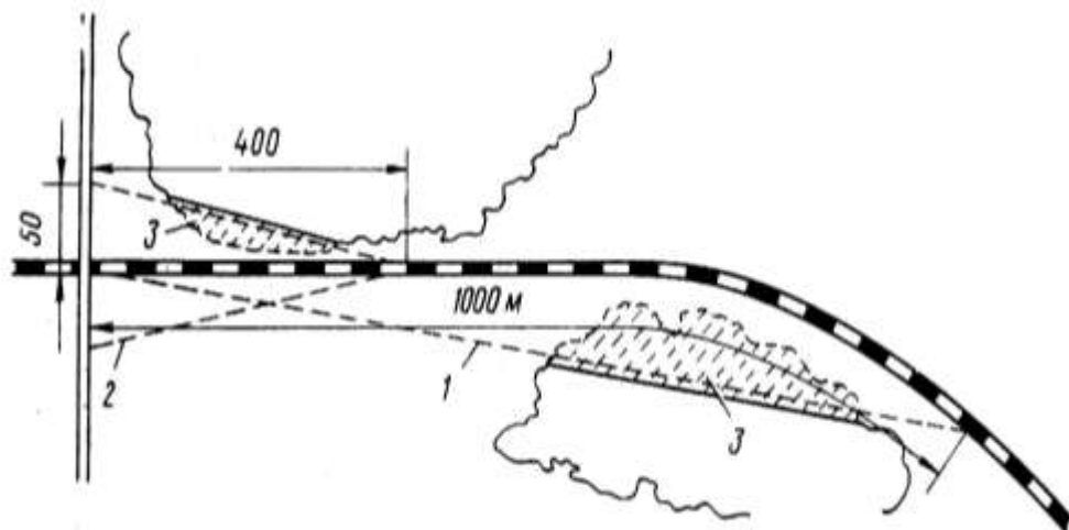
37-rasm. Yo'llarning temir yo'llar bilan kesishuvi.
