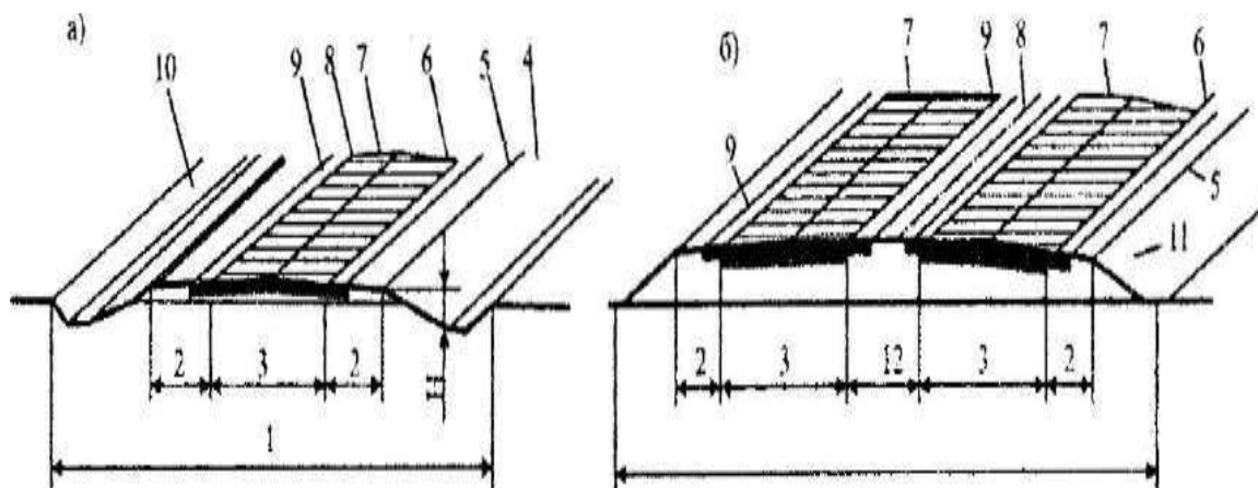
6-rasm. Yo'l ko'ndalang profilining elementlari
