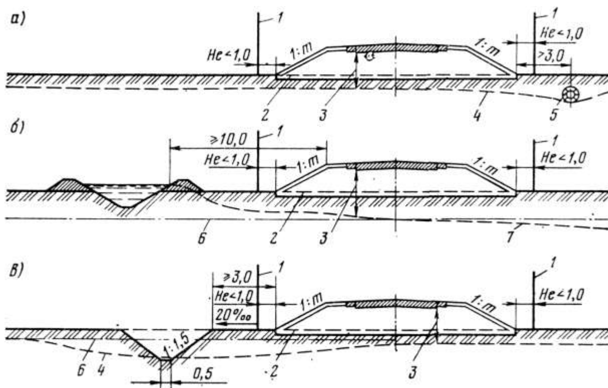
40-rasm. Sun'iy sug'orish xududlarida yo'llarning ko'ndalang kesimlari. a-yopiq zovurlar va kollektorlar bo'ylab; b-magistral ariqlar bo'ylab; v-ochiq kollektorlar bo'ylab; 1-ajratilgan joy chegarasi; 2-o'simlik gruntining olib tashlanadigan qatlami; 3-yo'l to'shamasi pastining hisobiy ko'tarilishi; 4-sizot suvlarining zovurlar yoki ariqlar bilan pasaytirilgan satxi; 5-quvursimon zovurlar-kollektorlar; 6-sug'orish tizimi qurilganiga qadar sizot suvlarining eng baland satxi; 7-sizot suvlarining eng ko'p sizadigan satxi
