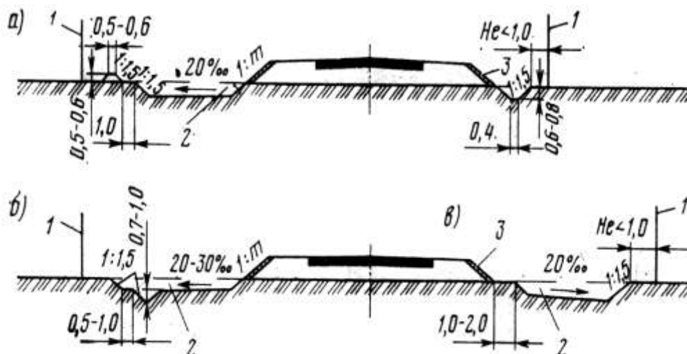
a-bir tomonida rezerv joylashgan ko'tarma; b-rezervli va bo'ylama novli ko'tarma; v-bermali va chuqurrezervli ko'tarma; 1-ajratilgan joy polosasi; 2-rezerv; 3-yo'l poyining yon tomonini mustahkamlash
