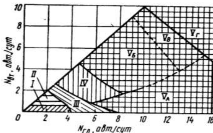
29-rasm. Turli sathlardagi kesishishlar. N_{gl} , N_m - asosiy va ikkinchi toifali yo'llarda harakat jadalligi; I-oddiy jixozlanmagan kesishishlar; II-ikkinchi darajali yo'lda yo'naltiruvchi orolchalari bo'lgan qisman kanallashtirilgan kesishishlar; III - asosiy va ikkinchi toifali yo'llarda yo'naltiruvchi orolchalari bo'lgan va asosiy yo'lda o'tish-tezkor polosalari bo'lgan kanallashtirilgan kesishishlar; IV - xalkasimon kesishishlar; V_A - eng tig'iz yo'nalish bo'yicha eng yaxshi harakat sharoitlarini ta'minlovchi xalkasimon kesishishlar; V_B - xalkasimon kesishishlar bosqichli qurilishning birinchi bosqichi sifatida, keyin esa ular turli satxlarda loyihalalanib, qayta quriladi; V_r - turli satxlardagi kesishishlar.
