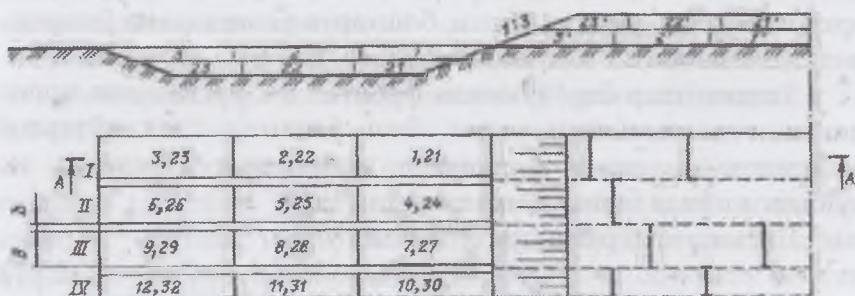
2.45-расм. Ён резервдан грунт олиб кўтарма қуриш
