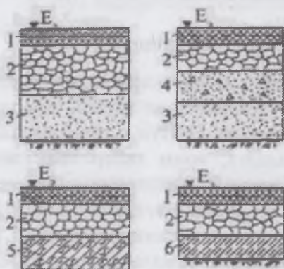
3.1-расм. Эквивалент модуллари E_z=60-70 МПа ли юқори тоифали нобикир йўл тўшамаларининг тузилиши: 1- икки қатламли асфальт-бетон; 2- сараланган чақилган тош; 3- қум; 4- шлак; 5- боғловчилар билан ишлов берилган грунт; 6- кам миқдорда боғловчилар билан ишлов берилган грунт.
