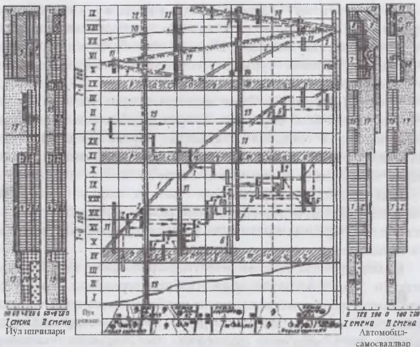
4.11-расм. Йўл қурилиши календарь графиги (2- вариант)
