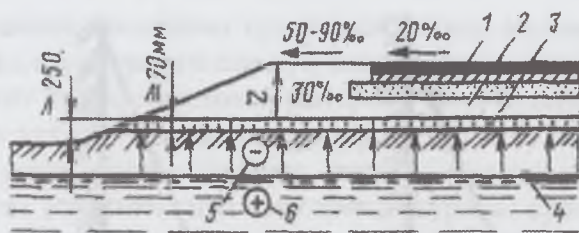
2.28-расм. Капилляр тўсувчи қатламчалар: 1-йўл тўшамаси; 2-йўл пойи грунги; 3-капилляр тўсувчи қатламча; 4-грунт сувлари сатҳи; 5-капилляр сувларининг худуди; 6-эркин сув худуди; Z-катламчанинг ётиш чуқурлиги.
