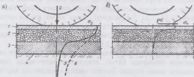
3.3-расм. Кўп қатламли йўл тўшамасида автомобилларнинг гидиракларидан ҳосил бўладиган кучланиш: а - вертикал кучланишлар \sigma_z эпюраси; б - горизонтал кучланишлар \sigma_x эпюраси; 1- қоплама; 2-асос; 3-асоснинг қўшимча қатлами; 4-тўшама грунт; 5-йўл тўшамасидаги кучланиш эпюра чизиги; 6-бир жинсли грунтдаги кучланиш эпюра чизиги.
