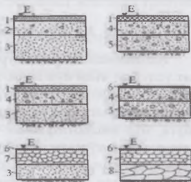
3.2-расм. Эквивалент модуллари E_z=50-35 МПа ли қуйи тоифали нобикир йўл тўшамаларининг тузилиши: 1-бир қатламли асфальтбетон; 2-қуйинди; 3-қум; 4- чақик тош; 5-шағал; 6-устки ишлов қатлами; 7-сараланган чақик тош; 8- кам мустаҳкамликка эга бўлган тош материали.
