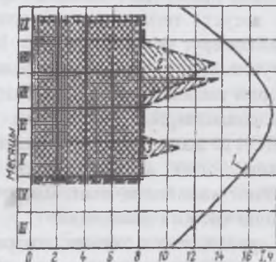
4.12-расм. Хусусий потокларнинг сутка давомидаги иши давомийлиги графиги: 1- ёруғ кун давомийлиги; 2-цементбетон коплamani қуриш бўйича смена давомийлиги; 3 цементгрунт асосни қуриш бўйича смена давомийлиги.
