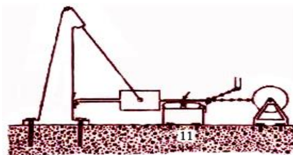
46-rasm. Golitsin seysmogrofi
