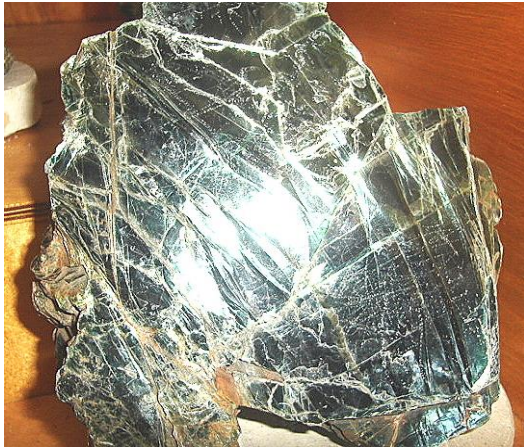
7-rasm. Xlorit (Ural)
