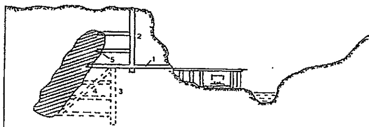
6.1-rasm. Konni shtolnya bilan ochib, tik ko'r stvolga o'tish sxemasi.
