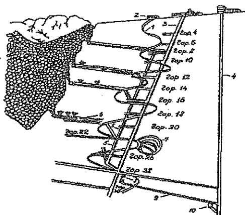
6.11-rasm. «Kreyton» rudnigini ochish sxemasi (Kanada)
