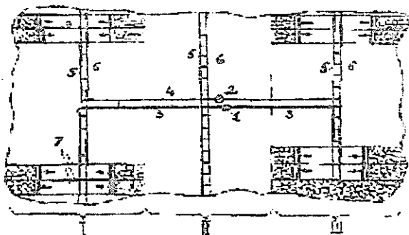
7.12-rasm. Gorizontal joylashgan ruda tanasini panel usulda tayyorlash.
