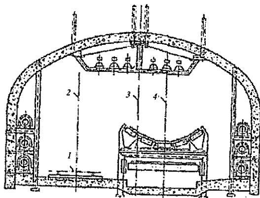
6.18-rasm. Qiya stvol ko'ndalang kesimi yuzasi rudani relsli yo'l va konveyerda chiqarish usuli: 1 – relsli yo'l kallagi balandligi, 2, 3, 4 – konveyer va relsli yo'llar joylashish o'qi.
