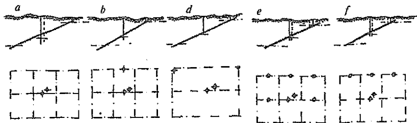
6.16-rasm. Shaxta maydoni chegarasida bosh va yordamchi stvollarni joylashtirish
