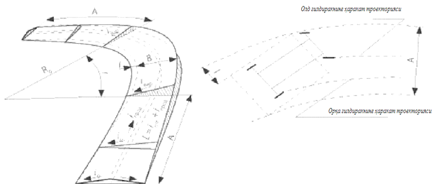
5.2-rasm. Viraj sxemasi: A – o'tuvchi egri chiziqli virajni olib qochish joyi; V—qatnov qismining kengligi; io—ikkitarafлама nishablikli kesimning bo'ylama nishabligi; ivir—virajning ko'ndalang nishabligi; iomg—virajni olib qochish joyidagi bo'ylama nishablik; iprod—virajdagi bo'ylama nishablik; l—kengaytirish; r—aylanma egri chiziq; R0 – dumaloqlash radiusi.
