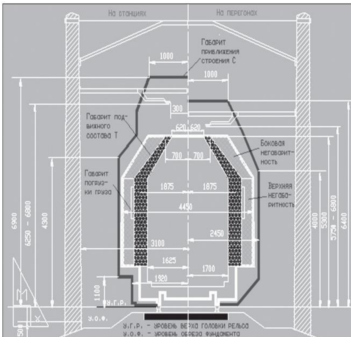
2.15-rasm. Asosiy o‘lcham o‘lchovlari.
