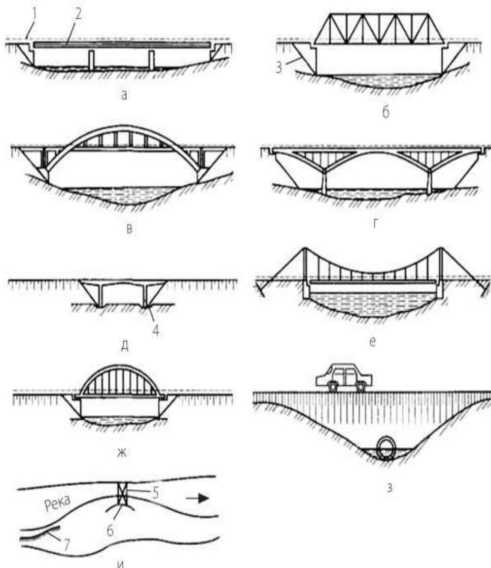
5.15-rasm. AVTOMOBIL yo'llaridagi sun'iy inshootlar: a-yuqoridan harakatladigan to'sinli ko'priq; b-ikki tomonda fermali ko'priq (harakat pastda); v-arkali ko'priq; g-arka-konsolli ko'priq; d-romli ko'priq; ye-osma ko'priq; j-aralash tizimli ko'priq (qattiq to'sinli yaxlit arka); z-suv o'tkazuvchi quvur; i-ko'priqka o'tish sxemasi; 1-to'shama (ko'priqka kirish); 2-oraliq qurilma; 3-tirgak; 4-tayanch; 5-ko'priq; 6-suv oqimini yo'naltiruvchi to'g'on; 7-doimiylik inshootlari.
