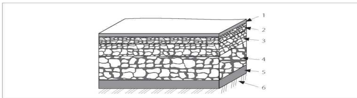
5.11-rasm. Yo'l to'shamasi: 1-yedirilish qatlami; 2-qoplamaning yuqori qatlami; 3-qoplamaning pastki qatlami; 4-asosi; 5-qo'shimcha qatlam; 6-to'shalgan tuproq.
