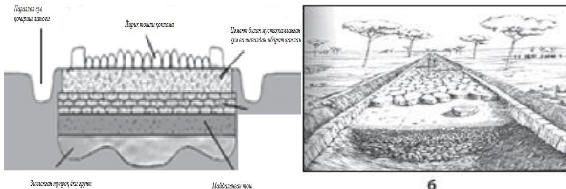
1.3.1-rasm. “Appii yo‘li”ning ko‘ndalang kesimi.
