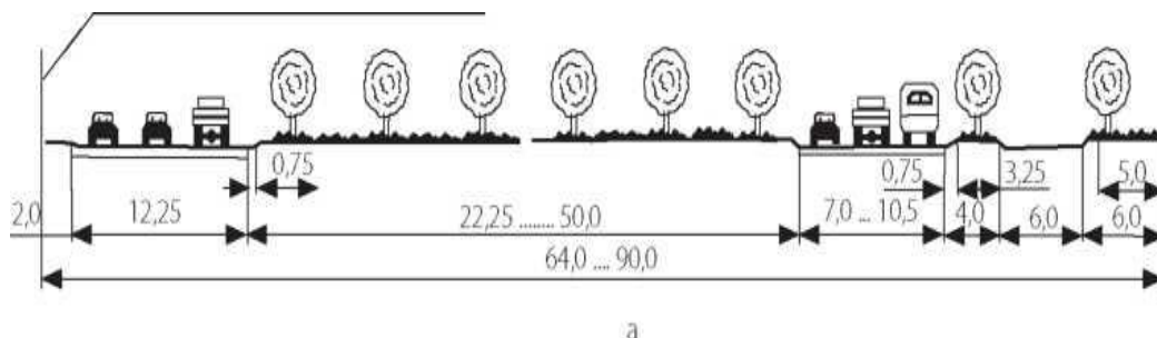
5.7-rasm. Shahar tezyurar yoʻlining koʻndalang kesimi (oʻlchamlar metrda berilgan).
