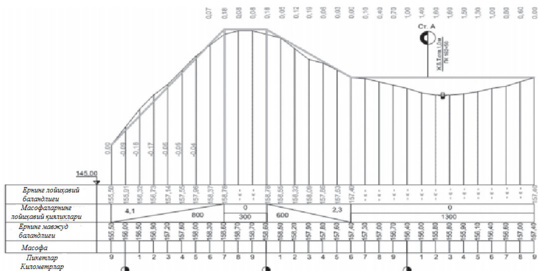
2.9-rasm. Bo‘ylama kesim
