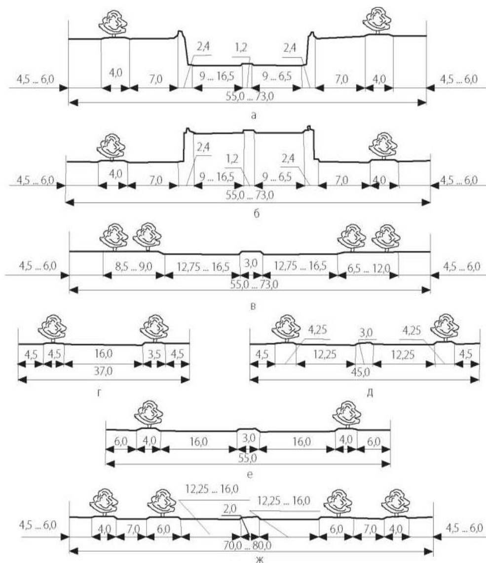
5.8-rasm. Uzluksiz harakat bilan (a-v) va turli o'lchamdagi harakat bilan (g-j) umumshahar ahamiyatidagi magistral ko'chaning ko'ndalang kesimlari (o'lchamlar metrda berilgan):
