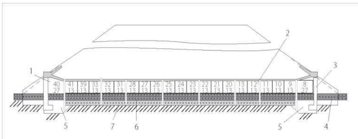
5.14-rasm. Suv o'tkazuvchi quvur. 1-quvurning konus shaklidagi qismi; 2- bo'laklar; 3-truba boshining portalli bloki; 4-monolit betonli nov; 5-qum-shag'alli tayyorgarlik; 6-choqiqtoshli tayyorgarlik; 7-poydevor bloki.
