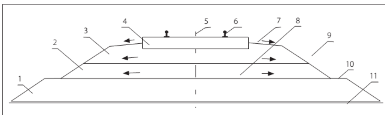
2.14-rasm. Temir yo‘l konstruksiyasining sxemasi: 1–yo‘l poyi (asosiy maydoni); 2–yostiqcha (ballast prizmasining pastki qismi); 3–chaqiqtoqli ballast prizma; 4–temir yo‘l ostiga o‘rnatiladigan temir-beton yoki yog‘och shpala; 5–temir yo‘lning o‘qi; 6–rels; 7–rels–shpalali katakning mustahkamligini ta‘minlash uchun ballast prizmaning yelkasi; 8–to‘kish prizmasining yuzasi; 9–qurilgan yonbag‘ir; 10–yo‘l cheti; 11–yo‘l poyining etagi-asosi.
