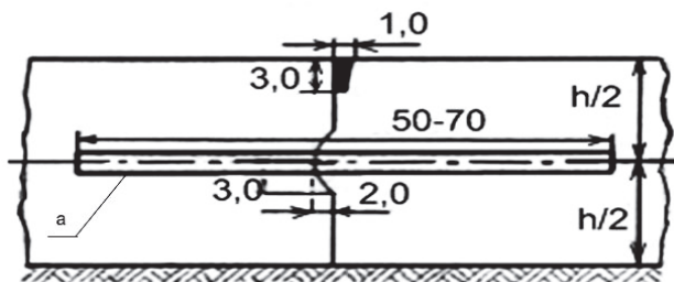
4.17-расм. Ишчи чокнинг тузлиши: а — штир-анкер.
