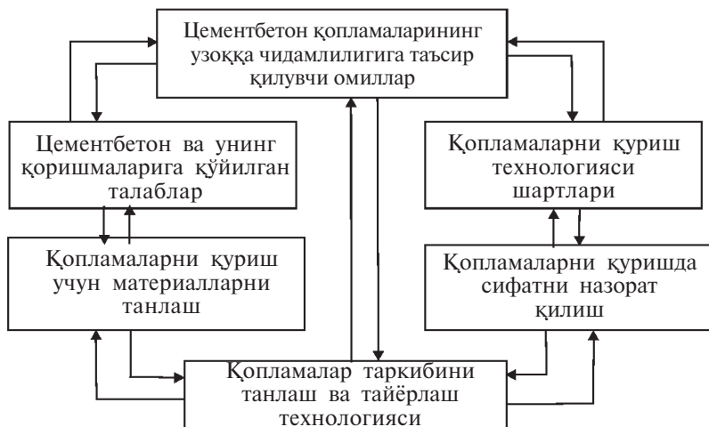
1.1-расм. Цементбетон қопламаларнинг узоққа чидамлигига таъсир қилувчи омилларнинг ўзаро боғлиқлиги (стрелкалар билан ўзаро таъсир кўрсатилган).
