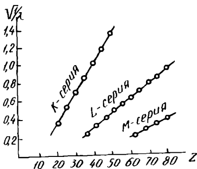
III.2-расм. Элементларнинг тартиб рақами билан уларнинг рентген спектрларидаги характерли чизиқ тақрорлиги орасидаги боғланиш.
