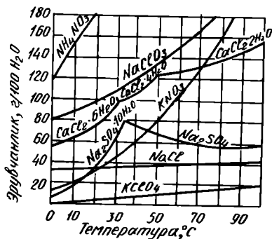
VIII.3-рasm. Турли моддалар эрувчанлигининг температурага боғлиқлиги.
