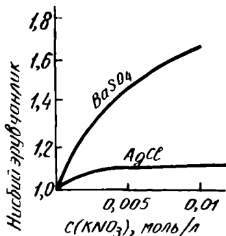
IX.2-расм. Сувда ёмон эрийдиган тузлар эрувчанлигининг бегон туз концентрацияси ортиб бориши билан нисбий ўзгариши
