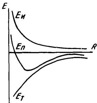
V.1-расм. Икки атомдан иборат ионли молекуладаги тортишиш ( E_t ), итаришиш ( E_n ) ва молекуланинг потенциал энергиялари ( E_m ) нинг атомлараро масофага қараб ўзгариши.
