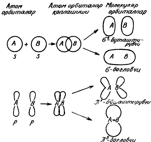
V.11-расм. s - ва p -орбиталлар иштирокида боғловчи ( \sigma , \pi ) ва бўлаштирувчи ( \sigma^* , \pi^* ) молекуляр орбиталларнинг ҳосил бўлиши.
