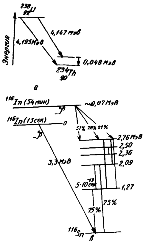
IV.4-расм. β-емирилишдан кейин ҳосил бўладиган γ-нурланиш схемаси: α— ^{238}_{92}\text{U} нинг
