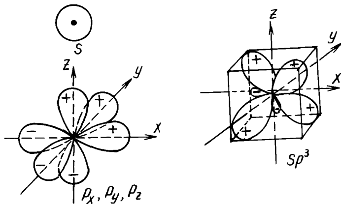
В.4-расм. Битта s - ва учта p -орбиталлардан тўртта sp^3 -гибрид орбиталларининг ҳосил бўлиши.
