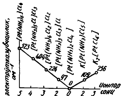
ХI.2-расм. Вернер-Миолати қаторига тегишли моддалар электр ўтказувчанлигининг ўзгариши.
