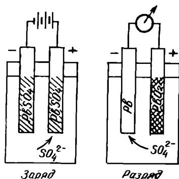
Х.5-расм. Қўрғошин аккумуляторининг зарядлашга ва разрядлашга тайёр ҳолатлари
