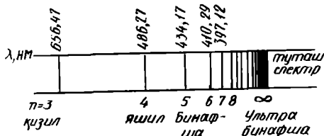
III.3-рasm. Водород атоми электромагнит тўлқинларининг кўзга кўринадиган соҳаси (Бальмер серияси)даги спектрал чизиклар.
