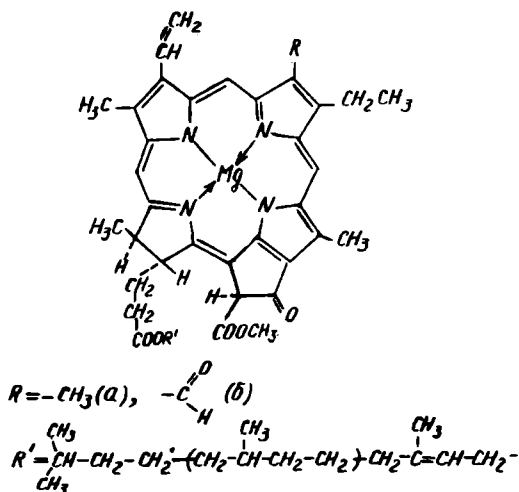
XI.16-расм. Хлорофилл — a ва хлорофилл — b ларнинг тузилиш формулалари.
