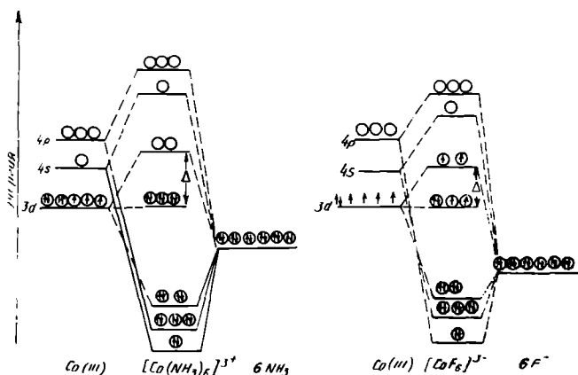
XI.9-расм. Паст спинли (кучли майдон ҳолати) [\text{Co}(\text{NH}_3)_6]^{3+} ва юқори спинли (кучсиз майдон ҳолати) [\text{CoF}_6]^{3-} координацион бирикмаларда молекуляр орбиталарининг энергетик диаграммаси.
