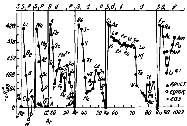
VII.1-рasm. Элементлар хлоридларининг ҳосил бўлиш стандарт иссиқликлари ва элементлар тартиб рақамлари орасидаги боғланиш диаграммаси.
