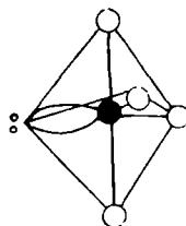
V.25-расм. \text{AX}_5\text{E} типдаги молекуланинг геометрияси.
