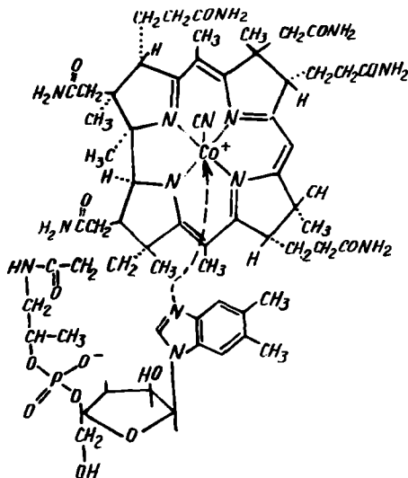
XI.15-расм. Витамин B_{12} (цианкобаламин) молекуласининг тузилиши.
