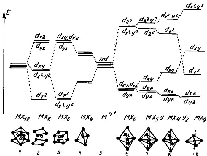
ХI.6-расм. Металл ионларидаги d -орбиталларнинг турли симметрияли майдон таъсирида энергиясининг тақсимланиши: a —икосаэдр, b —антипризма, c —куб, d —тетраэдр, e —сферик симметрия, ж, з —октаэдр, и —октаэдр (транс-изомер учун), к —текис квадрат.
