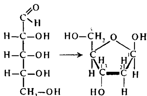
D-2-dezoksiriboza
