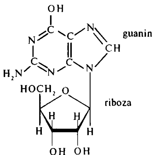
guanozin
