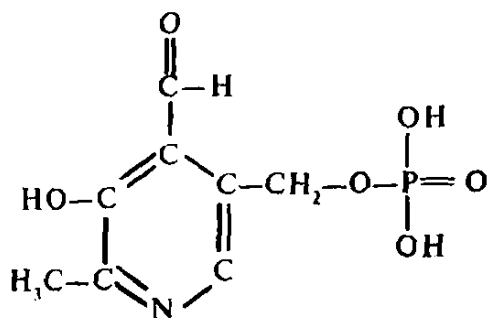
piridoksalfosfat
