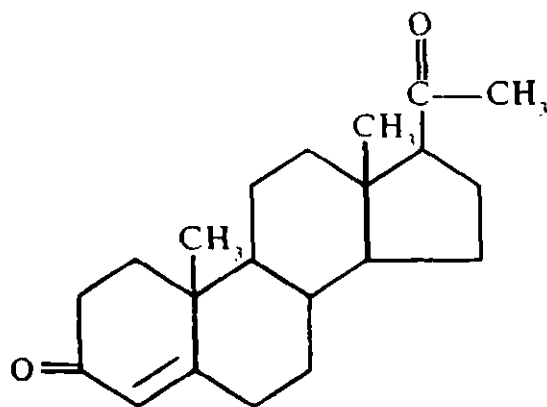
progesteron
