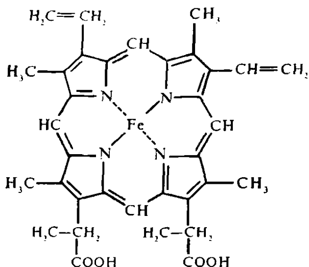
Gem
