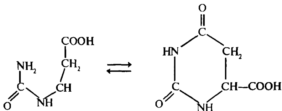
Karbomoilaspartat kislota
