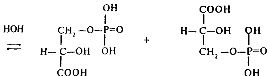
3-fosfoglitserat kislota
