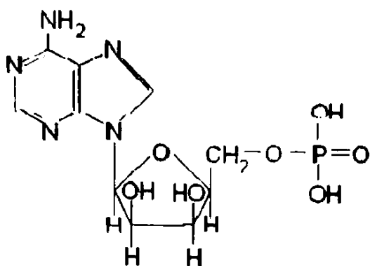
Adenilat kislota (AMF)
