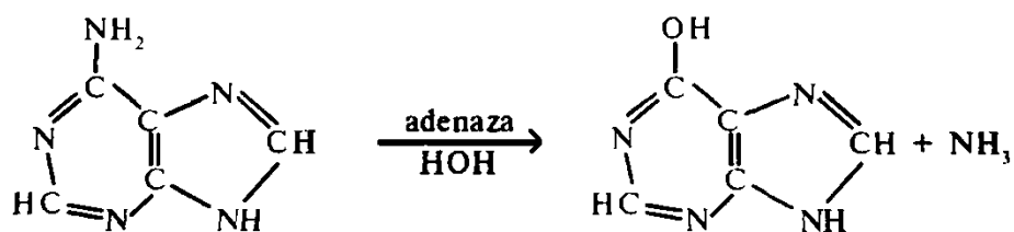
Adenin
