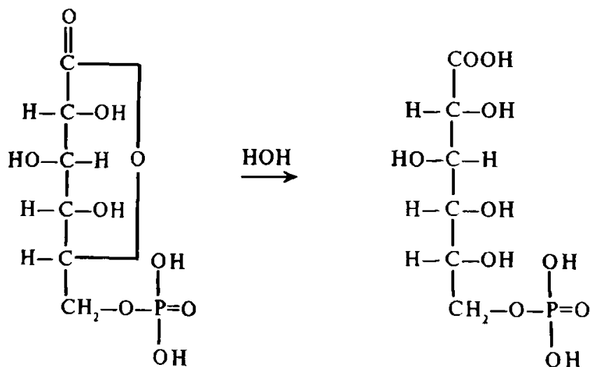
6-fosfatglukolakton
