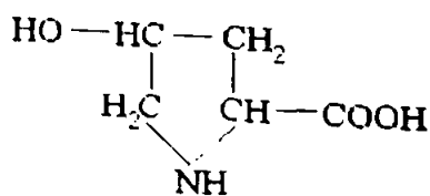
Oksiprolin
