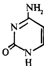
sitozin
