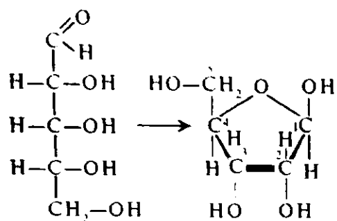
D-riboza
