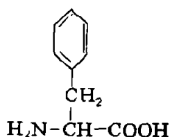
Fenilalanin
