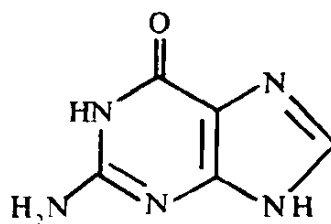
Guanin
