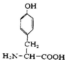
Tirozin
