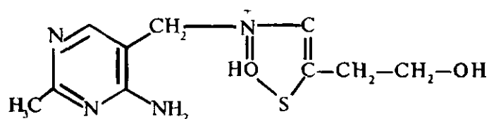
B 1 vitamini
