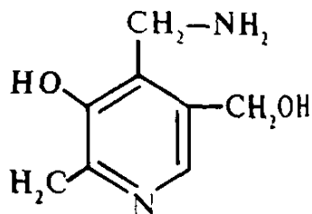
Pirididoksiamin
