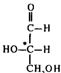
(+) glitserat-aldegid
