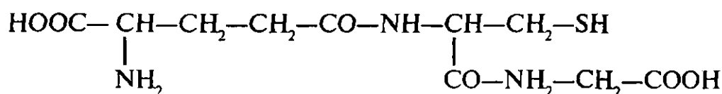
Qaytarilgan glutation
