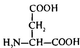
Aspartat kislota
