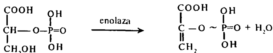
2-fosfoglitserat kislota
