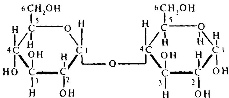
Maltoza
