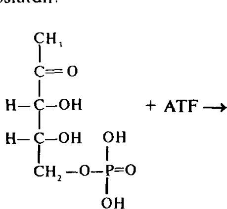
Rubuloza -5- fosfat
