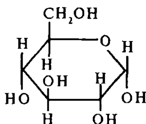
D-glukopiranoza
