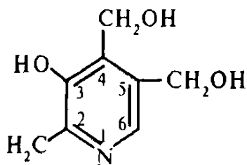
Piridoksin
