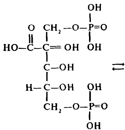
oraliq modda
