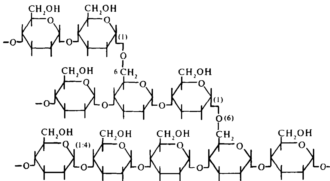
Amilopektin
