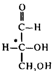
(+) glitserat-aldegid
