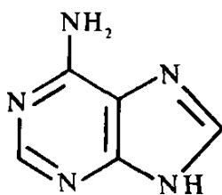
Adenin
