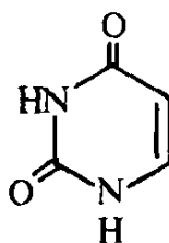
uratsin
