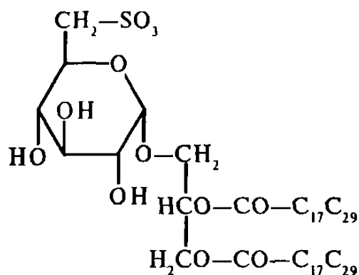
O'simlik sulfolpidi
