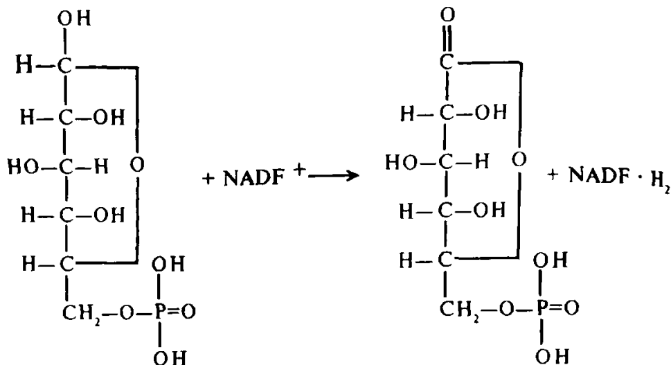
6-fosfatglukolakton kislota
