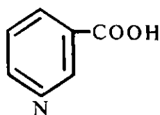
nikotinat
