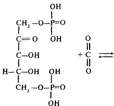
Ribuloza -1,5- difosfat
