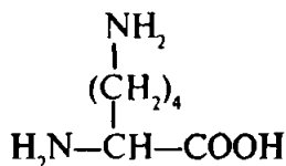
Lizin
