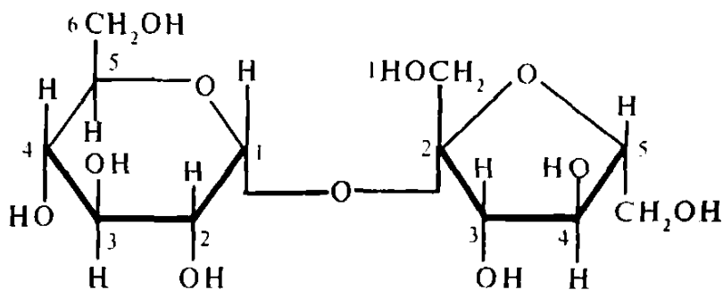
Saxaroza
