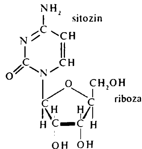
sitidin
