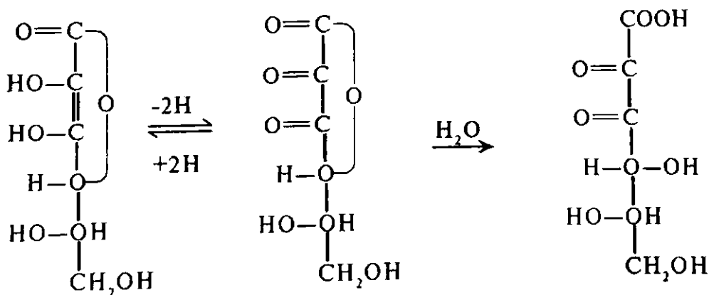
L- askorbat kislota
