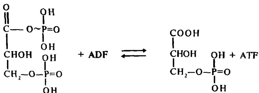
1,3-difosfoglitserat kislota
