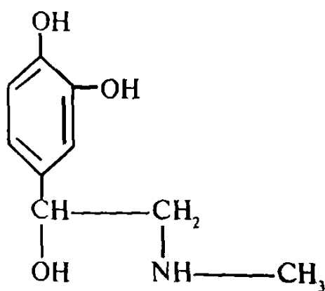
Adrenalin
