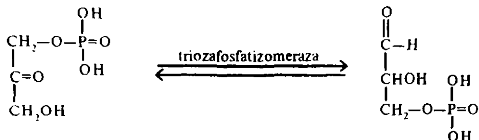
fosfodioksiatseton
