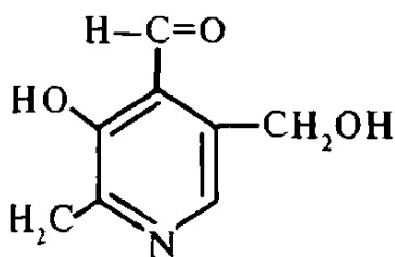
Piridoksal
