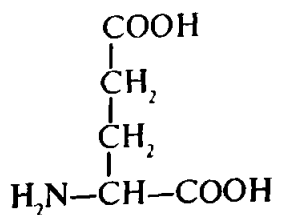
Glutamat kislota
