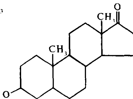
androsteron
