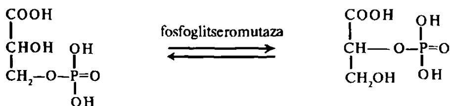
3-fosfoglitserat kislota
