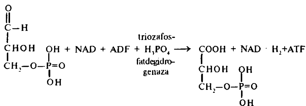
3-fosfoglitserin aldegid
