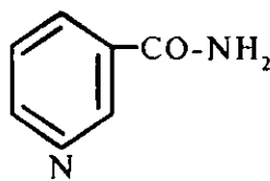
nikotinamid
