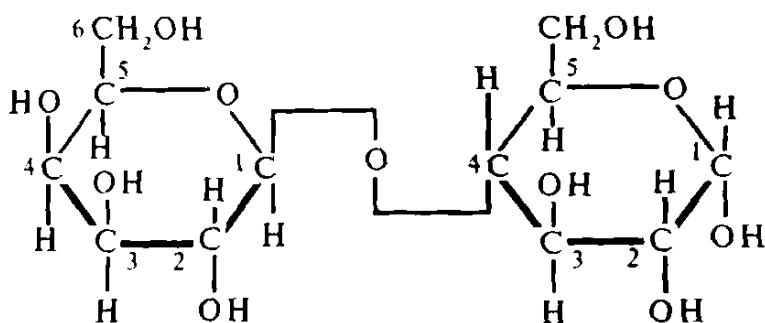
Laktoza
