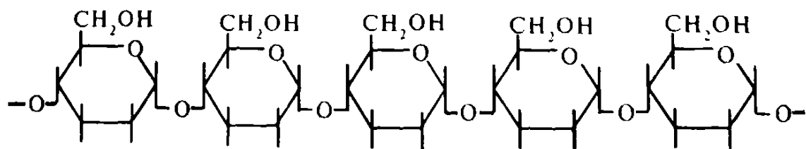
Selluloza
