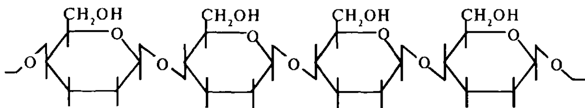
amiloza
