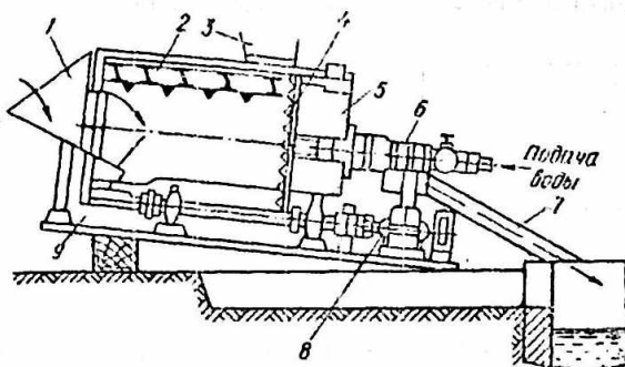
3.3-rasm. Uzlüksiz termomexaniq ohak so'ndirgich chizmasi.
