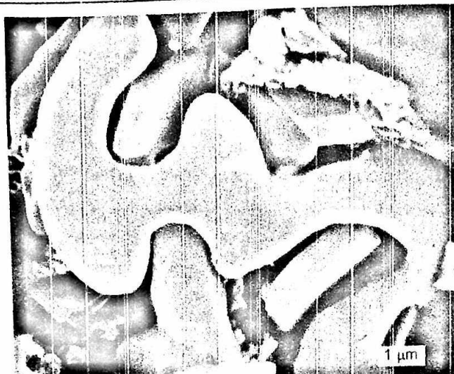
Рис. 2.20. б) Алит, покрытый оболочкой затвердевшего щелочного сульфата, 10000-кратное увеличение
