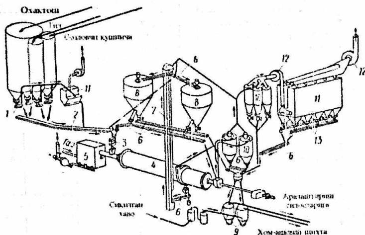
5.4-rasm. Xomashyoviy materiallarning tegirmonlarda quritish va maydalash texnologik chizmasi:
