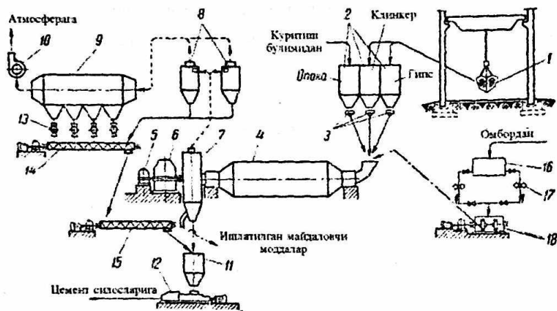
20-rasm. Ochiq sikl bo'yicha klinker maydalash uchun moslama chizmasi
