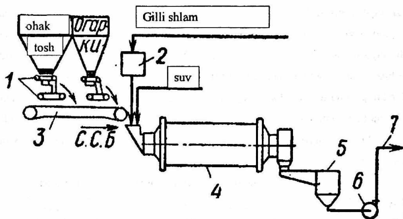
5.2-rasm. Xom ashyoviy moddalarni maydalash chizmasi.
