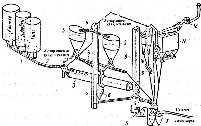
20-rasm. Klinker, gips va qo'shimchalarni maydalash texnologik chizmasi. 1-dozatorlar; 2-tasmali transporter; 3-tegirmon; 4-elevator; 5-separatorlar; 6-aerogelob; 7-kamerali nasos; 8-siqilgan havo filtri; 9-shaxta; 10-siklon; 11-yengsimon filtri; 12-ventilator.
