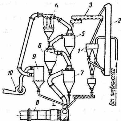
6.3-rasm. Siklonli issiqlik almashtiruvchilar tizimi.
