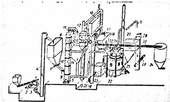
2.2-rasm. Xom ashyoni quritib gips olish sxemasi
