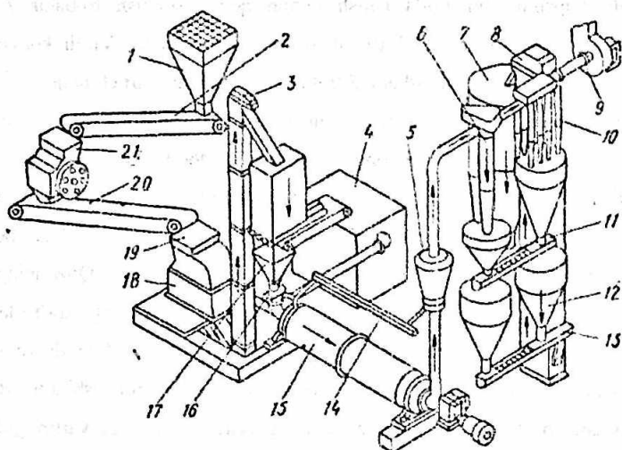
2.9-rasm. Qurilish gipsini maydalash va kuydirish jamlangan chizma.
