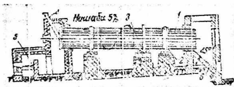
2.5-rasm Quritkich baraban.
