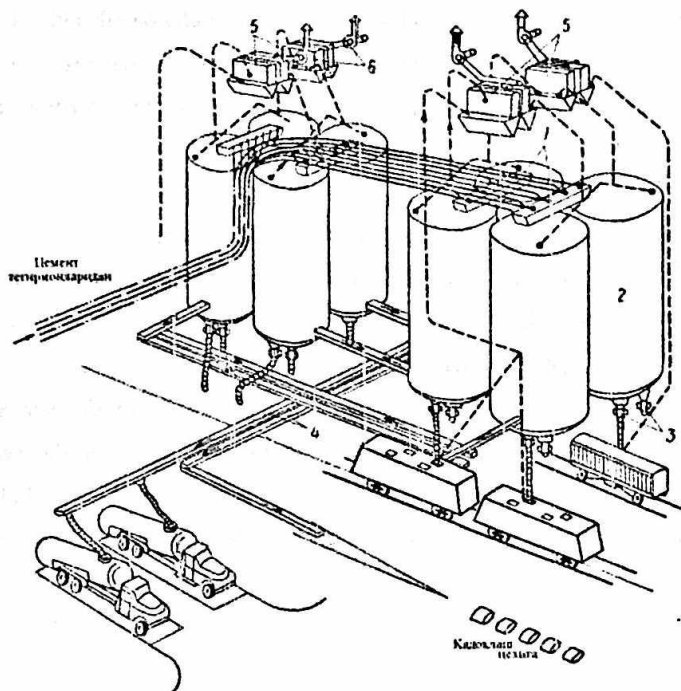
21-rasm. Sementlar uchun siloslarning texnologik chizmasi.
