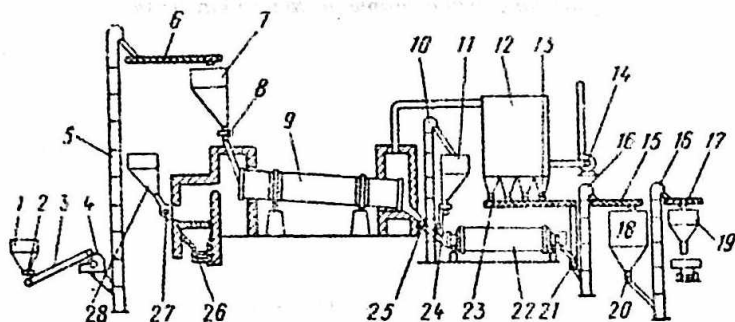
2. 11-rasm. Qurilish gipsini aylanma pechlar (quritish barabanlari)da kuydirish chizmasi: 1-qabul qiluvchi bunker; 2-Lotkli oziqlantiruvchi; 3 – Tasmali konveyer; 4 – Bolg'ali maydalag'ich; 5-Elevator; 6- Shnek; 7-Gipstosh bunkeri; 8,24 - likopchasimon oziqlantiruvchi; 9- quritish barabani; 10-elevator; 11-kuydirilgan gipstosh bunkeri; 12-chang cho'kirtiruvchi kamera; 13,15,17,20,21,23,25 – shneklar; 14 ventilator; 16-elevator; 18,19-tayer mahsulot bunkeri; 22-sharli tegirmon; 26 – Qirib oluvchi konveyer; 27-ko'niirni pnevmomexaniq yuklantiruvchisi; 28- ko'niir bunkeri.
