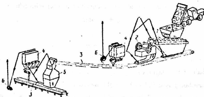
5.1-rasm. Ohaktoshni lunjli, bolg'ali maydalagichda maydalashni texnologik chizmasi: 1,4-yengsimon filtrlar; 2-lentali konveyer; 3-ventilator; 5-lunjli maydalagich; 6-plastinkali oziqlantiruvchi; 7-bolg'ali maydalagich.
