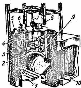
2.1-rasm. Gips pishirish qozoni. 1-o'txona; 2-tuglik; 3-korpus; 4-o't quvurlari; 5-tutun quvuri; 6-bug' olib ketiladigan quvur; 7-aralashtirgich; 8-ohak solinadigan qopqoq; 9-ohak tushirish moslamasi; 10-etishtirish kamerasi.
