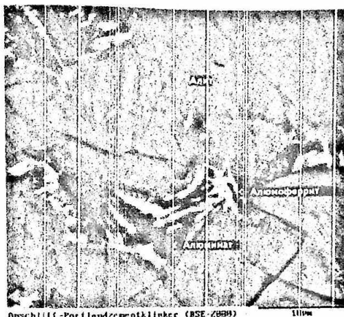
Рис. 2.16. Алюмоферритный аншлифт порцелимента (буз протравливания), изображение в отраженном свете
