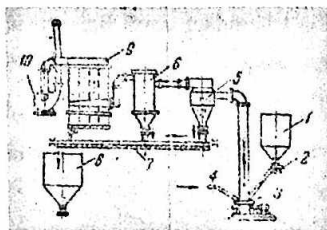
2.4-rasm. Shaxta tegirmondan foydalanib va bir yo'la tuyib- kuydurib gips tayyorlash sxemasi.
