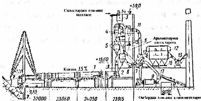
20-rasm. Aylanma o'choq va siklonli issiqlik almashtiruvchilar kuvdirish sexi.
