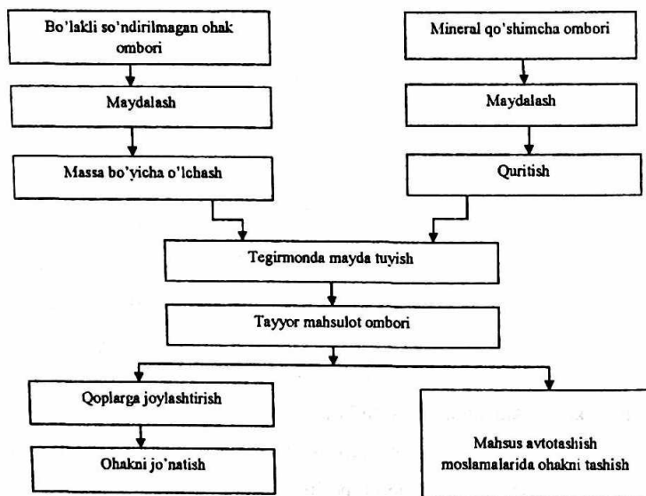
Maydalangan so'ndirilmagan ohakni ishlab chiqarish texnologik chizmasi.
