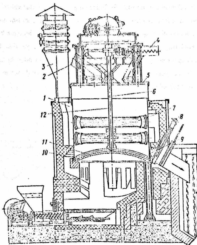
2.8-rasm. Gips pishirish qozoni.
