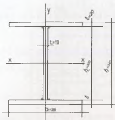
6.4-rasm. Ustunning kesim yuzasi
