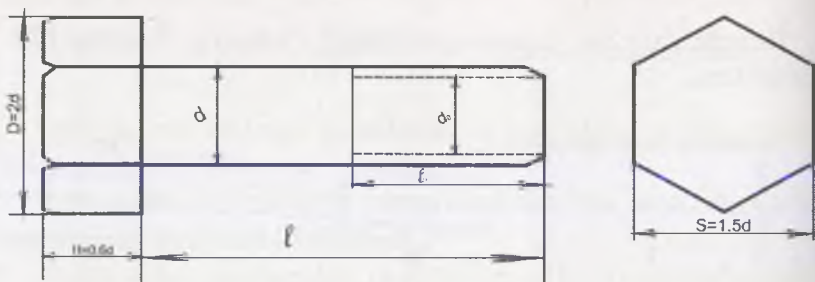
4.6-asm. Bolt
