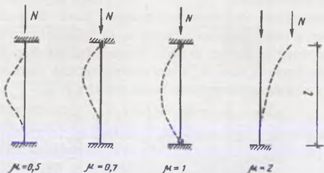
12.5-rasm. Ustunning hisobiy uzunligini aniqlash.
