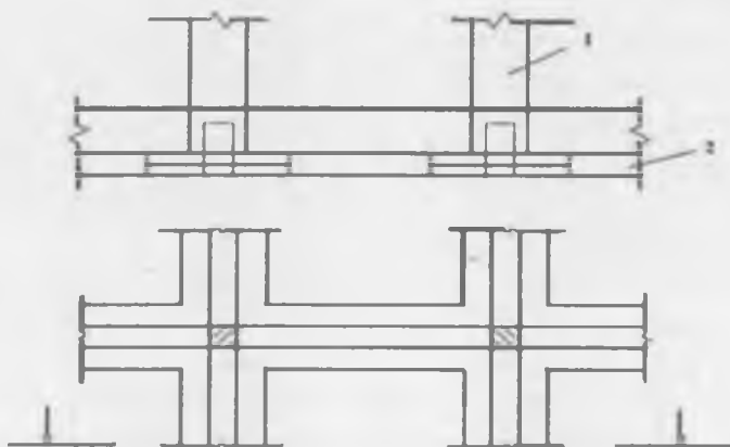
19.3-rasm. Tasma shaklidagi o'zaro kesishgan poydevorlar
