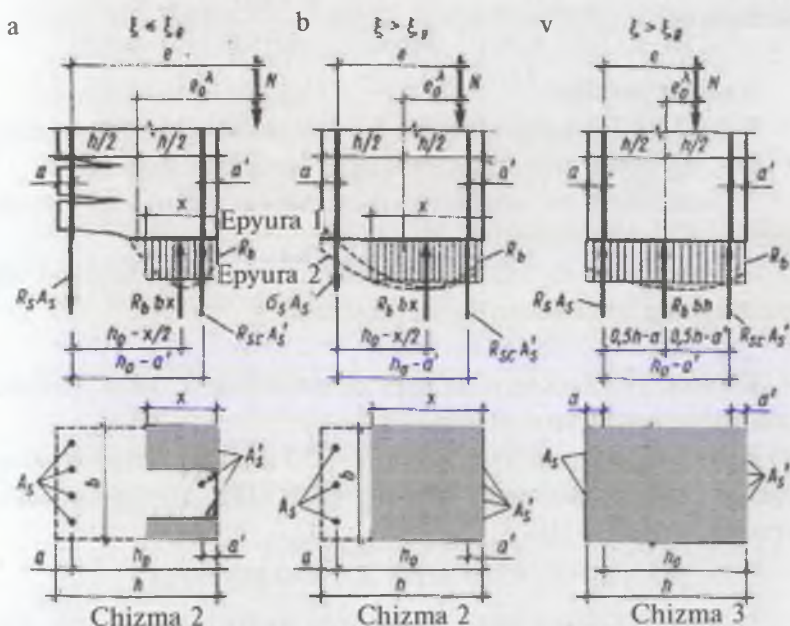
12.5-rasm. Siqiluvchi elementlarni hisoblash tarhi: a – tasodifiy yelka – I_0 ; b – x \leq \xi_R bo'lgan hol uchun; v – x \geq \xi_R bo'lgan hol uchun.
