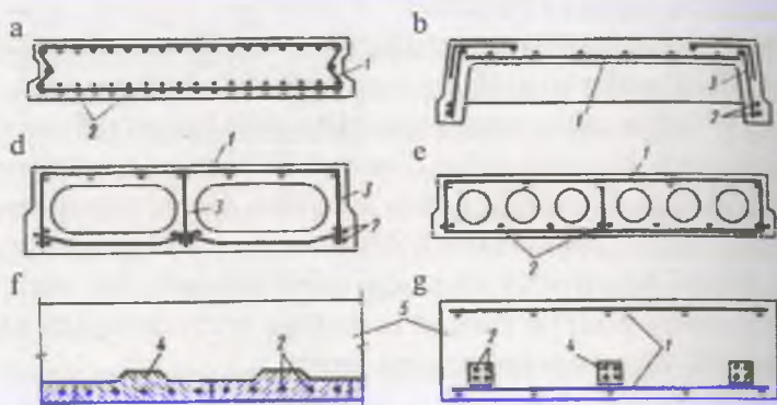
11.2-rasm. Yig'ma, yig'ma-monolit plitalarning ko'ndalang kesimlari:
