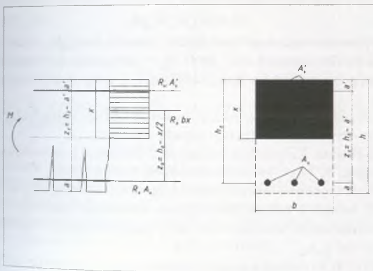
11.8-rasm. To'g'ri to'rtburchak shaklidagi qo'sh armaturali kesimni hisoblash
