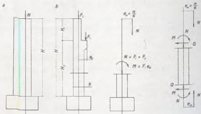
12.1-rasm. Siqilgan elementlar
