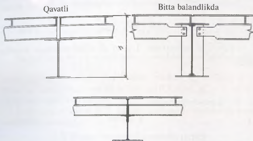
5.2-rasm. Murakkab to'sinli katakda to'sinlarning bir-biriga biriktirilishi
