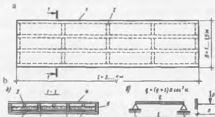
18.2-rasm. Yelimfanerali to'shama: a — to'shama rejasi; b — to'shama qirgimi; v — to'shama hisob sxemasi; 1 — bo'yлама qobirg'a; 2 — ko'ndalang qobirg'a; 3 — ventilyatsiya uchun teshik; 4 — qurilish faneraasi; 5 — namdan himoya qatlami; 6 — to'shama qobirg'asi; 7 — issiqlik saqlovchi qatlam
