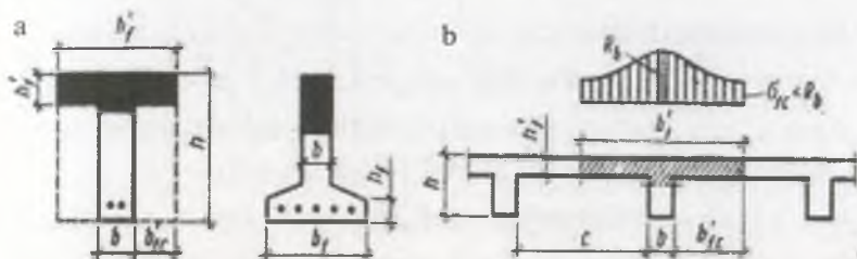
11.9-rasm. Tavr shaklli kesimli to'sinni hisoblashga doir
