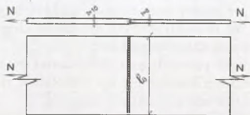
4.4-rasm. Tutash biriktirilgan payvand chok
