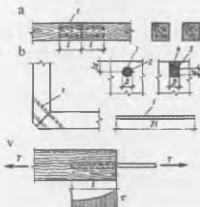
17.5-rasm. Yelimlangan po'latni o'zak orqali birlashtirish: a — bo'yлама yelimlangan; b — qiya tekislik bo'yicha yelimlangan; v — ishlash sxemasi; 1 — po'lat o'zak; 2 — o'zak uchun qoldirilgan tekislik; 3 — o'zak uyasi; 4 — taxta reyka
