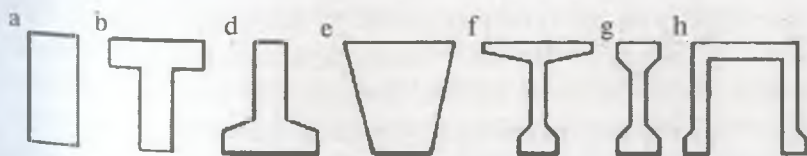
11.3-rasm. Temir-beton to'sinlarning ko'ndalang kesim yuzalari
