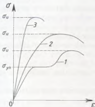
2.1-rasm. Po'latning cho'zilishdagi diagrammasi
