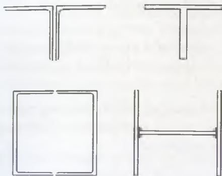
7.2-rasm. Ferma elementlarining kesim yuzasi
