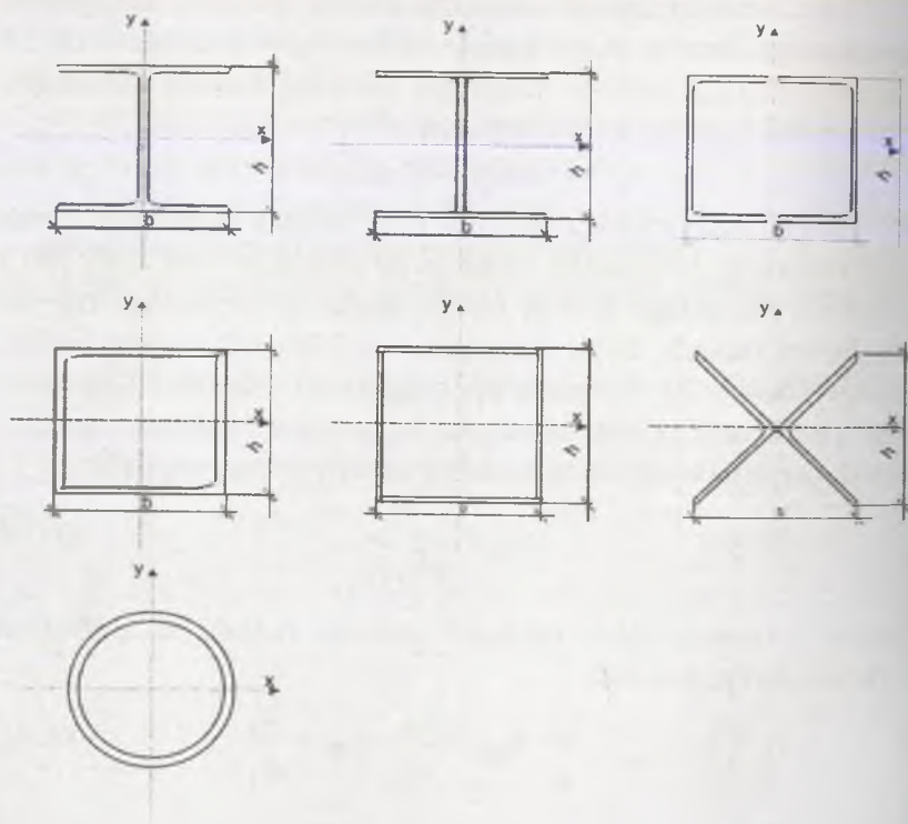
6.1-rasm. Ustunning kesim yuzalari
