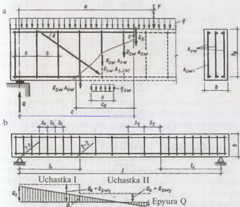
11.12-rasm. Og'ma kesimning ko'ndalang kuchga hisoblash tarhi
