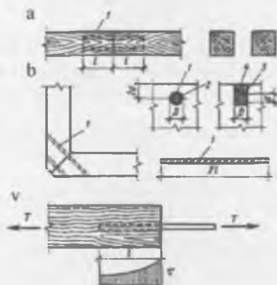
17.5-rasm. Yelimlangan po'latni o'zak orqali biriktirish: a — bo'ylama yelimlangan; b — qiya tekislik bo'yicha yelimlangan; v — ishlash sxemasi; 1 — po'lat o'zak; 2 — o'zak uchun qoldirilgan tekislik; 3 — o'zak uyasi; 4 — taxta reyka
