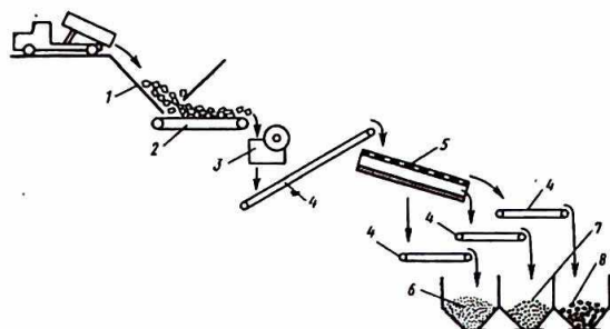
3.10-rasm. Eng oddiy maydalash-navlarga ajratish korxonasi:
