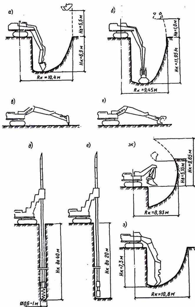
2.8-rasm. Turli ishchi jihozlarga ega bo'lgan EO-5122 ekskavatorning ko'rsatkichlari: a - teskari cho'michli, b - mustahkam shtangadagi greyfer, v - gidravlik bolg'a, g - tutgich, ye - teleskopik shtangadagi greber, j - cho'michi to'g'ri joylashgan, z - yumshatgich, H k - kavlash chuqurligi; H b - kavlash balandligi.
