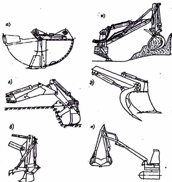
2.7-rasm. Ko'p maqsadli ekskavator ishchi jihozlari:
