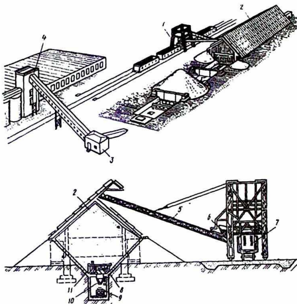
3.17-rasm. To'ldiruvchining shtabel-yarimbunkerli yopiq omborxonasi:
