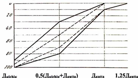
2.6-rasm. Shag'al(chaqiqto'sh)ning donadorlik tarkibi grafigi:
