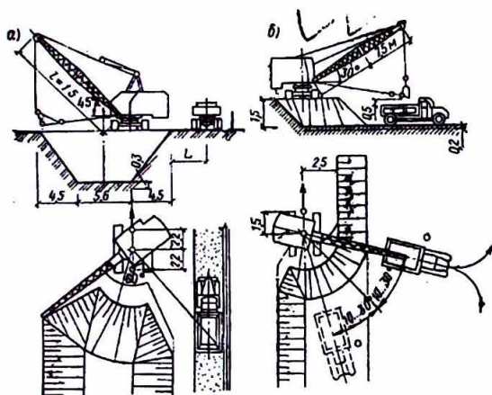
3.6-rasm. Draglayning ishlash sxemasi: a - «peshona» boʻyicha ishlash; b - yonlama boʻyicha ishlash.
