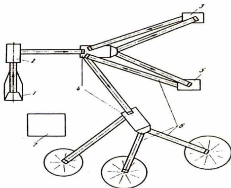
3.15-rasm. Harakatlanuvchi maydalash-navlarga ajratish uskunasi PDSU-85: 1-ta'minlovchi bilan birgalikda qabul bunker; 2-yiriklashtirib maydalash uskunasi; 3- o'rtacha maydalash uskunasi; 4-navlarga ajratish uskunasi; 5- o'ta maydalash uskunasi; 6-lentali konveyrlar; 7-boshqaruv tugmasi uskunasi.
