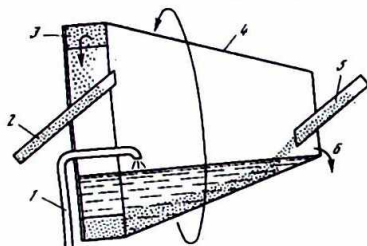
3.3-rasm. Qum yuvish apparati:
