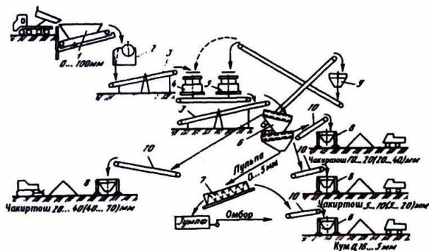
3.14-rasm. O'tqindi jinslarni qayta ishlovchi avtomatlashgan maydalash liniyasi SADL-1-400 sxemasi:
