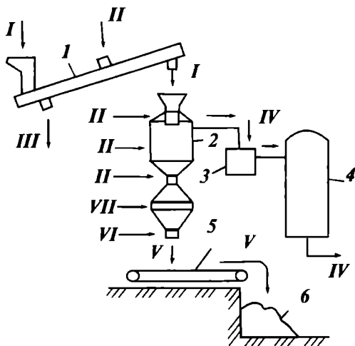
16.2-расм. Кира таркибидан асфальт ва суюқ битум — мальтани олиш технологияси:
