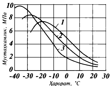
17.13-расм. Асфальт-бетоннинг эгилишга бўлган мустаҳкамлигига ҳароратнинг таъсири:
