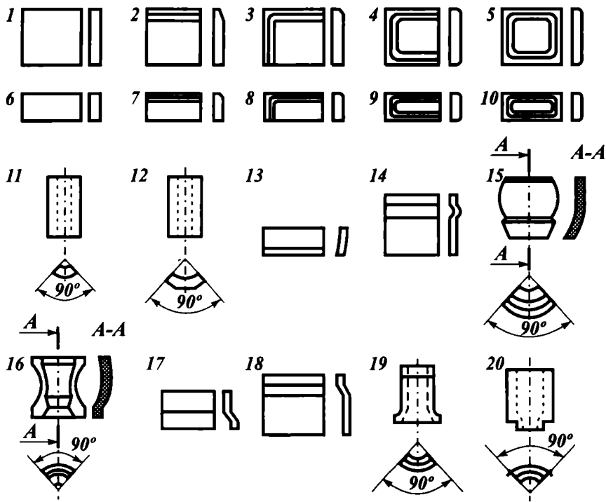
7.12-расм. Ички деворларни қоплашда ишлатиладиган сопол тахтачаларнинг хиллари:
