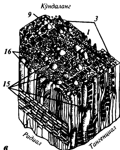
4.2-расм Дарахтларнинг микротузилиши:
