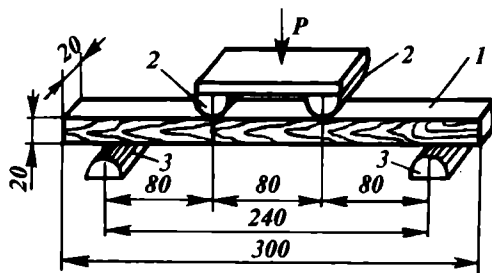
4.11-расм. Ёғоч намунани статик эгилишга синаш:
