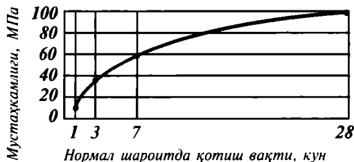
12.7-рассм. Бетон мустаҳкамлигининг ортиши.
