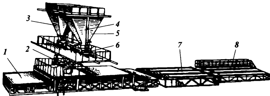
10.6-ра с м. Гипс бетон панелларини прокат усулда ишлаб чиқариш:
