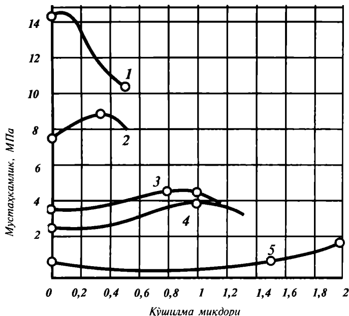
11.2-расм. Қўшиладиган оҳак ва тупроқнинг миқдорига қўра қоришма мустаҳкамлигининг ўзгариши:
