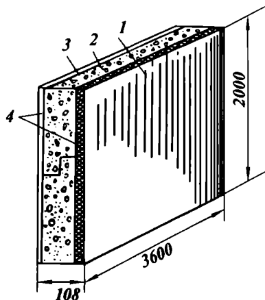
8.3-расм. Кўп қатламли ойна тахта панел:
