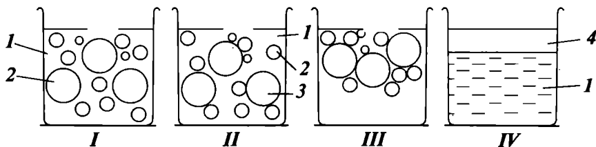
16.3-расм. Эмульгатор қўшилмаган сувдаги битум заррачаларининг ҳолати: I—IV — битум заррачаларининг сараланиши; 1—сув; 2—битум заррача; 3—ўзаро ёпишиб қолган зарра; 4—ўзаро бирлашган битум қатлами.
