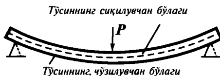
2.11-расм. Икки таянчдаги тўсиннинг эгилиши.
