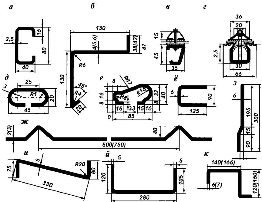
13.5-расм. Букилган узун пўлат буюмлар:
