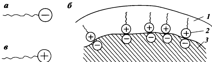
17.6-расм. СФМ қўшилган битумнинг тўлдиргич дона сиртига ёпишиш схемаси:
