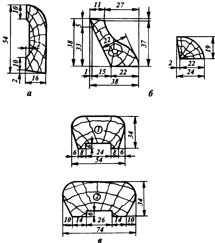
4.28-расм. Плинтус (а), галтель (б), зина тутқичлар (в).
