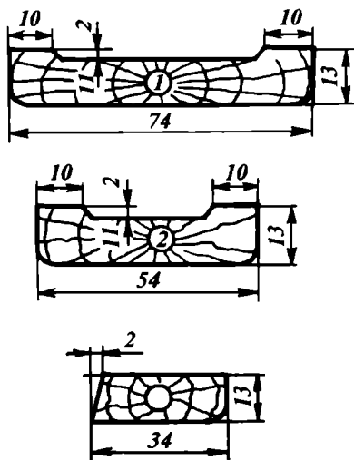
4.27-рasm. Часпақлар (доира ичидаги рақам часпақ типини билдиради).
