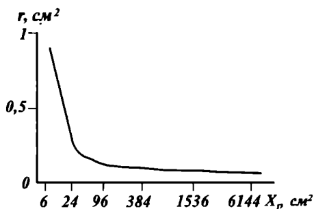
1.3-расм. Туйилган заррача ўлчамининг (г) солиштирма сирти билан боғлиқлиги.
