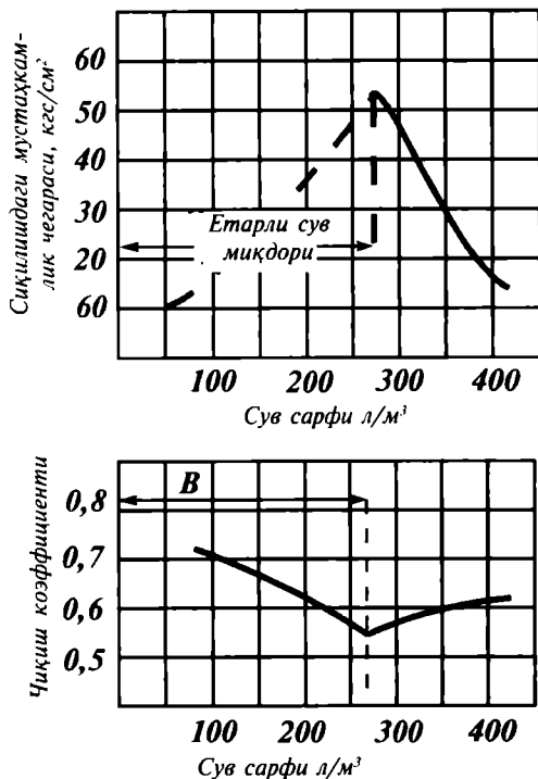
12.14-расм. Енгил бетоннинг мустаҳкамлиги ва унинг чиқиш коэффициенти билан сув миқдори орасидаги боғланиш.
