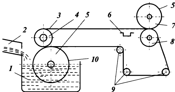
10.3-расм. Асбест-цемент буюмлари ишлаб чиқаришда ишлатиладиган қолипловчи машинанинг ишлаш схемаси:
