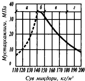
12.5-расм. Бетоннинг сиқилишдаги мустаҳкамлигининг сув миқдoriga боғлиқлиги:
