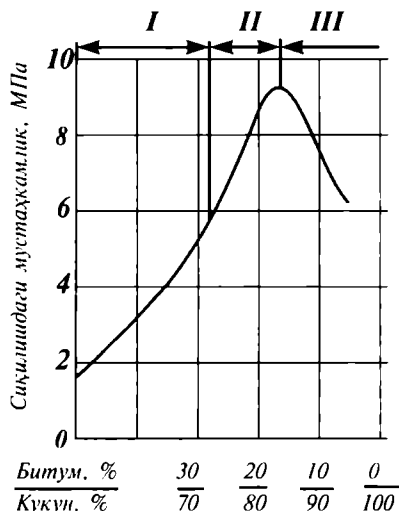
17.5-расм. Минерал кукунининг асфальт-бетон мустаҳкамлигига таъсири.
