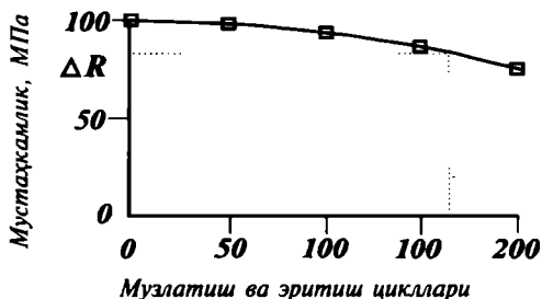
2.4-расм. Музлатиб, эритиш жараёнининг бетон мустаҳкамлигига таъсири.
