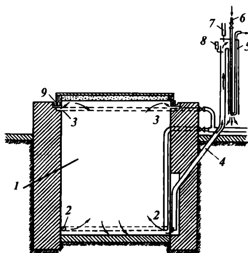
12.11-расм. Буғлаб қотирувчи автомат бўлма схемаси:
