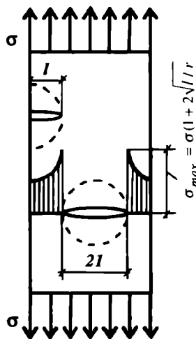
2.14-расм. Ўртаси дарзли тахтачада кучланишнинг тарқалиши.
