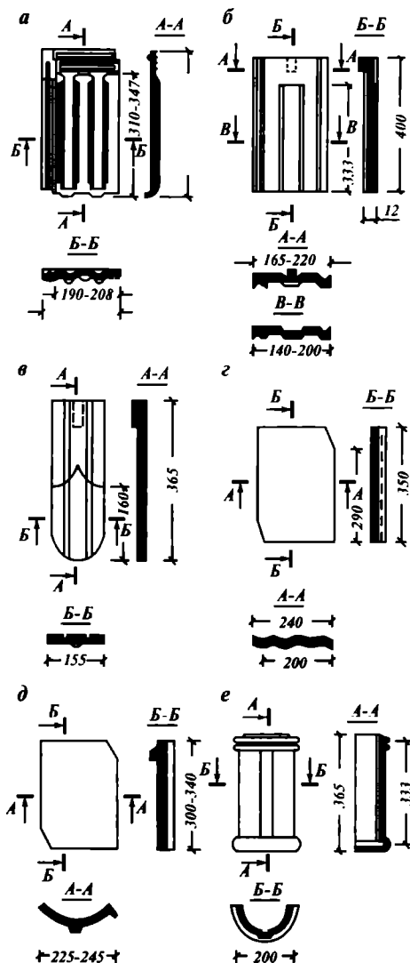
7.13-расм. Томбоп сопол черепица турлари:
