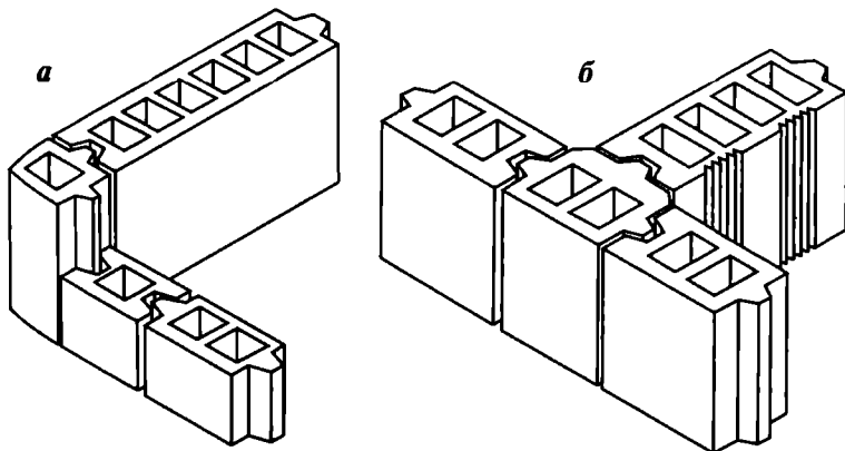
10.5-расм. Экструзия усулида тайёрланган деворбоп панеллар:
