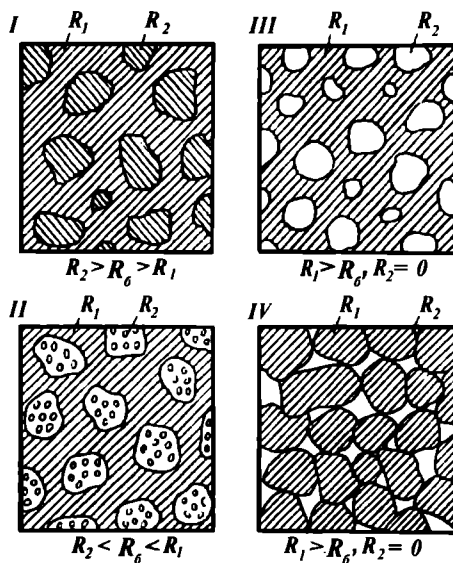
12.8-расм. Бетон структурасининг турлари:
