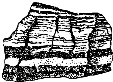
5.7-расм. Қатлам тузилишидаги гнейс.
