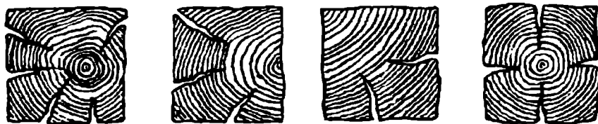
4.7-расм. Тўсиннинг тез қуриши натижасида ёрилиши.
