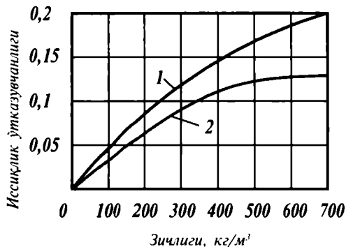
15.1-расм. Қурилиш ашёларининг иссиқлик ўтказувчанлиги билан зичлиги орасидаги боғлиқлик:
