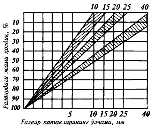
12.13-расм. Енгил бетонлар учун майда-йирик-лиги энг қулай бўлган тўлдиргичлар. Доналар-нинг энг йириги:
