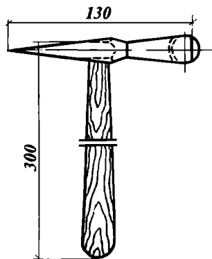
2.22-расм. Физделнинг золдирли болғаси.
