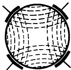
4.32-расм. Ёғочни юқори частотали ток билан қуритиш схемаси.
