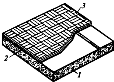
4.30-расм. Паркет пол:
