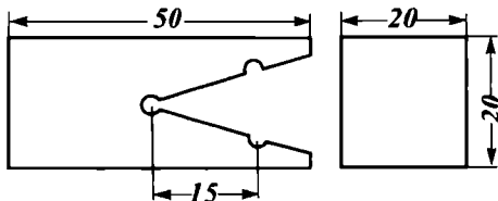
4.10-расм. Ёғочни ёрилишга синаш учун тайёрланган намуна.
