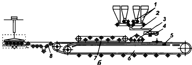
14.6-расм. Темир-бетон буюмлар тайёрлайдиган тебратма-прокат стани:
