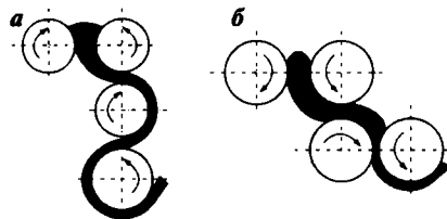
18.3-расм. Тўрт жўвали каландрнинг ишлаш схемаси:
