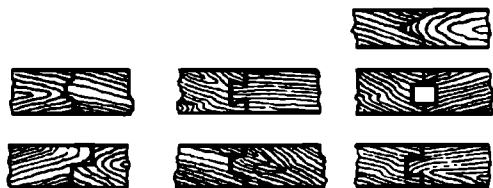
4.26-рasm. Шпунтли тахталар.
