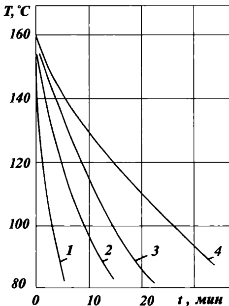
17.10-расм. Асфальт-бетон совиш тезлигининг қатламининг қалинлигига боғлиқлиги: 1—2 см; 2—4 см; 3—6 см; 4—8 см.
