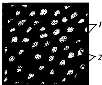
17.4-расм. Минерал кукунининг битум бўтқаси:
