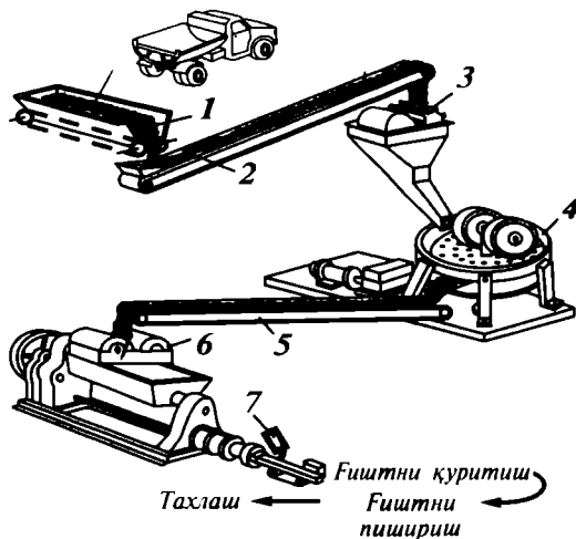
7.2-расм. Пластик усулда фишт ишлаб чиқариш схемаси:
