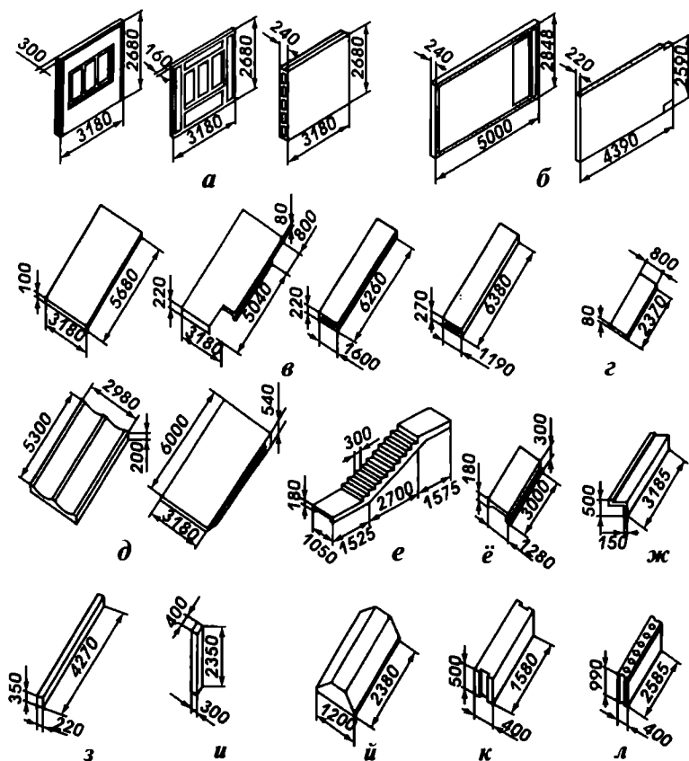
14.11-расм. Турар жой биноларида ишлатиладиган йўғма темир-бетон буюмлар:
