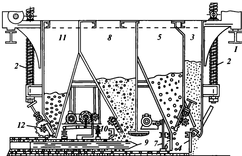
14.9-расм. Кўп бўшлиқли ёпма плиталарни қопловчи агрегат:
