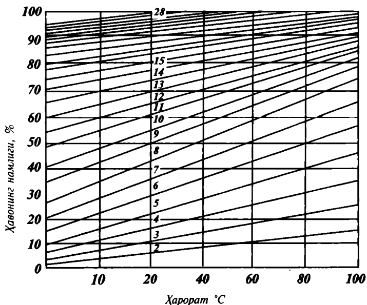
4.6-расм. Ёғочнинг мувозанат намлигини аниқлайдиган номограмма.
