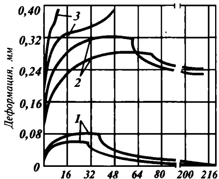
17.14-расм. Бир хил кучланишдаги асфальт-бетоннинг деформацияси:
