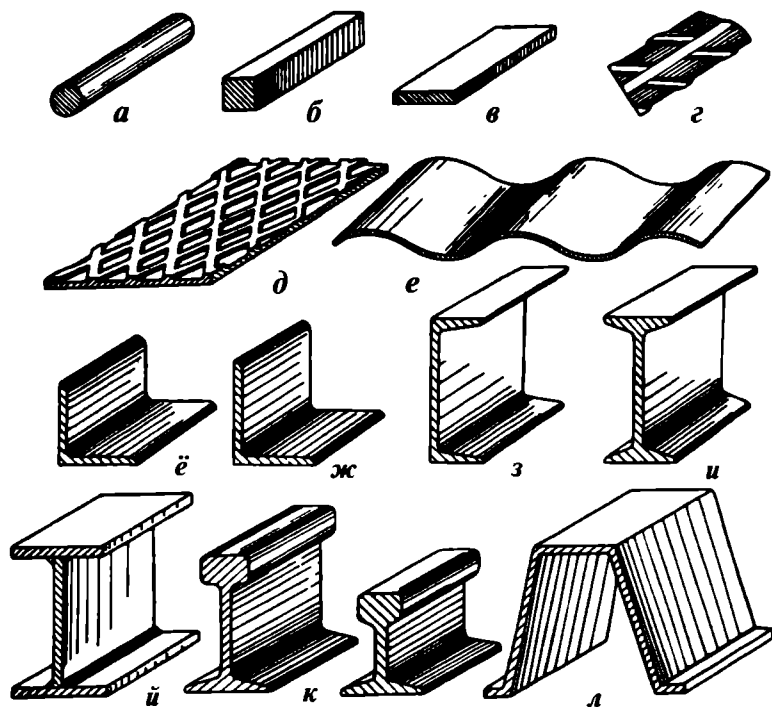
13.4-расм. Пўлат навлари:
