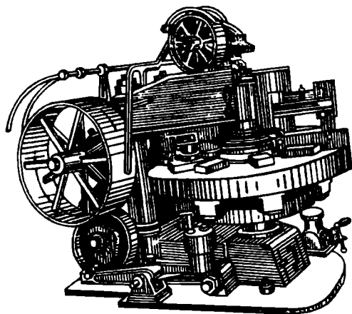
10.1-расм. Силикат гиштни қолипловчи пресс.
