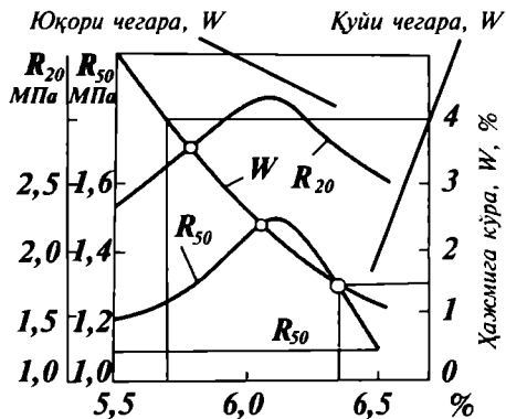
17.9-рasm. Асфальт-бетон қоришмаси учун битум миқдорини аниқлаш.
