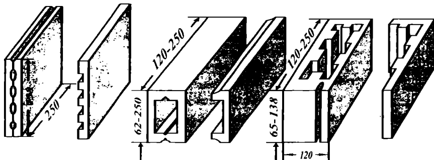
7.9-расм. Фасадбоп қоплама сопол тахтача.
