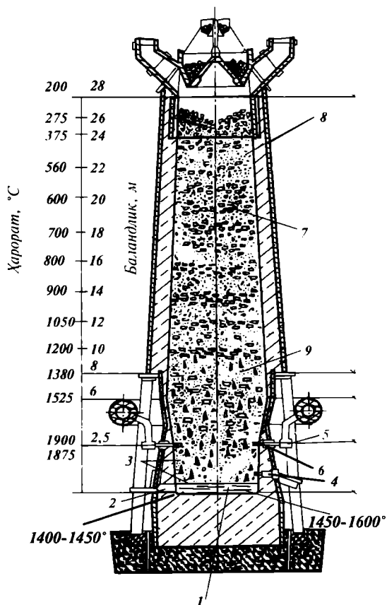
13.2-расм. Домна ўчоғи:
