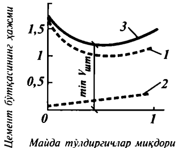
12.4-расм. Кум ва шағал миқдорига кўра цемент бўтқасининг сарфи: 1—тўлдиргич доналариаро бўшлиқни тўлғизиш; 2—доналар юзасини қоплаш; 3—майда ва йирик тўлдиргич оғирлиги.
