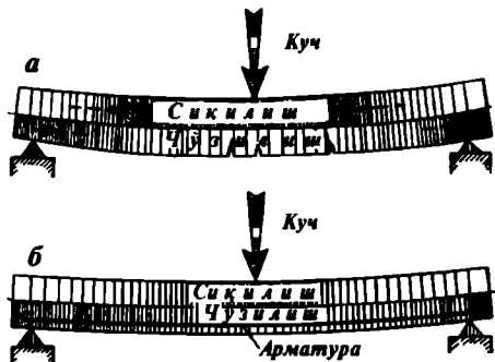
14.1-расм. Бетон ва темир-бетон тўсиннинг эгилиш схемаси:
