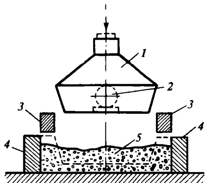
12.9-расм. Титратиб штамплаш усули билан буюм тайёрлаш:
