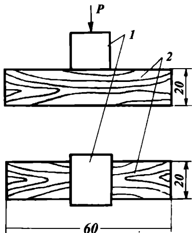
4.9-расм. Ёғочнинг толаларига кўндаланг сиқилишдаги мустаҳкамликни аниқлаш.
