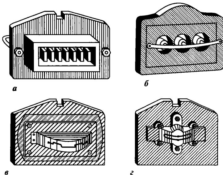
7.3-расм. Тасмали зичлагичга ўрнатиладиган мундштук: а — ичн говак гиштбон мундштук; б — қувур мундштуғи; в, г — тасмали черенина мундштуғи
