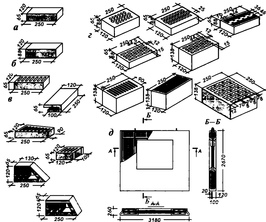
7.5-расм. Деворбоп сопол ашёларнинг асосий турлари:
