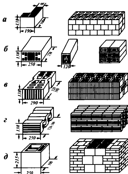
7.6-расм. Ёриқ кавакли тошлар ва улардан девор териш:
