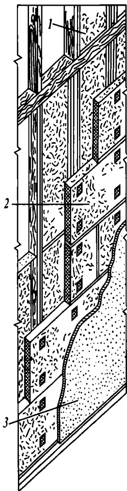
15.2-расм. Ёғоч синчли бино деворларини фибролит билан қуриш:
