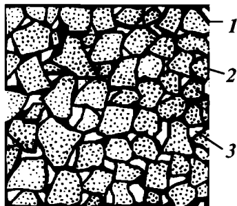
17.2-расм. Зичланган қора шағалли қоришманинг тузилиши:
