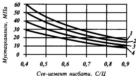
12.6-расс. Бетон мустақхамлиги билан C/\Pi нисбати ўртасидаги боғланиш: 1—М600; 2—М500; 3—М400; 4—М300.
