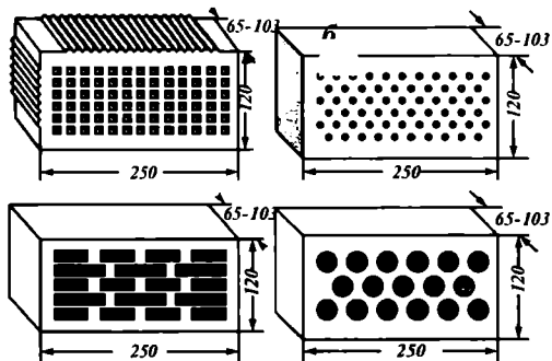
7.7-расм. Кўп тешикли ғиштлар.
