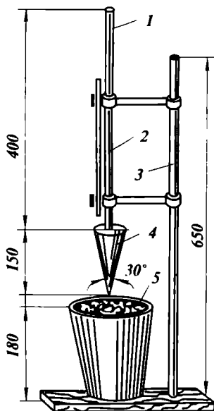
11.1-рasm. Қоришма ёйилувчанлигини аниқлайдиган конус:
