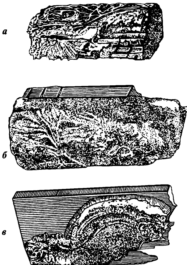
4.22-расм. Ёғочнинг замбуруғ касаллиги билан шикастланиши: а—ҳақиқий уй замбуруғи; б—духоба уй замбуруғи; в—юпка қатламли замбуруғ.
