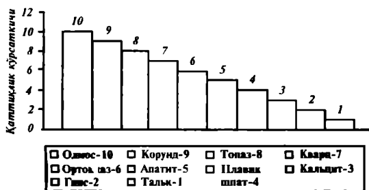
5.8-расм. Минералларнинг қаттиқлик шкаласи.
