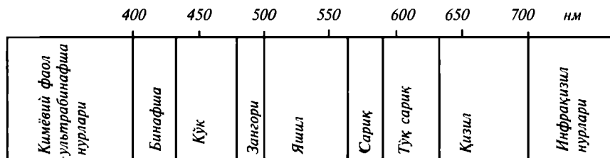
2.19-расм. Спектрнинг тўлқин узунлиги.
