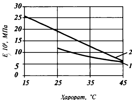
17.3-расм. Иссиқ ҳароратда Бекобод тошқоли ишлатилган асфальт-бетон эластиклик модули динамикасининг ўзгариши: 1—икки ҳафталик намуна; 2—беш ойлик намуна.
