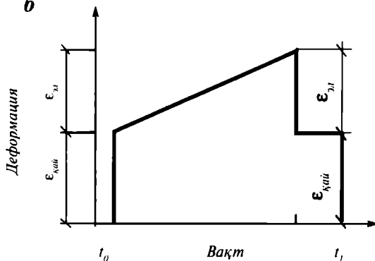
2.17-расм. Эластик ва қайишқоқ хоссали ашё модели:
