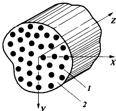
3.1-рasm. Монотроп композит кесими:
