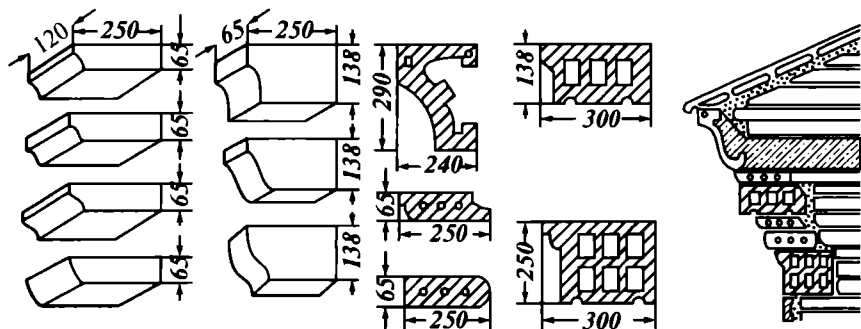
7.8-расм. Профилли деворбоп гиштлар ва қисмлар.
