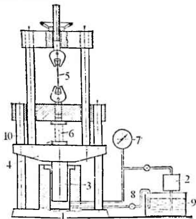
3.1-chizma. Gidravlik sinov mashina sxemasi
