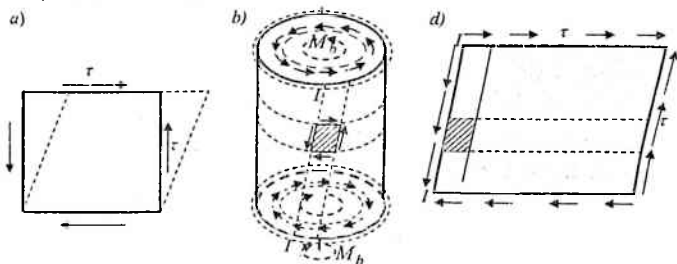
5.1. Brusdan ajratilgan elementning sof siljish holati
