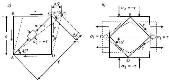
5.3-chizma. Ajratilgan elementda hosil bo'lgan kuchlanishlar
