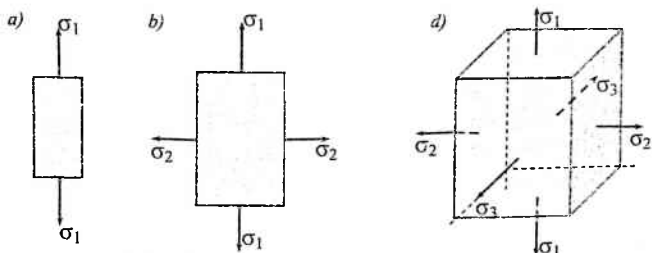
4.15-chizma. Kuchlanganlik holati turlari
