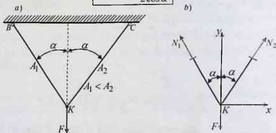
2.16-chizma. Sterjenlar sistemasi
