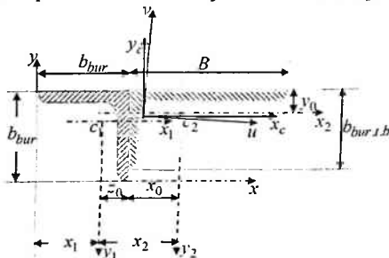
6.15-chizma. Teng yonli va teng yonli bo'lmagan burchakdan tashkil topgan murakkab kesim bosh o'qlar holati
