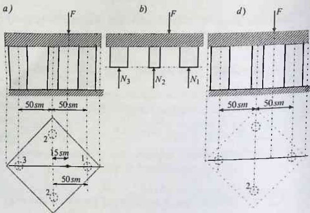
2.25-chizm. To'rtta ustunga tayangan plita
