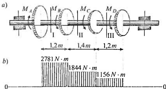
7.10-chizma. Buruvchi moment epyurasi
