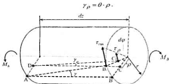
7.4-chizma. Uzunligi dz bo'lgan ajratilgan element
