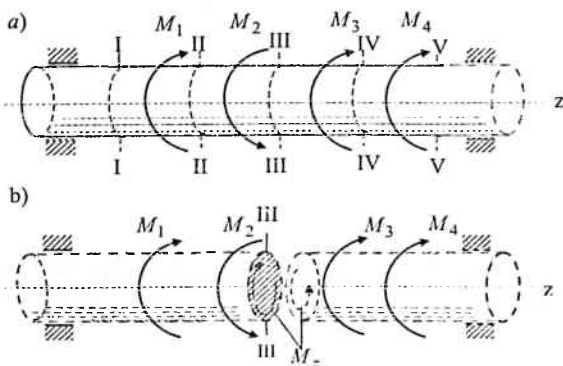
7.1-chizma. Turli ko'ndalang kesimlariga qo'yilgan sirtqi momentlar ta'siridagi val
