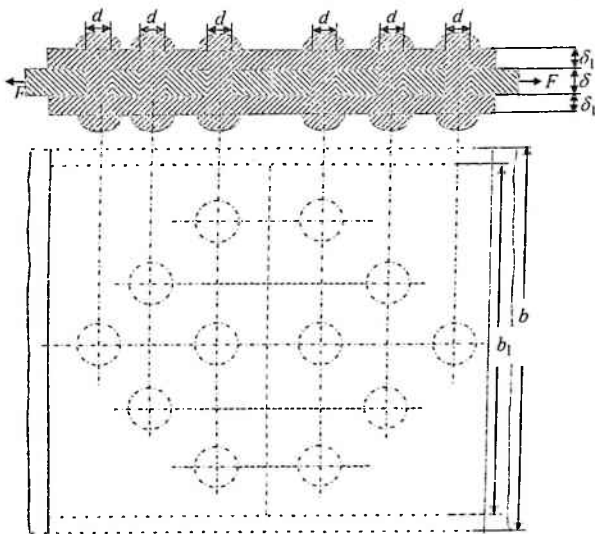
5.18-chizma. Ustqo'ymali ikki kesimli parchin mixli birikma
