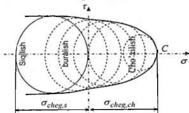
4.18-chizma. Bosh kuchlanishlari turlicha bo'lgan chegaraviy doiralarni o'rab turuvchi egri chiziq
