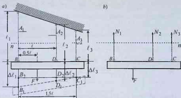
2.11-chizma. Sterjenlar sistemasi
