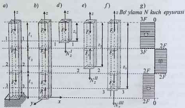
2.2-chizma. To'plangan kuchlardan cho'zilgan siqilgan sterjen
