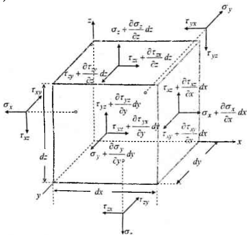
4.12-chizma. Tomonlari koordinatalar tekisliklariga parallel bo'lgan element
