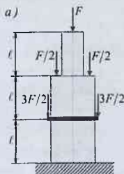
2.29-chizma. Ikki pog'onali siqilgan sterjen
