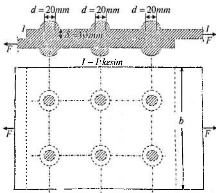
5.20-chizma. Ustma-ust qo'yilgan bir kesimli ikki qatorli parchin mixli birikma
