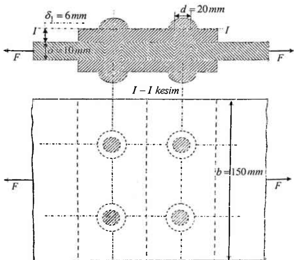
5.21-chizma. Ustqo'ymali bir kesimli ikki qatorli parchin mixli birikma
