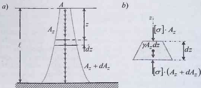
2.8-chizma. Teng qarshilikli sterjen
