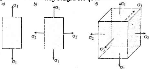
4.2-chizma. Kuchlanganlik holati turlari
