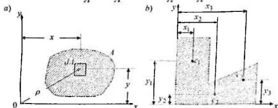
6.2-chizma. Tekis kesim yuzalari
