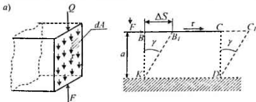
5.2-chizma. Brusning ko'ndalang kesimlarida urinma kuchlanish
