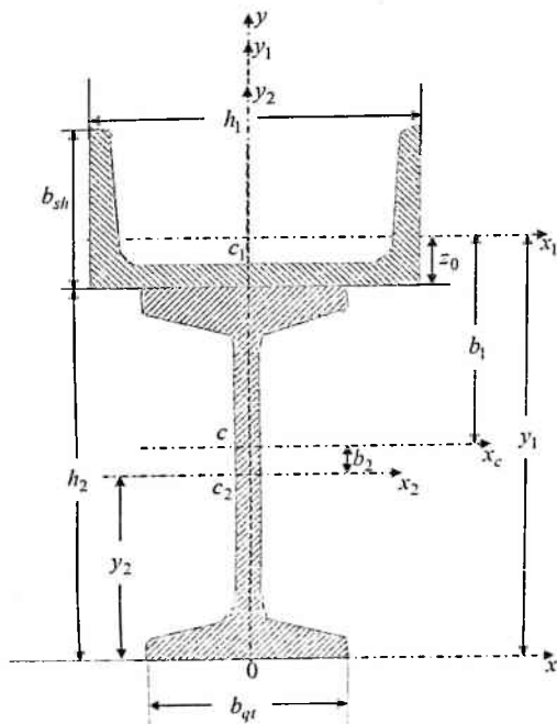
6.11-chizma. Qo'shtavr va shvellardan tuzilgan murakkab ke-sim.
