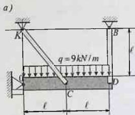
2.30-chizma. Ikki tortqi yordamida osilgan konstruksiya
