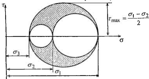
4.17-chizma. Mor doirulari
