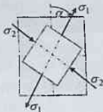
2.34-chizma. Bosh kuchlanishlar ta'siridagi element
