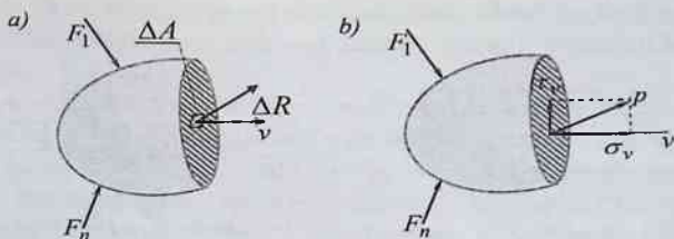
1.5-chizma. Jism kesimidagi kuchlanishlar
