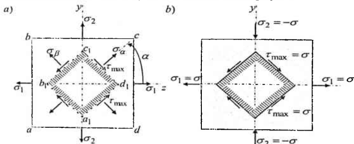
4.8-chizma. Ekstremal urinma kuchlanishlarni aniqlash uchun element
