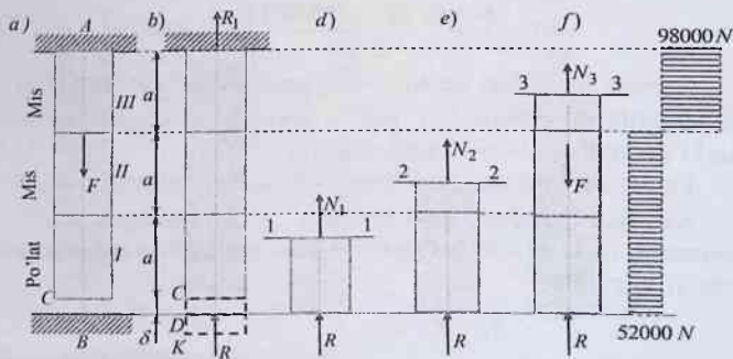
2.26-chizma. Statik aniqlanmas sterjen
