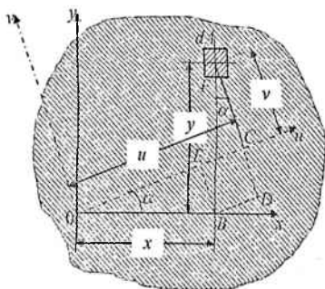
6.7-chizma. Koordinata o'qlari burilganda inersiya momentlarining o'zgarishi
