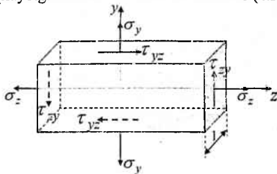
4.3-chizma. Tekis kuchlanganlik holatidagi element
