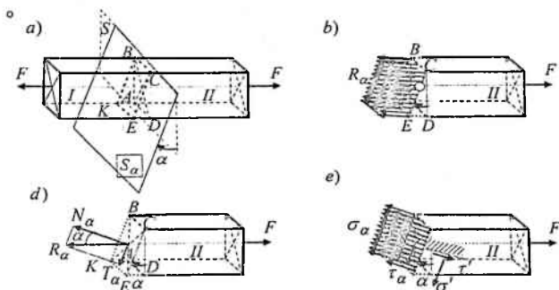
4.4-chizma. Tashqi kuchlar ta'siridagi sterjen
