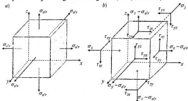
4.13-chizma. Shar va deviator tenzor kuchlanganlik holatlari
