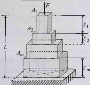
2.9-chizma. Pog'onali sterjen
