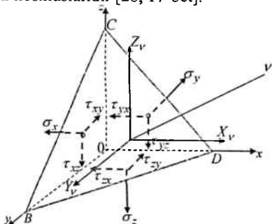
4.14-chizma. Parallelepipedning qiya kesim yuzasi
