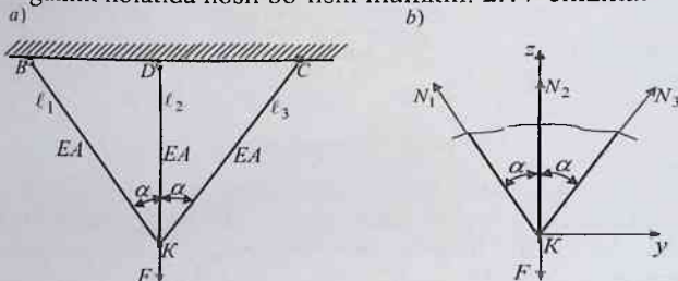
2.17-chizma. Statik aniqmas sterjenlar sistemasi
