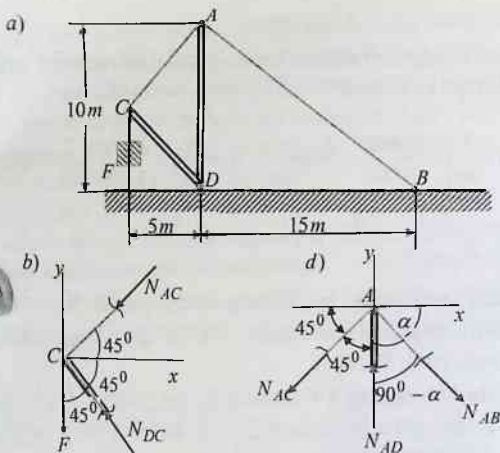
2.21-chizma. Yuk ko'tarish krani sxemasi
