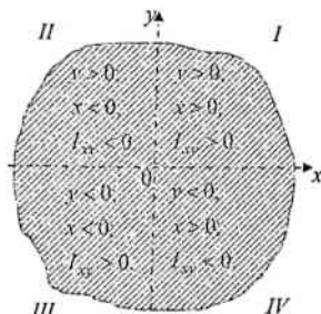
6.3-chizma. Markazdan qochirma inersiya moment ishoralari
