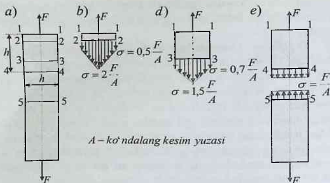
1.7-chizma. To'plangan kuchdan cho'zilgan sterjen
