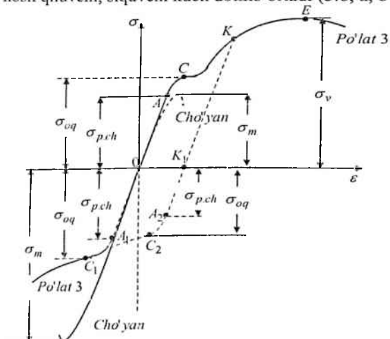
3.8-chizma. Po'lat va cho'yan namunaning cho'zilish va siqilish diagrammalari
