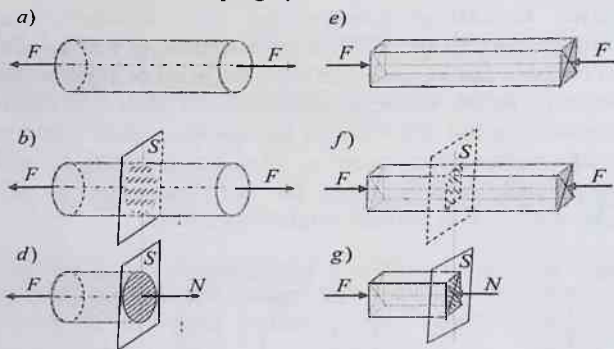
2.1-chizma. To'g'ri o'qli sterjenning cho'zilishi va siqilishi
