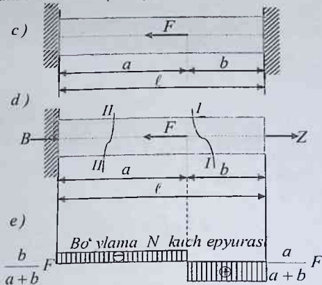
2.10-chizma. Statik aniqlamas sterjen
