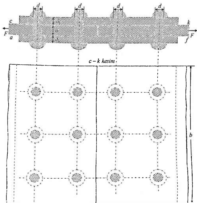
5.5-chizma. Ustqo 'ymali parchin mixli birikma
