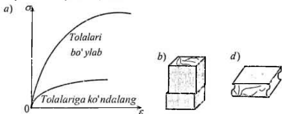
3.11-chizma. Yog‘och namunaning siqilish diagrammalari
