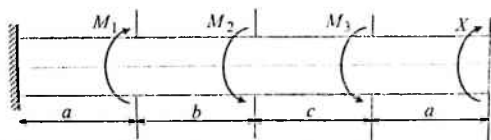
10.8-chizma. Buruvchi momentlar bilan yuklangan val
