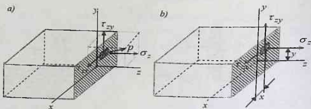
1.6-chizma. To'la kuchlanishning tashkil etuvchilari
