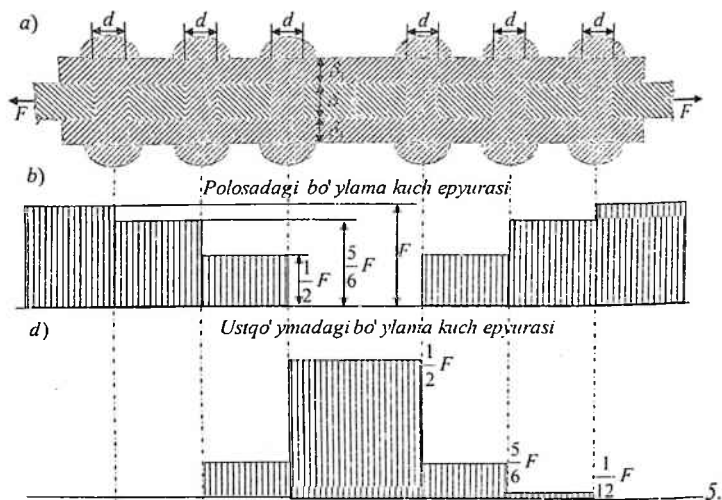
19-chizma. Zo'riqish kuchlari epyuralari
