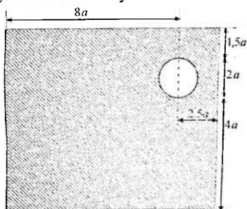
6.18-chizma. Doiraviy shakldagi teshigi bo'lgan to'rt burchakli murakkab kesim
