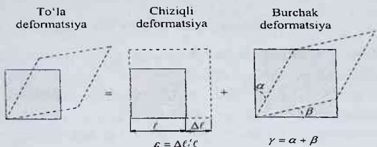
1.4-chizma. Deformatsiyalar
