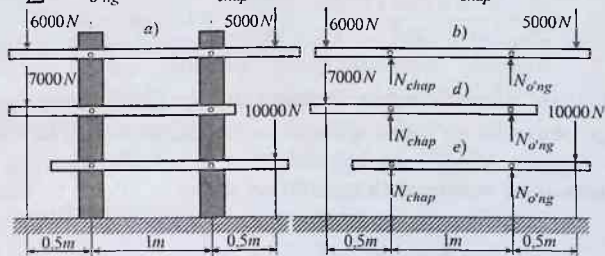
2.18-chizma. Gorizontaal bikir elementlar sharnirli ikkita ustunga biriktirilgan konstruktsiya
