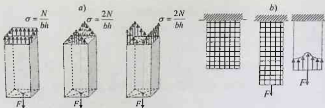
2.3-chizma. Normal kuchlanishning tarqalish qonunlari
