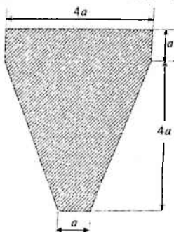
6.16-chizma. Konussimon murakkab kesim
