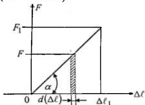
3.14-chizma. Cho'zilish diagrammasi
