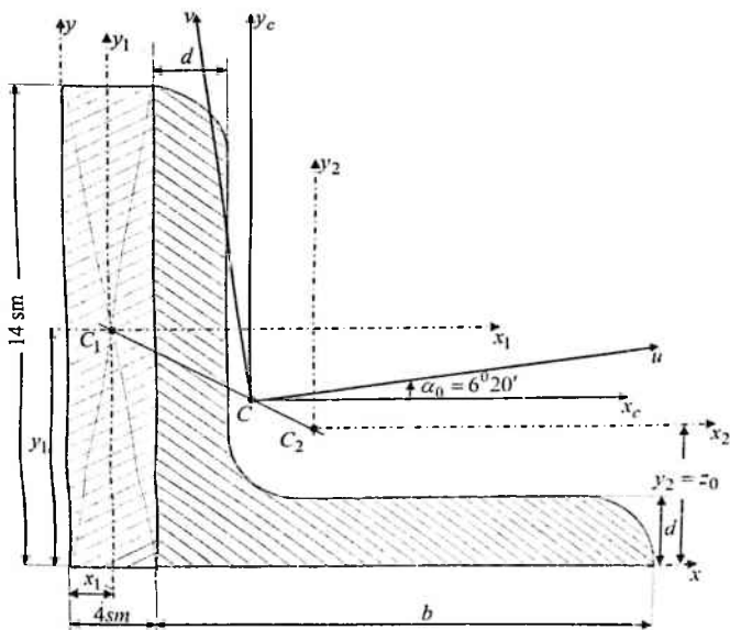
6.10-chizma. To'g'ri to'rtburchak va burchakdan tashkil topgan murakkab kesim
