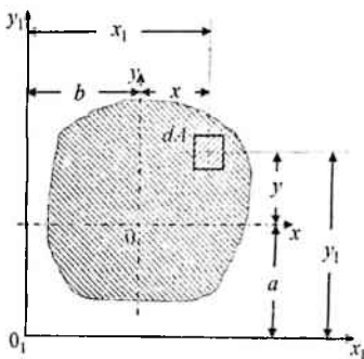
6.6-chizma. Parallel koordinatalar tizimida joylashgan tekis kesim
