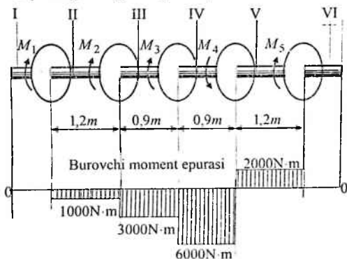
7.2-chizma. Burovchi moment epyurasi
