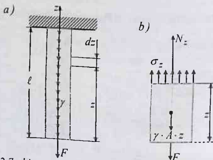
2.7-chizma. Xususiy og'irlikli uzun sterjen
