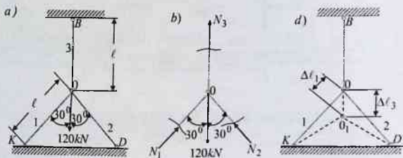
2.23-chizma. Ferma.
