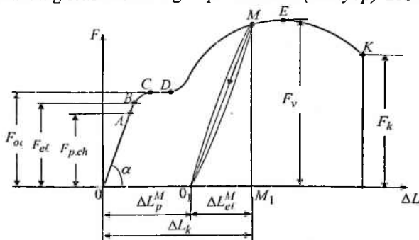
3.6-chizma. Kam uglerodli po'latning cho'zilishi diagrammasi
