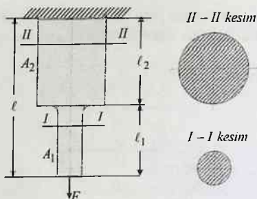
2.15-chizma. Pog'onali sterjen
