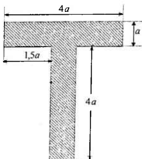
6.17-chizma. Tavr shaklidagi kesim
