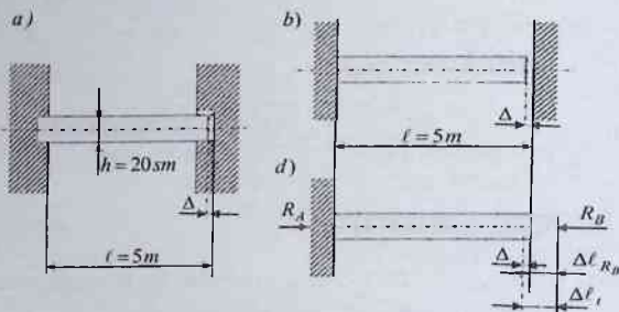
2.27-chizma. Temperatura ta'siridagi tirqishli sterjen
