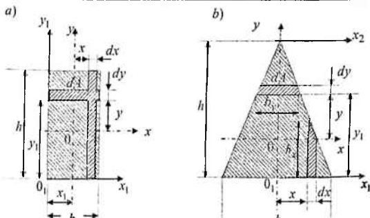
6.4-chizma. To'g'ri to'rtburchak va uchburchak kesim yuzalari
