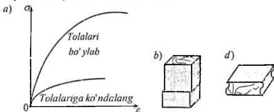
3.11-chizma. Yog‘och namunaning siqilish diagrammalari
