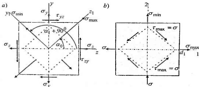
4.7-chizma. Tekis kuchlanganlik holatidagi element
