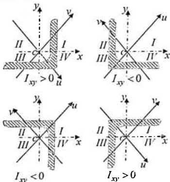
6.9-chizma. Bosh o'qlar ma'lum bo'lganda markazdan qochirma inersiya moment ishoralari
