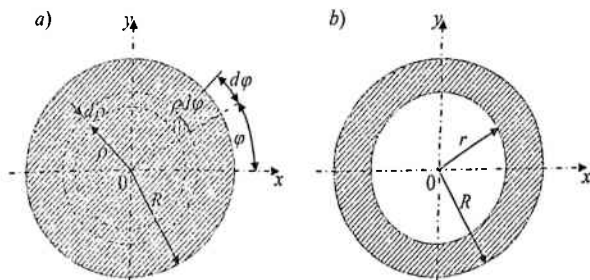
6.5-chizma. Doira va halqa kesim yuzalar
