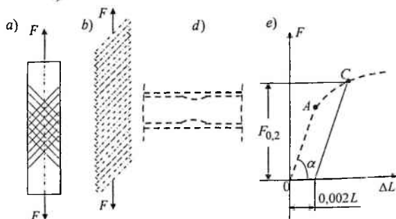
3.5-chizma. Deformatsiyaning hosil bo'lish mexanizmi
