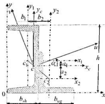
6.12-chizma. Shveller va burchakdan tashkil topgan murakkab kesim
