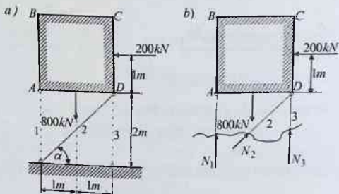
2.20-chizma. Poydevorga uchta sterjenlar yordamida biriktirilgan konstruksiya
