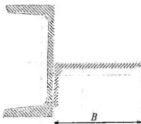
6.20-chizma. Shveller va teng yonli bo'lmagan burchakdan tashkil topgan murakkab kesim
