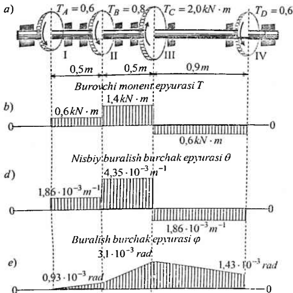
7.11-chizma. Burovchi moment va buralish burchak epyuralari
