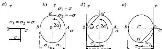
4.11-chizma. Turli kuchlanganlik holatlari uchun Mor doirasi
