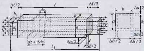
2.4-chizma. Cho'zuvchi kuch ta'siridagi sterjen
