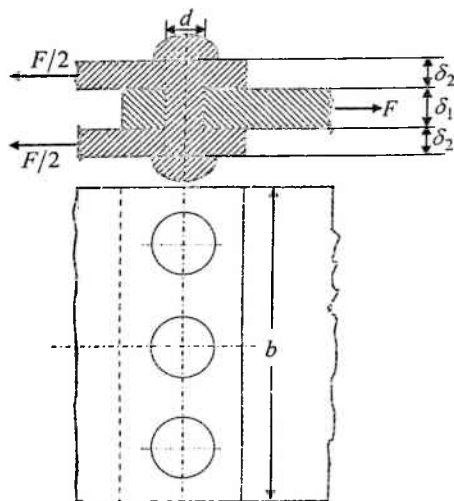
5.16-chizma. Ustma-ust qo'yilgan ikki kesimli parchin mixli birikma
