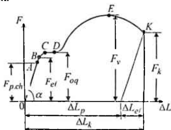
3.3-chizma. Kam uglerodli po'lat namunaning cho'zilish diagrammasi
