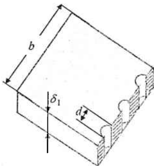
5.17-chizma. Polosaning ko'ndalang kesimi
