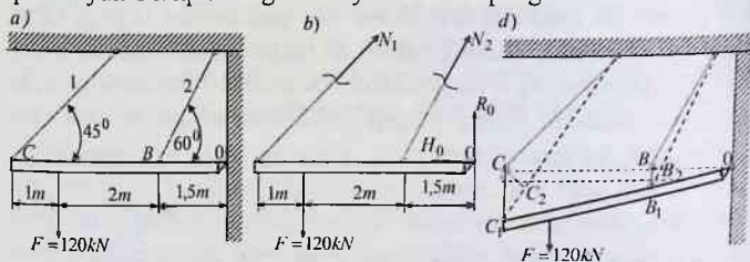
2.24-chizma. Ikkita tortqi bilan ushlab turilgan konstruksiya
