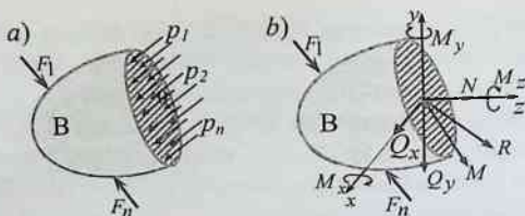
1.3-chizma. Tashqi va ichki kuchlar ta'sirida muvozanat holatdagi jism
