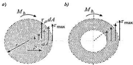
7.5-chizma. Urinma kuchlanishning kesim bo'yicha o'zgarar qonuni
