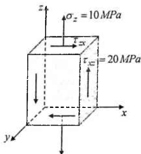
4.23-chizma. Tekis kuchlanganlik holatidagi element
