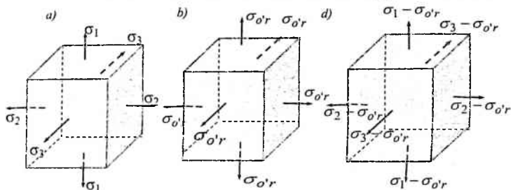
4.16-chizma. Shar va devaztor kuchlanganlik holatlari
