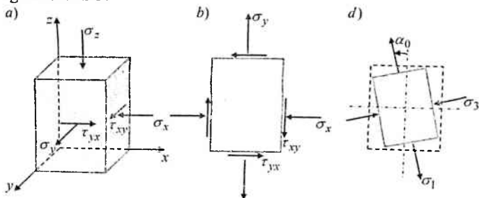
4.22-chizma. Konstruksiya elementining kuchlanganlik holati
