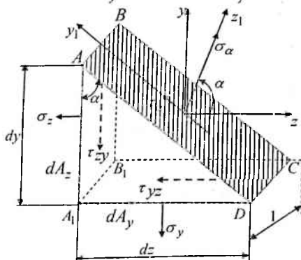
4.6-chizma. Elementar uchburchak prizma
