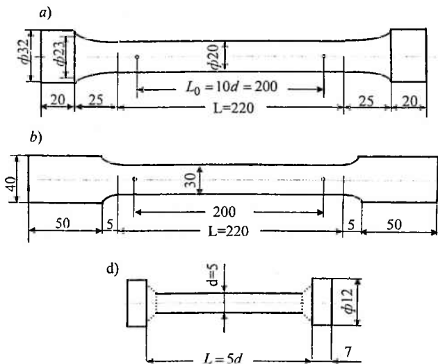
3.2-chizma. Silindrik va tekis shakldagi maxsus namunalar
