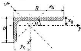
6.14-chizma. Teng yonli bo'lmagan burchak.
