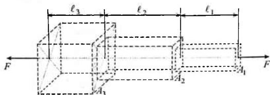
3.17-chizma. Pog'onali prizmatik sterjen
