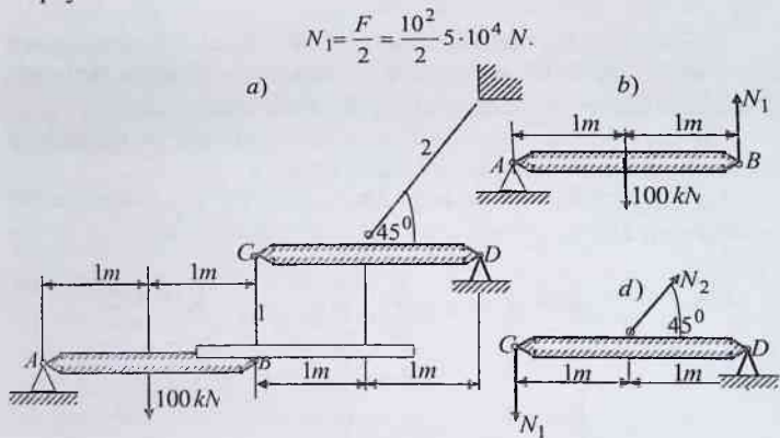
2.22-chizma. Ikkita absolyut qattiq gorizontaal brusli konstruktsiya
