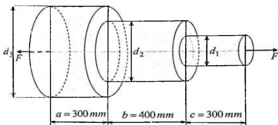
3.18-chizma. Pog'onali silindrik sterjen.
