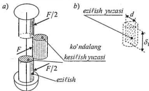
5.6-chizma. Parchin mix va uning ishlovchi yuzalari
