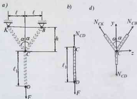
2.31-chizma. Ferra
