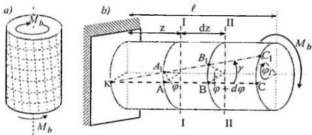
7.3-chizma. To'g'ri o'qli brus
