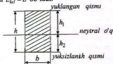
5.10-chizma. To'g'ri to'rtburchakli ko'ndalang kesimi.
