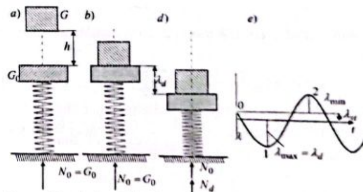
6.6-chizma. Vertikal zarbda dinamik koeffitsientni aniqlash modeli.
