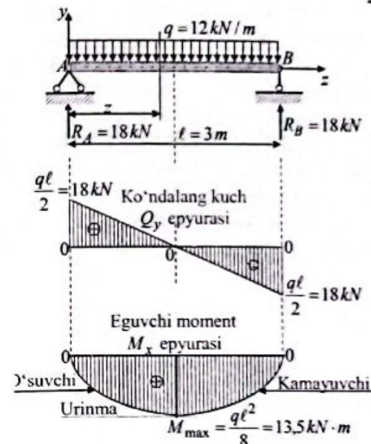
1.17-chizma. Tekis taqsimlangan kuchlar ta'siridagi oddiy to'sin.
