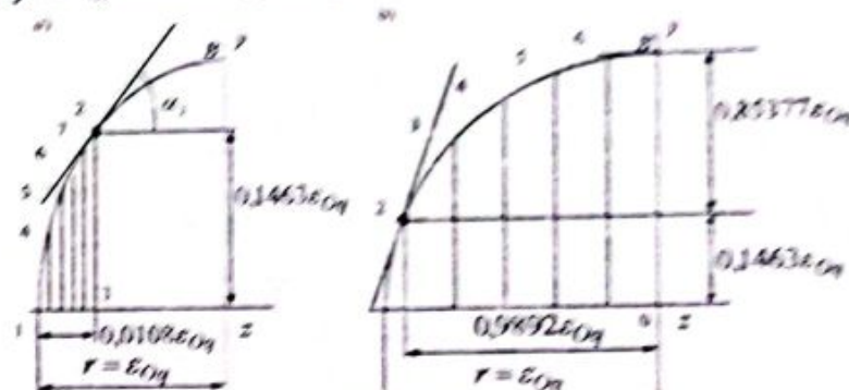
5.15-Silliq o'tish yoylari.
