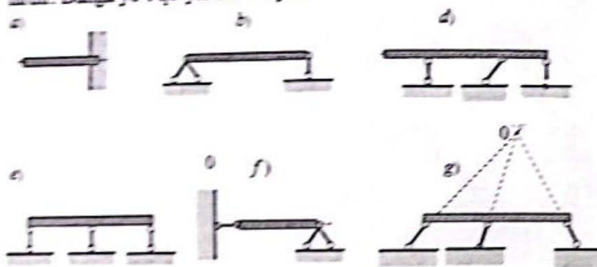
1.6-chizma. To'sinlar hisob sxemasi.
