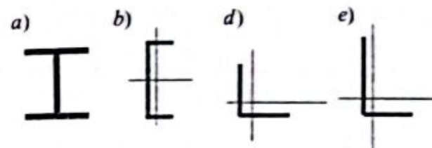
5.18-chizma. Qo'shtavr, shveller, burchak kabi ko'ndalang kesim yuzalari.
