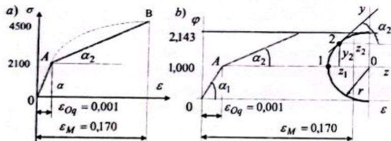
5.14-chizma. Sterjen materialining ikki modulli siqilish diagrammasi.
