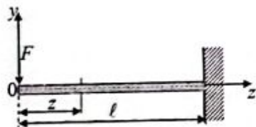
3.3-chizma. To'plangan yuk bilan yuklangan konsol balka.
