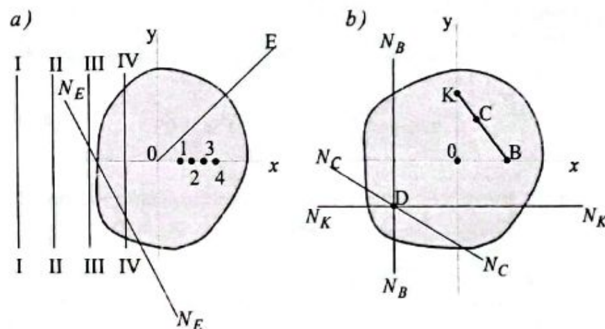
4.19-chizma. Neytral chiziq holatlari.
