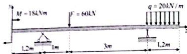
3.26-chizma. Tekis taqsimlangan, to'plangan yuklar va juft kuch bilan yuklangan konsolli to'sin.
