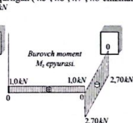
4.6-chizma. Burovchi moment epyurasi.
