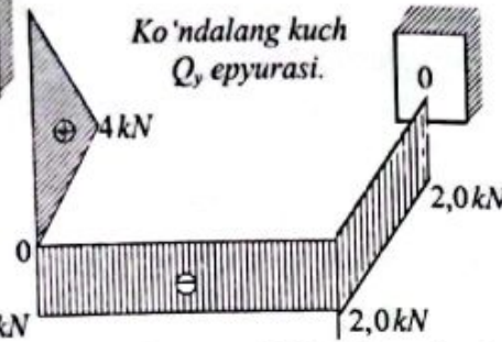
4.8-chizma. Ko'ndalang kuch Q_y epyurasi.
