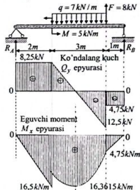
2.16-chizma. To'plangan yuklar bilan yuklangan oddiy to'sin.
