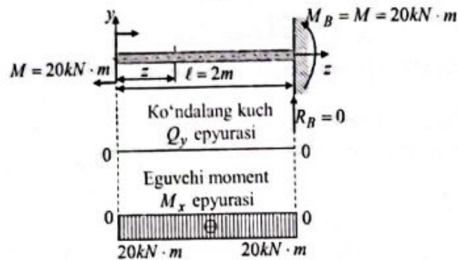
1.13-chizma. Juft kuch bilan yuklangan konsol.
