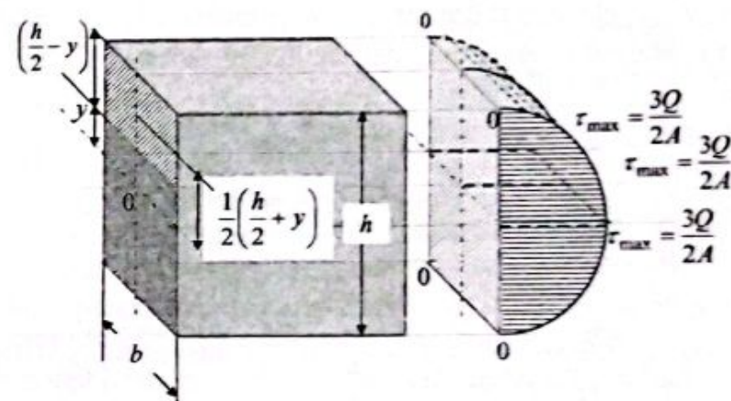
2.7-chizma. To'g'ri to'rtburchakli kesimda urinma kuchlanishlar epyurasi.
