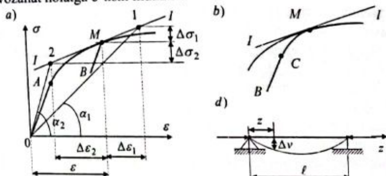
5.12-chizma. Sterjen materiali siqilish diagrammasi.
