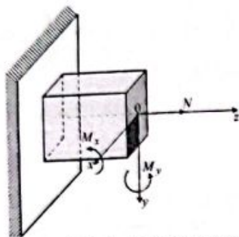
4.3-chizma. Musbat yo'nalishdagi ichki zo'riqish kuch omillari.
