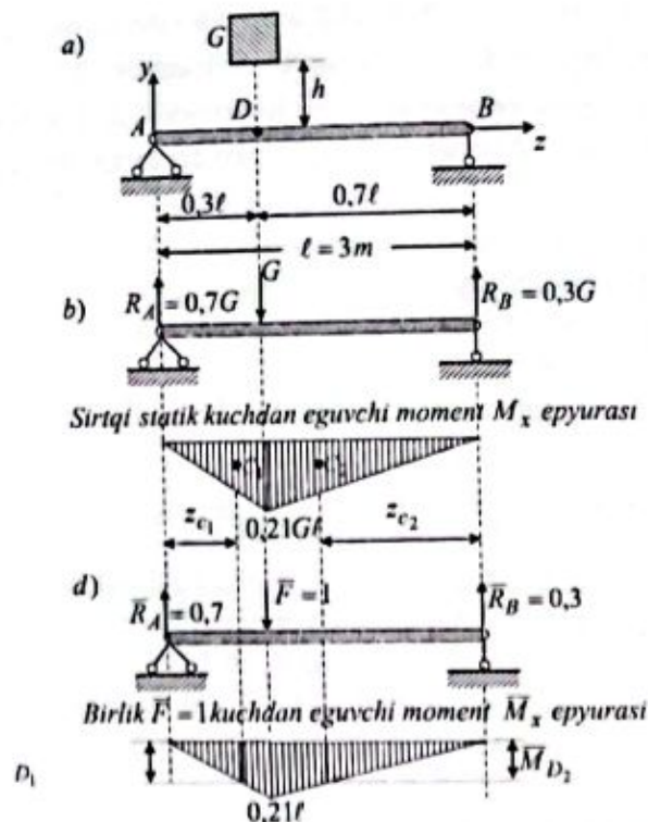
6.14-chizma. Sirtqi va birlik yuklari ta'siridagi to'sin.
