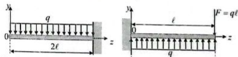
3.18-chizma. Tekis taqsimlangan yuk va to'plangan kuch bilan yuklangan konsollar.
