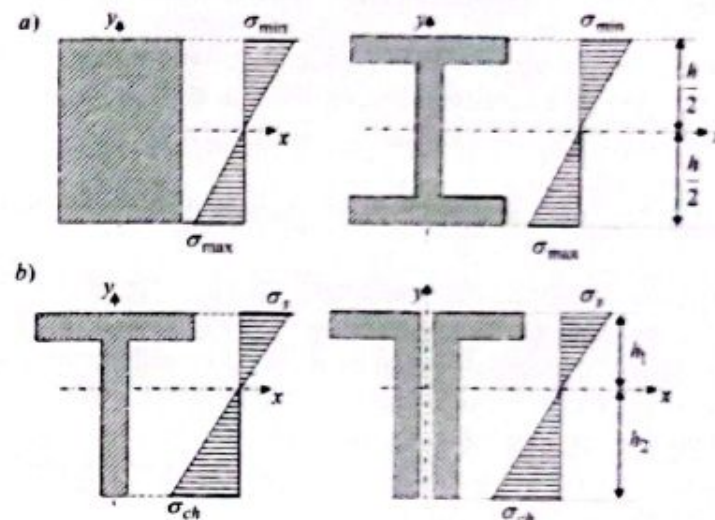
2.4-chizma. Turli shakldagi ko'ndalang kesimlarda normal kuchlanish epyuralari.
