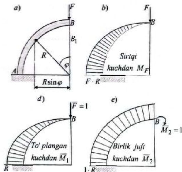
4.11-chizma. Egri chiziqli konsol.
