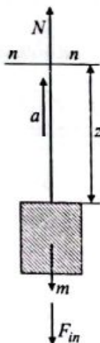
6.9-chizma. Po'lat arqonda yuqoriga ko'tarilayotgan lift kabinasi.
