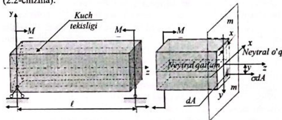
2.2-chizma. To'sindan kesib olingan chap qismi.
