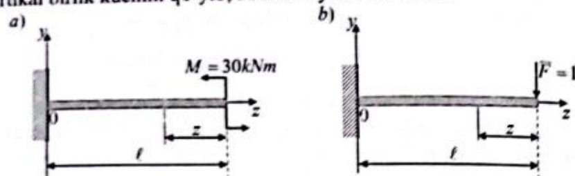
3.8-chizma. To'plangan va birlik yuk bilan yuklangan konsollar.
