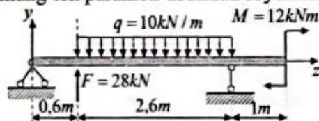
3.20-chizma. To'plangan va juft kuchlar bilan yuklangan konsolli to'sin.
