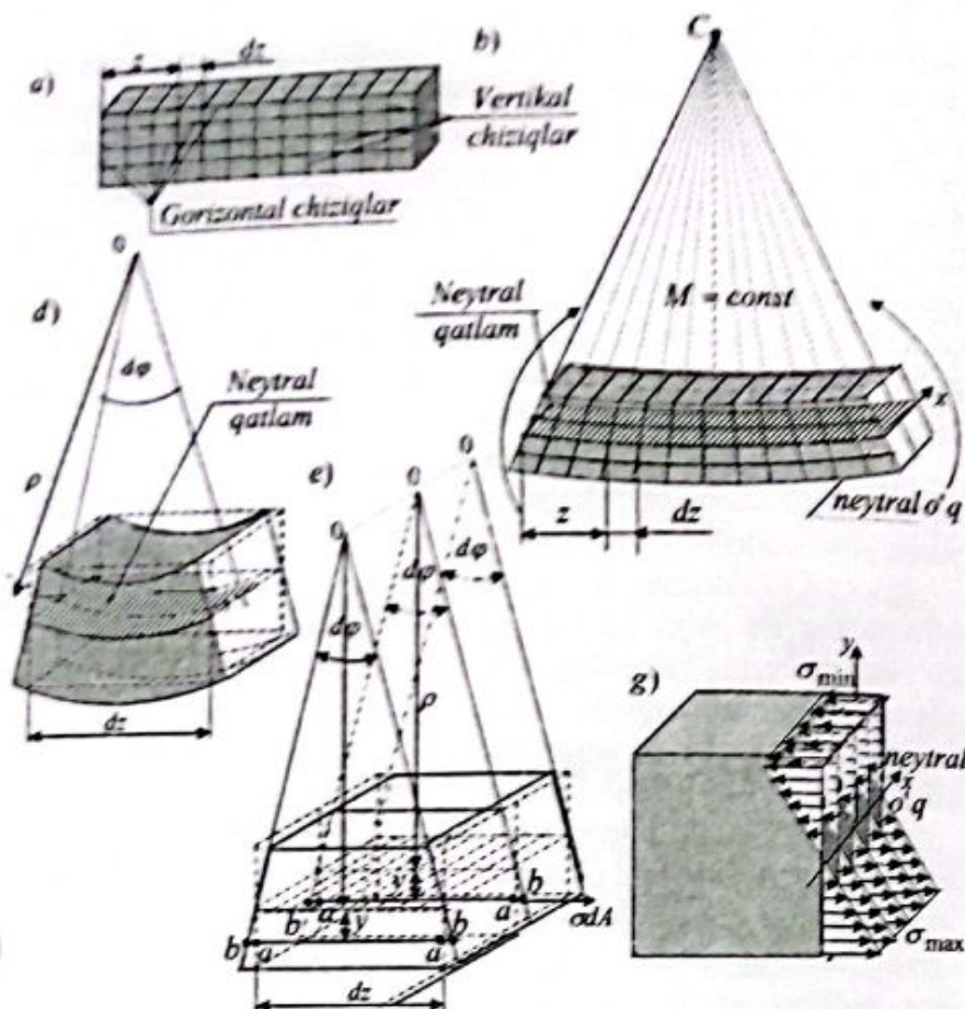
2.3-chizma. To'sinning egilish jarayonidagi va keyingi holati.
