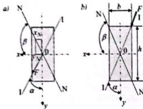
4.12-chizma. Kuchning to'g'ri to'rtburchakli kesim diagonali bo'yicha ta'siri.
