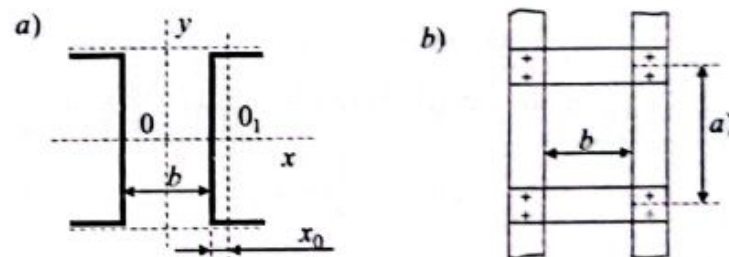
5.19-chizma. Qurama ko'ndalang kesim yuzasi.
