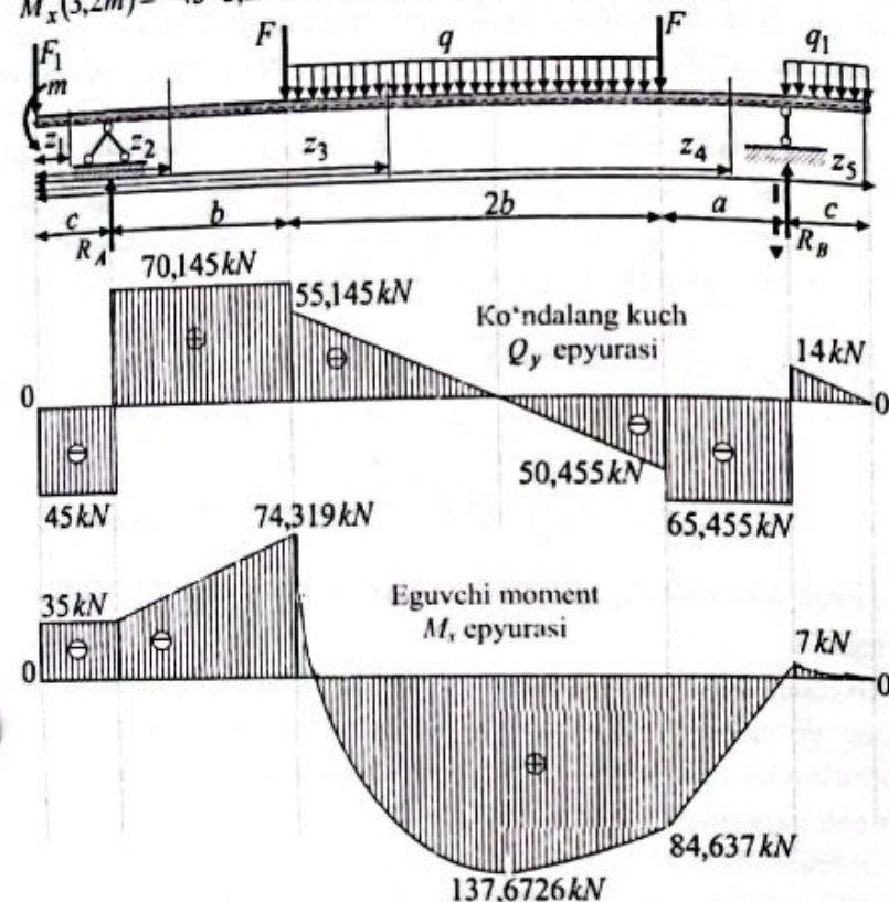
1.20-chizma. Ko'ndalang kuch va eguvchi moment epyuralari.
