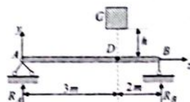
6.19-chizma. ko'ndalang kesimi № 14 qo'shtavr shaklidagi oddiy to'sin.
