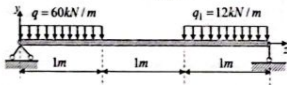
3.21-chizma. Tekis taqsimlangan yuk bilan yuklangan konsolli to'sin.
