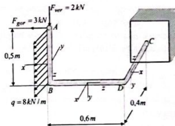
4.4-chizma. Siniq o'qli brus.
