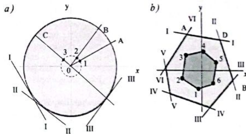
4.20-chizma. Ustu ko'ndalang kesim yuzalari.
