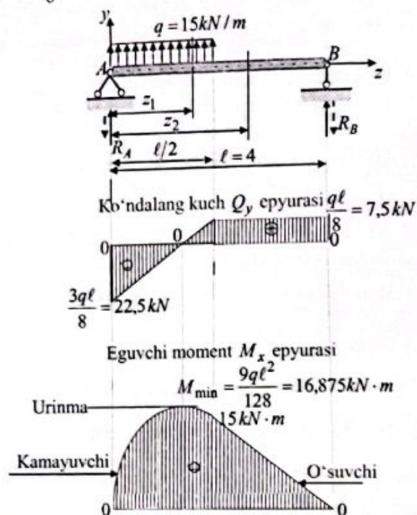
1.18-chizma. Tekis taqsimlangan kuchlar ta'siridagi oddiy to'sin
