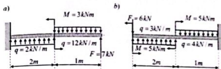
2.18-chizma. Tekis taqsimlangan, to'plangan va juft kuchlar bilan yuklangan konsollar
