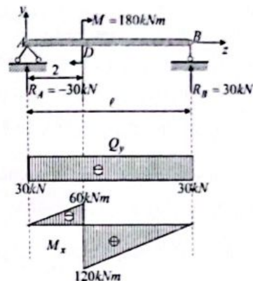
3.17-chizma. Juft kuchi bilan yuklangan oddiy to'sin.
