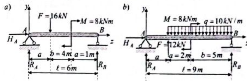
1.8-chizma. Tashqi kuchlar ta'siridagi oddiy to'sin.
