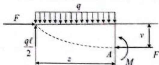
5.21-chizma. Bo'ylama va ko'ndalang kuch ta'siridagi element muvozanati.
