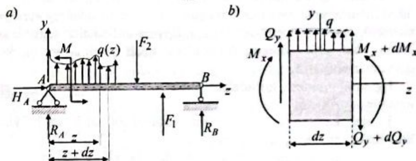
1.10-chizma. To'sindan ajratib olingan kichik element.
