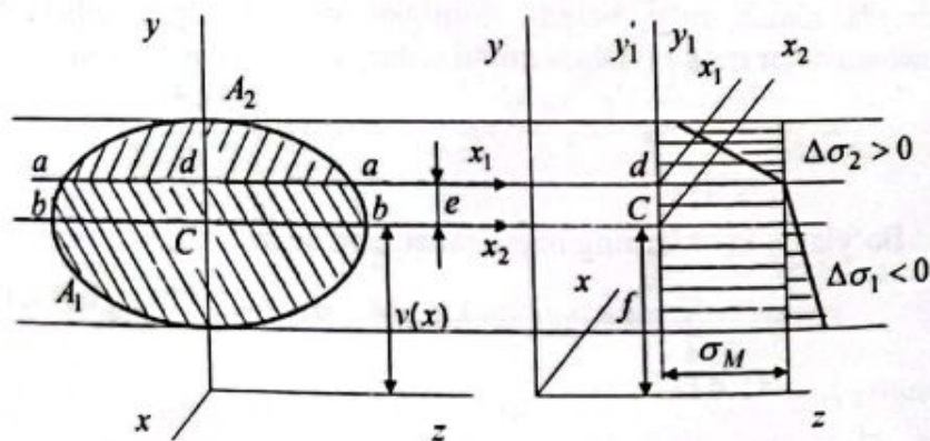
5.9-chizma. Sterjenning ko'ndalang kesim yuzasi.
