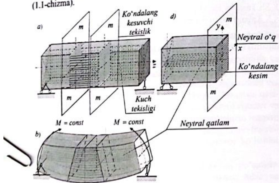
1.1-chizma. Tashqi kuchlar ta'sirida to'sinning egilishi.
