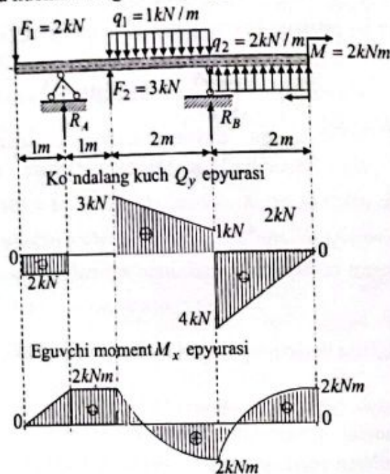
2.17-chizma. To'plangan yuklar ta'siridagi ikki konsolli to'sin.
