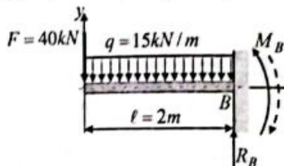
1.19-chizma. Tekis taqsimlangan yuk ta'siridagi konsol.
