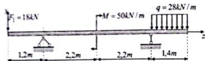
3.27-chizma. Tekis taqsimlangan yuk va to'plangan yuklar bilan yuklangan konsolli to'sin.
