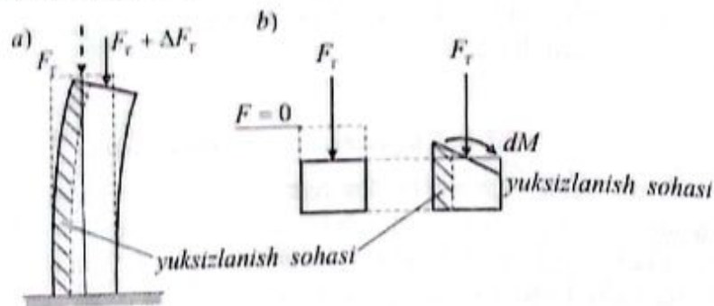
5.11-chizma. Siqilgan sterjen yüksizlanish sohasi.
