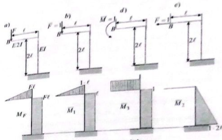
3.14-chizma. Siniq o'qli brus.
