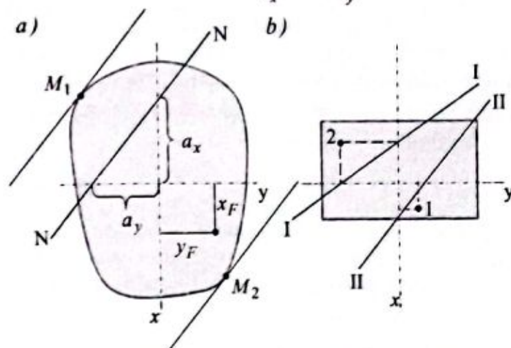
4.18-chizma. Ustunning ko'ndalang kesim yuzasi.
