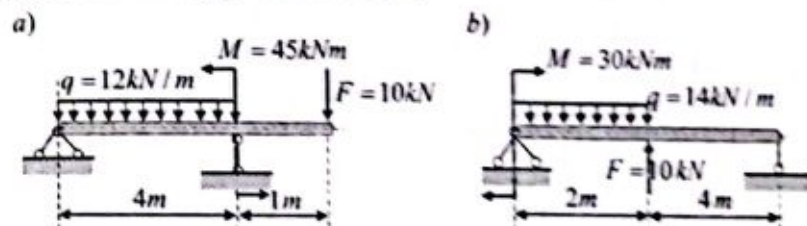
2.19-chizma. Tekis taqsimlangan, to'plangan va juft kuchlar bilan yuklangan to'sinlar.
