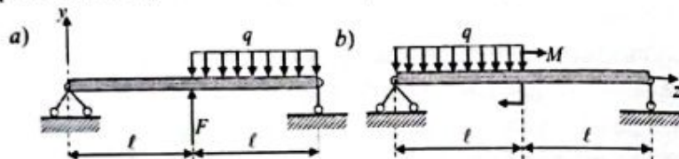
3.19-chizma. Tekis taqsimlangan yuk va to'plangan kuch va juft kuchlar bilan yuklangan to'sinlar.
