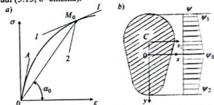
5.13-chizma. Sterjen materialining ikki modulli siqilish diagrammasi.
