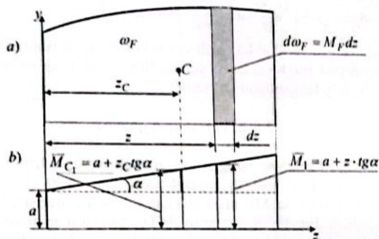
3.12-chizma. Sirtqi va birlik kuchlar epyuralari.
