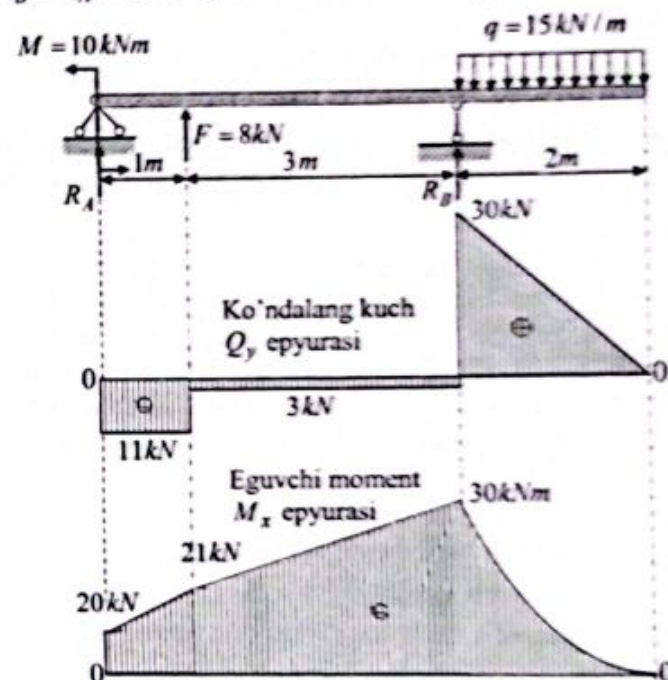
2.14-chizma. To'plangan yuklar bilan yuklangan konsolli to'sin.
