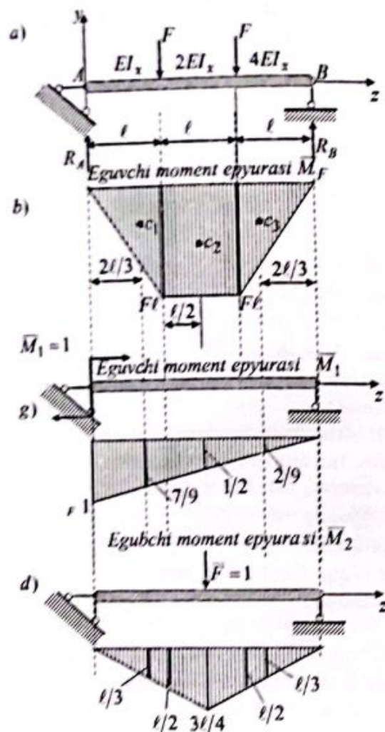
3.16-chizma. Bikirligi o'zgaruvchi to'sin.
