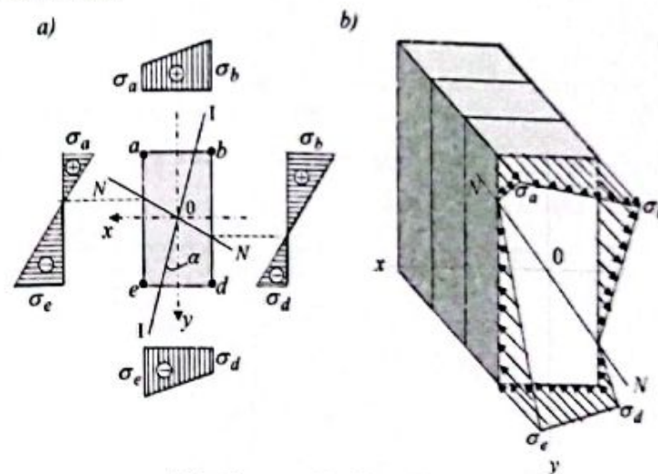
4.13-chizma. Kuchlanish epyurasi.
