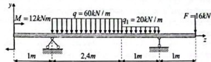
3.25-chizma. Tekis taqsimlangan, to'plangan yuk va juft kuch bilan yuklangan konsolli to'sin.
