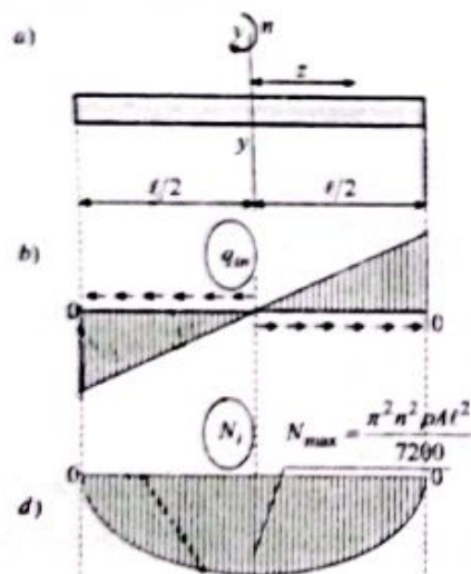
6.11-chizma. Vertikal o'q atrofida aylanayotgan gorizontal sterjen.
