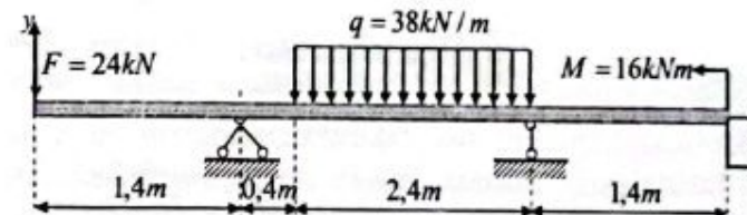
3.24-chizma. Tekis taqsimlangan, to'plangan yuklar va juft kuch bilan yuklangan konsolli to'sin.
