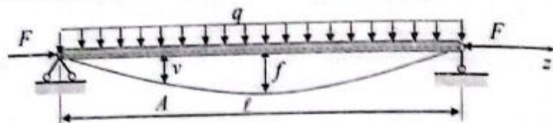
5.20-chizma. Siquvchi bo'ylama kuchi bilan ko'ndalang kuchning sterjenga ta'siri.
