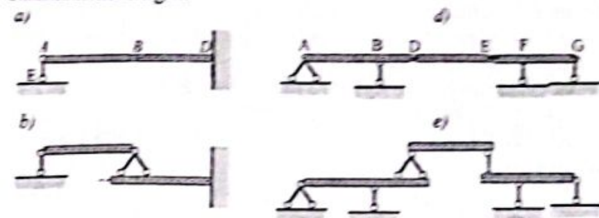
1.7-chizma. Ko'p oraliqli sharnirli to'sinlar.
