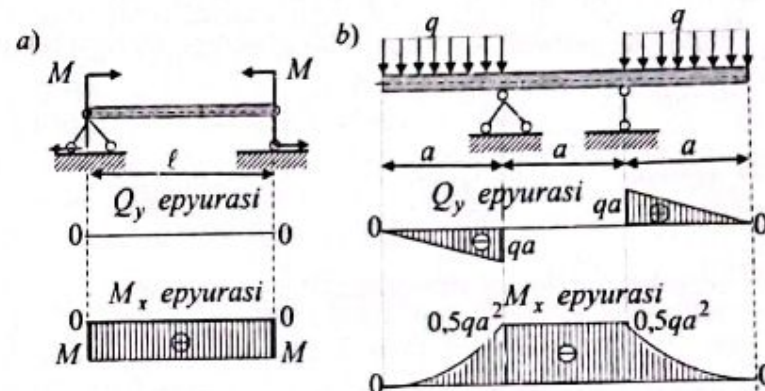
2.1-chizma. Sof egilishdagi to'sinlar.
