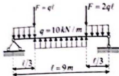
1.21-chizma. Tekis taqsimlangan yuk va to'plangan kuchlar bilan yuklangan oddiy to'sin.
