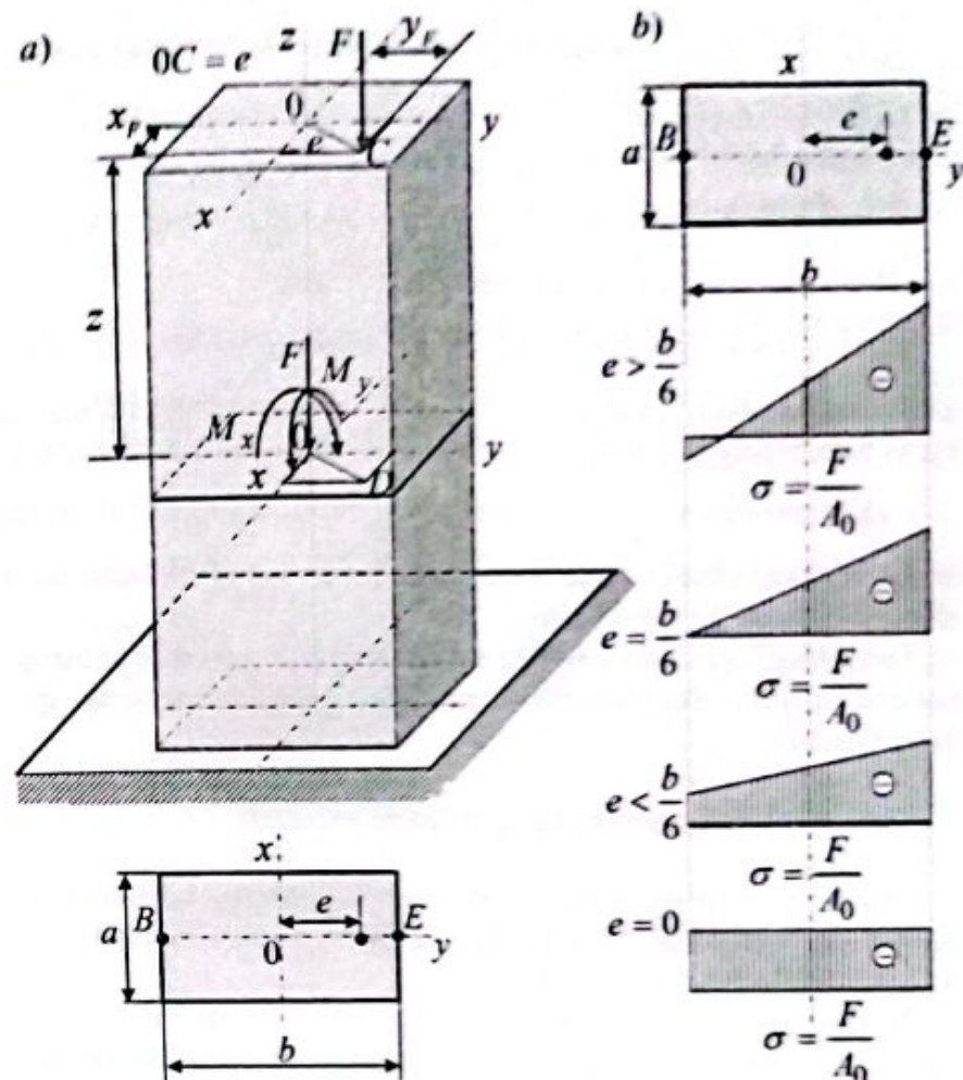
4.17-chizma. Ko'ndalang kesimi to'g'ri to'rtburchakli siqilgan ustun.
