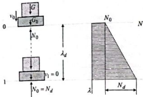
6.7-chizma. Zarbdan keyin bajarilgan ishni hisoblash uchun sxema.
