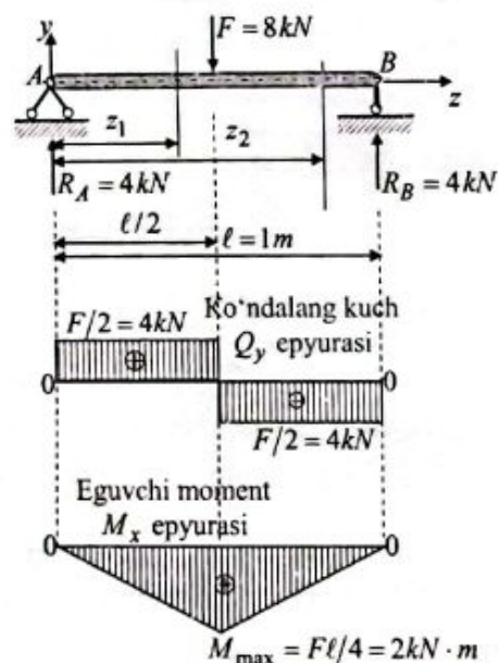
1.15-chizma. To'plangan kuch ta'siridagi oddiy to'sin.
