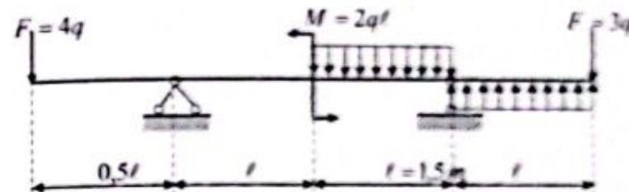
2.25-chizma. To'plangan kuch va juft kuchlar bilan yuklangan konsolli to'sin.
