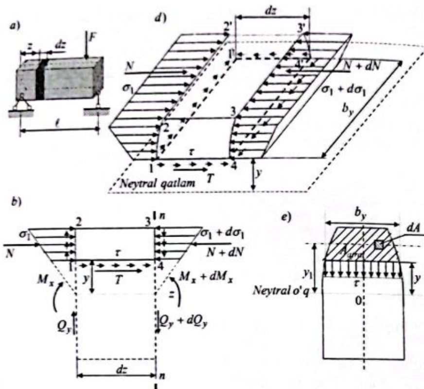
2.6-chizma. Ajratilgan ko'ndalang kesimlardagi kuchlanishlarning taqsimlanishi.
