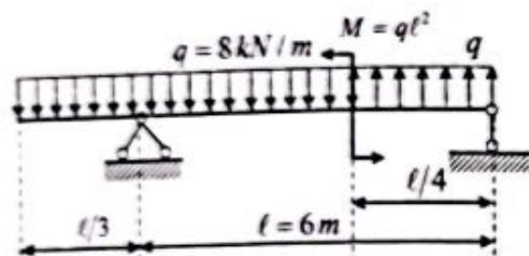
1.22-chizma. Tekis taqsimlangan yuk va juft kuchlar bilan yuklangan konsolli to'sin.
