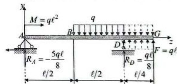
3.7-chizma. Konsolli to'sin.
