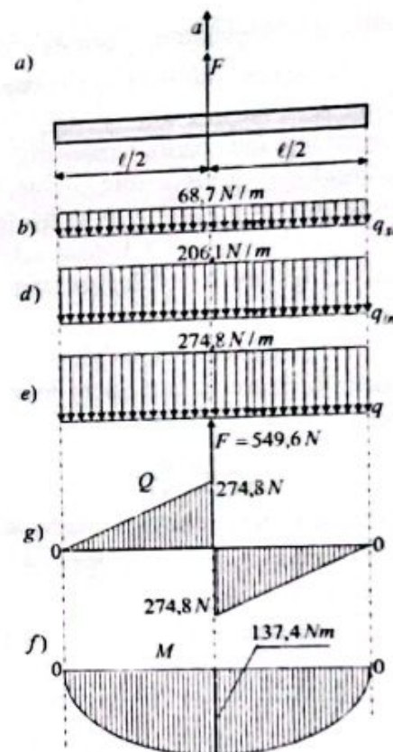
6.10-chizma. O'zgarmas tezlanish bilan ko'tarilayotgan gorizonta to'sin.
