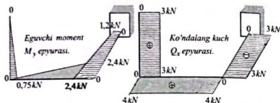
4.9-chizma. Eguvchi moment epyurasi.
