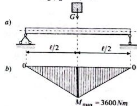
6.13-chizma. Zarb yuk ta'sirdagi oddiy to'sin.
