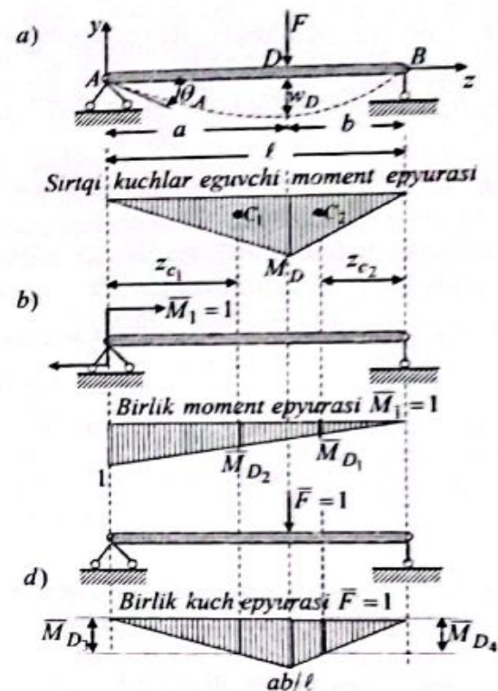
3.13-chizma. Birlik kuch juft kuch, to'plangan birlik kuch va sirtqi kuchlar epyuralari.
