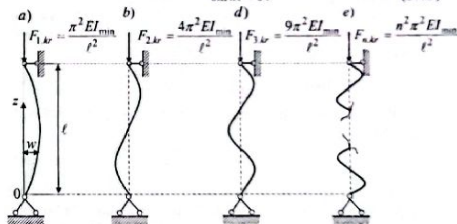
5.5-chizma. Sterjenning turli kritik kuchlarga mos keluvchi muvozanat holatlari
