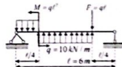
2.26-chizma. Tekis taqsimlangan yuk, to'plangan kuch va juft kuchlar bilan yuklangan oddiy to'sin.
