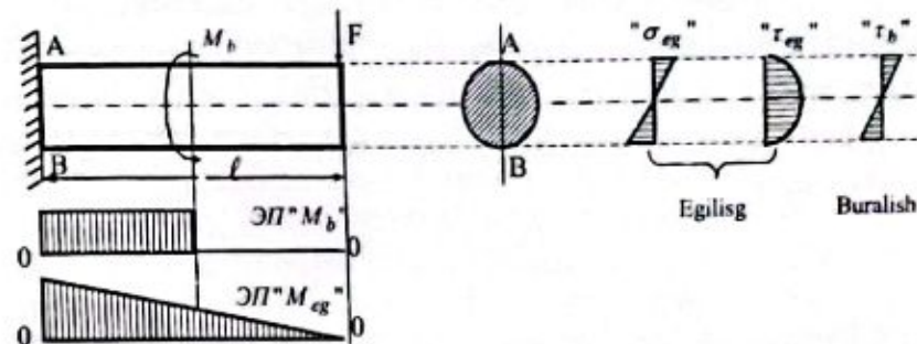
4.24-chizma. Egilish bilan buralishning birgalikdagi ta'siri.
