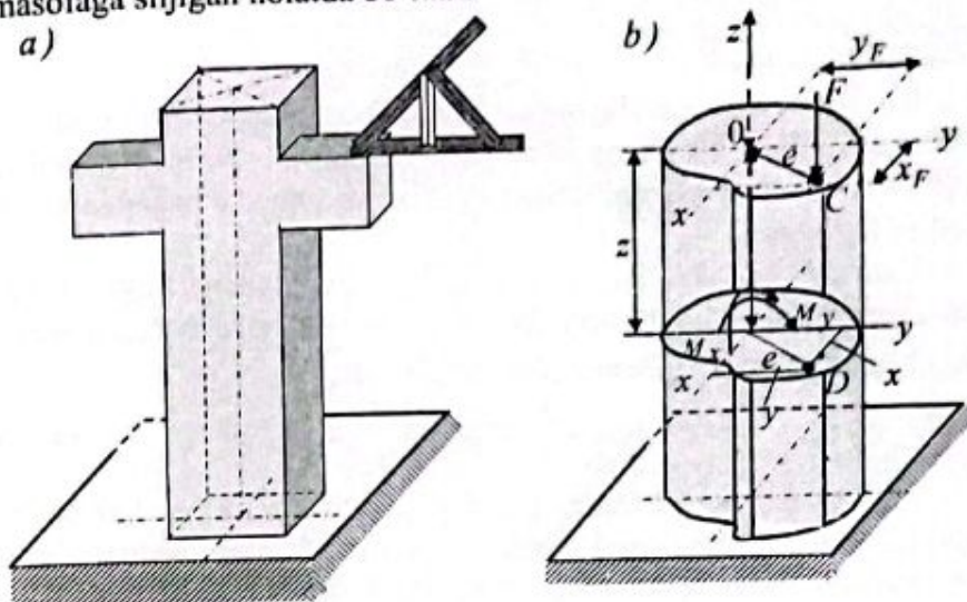
4.16-chizma. Nomarkaziy siqilgan ustunlar.
