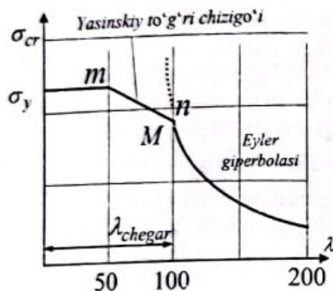
5.7-chizma. Kritik kuchlanish bilan egiluvchanlik orasidagi bog'lanish grafigi.
