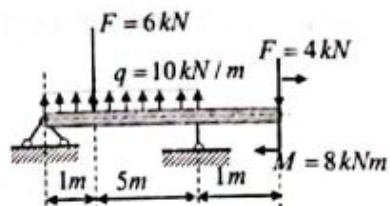
2.20-chizma. Tekis taqsimlangan va to'plangan kuchlar bilan yuklangan to'sin.
