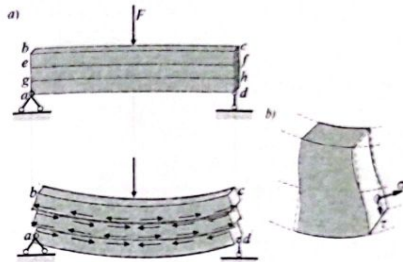
2.5-chizma. Urinma kuchlanishlarning kesimlar bo'yicha taqsimlanishi.
