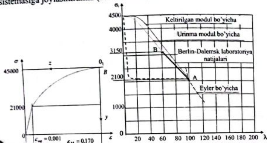
5.16-chizma. Sterjen material siqilish diagrammasi va qurilish po'lati uchun kritik kuchlanish bilan egiluvchanlikka o'rtasidagi grafik.
