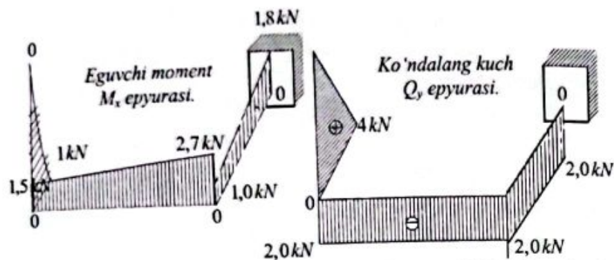
4.8-chizma. Ko'ndalang kuch Q_y epyurasi.
