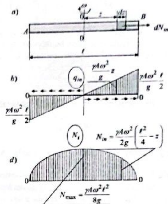
6.4-chizma. \omega burchak tezligi bilan aylayotgan to'sin.
