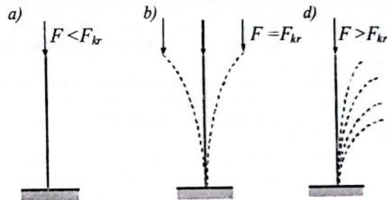
5.2-chizma. To'g'ri o'qli siqilgan ingichka sterjenning muvozanat holati.
