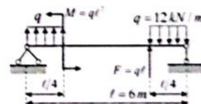
2.27-chizma. Tekis taqsimlangan yuk, to'plangan kuch va juft kuchlar bilan yuklangan oddiy to'sin.
