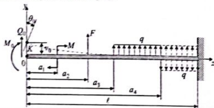
3.6-chizma. Elastik chiziq tenglamasini keltirib chiqarish uchun yuklangan to'sin.
