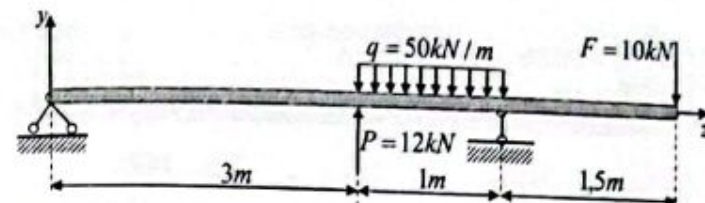
3.22-chizma. Tekis taqsimlangan va to'plangan yuklar bilan yuklangan konsolli to'sin.
