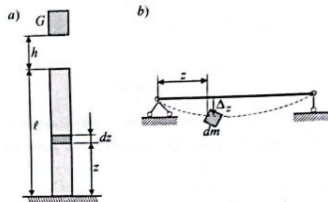
6.8-chizma. Bo'ylama va ko'ndalang zarb.
