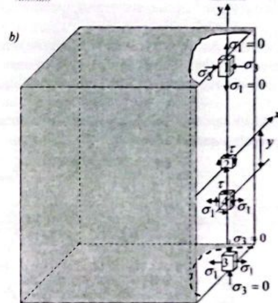
2.10- chizma. To'sin turli qatlamlaridagi elementlar.
