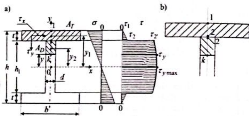
2.8-chizma. Qo'shtavr kesimda urinma kuchlanishlar epyurasi.
