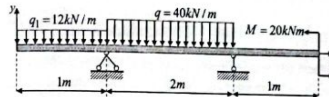
3.23-chizma. Tekis taqsimlangan yuk va juft kuch bilan yuklangan konsolli to'sin.
