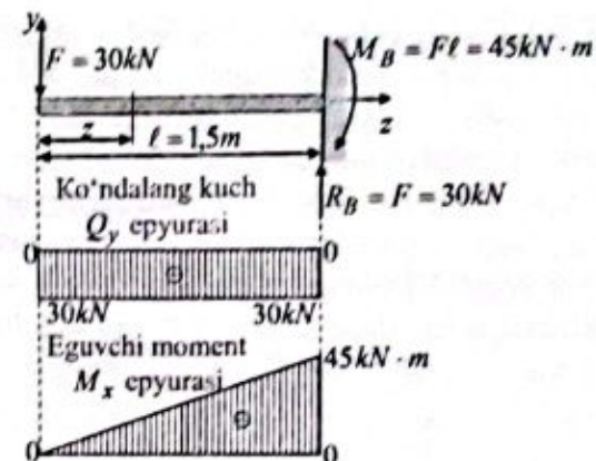
1.12-chizma. To'plangan kuch ta'siridagi konsol.
