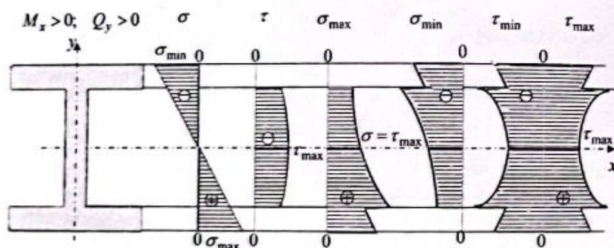
2.11-chizma. Qo'shtavr kesimdagi kuchlanishlar epyuralari.
