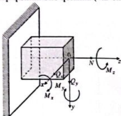
4.2-chizma. Ichki zo'riqish kuch omillari yo'nalishlari.
