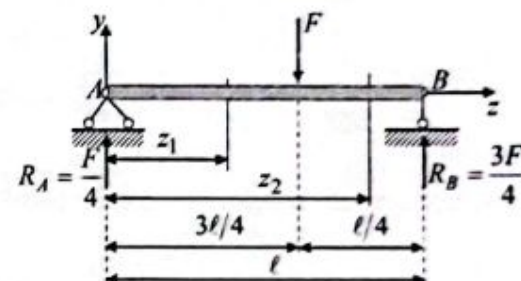
3.5-chizma. To'plangan yu'k bilan yuklangan oddiy to'sin.
