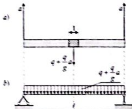
6.16-chizma. O'zgaras tezlanish bilan ko'tarilayotgan to'sin.
