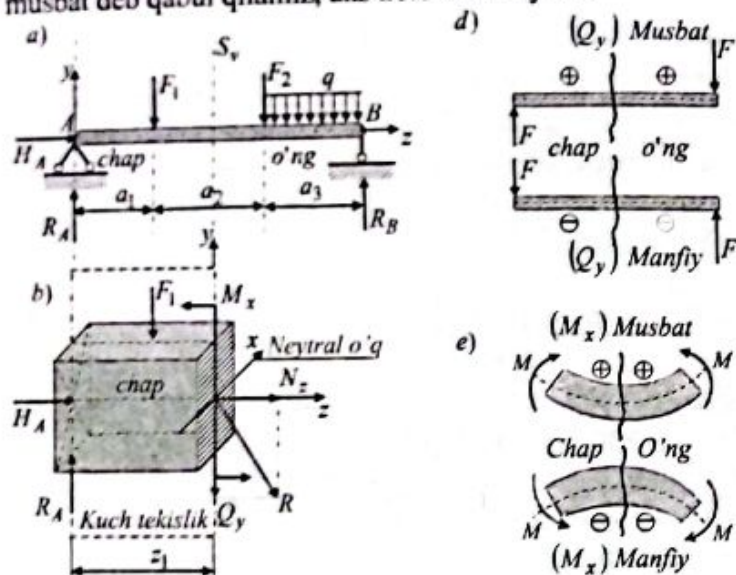
1.9-chizma. Muvozanatdagi oddiy to'sin.
