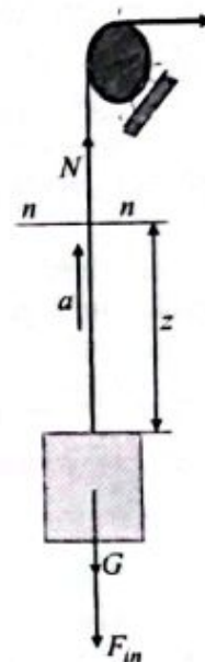
6.2-chizma. Yuqoriga a tezlanish bilan ko'tarilayotgan yuk.
