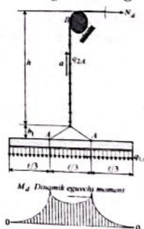
6.3-chizma. Tezlanish bilan ko'tarilayotgan to'sin.
