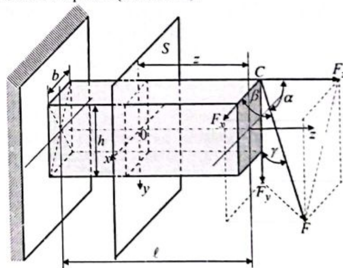
4.1.-chizma. Bir uchi qistirib mahkamlangan, erkin uchiga qo'yilgan to'plangan kuch ta'siridagi brus.
