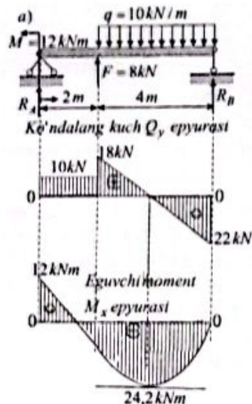
2.12-chizma. To'plangan va tekis taqsimlangan yuklar bilan yuklangan oddiy to'sin.
