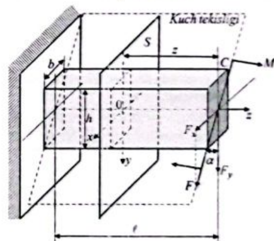
4.11-chizma. Konsol to'sinning ko'ndalang qiyshiq egilishi
