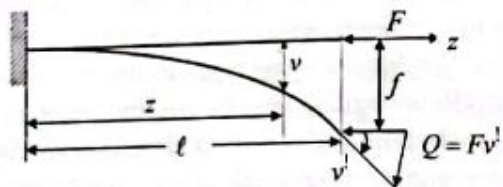
5.3-chizma. Bir uchi qistirib mahkamlangan erkin uchi bilan siqilgan sterjenning muvozanat holati.
