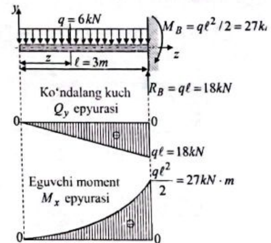
1.14-chizma. Tekis taqsimlangan kuch ta'siridagi konsol.
