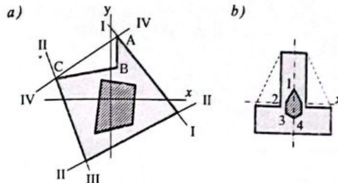
4.21-chizma. Tavr va ichki burchakli ko'pburchak.
