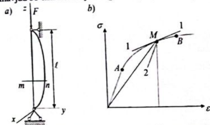
5.8-chizma. Sterjen materialining siqilish diagrammasi.
