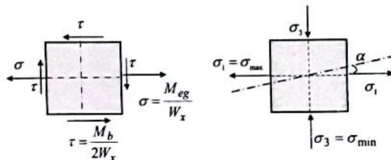
4.24-chizma. Egilish bilan buralishning birgalikdagi ta'siri.
