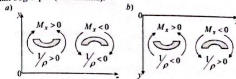
3.2-chizma. Egrilik ishorasi bilan eguvchi moment ishorasi orasidagi bog'lanish.
