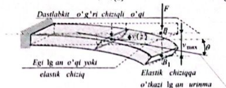
3.1-chizma. Bir uchi bilan qistirib mahkamlangan erkin uchiga qo'yilgan to'plangan kuchdan to'sin egilgan o'qi.
