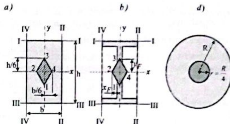
4.23-chizma. To'g'ri turtburchak, qo'shtavr va doira shaklidagi kesimlar.
