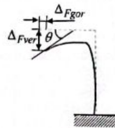
3.15-chizma. Siniq o'qli sterjenning deformatsiyalangan holati.
