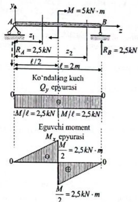
1.16-chizma. To'plangan juft kuch ta'siridagi oddiy to'sin.
