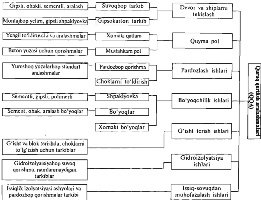
11.7-rasm. Ishlatilishiga ko'ra QQA lar tasnif.
