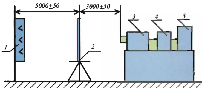
9.20-rasm. Oynataxtalarning optik xossalarini aniqlash yig'ilmasining sxemasi
