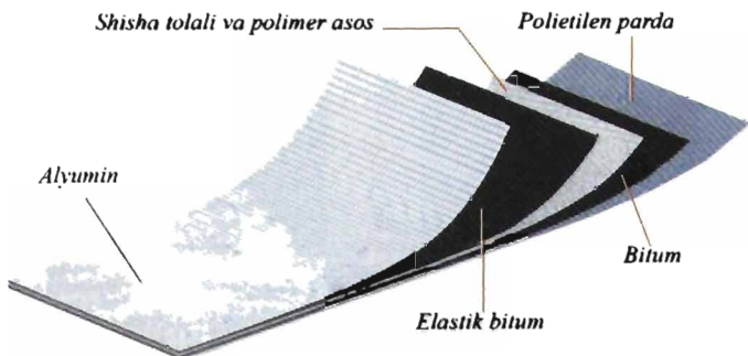
3.12-rasm. «Poliester» tombob besh qatlamli o'rama membranası.
