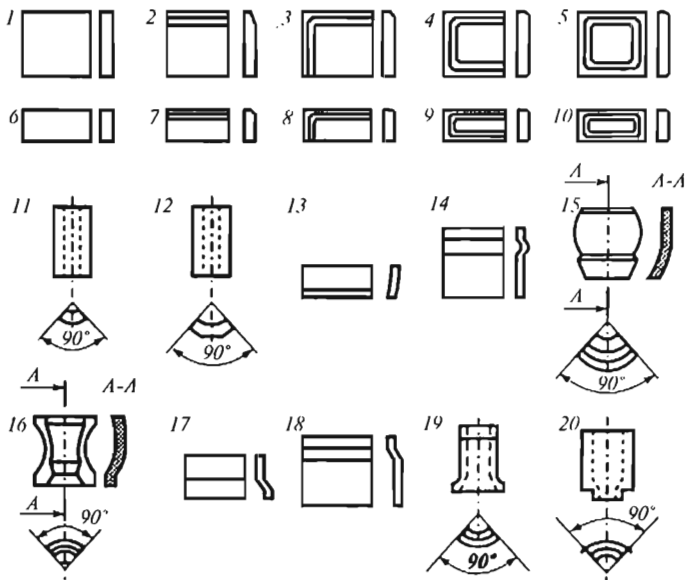
8.11-rasm. Yuzasi glazur bilan sirlangan sopol buyumlarining xillari: 1-5 – kvadratlil; 6-10 – to'rtburchakli; 11,12 – shakldor burchakbop; 13-16 – murakkab shaklli (karnizbop); 17-20 – shakldor chaspak (plintusbop).
