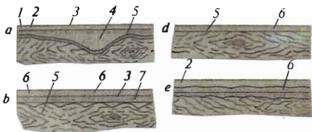
6.25-rasm. Yog'ochni bezaksiz pardoqlash qoplamasining tuzilishi:
