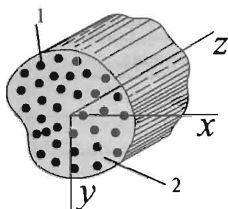
4.7-rasm. Monotrop kompozit kesimi: 1 – pishiqlikni ta'minlovchi armaturasimon qism; 2 – matritsa.
