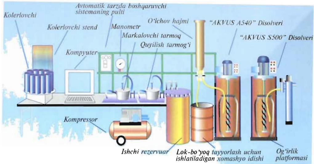
5.1-rasm. Lok-bo'yoq ishlab chiqaradigan kichik zavodning texnologik sxemasi.
