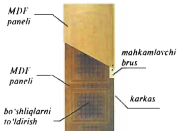
6.19-rasm. MDF dan ishlangan turli eshiklar va ularning tuzilishi.
