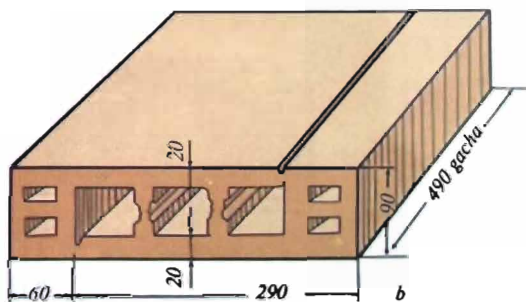
8.8-rasm. Fasadbop qoplama sopol plitkalar: a—kichik o'lchamli plitkalar; b—yirik sopol plitka.
