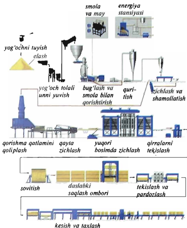
6.18-rasm. MDF ishlab chiqarishning texnologik jarayoni.
