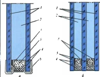
9.9-rasm. Energiyatejamkor metallplastik deraza romlar va ulardagi oyna qatlamlarni o'zaro bog'lash sxemasi:
