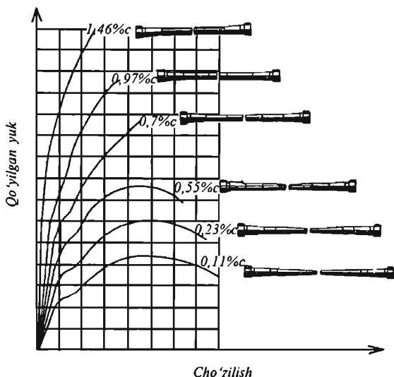
13.3-rasm. Po'lat tarkibidagi uglerodning miqdoriga ko'ra cho'zilishga mustahkamlik diagrammasi.
