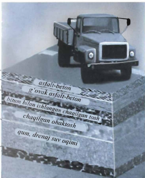
3.3- rasm. 1 va 2- tofadagi magistral asfalt-beton yo'l qatlamlar sxemasi.
