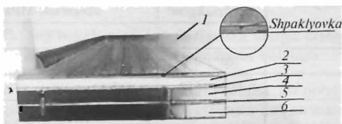
6.11-rasm. Parket polning kesimi:
