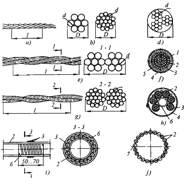
13.5-rasm. Oldindan taranglangan konstruksiyalar uchun arqonsimon to'qima armaturalar: a-7 ta simli; b-19 ta simli; d va e-2 ta arqonli kanatlar; f-3 ta arqonli kanat; g va h-sochilgan armaturali to'qimalar; i va j-ko'p arqonli to'qima kanatlar. 1-o'qdagi armatura; 2-ishchi simlar; 3-to'qima arqonlar; 4- va 5-tashqi muhofaza qatlami; 6-spiral; 7-korotish.
