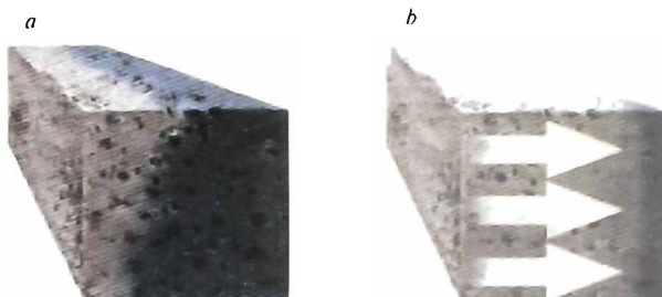
3.14-rasm. Nam betonni penetron eritmasi bilan mo'yqalamda (a) yoki shimdirish usuli bilan (b) izolyatsiya qilish.
