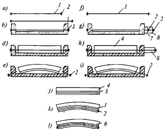
12.15-rasm. Armaturalarni oldindan taranglash usullari:
