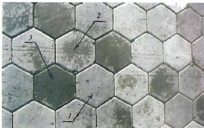
15.2-rasm. Suvning shimilish tezligi orqali qoplama beton toshlarni navlarga bo'lish: 1—eng sara yuqori sifatli; 1-nav qoplama tosh; 2—sifati o'rtacha 2-navli tosh; 3—sifatsiz 3-navli qoplama tosh.
