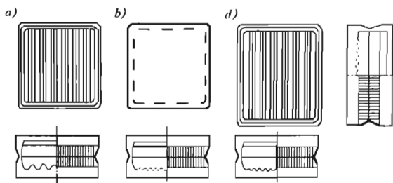
9.13-rasm. Shisha blok turlari:
