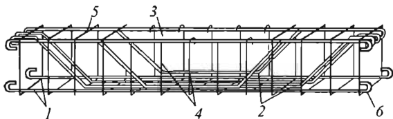
12.14-rasm. Temirbeton to'sinbop armatura karkas:
