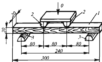
6.30-rasm. Yog'och namunani statik egilishga sinash sxemasi: 1 – namuna; 2 – kuch tushuvchi yuza; 3 – tayanchlar.
