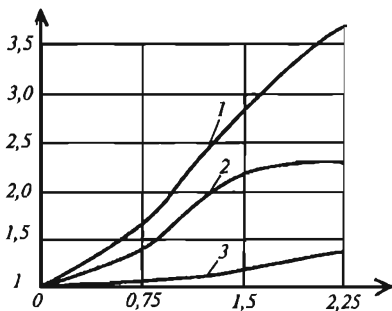
12.7-rasm. Beton mustahkamligiga tola shaklining bog'liqlik grafiqi:
