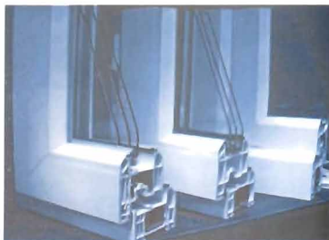
9.9-rasm. Energiyatejamkor metallplastik deraza romlar va ulardagi oyna qatlamlarni o'zaro bog'lash sxemasi:
