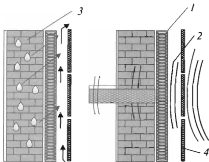
8.15-rasm. «Nafas oluvchi» devor kesimining sxemasi:
