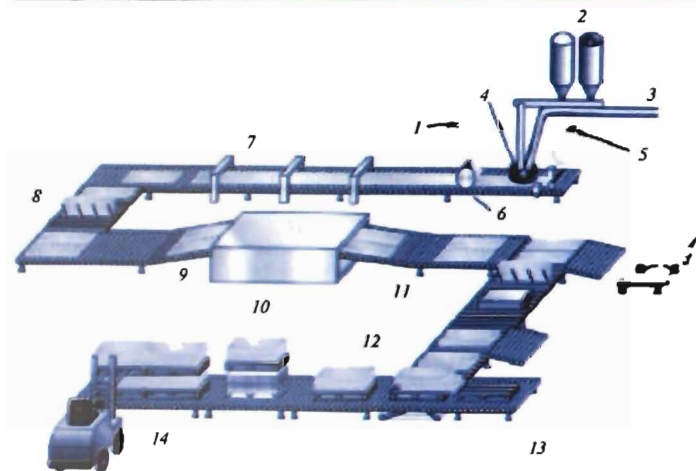
10.2 -rasm. Gips-karton ishlab chiqarish korxonasi va mahsulot tayyorlashning texnologik jarayonlar sxemasi:
