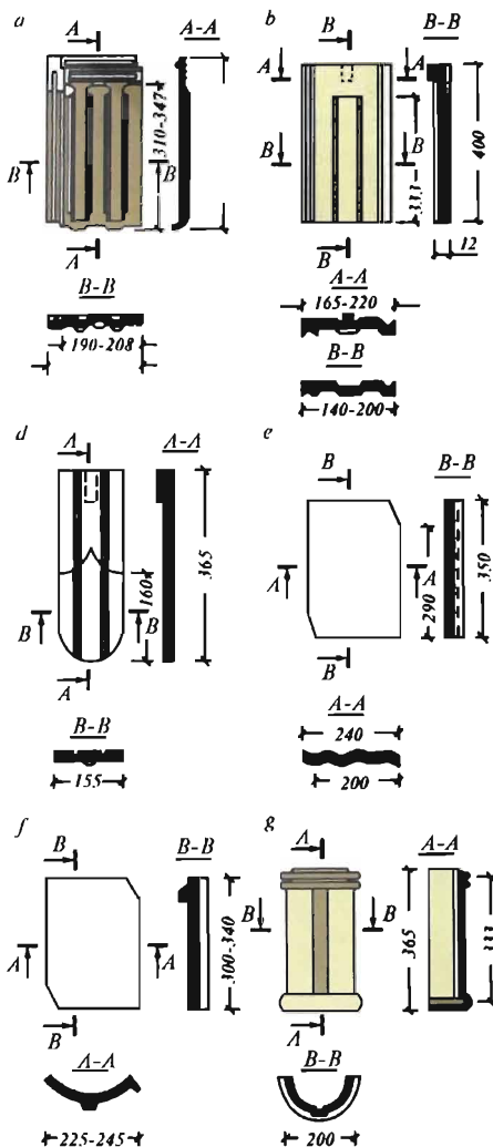
8.13-rasm. Tombop rangli sopol cherepitsa: a—ariqcha o'yiqli; b—ariqchali; d—tekis; e—to'lqinli; f—shaklli; g—yarimdoirali.
