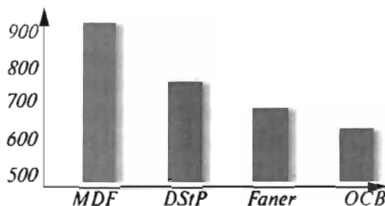
6.20-rasm. MDFni egilishga bo'lgan mustahkamligini taqqoslash diagrammasi, \text{n/mm}^2 .
