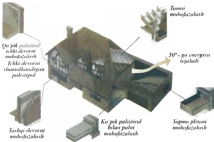
4.3-rasm. Issiqlikni kam o'tkazadigan ko'pik polistirolning bino qismlarida ishlatilishi.
