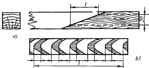
6.29-rasm. Yog'ochning yillik halqalari soni bilan kech yetilgan yoz yog'ochligi miqdorini aniqlash.
