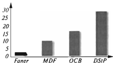
6.17-rasm. MDF ni 24 soat nam ta'sirida shishish ko'rsatkichiga ko'ra taqqoslash, % da.
