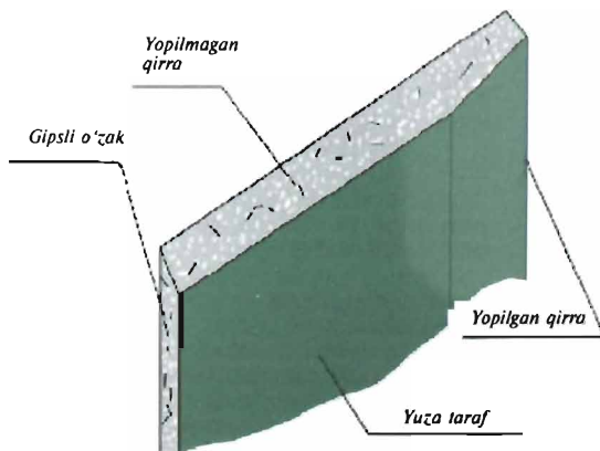
10.4-rasm. KNAUF gips-karton qoplamaning tuzilishi.
