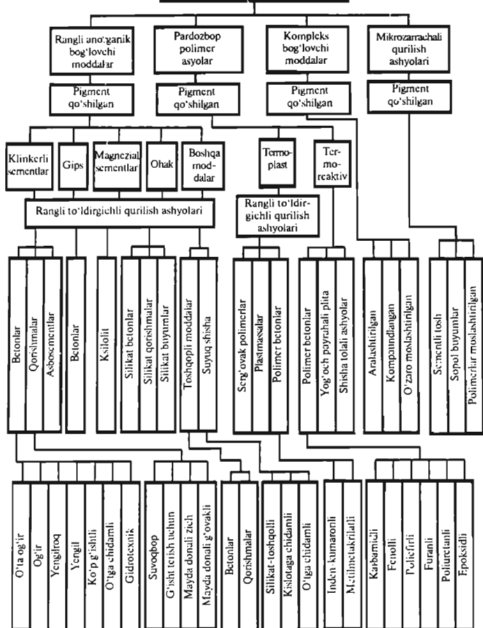
2.1-rasm. Pardozbop arxitekturaviy qurilish ashyolarining tsnifi.
