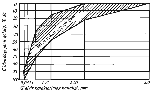
12.1.-rasm. Qumni beton yoki qorishma uchun yaroqli ekanligini uning mayda-yirikligiga qarab aniqlash grafigi.
