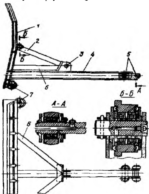
4.11-rasm. DZ-20V skreperining ketingi devori:
