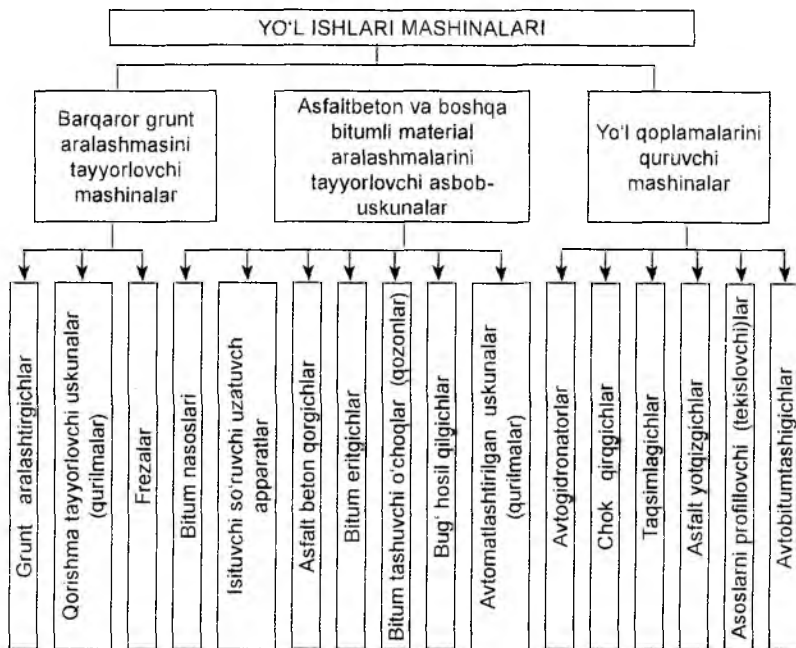
3.23-rasm. Yo'l ishlari mashinalari klassifikatsiyasi
