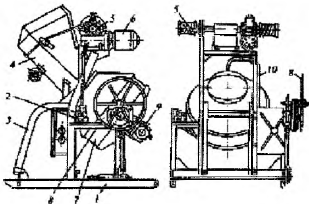
4.46-rasm. Qo'zg'aluvchan gravitatsion beton qorgichning chizmasi.
