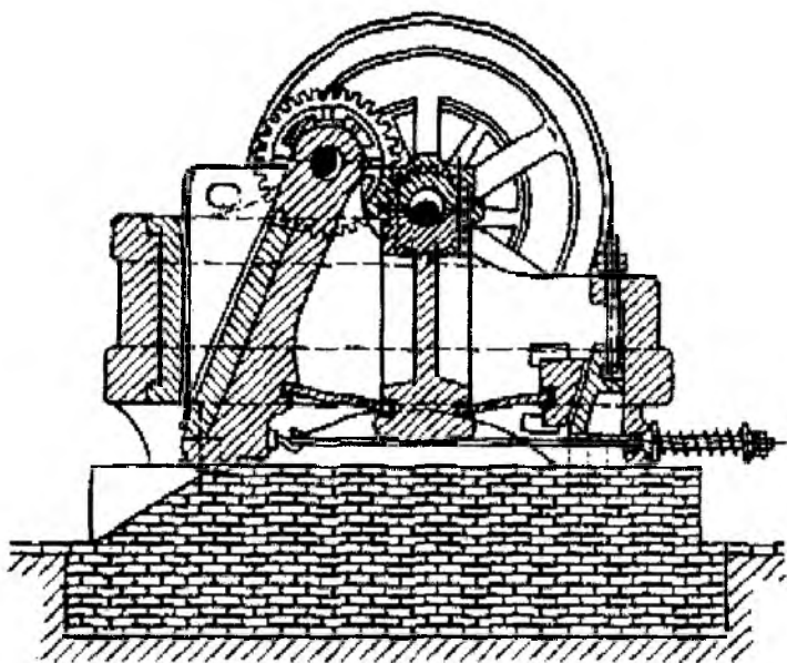
3.11-rasm. Rossiyada birinchi marta ishlab chiqilgan bug' mashina bilan harakatlanuvchi jag'li tosh maydalagich
