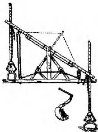
3.13-rasm. Yer qazuvchi mashinaning muvozanatlashgan greyferli mexanizmi (1724-y.).
