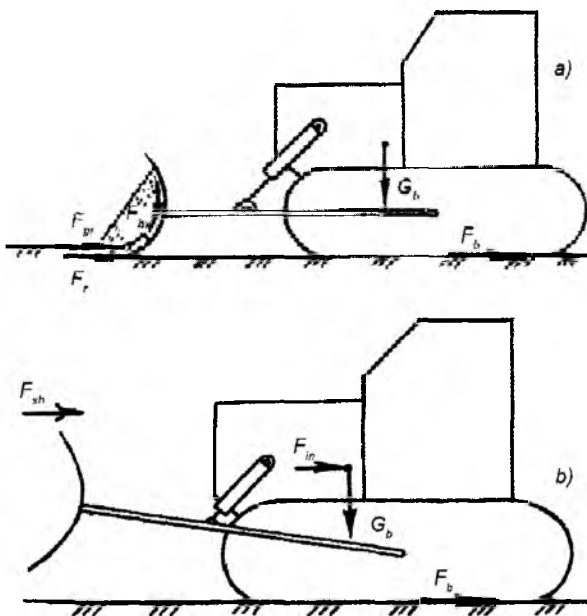
4.7-rasm. Buldozerga ta'sir etuvchi kuchlar tasviri: a) tuproq kesish jarayonida; b) yuruvchi (transport) holatida.
