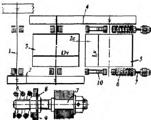
4.43-rasm. Valikli tosh maydalagich chizmasi.
