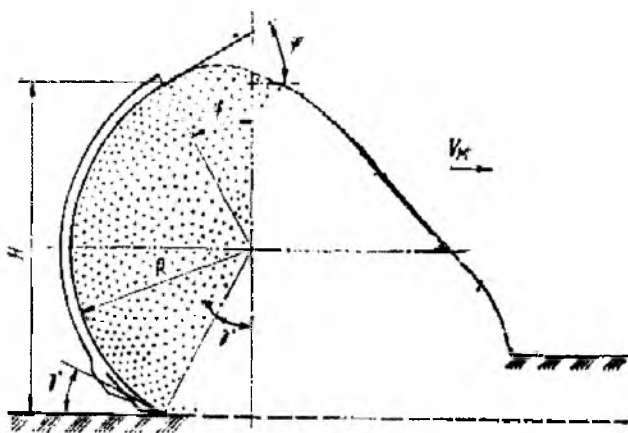
4.24-rasm. Kesilayotgan grunt bilan ag'dargichning ko'ndalang kesim chizmasi
