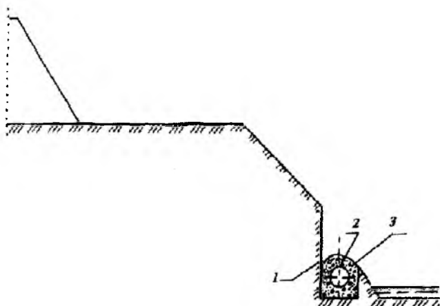
4.50-rasm. Yarim mexanizatsiyalashgan yopiq gorizontal drenaj qurish: 1—transheya; 2—drenaj quvuri; 3—sizdirgich.
