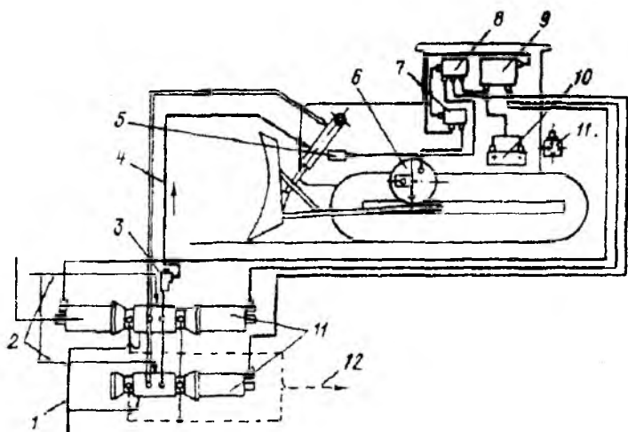
4.6-rasm. Ag'dargichni avtomatik boshqarish sistemasi:
