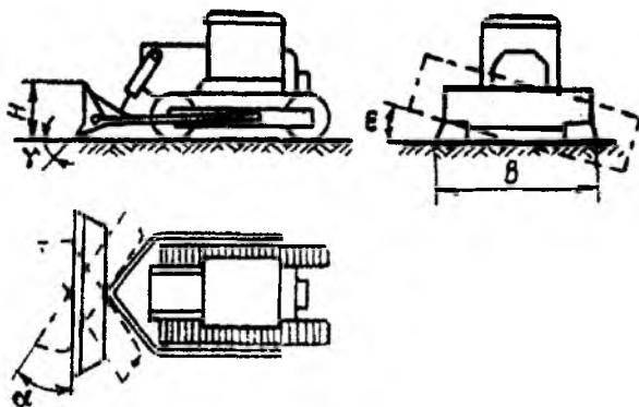
4.1-rasm. Buldozerlar asosiy parametrlarining belgilanishi:
