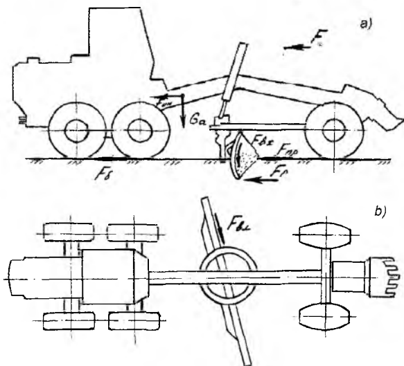
4.25-rasm. Avtogreyderga ta'sir etuvchi kuchlar tasviri.
