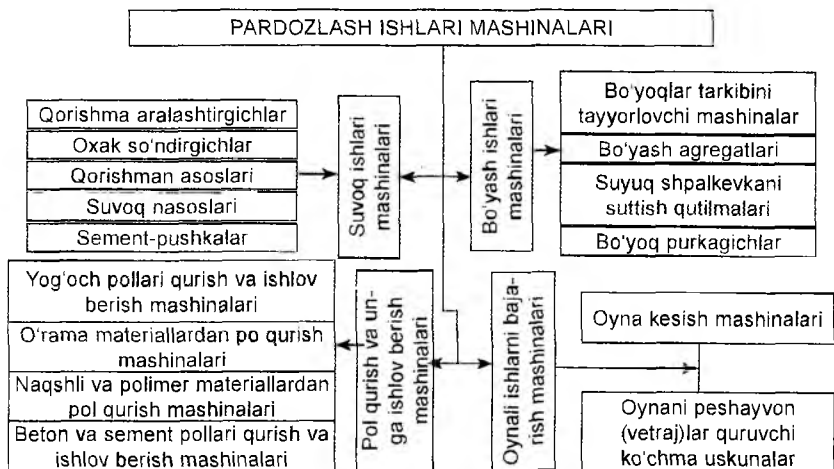
3.22-rasm. Pardoqlash ishlari mashinalari klassifikatsiyasi.
