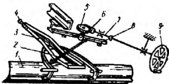
4.17-rasm. Ag'dargichni bir tomonga chiqaruvchi mexanizm:
