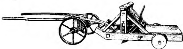
3.6-rasm. Qo'l bilan boshqariluvchi buriluvchan cho'michli ot tordadigan birinchi g'ildirakli skreper (1773-y.)
