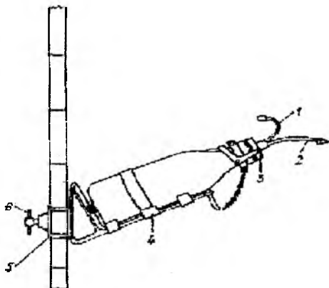
3.3-rasm. Shtangaga o'rnatilgan batometr–butilka: 1–havoni chiqaruvchi quvurcha; 2–suvni yig'uvchi; 3–metall qopqoq; 4–butilkani ushlab turuvchi belbog'; 5–shtanga muftasi; 6–qisuvchi vint.
