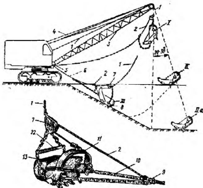
4.26-rasm. Draglaynli bir kovshli ekskavatorning konstruktiv sxemasi: I—osilgan kovshning vaziyati; II—kovsh qazimaga tushirilgan, III—gruntni olish; 1, 2, b—ko'taruvchi, bo'shatuvchi va tortuvchi kanatlar; 3—strela, 4—strela osiladigan kanatlar; 5—yo'naltiruvchi qurilma, 7—kovshni ko'taruvchi blok; 8—kovsh; 9—zanjirni kovshga mahkamlagich; 10, 13—tortuvchi va ko'taruvchi zanjirlar; 11—arka; 12—traversalar.
