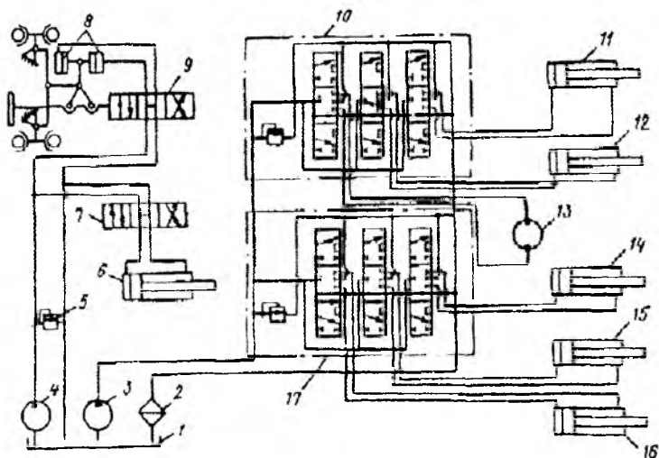
4.21-rasm. DZ-99-1-4 avtogreyderi gidrosistemasining sxemasi:
