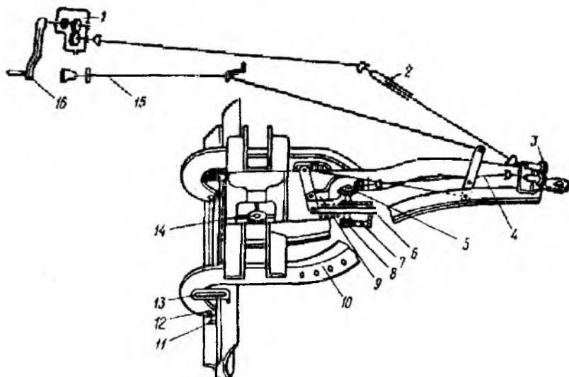
4.16-rasm. Ag'dargichni gorizontall tekislikda buruvchi mexanizm:
