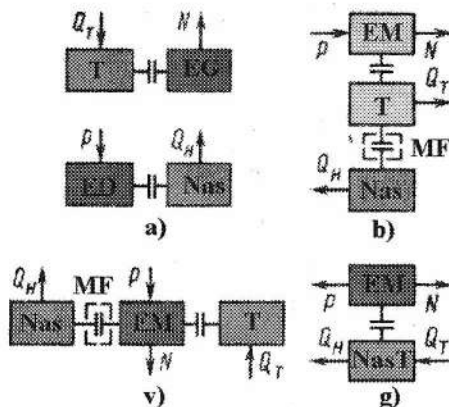
5.34-rasm. GAES agregatlari sxemasi:
