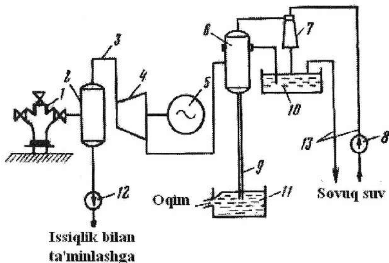
2.29-rasm. GeoIESning texnologik sxemasi.
