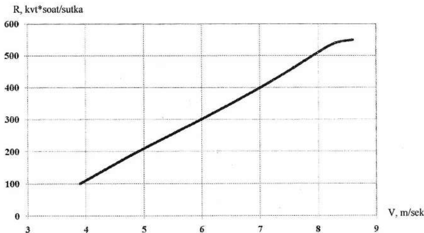
2.23-rasm. Elektr energiya ishlab chiqarishning shamol tezligiga bog'liqligi.
