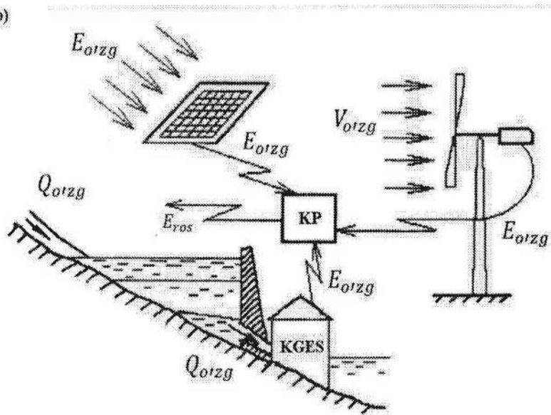
2.46-rasm. 2 yoki 3 elektr stansiya qurilmalarining kombinatsiyalashgan sxemalari
