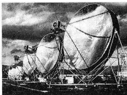
2.6-rasm. Aktiv quyosh tizimi konsentrlatorlari sxemasi va surati ( a ) - to'g'ri burchakli, b ) - parabolik ).
