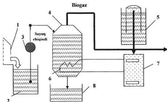
2.36-rasm. Biogaz ishlab chiqarish texnologik sxemasi.
