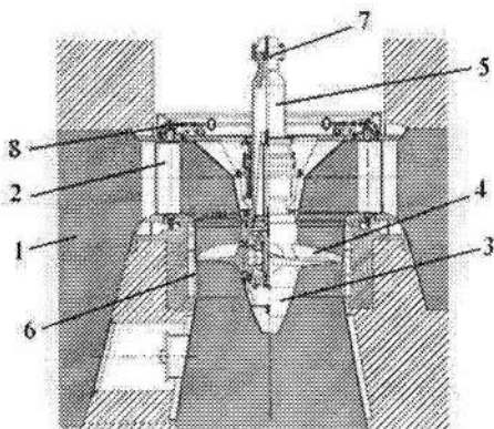
5.1-rasm. O'qiy turbina agregati tasviri:
