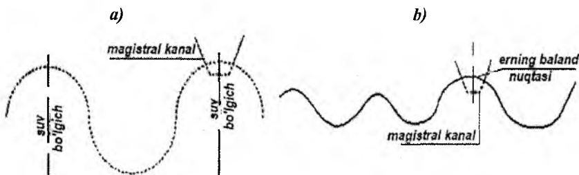
48-rasm. Suv bo'lish cho'qqilaridan (a) va erning baland nuqtalaridan (b) o'tkazilgan sug'orish tarmoqlari.
