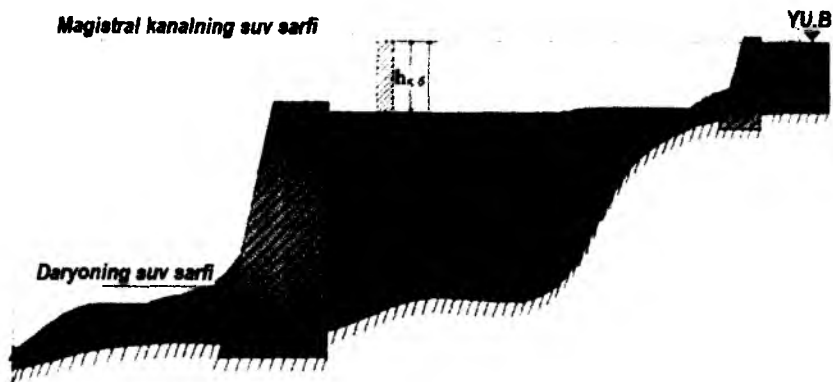
33-rasm. To'g'onni ko'chirish usuli bilan qo'shimcha bosim hosil qilish sxemasi.
