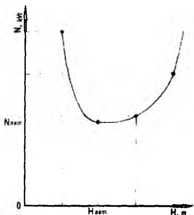
25-rasm. Irrigatsiya tarmog'idagi GES uchun samarali bosimni aniqlash- N = f(H) grafigi.
