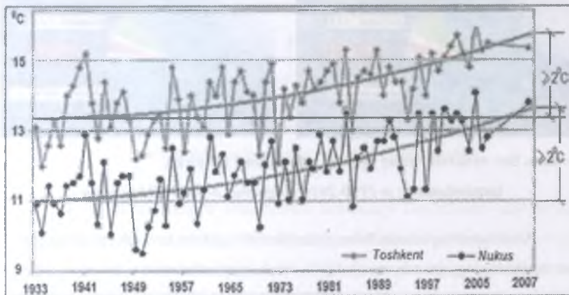
7-rasm. O'zbekistonda iqlim o'zgarishining dinamikasi.
