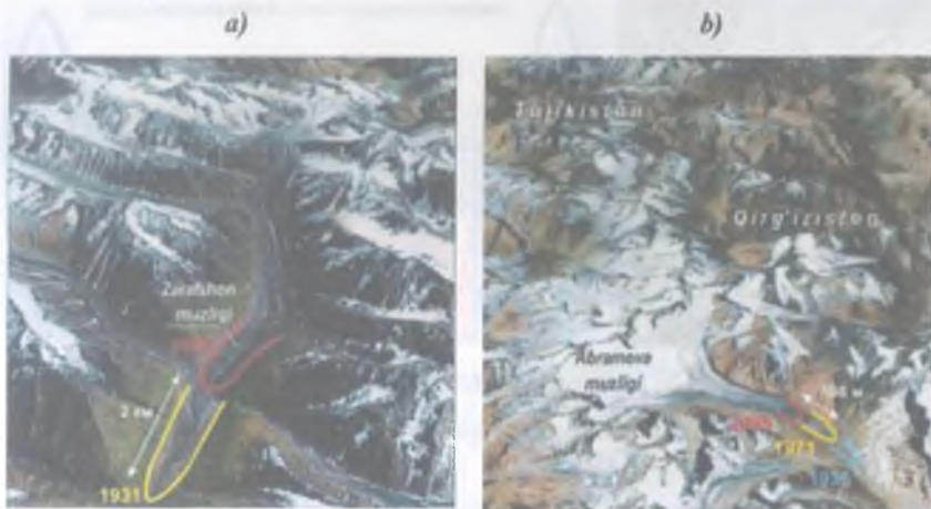
10-rasm. Iqlim o'zgarishi natijasida Zarafshon va Abramov(Qirg'iziston) muzligi o'lchamlari va hajmining qisqarib borishi.
