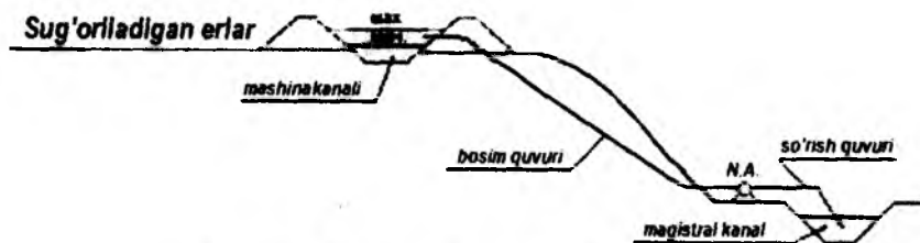
54-rasm. Mashinali suv ko'tarish sxemasi.
