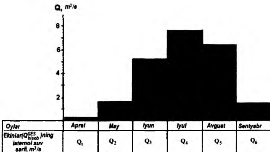
61 - rasm. Suv omboriga biriktirilgan sug'oriladigan erlardagi ekinlarning suv iste'mol qilish hamda GESning hisob suv sarfi pog'onali grafigi.
