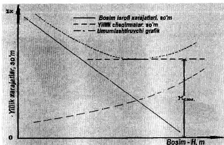
31-rasm. Eng samarador bosimni aniqlash grafigi.
