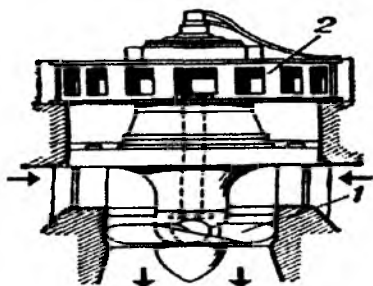
3 -rasm. Gidroagregat:
