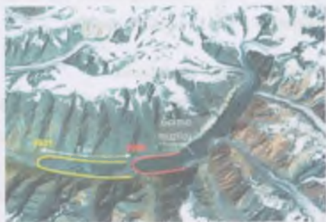
9-rasm. Iqlim oʻzgarishi natijasida Gorma va Batrud muzligi (Tojikiston) oʻlchamlari va hajmining qisqarib borishi
