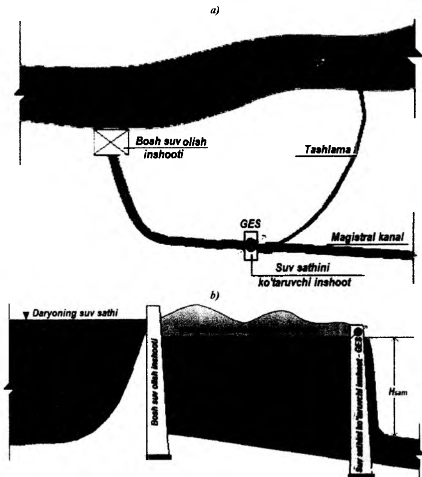
39-rasm. CHuqur qazilgan Magistral kanaldagi GES sxemasi: a-planda ko'rinishi; b-bo'ylama qirgimi.
