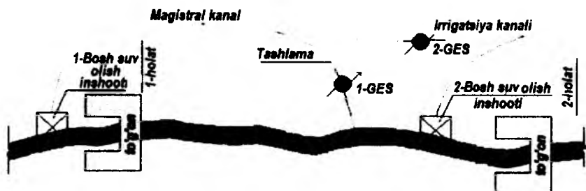
42-rasm. Irrigatsiya rejimini irrigatsiya-energetik rejimga aylantirish sxemasi.
