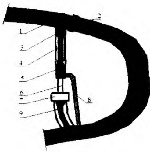
22-rasm. Irrigatsiya tarmog'ida yil bo'yi ekspluatatsiya qilinuvchi GESning sxemasi:
