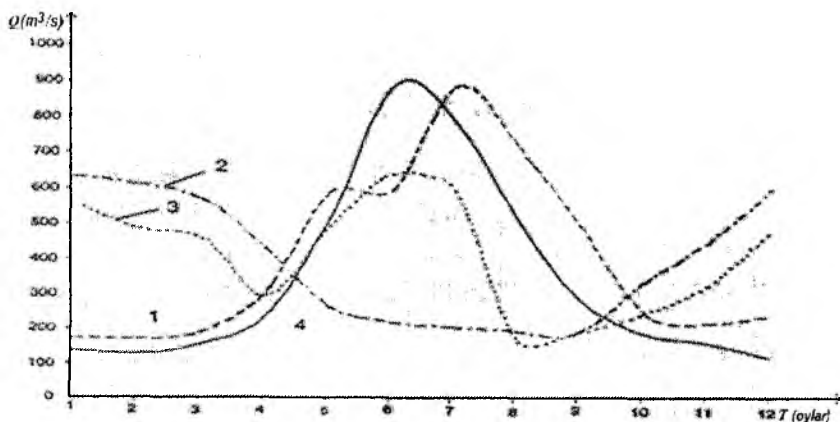
2-rasm. Har xil rejimda ishlayotgan suv omborining suv sarflari: 1-irrigatsion; 2-energetik; 3-birgalikda-(irrigatsion-energetik); 4-suv omboriga o'rtacha ko'p yillik suvni oqib kelishi.
