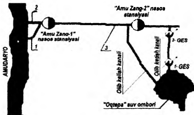
53-rasm. Oqtepa suv omborining olib ketish kanaliga o'rnatiladigan
