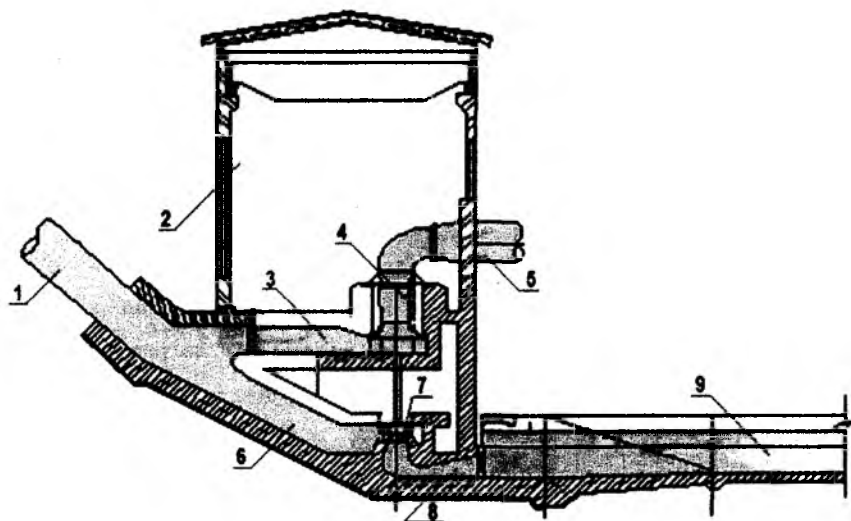
50-rasm. Turbonasos stantsiyasining umumiy ko'rinish sxemasi:
