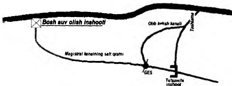
28-rasm. Magistral kanalning nishabligi daryo nishabligidan kichik bo'lgan ( I_{mag.kanal} < I_{daryo} ) holatda energiya ishlab chiqarish sxemasi.
