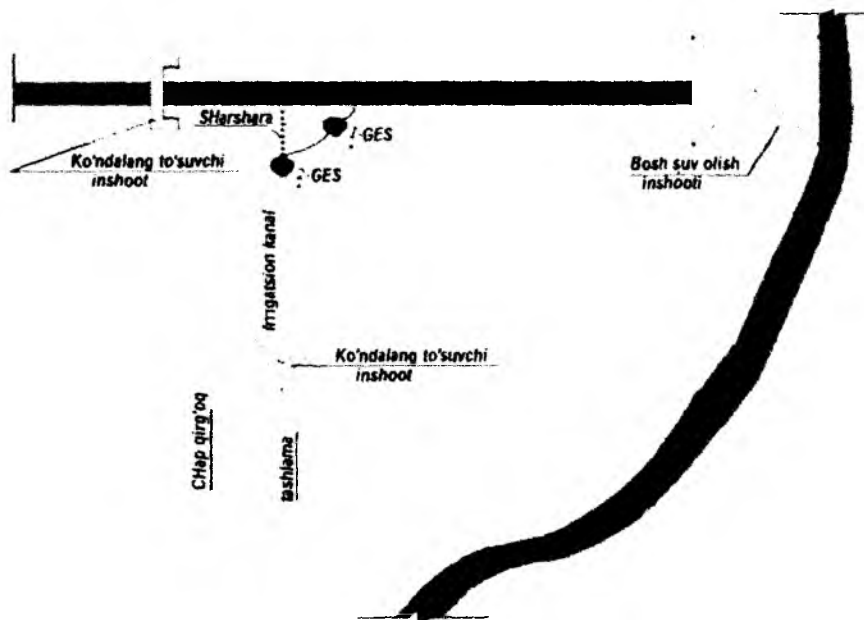
47-rasm. SHarshara va tashlamaga uzatilayotgan suvgao'rnatilgan GES sxemasi.
