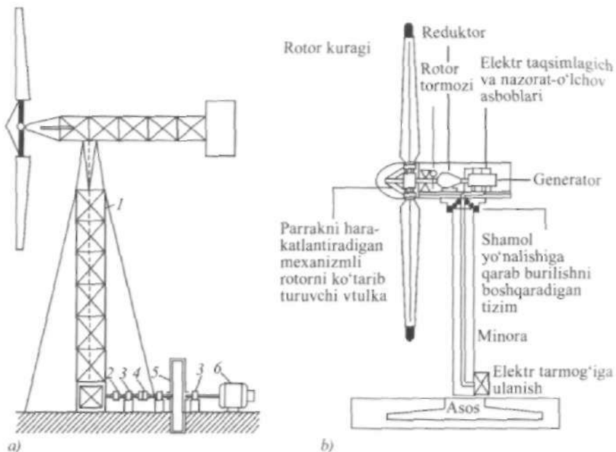
58-rasm. Ana'naviy (a) va zamonaviy sanoat (b) shamol energetik qurilmalarining sxemasi:
