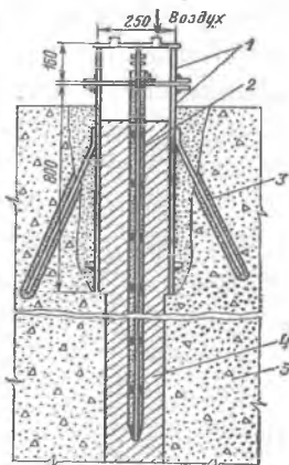
13.14 - rasm. Elektr isitish yordamida asfaltli mastika bilan shponkani qayta tiklash va uni siqilgan havo bilan zichlash:
