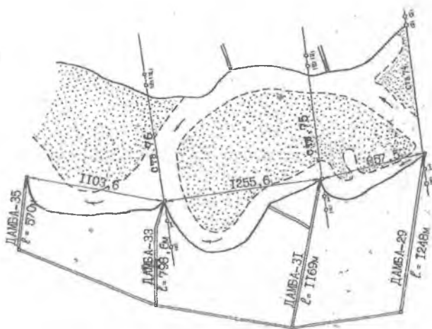
8.17 - rasm. Amudaryoning 29-35-travers dambalari joylashgan hududning 18.09.1987 y plani (s'yomka daryoning chap qirg'og'i bo'ylab-olingan).
