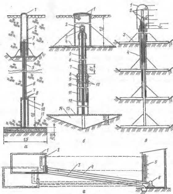
6.7 – rasm. Gruntli toʻgʻonlar tanasidagi choʻkishni oʻlchash uchun qoʻllaniladigan chuqurlik markalari:
