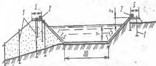
5.1 - rasm. Kanalda pezometrlar va markalarini joylashtirish sxemasi:
