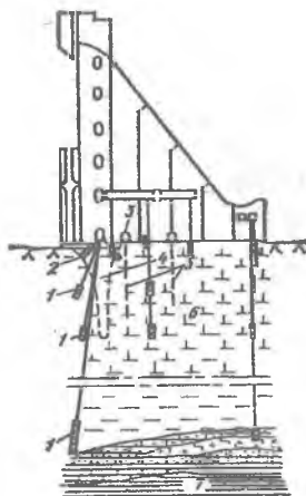
7.16- rasm. Usti-Ilm gravitatsion to'g'oni seksiyalari asosida pezometrlarni joylashtirilish sxemasi:
