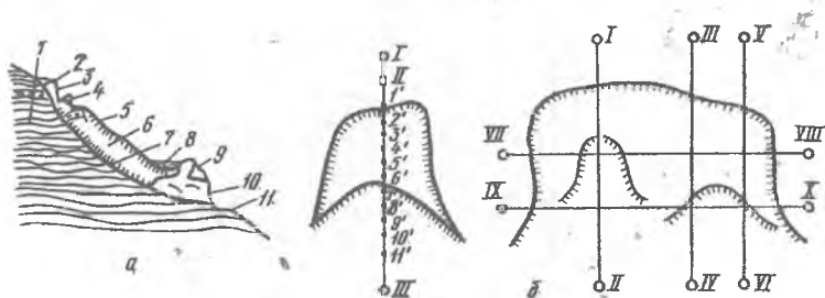
11.2 – rasm. O'pirilish (siljish, ko'chish) sxemasi (a) kuzatuv stvorlarini joylashuvi (b): 1 – ildiz massivi; 2 va 3 – o'pirilish cheti va devori; 4 – ajralish yorig'i; 5 – o'pirilish bosqichi; 6 – o'pirilish tanasi; 7 – o'pirilish to'shagi; 8 – suv turib qolgan joy; 9 – do'ppayish yorig'i; 10 – o'pirilish tili; 11 – o'pirilish asosining deformatsiyasi; I...X – tayanch belgilar; I'...11' – o'pirilishdagi markalar.
