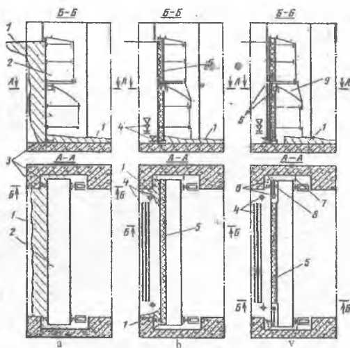
8.7 - rasm. Zatvorni isitish qurilmasini joylashish sxemalari:
