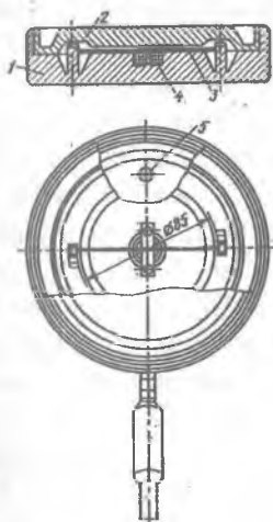
6.19 – rasm. Hidroprojektning to'rli grunt dinamometri:
