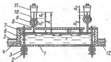
7.4-rasm. Gidrostatik nivelir:
