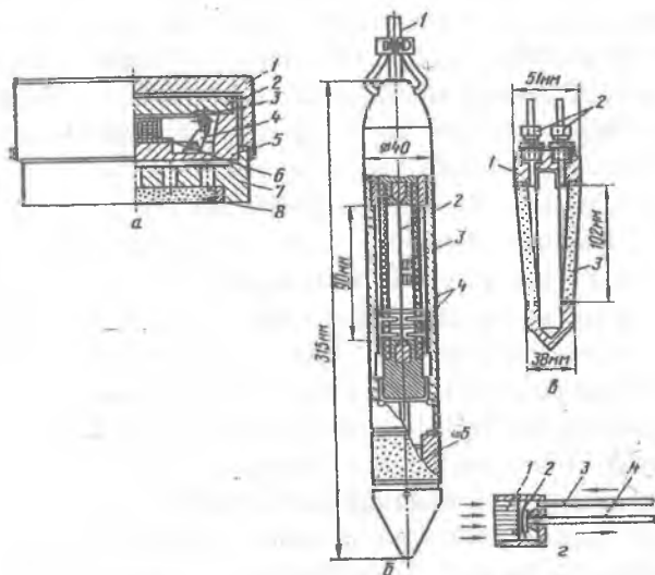
6.18 – rasm. Grunt g'ovakligidagi pezometrik naporni o'lchash uchun asboblari:
