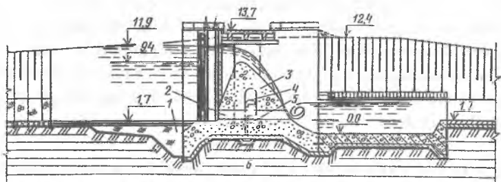
14.3 – rasm. Tezoqarning bosh qismiga qurilgan vodostiv to‘g‘onining ko‘ndalang kesimi: 1 – ponur; 2 – tub oldi suv qo‘ygich; 3 – vodostiv; 4 – ko‘rish (kuzatish) galereyasi; 5 – pezometr; 6 – argillta o‘xshash grunt.
