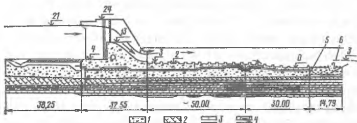
12.3 – rasm. Dnestr daryosidagi Dubossar gidrouzelingining suv tashlamasi bo'yicha qirgimi: 1 – shag'al tosh-qumli gruntlar; 2 – glinasimon mergel; 3 – o'rtacha zichlikdagi ohaktosh; 4 – mergel; 5 – shpunt; 6 – tubning yuvilishgacha bo'lgan sirti. O'lchamlari m.da
