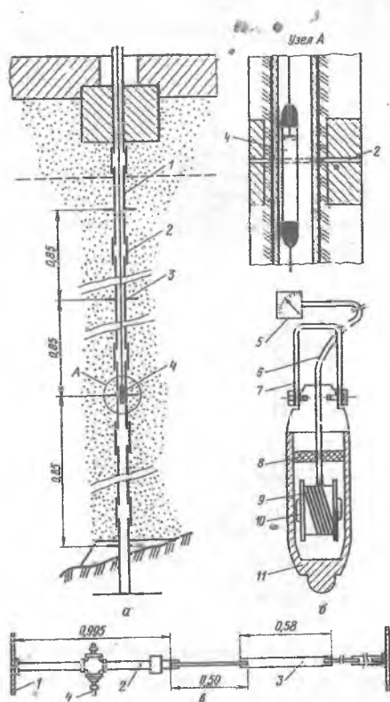
6.8 – rasm. To'g'on tanasining gorizonta va boshqa siljishlarini aniqlaydigan asboblari:
