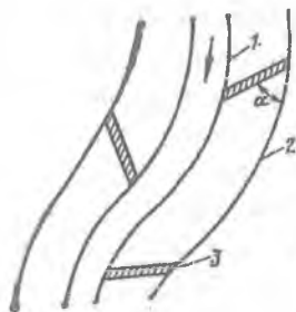
8.1 – rasm Tiqilish hosil bo‘lishiga qarshi kurashish uchun Dubossar suv omboridagi yarim zaprudalarni joylashuvi: 1- daryoda kam suvli davridagi sath; 2 – tiqilish paytidagi maksimal sath; 3 – yarim zapruda.
