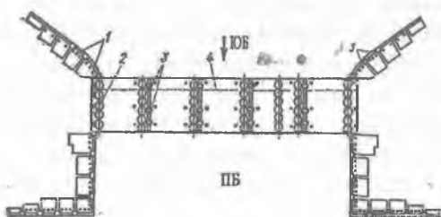
7.19 - rasm. Qoya toshsiz asos ustidagi suv o'tkazuvchi inshoot seksiyalari va qirg'oq ustunlarida NO'A joylashtirish sxemasi: 1 – balandlik markalari; 2 – o'lchagichlar; 4 – shpunt o'qi
