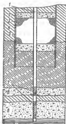
13.10 – rasm. Suv (bosimini) pasaytiruvchi kontakt bo'yicha filtratsiyani bartaraf qilish:
