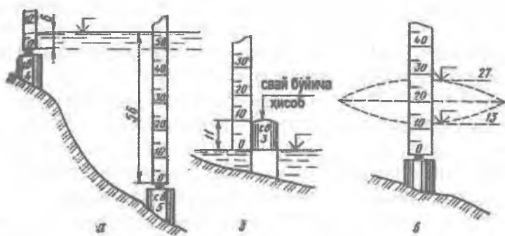
11.1 – rasm. Suv o'lchash postlarida suv sathini o'lchash variantlari: a – ikki svay bo'yicha; b – kuzatish nulidan pastda joylashgan suv sathi bo'lganda; v – erkin sathda to'liqinlanish bo'lgan sharoitda. O'lchamlari sm. da.
