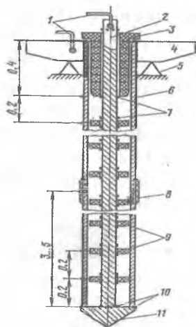
13.13 - rasm. Elektr qizdirgich sxemasi:
