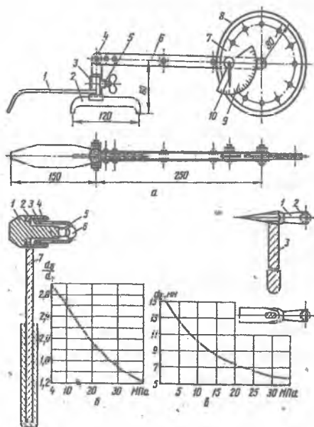
7.11-rasm. Betonni ahamiyatsiz buzush bilan inshootlar sirti mustahkamligini aniqlaydigan asboblari:
