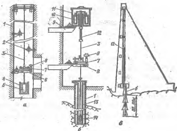
7.5.-rasm. Nisbiy gorizonttal siljishlarni o'lash uchun asboblari: a va b – to'g'ri va teskari otveslar; v – to'g'ri va teskari otveslardan birgalikda foydalanish sxemasi; 1- tushirish quvuri; 2 – ilgak; 3 – invar sim; 4 – tinchlantiruvchi (dempfiruyushaya) suyuqlik bilan bak; 5 – yuk; 6 – koordinatomer uchun stolcha; 7 – koordina- tomer; 8 – optik qurilma; 9 – kronshteyn; 10 – po'kak; 11 – otves boshi; 12 – po'kak shtoki; 13 – himoya quvuri; 14 – yakor.
