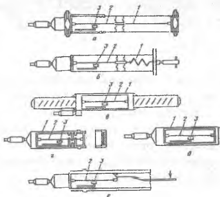
7.14.– rasm. To'rtli o'lchov preobrazovatellari:
