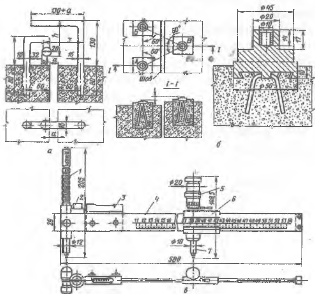
7.9 – rasm. Choklar (yoriqlar) tekislikda (a), fazoda (b) ochilishini o‘lchash uchun yoriq o‘lchagichlar va shtangen yoriq o‘lchagich (v) : 1 – tayanch ninasi; 2 va 3 – halqali va silindrik sath; 4 – shkalasi bilan lineyka; 5 – ninalar barabani; 6 – dvijok; 7 – mikrometrik nina. O‘lchamlari mm. da.
