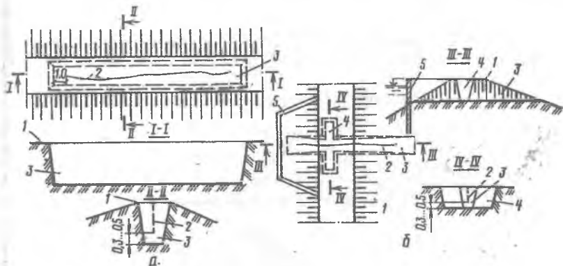
13.1 — rasm Grunt to'g'onlar yoriqlarini butlash:
