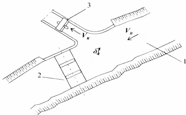
5.3 – rasm. Suv olish inshootining suv manbaiga nisbatan joylashishi.
