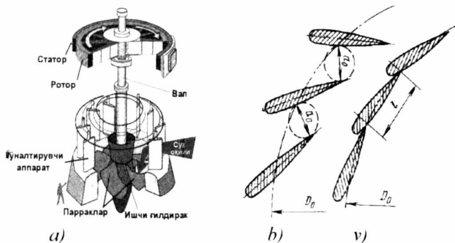
8.12 – rasm. Gidroturbining yo'naltiruvchi apparati.
