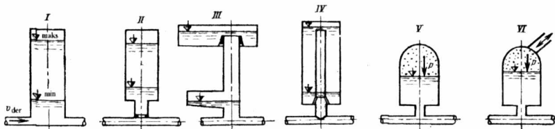
6.10 – rasm. Gidravlik zarba ta'sirini so'ndiruvchi rezervuarlar turlari.
