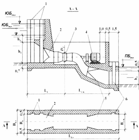
7.6 – rasm. Gorizontol o‘qiy gidroturbinali S shaklida joylashgan so‘rib olish quvuriga ega bo‘lgan o‘zanda joylashgan KGES binosi.
