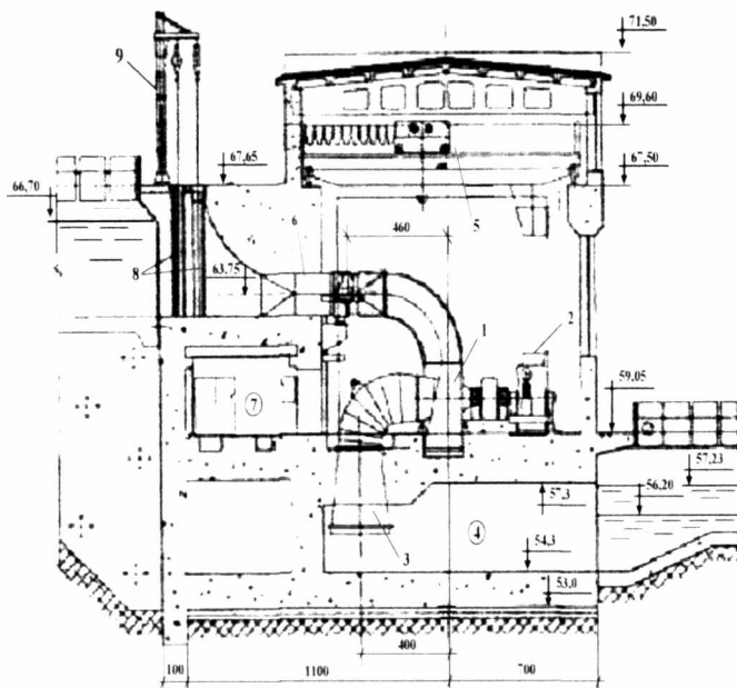
7.14 – rasm. Samarqand viloyatidagi aylanma Dargʻom kanalida joylashgan Urgut KGESi binosining qirqimi.
