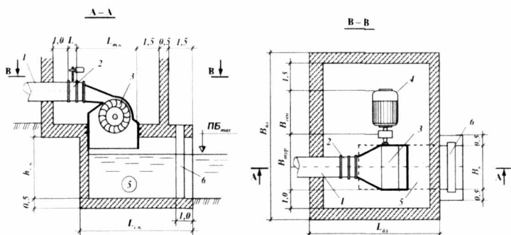
7.13 – rasm. Gorizontaal, ikki karra ta'sir qiluvchi turbina (Banki turbinalari) bilan jihozlangan KGES binosi
