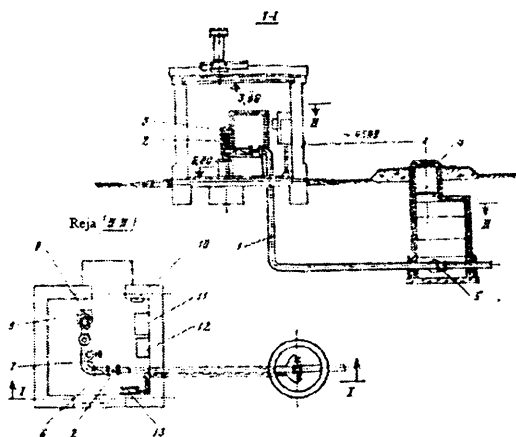
10.22.-rasm. Suvga botirilgan QJB nasos agregati bilan jihozlangan yer ustki nasos stansiyasi:
