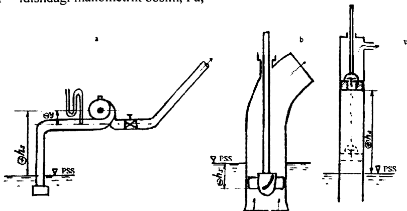
1.6-rasm. Nasoslarning geodezik so‘rish balandligini aniqlash tasvirlari: a- gorizontall valli markazdan qochma nasos; b-vertikal valli o‘qiy nasos; d - vertikal valli porshenli nasos.
