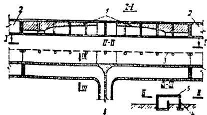
11.6 - rasm. Cho'ktirilgan tirqishli suv qabul qilish qurilmalari:
