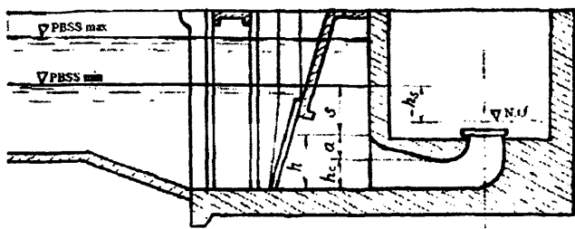
11.4-rasm. Suv keltirish quvurini minimal suv sathiga nisbatan botirilish chuqurligini aniqlash tasviri.
