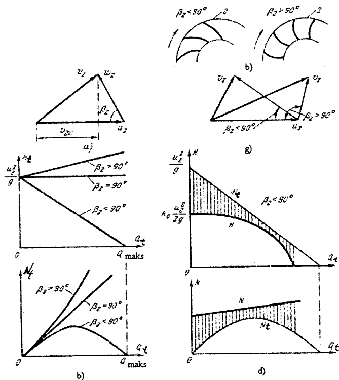
4.1- rasm. Markazdan qochma nasosning nazariy xarakteristikallari.
