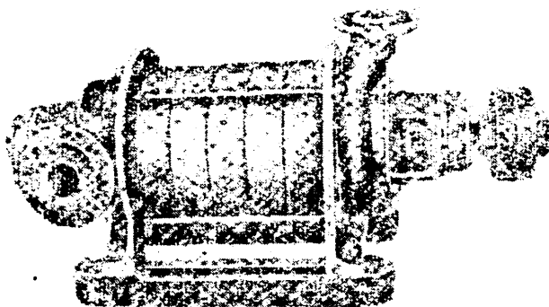
2.8-rasm. Ko'p pog'onali (seksiyali) MC (LHC) turdagi nasosning tashqi ko'rinishi.
