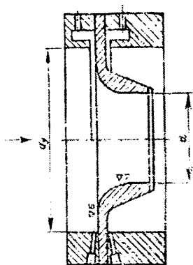
9.23-rasm. Konus naychali suyuqlik sarfi o'lchagichi.
