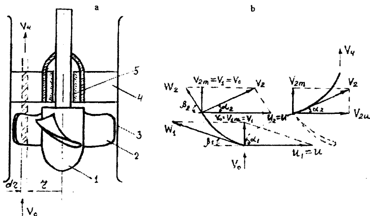
3.2-rasm. O'qiy nasos tasviri (a) va undagi oqimning kinematikasi (b): 1-ishchi g'ildirakning suyri gubchagi; 2-ishchi g'ildirak kuraklari; 3-ish bo'linmasi; 4-to'g'rilovchi moslama; 5- sirpanma podshipnik.
