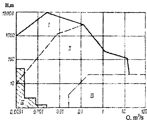
1.4-rasm Nasoslarning qo'llanish chegaralari: I-porshenli; II-markazdan qochma; III- o'qiy; IV- uyurmali; oqimchali; tebranma va boshqalar
