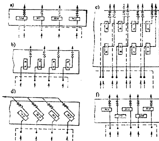
10.3-rasm. Gorizonttal valli nasos agregatlarining to'rtburchak shakldagi binoga joylashtirish.
