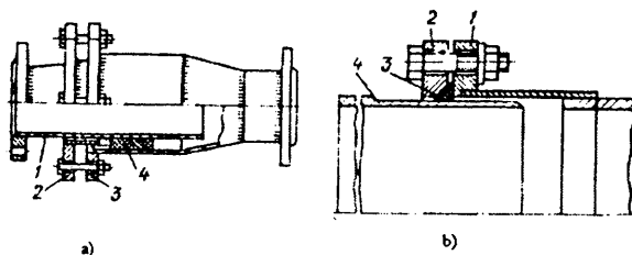
12.12 - rasm. Yig'ish ulamalari:
