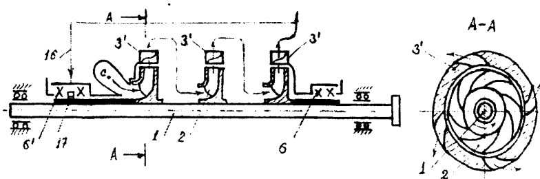
2.7-rasm. Ko'p pog'onali MC (LHC) nasosidagi suyuqlik harakati sxemasi:
