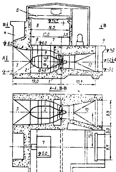
10.9-rasm. Kapsula agregatli nasos stansiya binosi: 1-poydevor; 2-kapsulali agregat; 3-suv chiqarish bo‘linmasi; 4-oraliq devor; 5-yuk ko‘tarishi 100 t li ko‘priksimon kran; 6-elekt kommunikasiyalari kanali; 7-ochiladigan tuynik; 8- mashina zali; 9-nasos joylashgan suv oqish qismi; 10-so‘rish quvuri.
