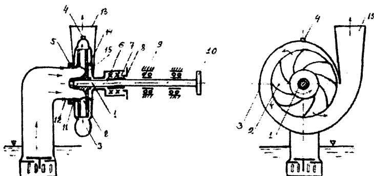
2.1-rasm. Markazdan qochma nasosning ishlash tasviri:
