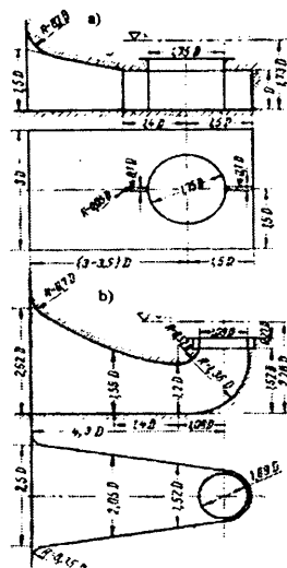
10.6-rasm. Suv keltirish quvurlari: a - to'rtburchak kesim yuzali; b- tirsaksimon.
