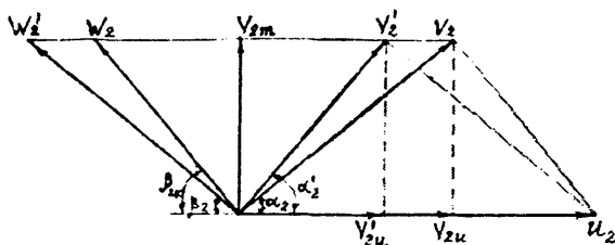
3.5-rasm. Kuraklar soni cheklanganda ishchi g'ildirak tezliklar parallelogramining o'zgarishi.
