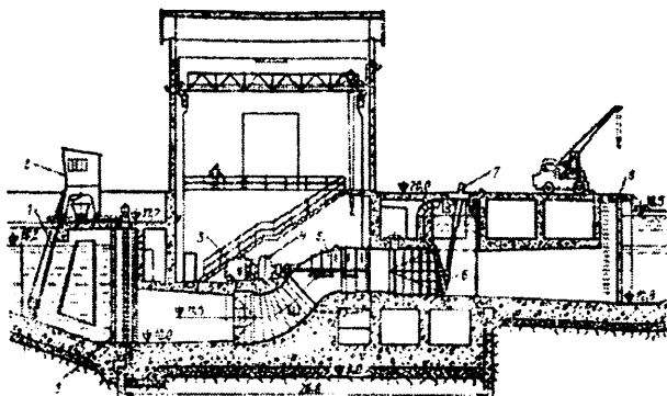
10.7-rasm. «Rivo Kolsoni» (Italiya) firmasining gorizontall valli o'qiy nasoslari o'rnatilgan Impianto Lepri nasos stansiyasi.
