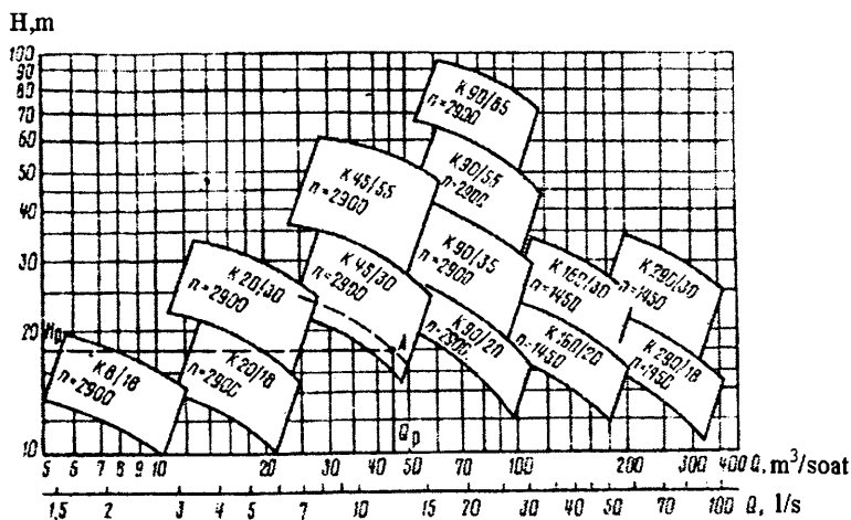
4.15-rasm. Markazdan qochma K turdagi nasoslarning jamlangan grafigi.
