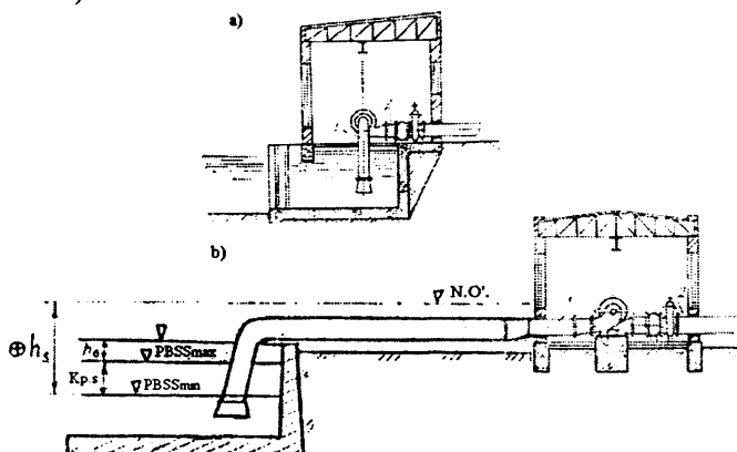
10.12-rasm. Yer ustki binolari:
