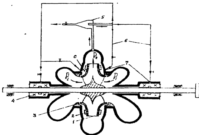
5.9-rasm. Markazdan qochma D turdagi nasoslarning ishchi g'ildiragi zichlash elementlarini kavitatsion-abraziv yeyilishdan saqlash sxemasi:
