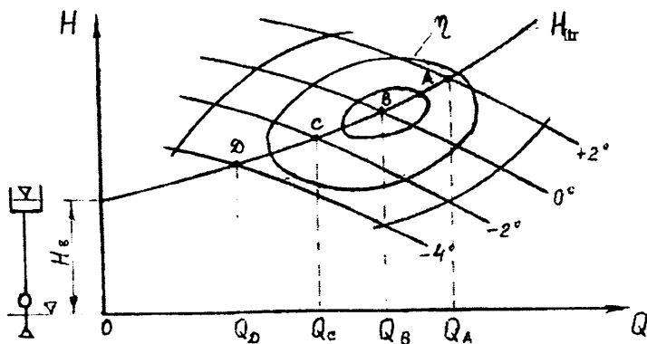
4.8-rasm. O'qiy nasos kuraklarini burilish burchagini o'zgartirib rostdlash.
