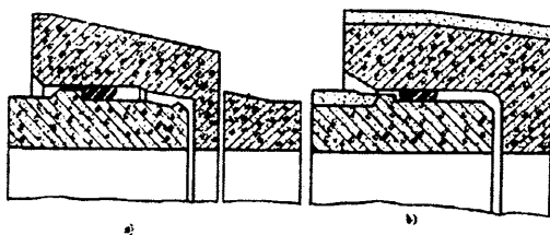
12.15 - rasm. Yig'ma temir-beton quvurlarning kengayma shakldagi ulanish qismi:
