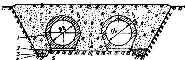
12.17 - rasm. Quyma temir - beton quvurlarni kesimi:
