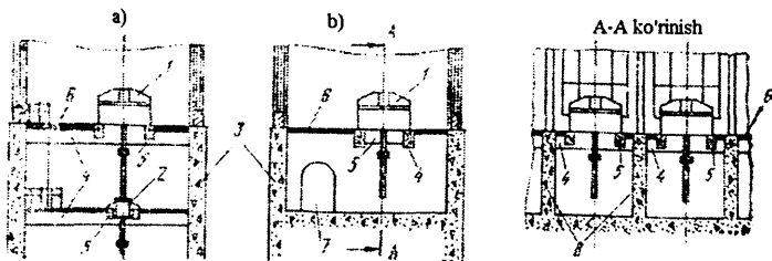
10.16-rasm. Vertikal valli elektr dvigatellarning tayanchlari konstruksiyalari:
