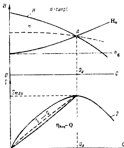
4.6-rasm. Nasosning haqiqiy ish tartibini aniqlash.
