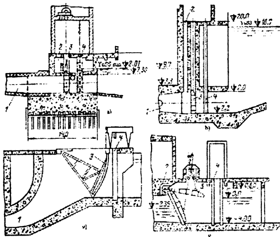
13.1 - rasm. Turli xil darvozalar oʻrnatilgan mexanik qulfakli suv chiqarish inshooti tasvirlari:
