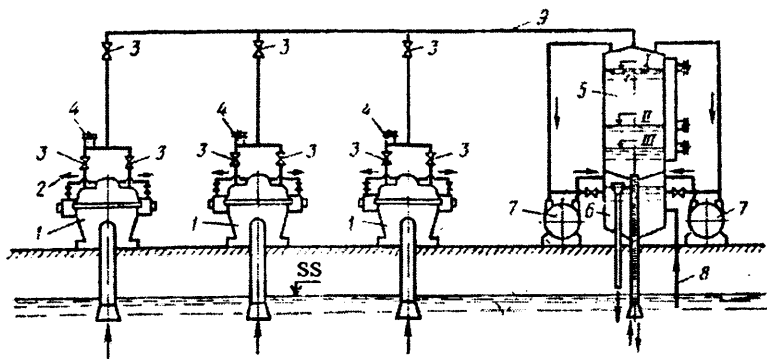
9.13 -rasm. Vakuum-qozonli vakuum hosil qiluvchi qurilma: 1- asosiy nasoslar; 2- salniklarga suv uzatuvchi quvurcha; 3 - ventil; 4 - suv sathi signalchisi; 5 - vakuum -qozon; 6- suv quyish idishi; 7- vakuum-nasoslar; 8- qo'l nasosi quvuri; 9- havo so'rish quvuri.
