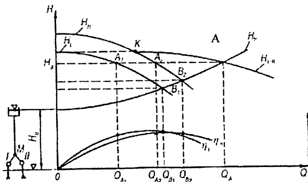
4.12-rasm. Ikkita har xil nasosning parallel ishlashi.
