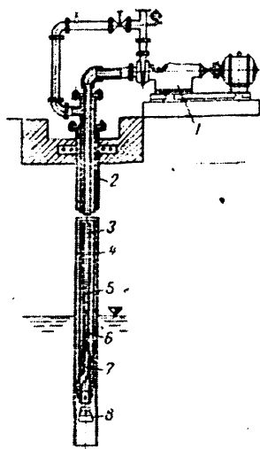
7.5-rasm. Quduqdan suv chiqaruvchi oqimchali nasos qurilmasining tasviri: 1-markazdan qochma nasos; 2-o'rama quvur; 3-oqimchali nasosning suv ko'tarish quvuri; 4-bosimli suv berish quvuri; 5-diffuzor; 6-aralashish bo'linmasi; 7-konus naycha; 8-so'rish qopqog'i.
