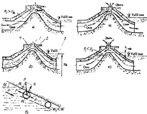
13.2 - rasm. Nasosni ishga solish va to'xtatish holatlarida sifonni ishlash tasviri:
