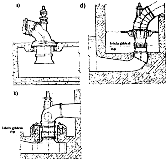
10.15-rasm. Vertikal valli O, OII turdagi o'q'iy nasoslarning o'rnatilishi.
