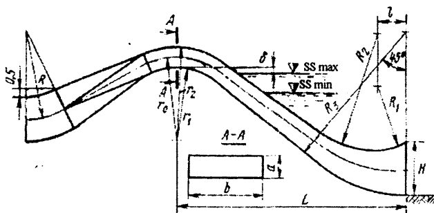
13.7-rasm. Qarshi magistral kanalidagi nasos stansiyalarining suv chiqarish inshootlari uchun tavsiya etilgan sifon shakli.
