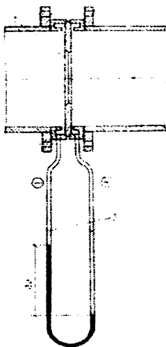
9.22-rasm. Diafragmali suyuqlik sarfi o'lhagichi: 1-diafragma, 2-bosim o'lchash bo'linmasi, 3-difmanometr.
