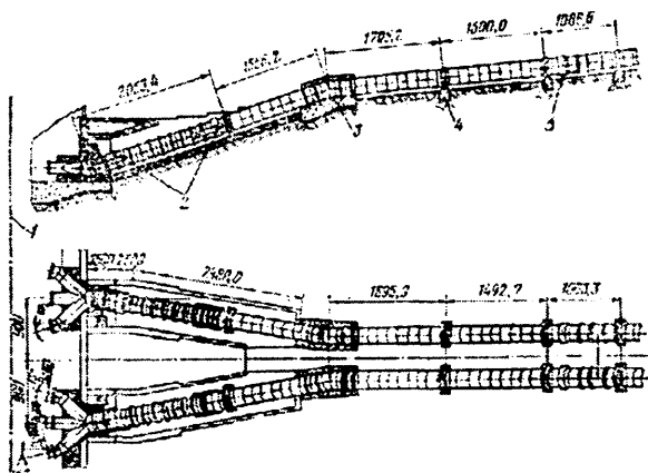
12.18 - rasm. Katta nasos stansiyadagi ochiq po'lat quvurlarni mujassamlanish tasviri:
