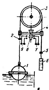
9.27-rasm Qalqovuchli suv sathi relesi: 1- qalqovuch (po'kak); 2 va 5 –chegaralovchi shaybalar; 3- blok; 4-koromisla; 6-yuk; 7 va 9- elektr simlari; 8-kontaktlovchi moslama.
