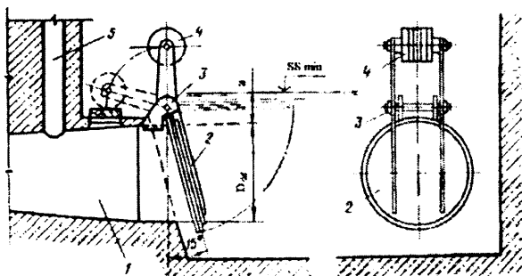
13.3-rasm. Teskari qopqoqli yopqich:
