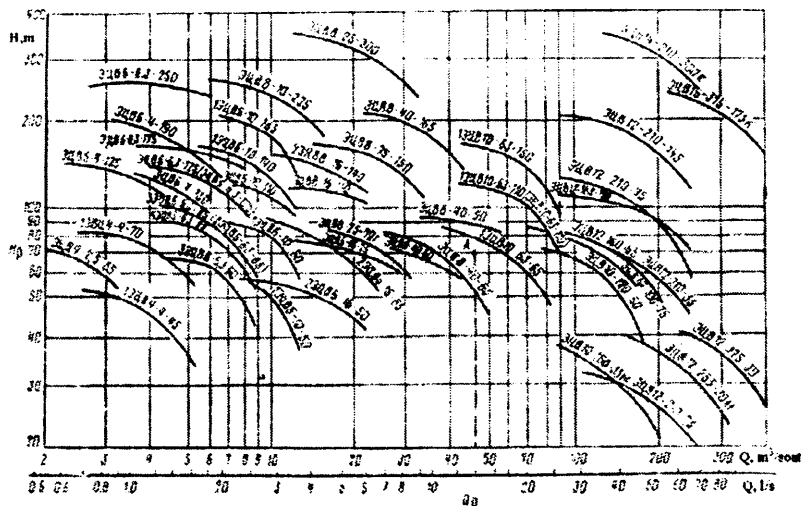
9.5-rasm. Markazdan qochma ЭЛБ turdagi artezion nasoslarning jamlangan grafiklari.
