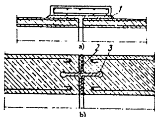
12.16 - rasm. Deformatsiya choklari a - qo'zg'almas temir - beton mufta; b - rezina shponkali egiluvchan chok; 1 - sement qorishma; 2 - bitum aralashmasi; 3 - rezina.
