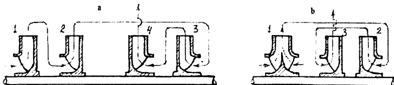
2.10-rasm. M va MD (QH) turdagi markazdan qochma nasoslarda suyuqlik harakati sxemasi: a-M nasosi; b-MD nasosi.
