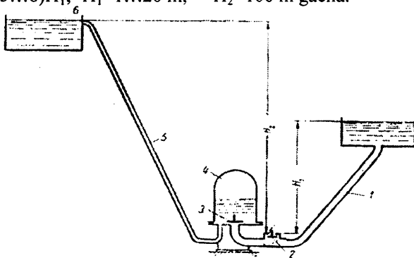
7.9-rasm. Gidravlik taran tasviri:
