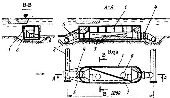
11.7 - rasm. Uyurma bo'linmali ochiq turdagi suv qabul qilish qurilmasi:
