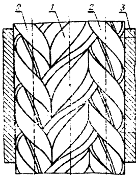
6.9-rasm. Uch vintli 3B nasos tasviri: 1-yetaklovchi vint, 2-ergashuvchi vint, 3-stator.
