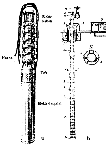
2.14-rasm. Cho'ktiriladigan elektr dvigatelli quduq nasosi-ning tashqi ko'rinishi (a) va o'rnatilish sxemasi (b):
