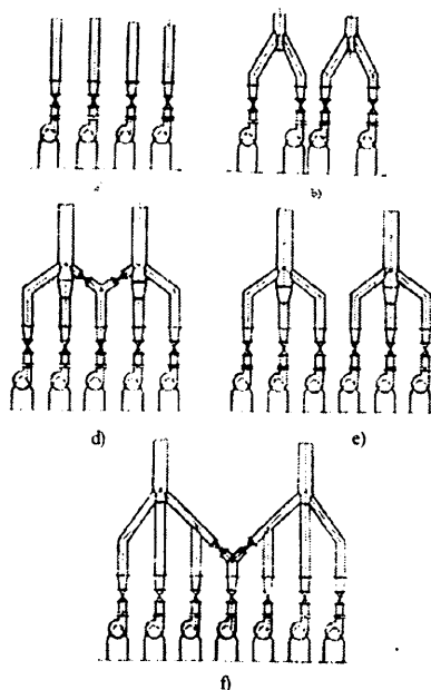
12.3 - rasm. Vertikal valli nasoslar o'rnatilgan sug'orish tizimi nasos stansiyalarining bosimli kommunikatsiyalari tasvirlari: a - alohida quvurlarga suv uzatish; b, d, e, f - ikkita quvurga suv uzatish.
