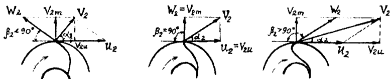
3.6-rasm. Kuraklarning egilishini turli holatlari.
