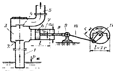
6.1-rasm. Bir tomonlama ishlovchi porshenli nasos tasviri: 1 va 5-soʻrish va bosimli quvurlari; 2 va 4-soʻrish va bosimli qopqoqlari; 3-ish boʻlinmasi; 6-porshen; 7-silindr; 8-dasta; 9-polzun (kreyskopf), 10- shatun; 11-krivoship.
