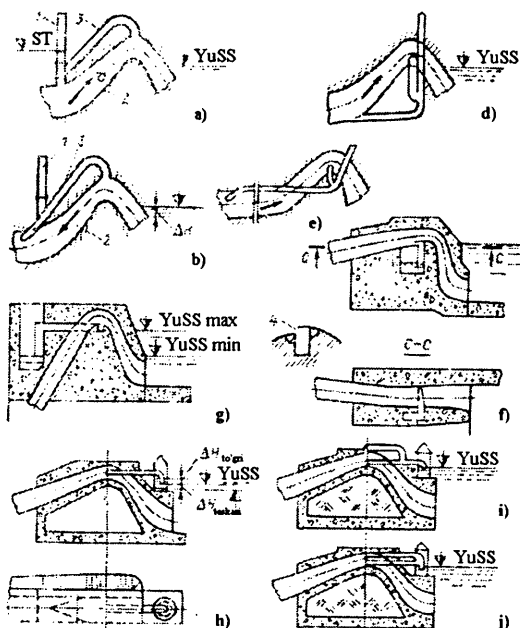
13.8- rasm. Gidravlik vakuum yo'qotish qopqoqlari tasvirlari: 1-stakan-pezometr; 2-yuqoriga ko'tariluvchi tarmoq; 3-havo quvurchasi.
