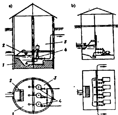
8.14-rasm. Chiqindi suvlarni chiqarish nasos stansiyalari tasvirlari: a - doira shaklidagi kesim yuzali; b - to'rtburchak shaklidagi kesim yuzali; 1 - suv qabul qilish hovuzi; 2 - panjara; 3 - mashina xonasi; 4-nasos.
