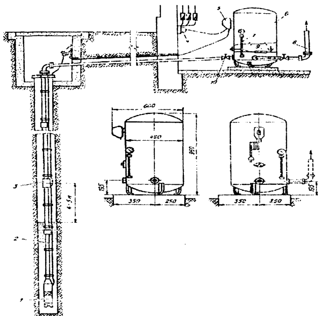
10.23-rasm. Suvga botirilgan nasos agregatli avtomatlashgan nasos stansiya:
