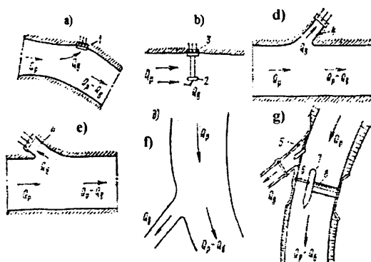
11.1 - rasm. Suv olish inshooti turlari:
