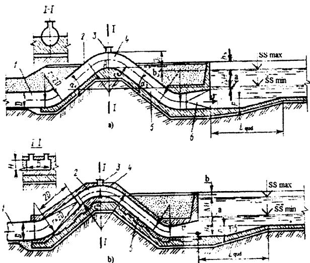
13.6 –rasm. Kesim yuzasi yumaloq (a) va to'rtburchak shakldagi sifonli suv chiqarish inshootlari (b):
