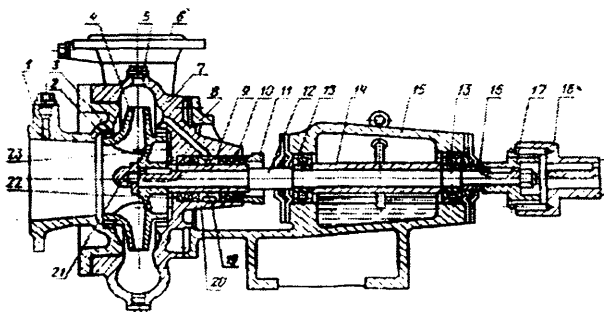
2.2-rasm. Konsolli K turdagi markazdan qochma nasosning tuzilishi:
