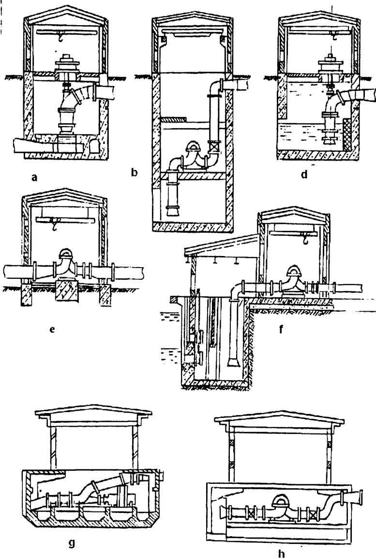
10.2-rasm. Nasos stansiya binolarining shakllari.
