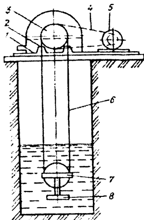
7.8-rasm. Tasmali suv uzatkich tasviri:
