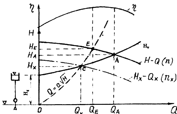
4.10-rasm. Nasosning xarakteristikasini aylanish chastotasini o'zgartirish usuli bilan qayta qurish
