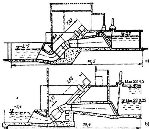
10.8-rasm. Qiya valli nasos agregatlari joylashgan nasos stansiyalar: a - «Xitochi» firmasining o'qiy nasoslari o'rnatilgan; b - shu firmaning diagonal nasoslari o'rnatilgan.
