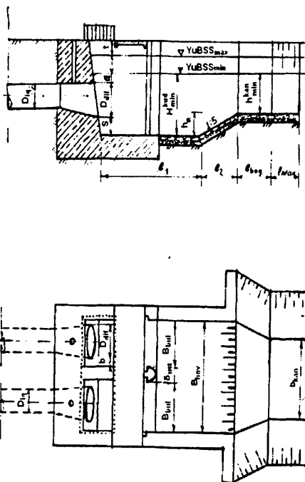
13.4-rasm. Mexanik qulfakli suv chiqarish inshootining o'lchamlarini aniqlash tasviri.
