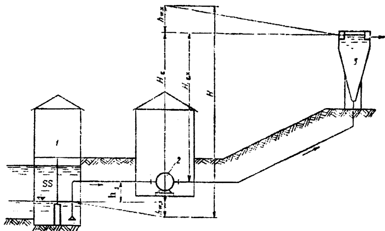
8.9-rasm. Suv ta'minoti tizimidagi birinchi ko'taruv nasos stansiya tasviri:
