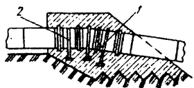
12.19- rasmi. Anker tayanchining tuzilishi: 1 - anker; 2 - xomut.
