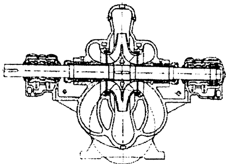
2.6-rasm. Markazdan qochma D turdagi nasosning bo'ylama kesimi.
