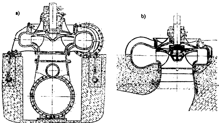
10.14-rasm. Vertikal valli B turdagi markazdan qochma nasoslarning o'rnatilishi
