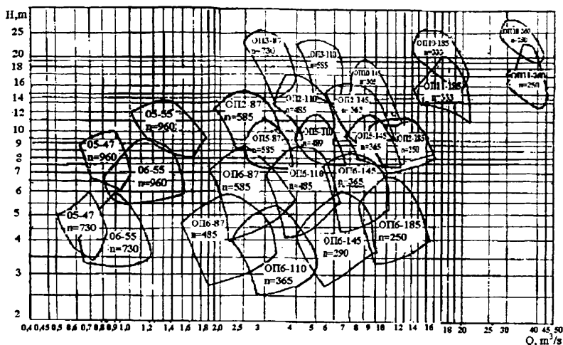
9.6 - rasm. O'qiy O va OII turdagi nasoslarning jamlangan grafiklari.
