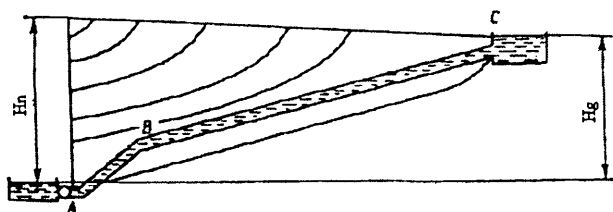
12.21-rasm. Bosimli quvurdagi bosim pasayish to'liqini tarqalish tasviri.
