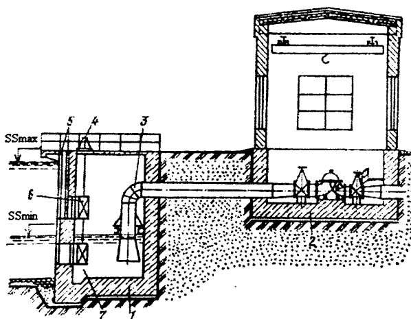
8.4-rasm. Alohida joylashgan qirg'oqdagi nasos stansiya tasviri: 1-qirg'oqdagi suv olish qudug'i; 2-nasos stansiya binosi; 3-so'rish quvuri; 4-qulfakni rostlash uskunasi; 5-panjara o'rnatish o'yilmasi; 6-to'suvchi qulfak; 7-chuqurcha.
