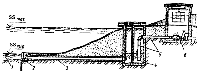
11.5 - rasm. Alohida quriladigan o'zandagi suv olish inshoti tasviri:
