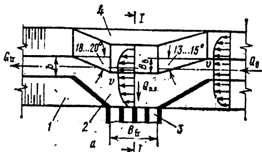
11.14 - rasm. Kanal yonidan suv olish inshooti:
