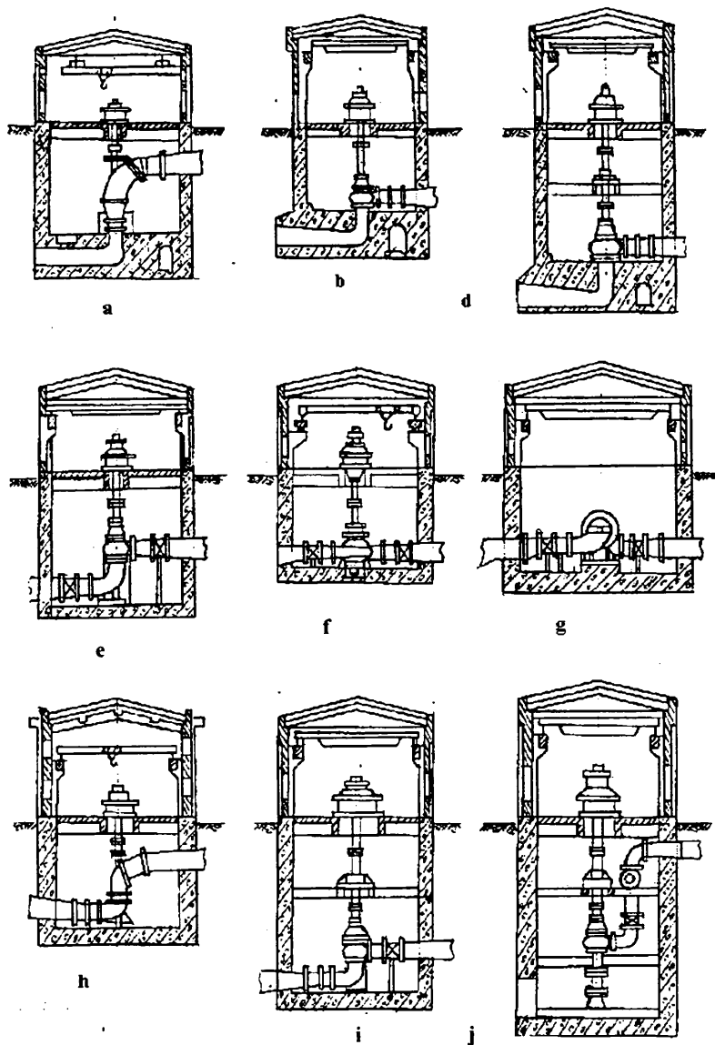
10.1-rasm. Nasos stansiya binolarining shakllari.
