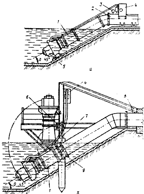
2.17-rasm. Cho'ktiriladigan monoblok shakldagi ОПБ nasoslarining o'rnatilish tasvirlari:
