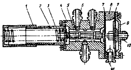
12.8 - rasm. Rostlovchi qopqoq tasviri:
