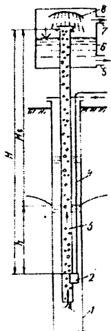
7.6-rasm. Erliftning o‘rnatilish tasviri: 1-quduq, 2-forsunka; 3-suv ko‘tarish quvuri; 4-havo uzatish quvuri; 5-olib ketish quvuri; 6-suv qabul qiluvchi idish; 7-havo chiqarish teshikchasi; 8-to‘suvschi devor.
