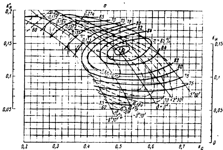
4.4-rasm. O'qiy OP5 turdagi nasosning o'lchamsiz xarakteristikasi.
