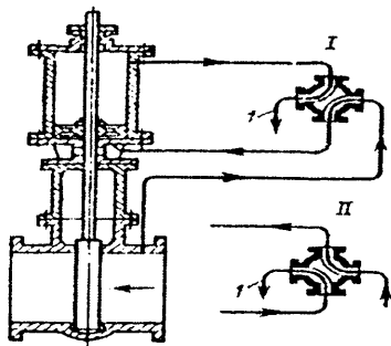
12.6 - rasm. Gidravlik uzatmali surilma qulfakni harakatlanish tasviri:
