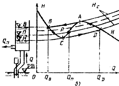
5.3-rasm. O'qiy nasosning beqaror ish tartiblari.
