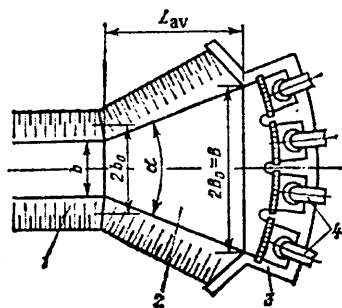
11.12 - rasm. Egri chiziq o'qli suv qabul qilish qurilmalariga ega bo'lgan suv olish inshooti:
