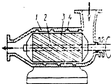
7.2-rasm. Labirintli nasos tasviri: 1-stator; 2-rotor; 3-rotorning vintli kanallari; 4 -halqali ariqchalar.
