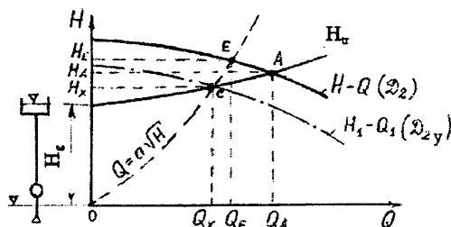
4.9-rasm. Ishchi g'ildiragini yo'nish yo'li bilan markazdan qochma nasos xarakteristikasini qurish.
