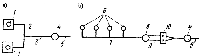
8.12 - rasm. Yer osti manbasidan suv olish tasvirlari: a-yakka quduqdan suv olish; b-guruhlangan quduqlardan suv olish; 1-nasos o'rnatilgan quduq; 2-kollektor; 3-bosimli quvur; 4-suv minorasi; 5-tarqatuvchi tarmoq (iste'molchi); 6-nasossiz quduqlar; 7-o'zi oqar yoki sifonli quvurlar; 8-yig'ish qudug'i; 9-so'rish quvurlari; 10-nasos stansiya binosi.
