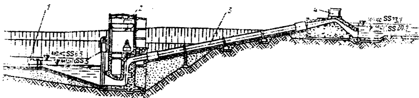
8.7-rasm. Qarshi magistral kanalidagi oraliq nasos stansiya: 1-xas-cho'p to'suvchi panjara; 2-nasos stansiya binosi; 3-bosimli quvurlar; 4-sifonli suv chiqarish inshooti.
