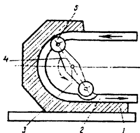
6.13-rasm. Shlangli nasos tasviri: 1-nasos qobig'i; 2-shlang; 3-podshipnik; 4-dasta; 5-juvoz.
