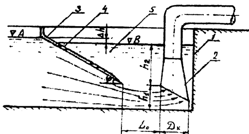
11.11 - rasm. Oqim yo'naltiruvchi devorchali suv qabul qilish bo'linmasi:
