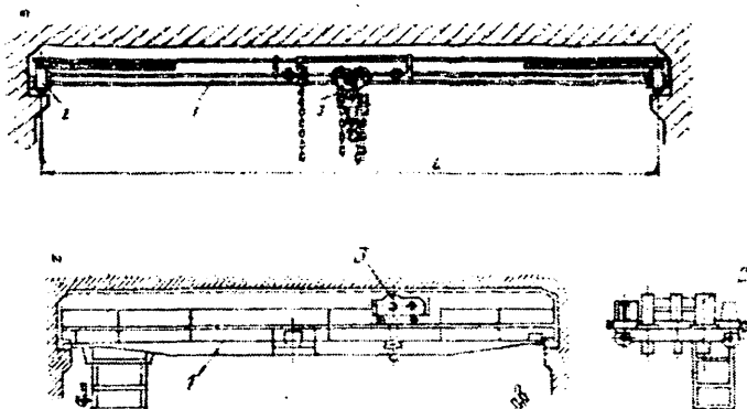
9.20-rasm. Ko'priksimon kranlar: a-qo'lda boshqariladigan (yuk ko'tarishi 3,2...8t); b-elektrlashgan (yuk ko'tarishi 5...50 t); 1-ko'priki; 2-ko'prikn harakatlantirish mexanizmi; 3- yukni ko'tarish va harakatlantirish mexanizmi.
