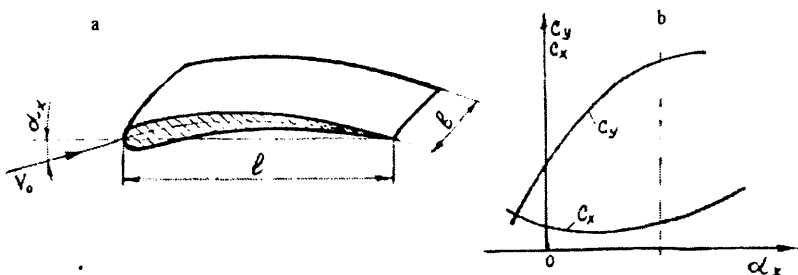
3.3-rasm. O'qiy nasos ishchi g'ildiragi kuragining profili (a), qarshilik va ko'tarish kuchlari koeffitsiyentlarining hujum burchagi \alpha , ga bog'likligi (b).
