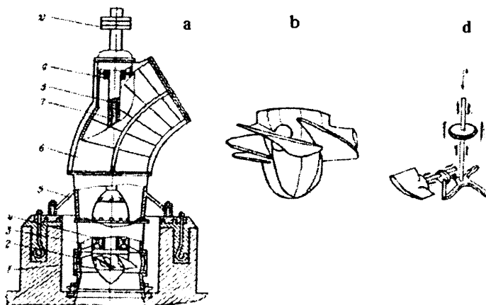
2.16-rasm. O‘qiy nasos tuzilishi (a), ishchi g‘ildiragi (b) va kuraklarini burish mexanizmi (d):
