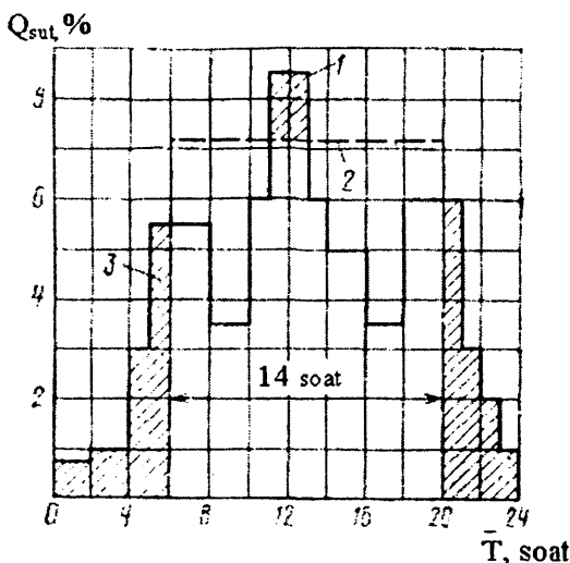
9.12 - rasm. Sutkalik suv iste'moli (1) va suv uzatish (2) grafiklari: 3 – suv minorasi idishidan suv sarfi.
