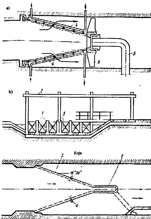
11.15 - rasmi. Konusli (a) va yassi to'rtli (b) baliq to'sish qurilmalari:
