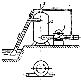
9.15-rasm. So'rish tormog'iga akkumulator – idish o'rnatilgan nasos qurilmasi tasviri:
