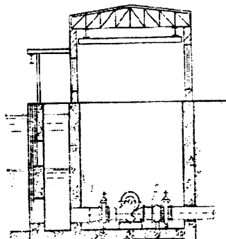
10.10-rasm. Gorizontall valli markazdan qochma nasoslar o'rnatilgan quruq bo'linmali bino: 1-so'rish tarmog'i; 2-bosimli tarmoq.
