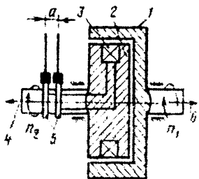
9.9- rasm. Elektr magnet muftaning tuzilishi: 1- yakor; 2- induktor; 3- qo'zg'atish cho'lg'amli; 4 –nasos vali; 5 – bog'lanish halqalari; 6- dvigatel vali.
