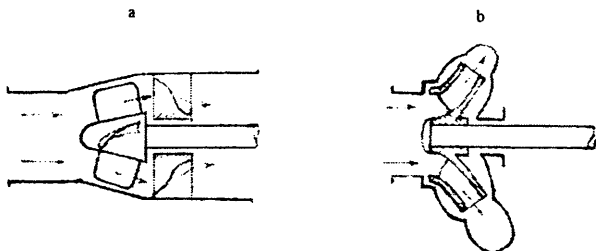
2.18-rasm. Diagonal nasoslar tasvirlari:
