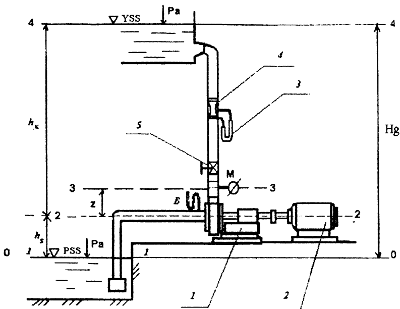
1.5-rasm. Nasos qurilmasining shakli.
