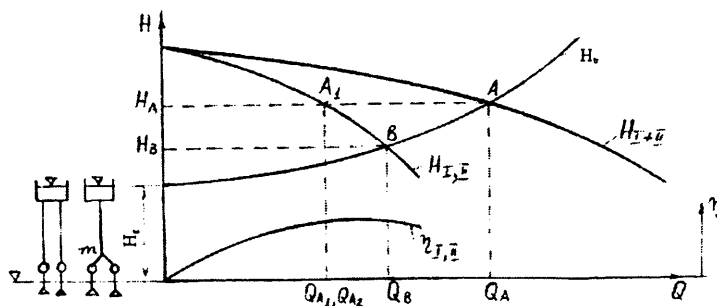
4.11-rasm. Ikkita bir xil nasosning parallel ishlashi.
