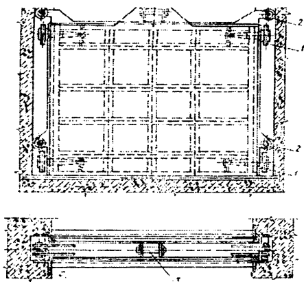
9.16- rasm. Yassi metall darvoza: 1-g'ildirak; 2-yo'naltiruvchi rolik; 3-osilchoq.
