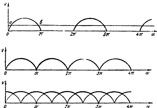
6.6-rasm. Porshenli nasoslarning suyuqlik uzatish grafiklari: a-bir tomonlama ishlovchi bir porshenli nasos uchun; b-ikki porshenli nasos uchun; d-uch porshenli nasos uchun.
