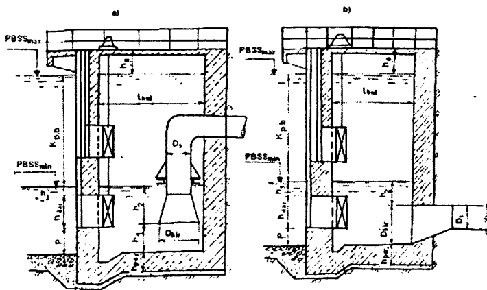
11.2-rasm. Qirg'oqdagi binodan alohida joylashtirilgan suv olish inshooti:
