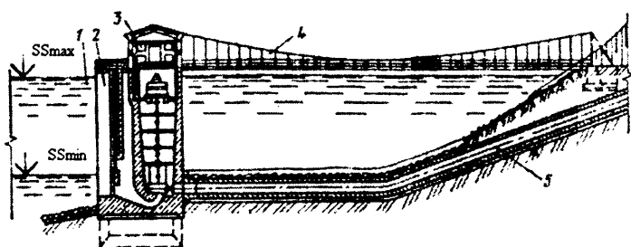
8.5-rasm. Daryo o'zanidagi birlashgan nasos stansiya tasviri: 1-manba; 2-suv olish inshooti; 3-nasos stansiya binosi; 4-ko'pirik; 5-bosimli quvur.
