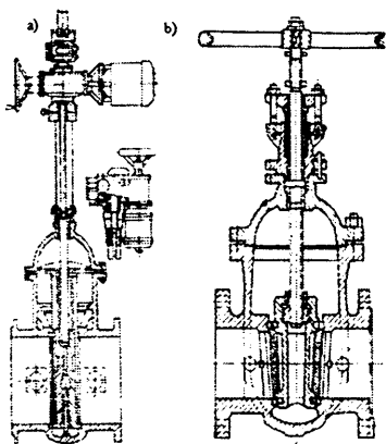
12.5 - rasm. Surilma qulfaklar: a-harakatlanuvchi shpindelli va elektr uzatmali parallel qulfak; b - harakatlanmaydigan shpindelli va qo'l uzatmali, ponali qulfak.
