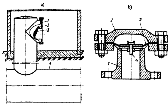
12.10 - rasm. Havo kiritish qopqoqlari:
