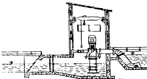
10.11-rasm. Suvga botirilgan o'qiy nasos o'rnatilgan ho'l bo'linmali bino.
