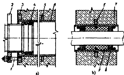
12.13 - rasm. Quvurlarni devoridan o'tkazilishda qo'llaniladigan salnikli zichlagichlar:
