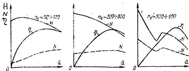
4.5-rasm. Kurakli nasoslarning xarakteristikalari shakllari.
