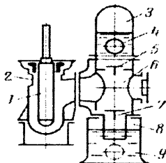
6.2-rasm. Bir tomonlama ishlovchi plunjerli nasos tasviri: 1-plunjer; 2-silindr; 9 va 3-soʻrish va bosimli havo qalpoqlari; 4-bosimli quvur; 7 va 5-soʻrish va bosimli qopqoqlari; 6-ish boʻlinmasi; 8-soʻrish havo boʻlinmasi.
