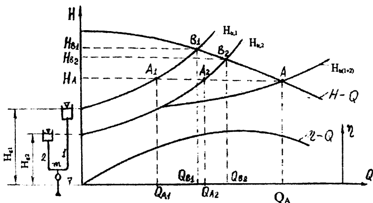
4.14-rasm. Nasosni ikkita quvurga suv uzatishi.
