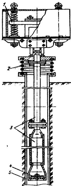
7.7-rasm. Yuzaga oʻrnatiladigan tebranma nasos:
