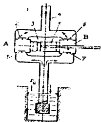
6.2-rasm. Bir tomonlama ishlovchi plunjerli nasos tasviri: 1-plunjer; 2-silindr; 9 va 3-soʻrish va bosimli havo qalpoqlari; 4-bosimli quvur; 7 va 5-soʻrish va bosimli qopqoqlari; 6-ish boʻlinmasi; 8-soʻrish havo boʻlinmasi.
