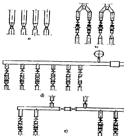
12.2-rasm. O'qiy va gorizontall valli markazdan qochma nasoslar o'rnatiladigan nasos stansiyalarining bosimli kommunikatsiyalari: a – o'qiy nasoslarning quvurlari; b, d, e - gorizontall markazdan qochma nasoslarni ikkita quvurga, berk sug'orish tarmog'iga, suv ta'minoti tarmog'iga suv uzatishi.
