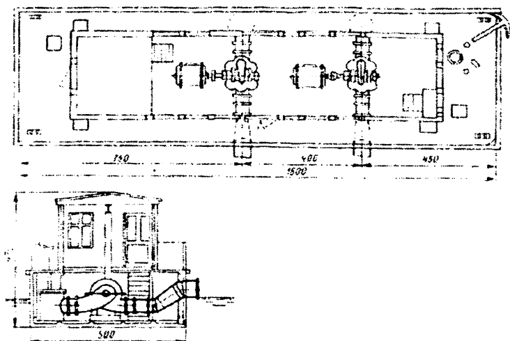
10.21-rasm. Suzuvchi nasos stansiyasi
