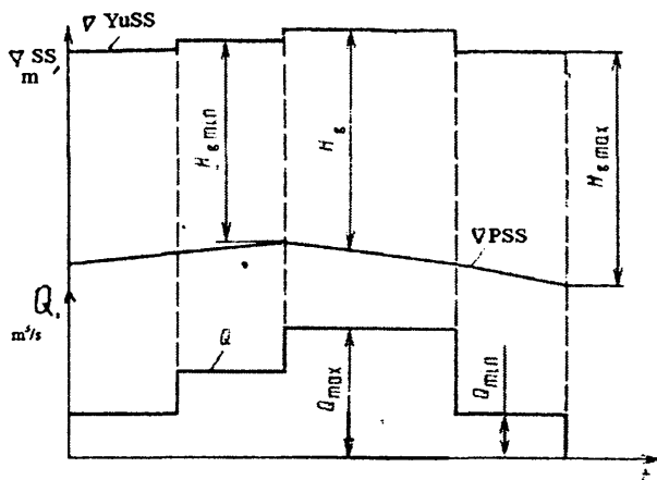
9.1- rasm. Nasos stansiyaning suv uzatish Q = f(t) hamda yuqori va pastki beflarida suv sathlarini yil davomida o'zgarish grafiklari
