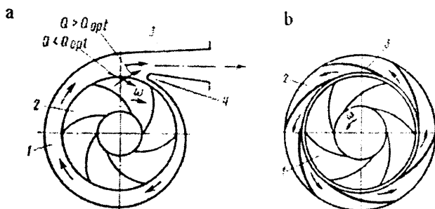
2.19-rasm. Nasoslarning olib ketish moslamalari tasvirlari:
