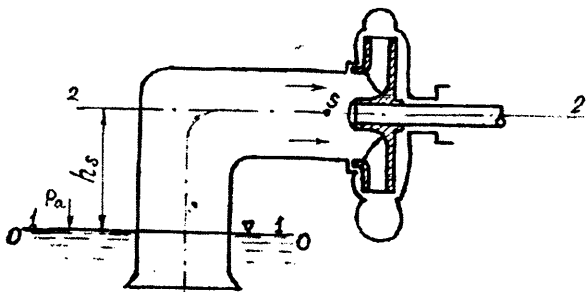
3.8-rasm. Nasosning so‘rish balandligini aniqlash tasviri.
