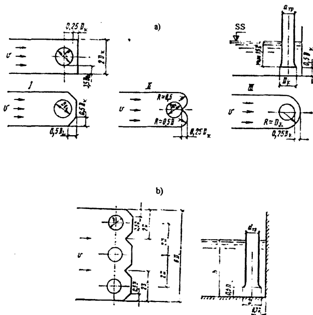
11.9- rasm. So'rish quvurlarini suv qabul qilish bo'linmalariga joylashtirish (Britaniya gidromexanik tadqiqotlari assotsiatsiyasi tavsiyalari bo'yicha):
