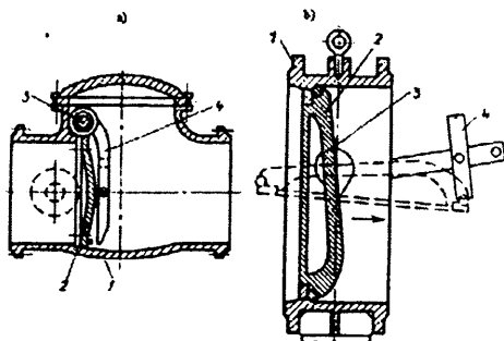
12.11 - rasm. Teskari qopqoqlar:
