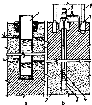
8.13-rasm. Yer osti manbalaridan suv olish qurilmalari:
