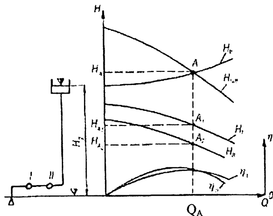
4.13-rasm. Ikkita nasosning ketma-ket ishlashi.
