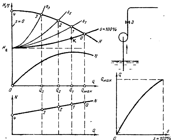
4.7-rasm Nasosning suv uzatishini qulfak bilan rostlash.
