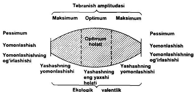
3-rasm. Ekologik omillarning ta'sir qilish nuqtalari (Kultiasov, 1982)
