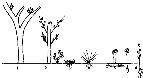
10-rasm. Raunkiye bo'yicha o'simliklarning hayotiy formalari
