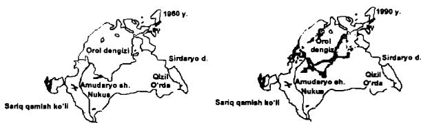
30-rasm. Orol bo'yida 1960 va 1990-yillar ichida galomorf landshaftlar (Qora rang)ning tarqalishi (Popov, 1998-yil)
