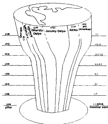
28-rasm. Yer yuzida insonlar sonining o'sish diagrammasi
