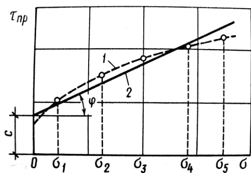
2.11-rasm. Changsimon-loyli grunt namunalarining siljishga qarshilik grafigi: 1 – sinov egri chizig'i; 2 – rostlangan grafik.
