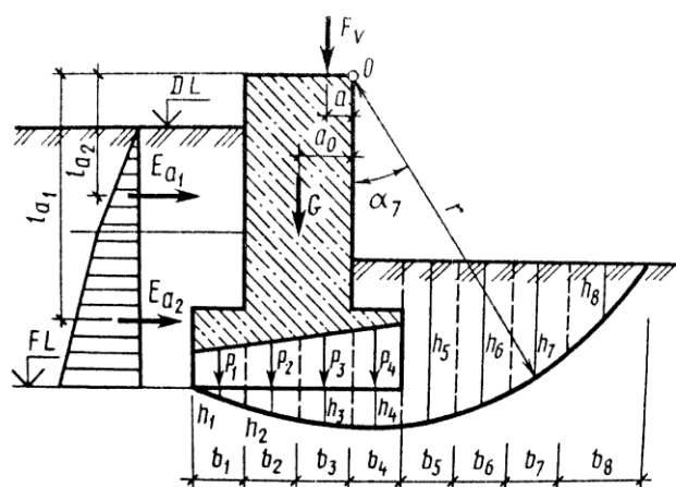
4.7-rasm. Poydevorning turgʻunligini yumaloq-silindrsimon sirpanish yuzasi usuli bilan hisoblashga doir sxema.
