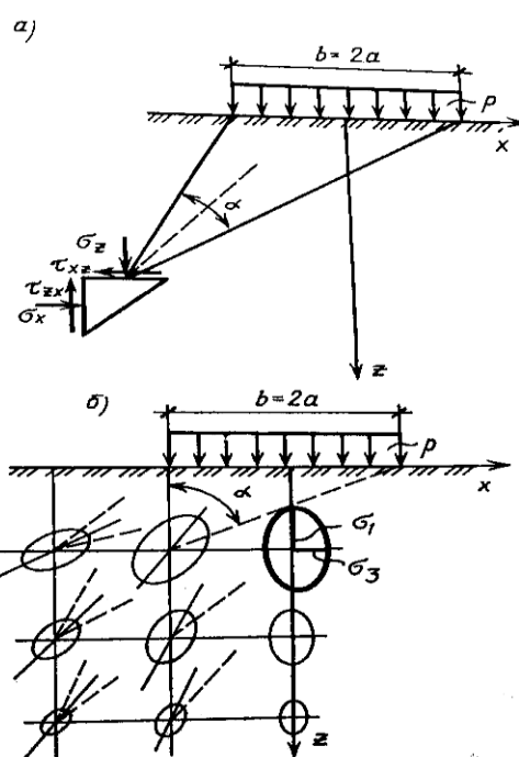
3.6-rasm. Tekis masala holatida zo'riqlarni hisoblash uchun sxema (a); zaminda zo'riqlar ellipslarining joylashuvi (b)
