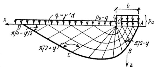
4.4-rasm. Vaznsiz ( \gamma=0 ) zamin uchun chegaraviy qo'shimcha yuk tushgan holda sirpanish chiziqlari
