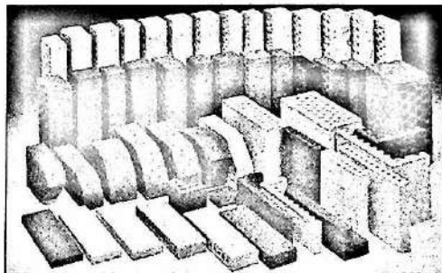
3.5-rasm. Kovakli g'isht va toshlar.
