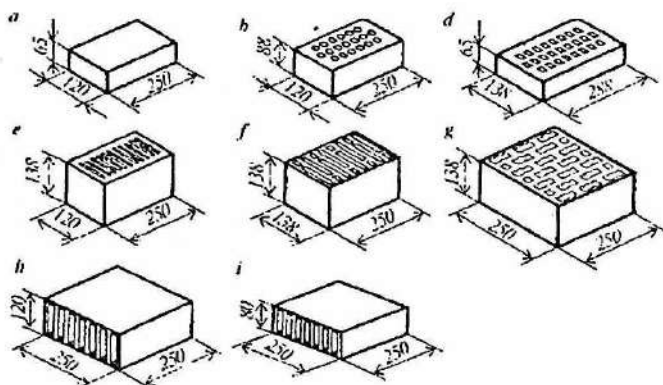
3.4-rasm. Keramik g'isht turlari.
