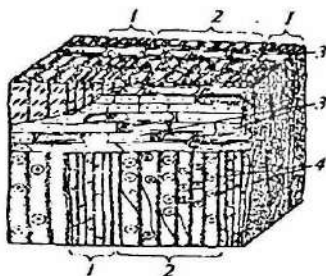
13.2-rasm. Qarag'ay yog'ochi mikrostrukturasi.
