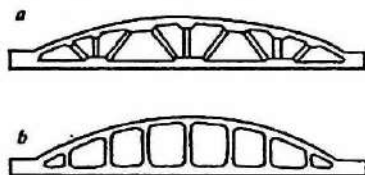
7.5-rasm. Yopmalarining segmentli (a) va qiya kergisiz (b) temirbeton fermalar.
