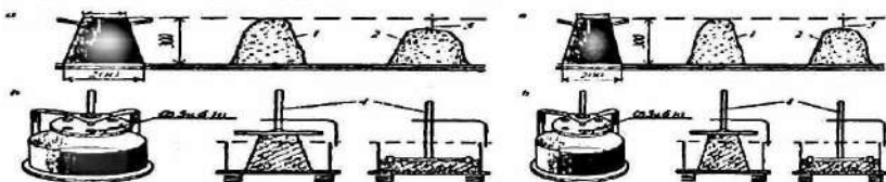
6.1-rasm. Beton qorishmasining qulay joylanuvchanligini aniqlash.
