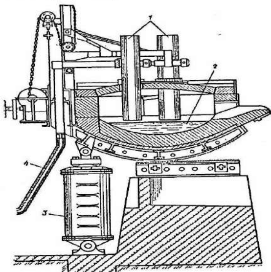
10.10-rasm. Voysimon elektr pechi sxemasi.
