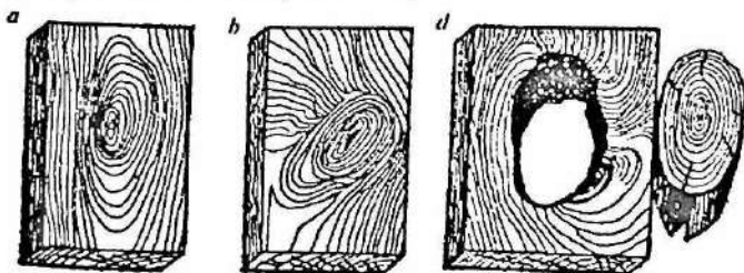
13.3-rasm. Yog'och ko'zlarining turlari.
