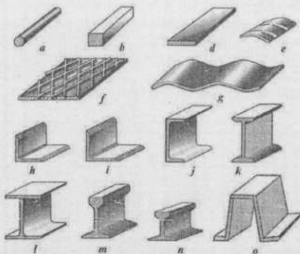
8.8-rasm. Po'lat navlari: a-dumaloq; b-kvadrat; d-tasmasimon; e-takroriy uzun; f-taram-taram; g-to'liqinli; h-teng burchakli; i-tengsiz; j-shveller; k-dvutavr; l-payvandlangan dvutavrli; m-temir yo'l izi (rel'si); o-devorbop shpunt.
