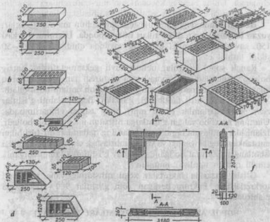
4.3-rasm. Devorbop sopol ashyolarning asosiy xillari: a, b — oddiy va samarali g'ishtlar; d — fasadbop kalibrlangan g'isht; e — bo'shliqli sopol g'isht va tosh; f — ikki qatlamli tashqi devorbop panel.
