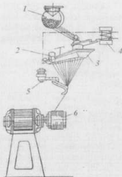
5.4-rasm. Shisha tolasini uzluksiz tortish usuli bilan ishlaydigan qurilma sxemasi: 1—shisha donalarini qabul qiluvchi chomich; 2—avto- matika uskunasi; 3—elektr o'chog'i; 4—transformator; 5—tolani moylovchi uskuna; 6—g'altak.
