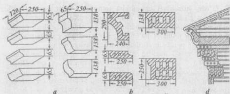
4.6-rasm. Profilli devor yuzasibop g'ishtlar va qismlar: a, b — ko'rinish, d — ishlatilishi.
