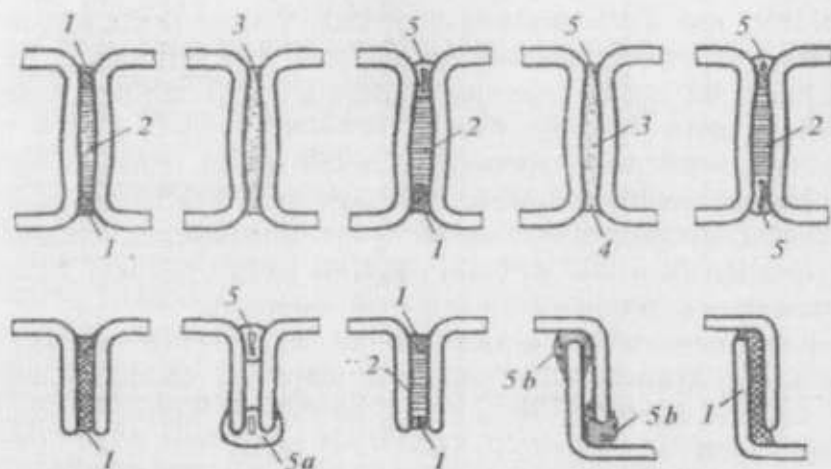
5.6-rasm. Biriktirilgan profilni shisha buyumlarining turi va shakli: 1-hermetik; 2-prokladka; 3-qorishma; 4-mastika; 5-profilni prokladka.
