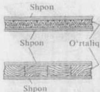
2.21-rasm. Duradgorlik plitalari.
