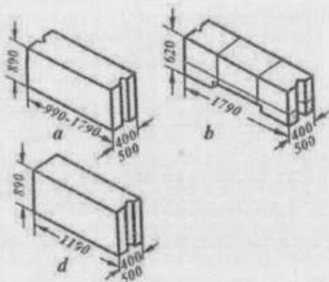
3.13-rasm. Tabiiy tosh buyumlarning xillari. a -chorqirra tosh; b -yo'nilgan; d -to'sinbop.
