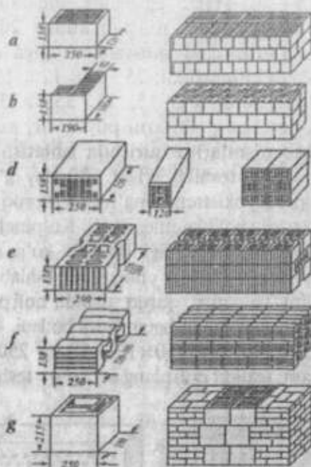
4.4-rasm. Yirik kovakli toshlar va ulardan devor terish: a — G-simon; b — kovaklari turlicha bo'lgan devorbop tosh; d — kovaklari tik yo'nalgan tosh bilan devor terish; e — gorizontal kovakli tosh bilan devor terish; f — shamollatish va gaz uzatish uchun mo'ljallangan tosh. g — mo'ribop sopol g'isht.
