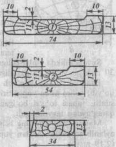
2.17-rasm. Chaspaklar (doura ichidagi raqam chaspak tipini bildiradi).
