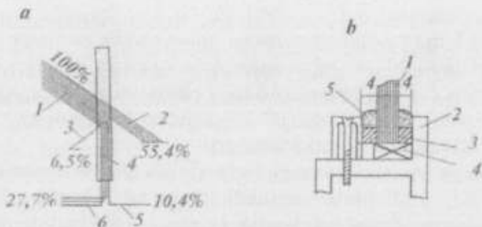
5.5-rasm. Shishaning issiqlikni yutishi. a -quyosh nurining o'tish sxemasi; 1-quyoshdan kelayotgan issiqlik manbai; 2-shishadan o'tgan issiqlik manbai; 3-qaytarilgan issiqlik manbai; 4-yutilgan issiqlik manbai; 5-xonadagi ikkilamchi radiatsiya; 6-tashqaridagi ikkilamchi radiatsiya. b -issiqlikni yutuvchi taxta oynani romga o'rnatish sxemasi; 1-issiqlikni yutuvchi shisha; 2-rom; 3-tayanch va chokbop yostiqcha; 4-g'ovak rezina; 5-qotmaydigan bo'tqa.
