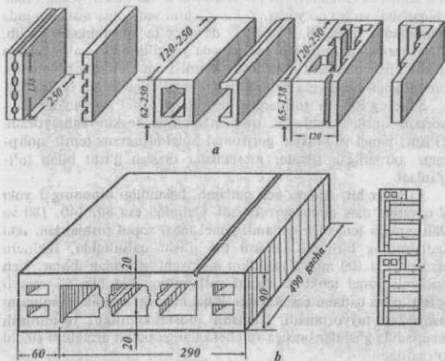
4.7-rasm. Fasadbop qoplama sopol plitkalar: a-kichik o'lchamli plitkalar; b-yirik sopol plitka.
