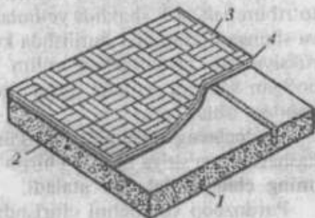
2.20-rasm. Паркет пол: 1-бетонли zamin; 2-mastika; 3-parket taxtachalar; 4-sementli suvoq.
