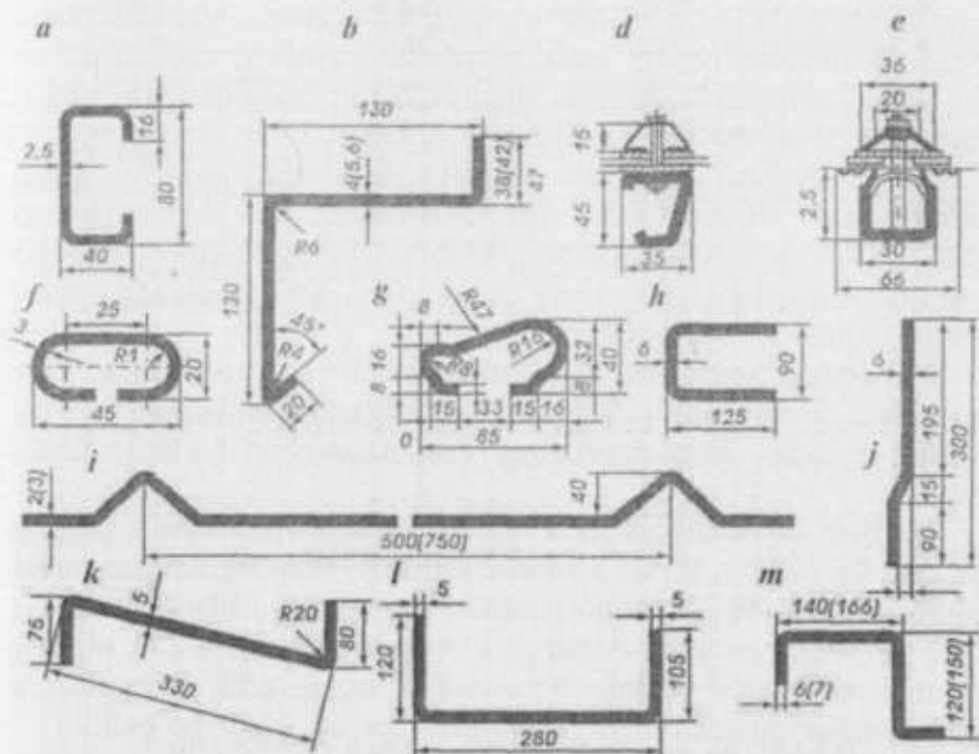
8.9-rasm. Bukilgan uzun po'lat buyumlar: a, b, d — yuk ko'taruvchi konstruksiyalar; e, f — derazabop; g — zinapoya tutqichi; h — rezervuarbop; i, j, k, l, m — yaroqli temir buyumlar.
