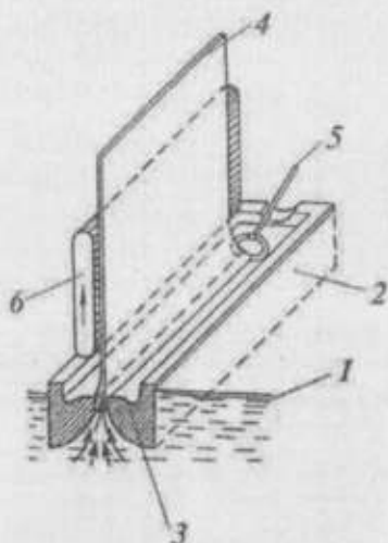
5.2-rasm. «Qayiq» usuli bilan shisha bo'tqasini uzluksiz tortib oynabop taxtalar olish sxemasi: 1—erigan shisha bo'tqa; 2—«Qayiq»; 3—shisha bo'tqasini so'rish sxemasi; 4—oynabop shisha taxta; 5—qisqich; 6—sovutkich.
