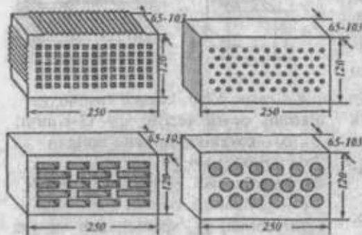
4.5-rasm. Ko'p teshikli g'ishtlar.
