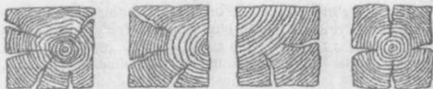
2.11-rasm. To'sinning tez qurishi natijasida yorilishi.
