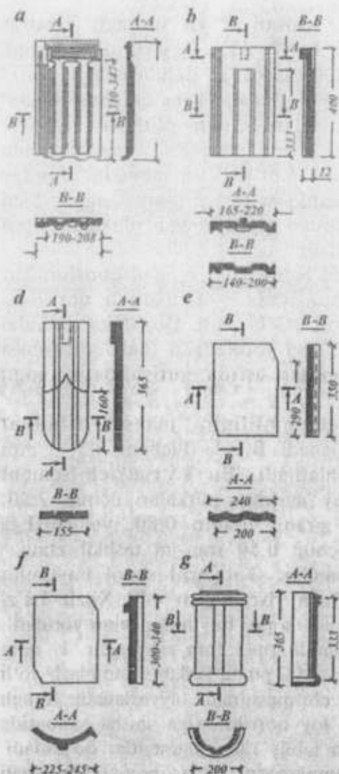
4.12-rasm. Tombop rangli sopol cherepitsa: a—ariqcha o'yiqli; b—ariqchali; d—tekis; e—to'liqli; f—shakli; g—yarim doirali.
