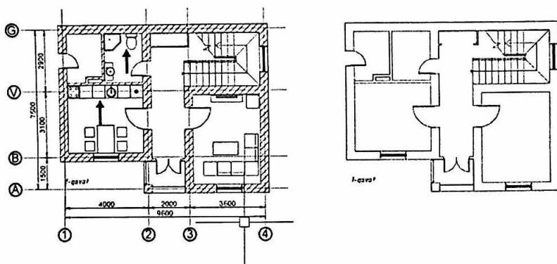
6-rasm. 1-qavat tarh eskizi.
