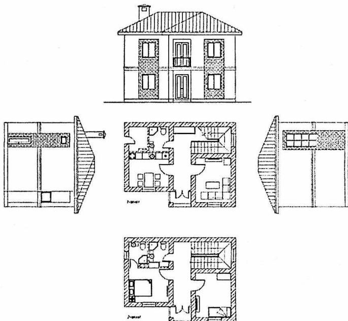
1-rasm. Binoning eskiz chizmasi.
