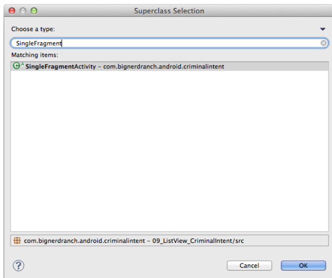
Рис. 9.4. Выбор SingleFragmentActivity
