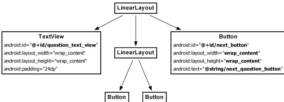
Рис. 2.6. Новая кнопка
