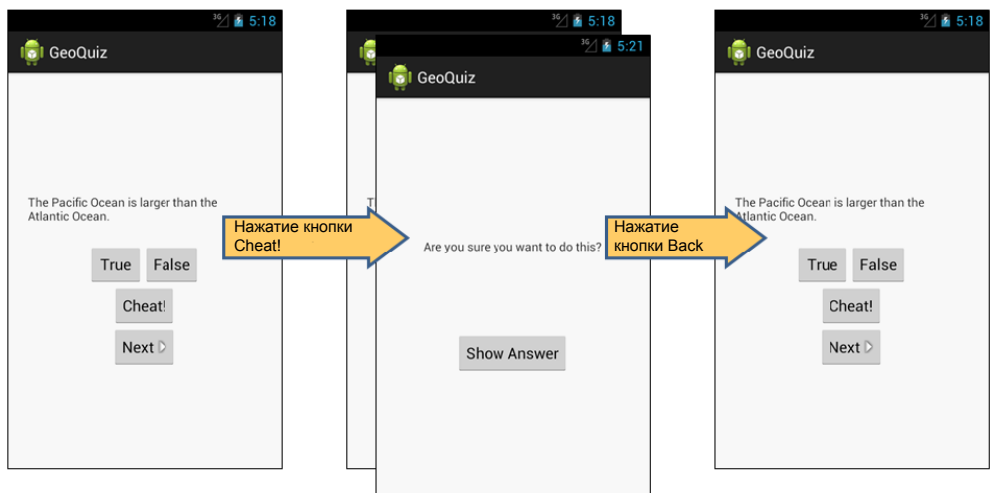
Рис. 5.13. Стек GeoQuiz
