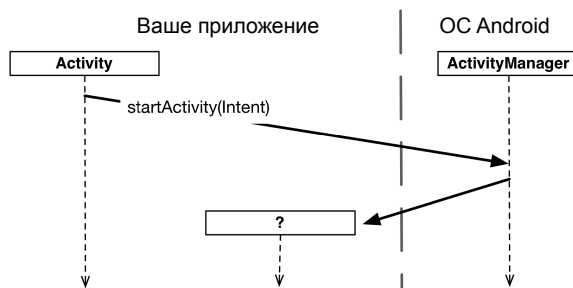
Рис. 5.8. Запуск активности
