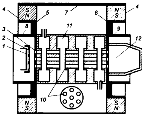
Рис. 9.12 Конструктивная схема многолучевого четырёхрезонаторного клистропа
