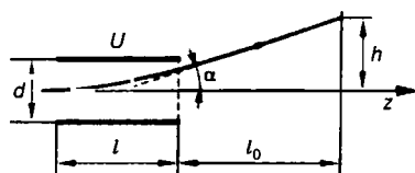
Рис. 7.21 Квазиэлектростатическое отклонение электронного луча
