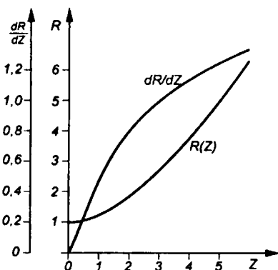
Рис. 5.30 Универсальные кривые для расчета огибающей аксиально- симметричного пучка
