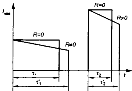
Рис. 8.3 Импульсы наведенного тока
