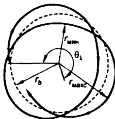
Рис. 6.7 Проекция электронной траектории на плоскость r\theta для потока типа бриллюэновского ( B_K = 0 ) при относительных пульсациях r_m/r_b = 0,2
