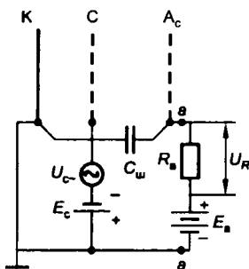
Рис. 7.9 Триодное устройство с анодной нагрузкой
