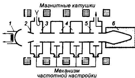
Рис. 9.9 Многорезонаторный пролетный усилительный клистрон
