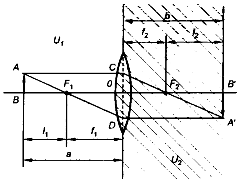
Рис. 4.2 Построение изображения в тонкой линзе
