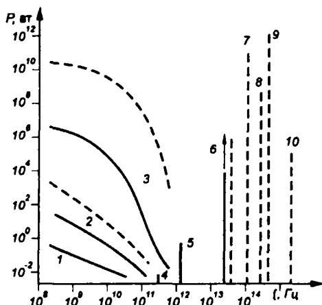
Максимальные уровни мощности СВЧ-приборов и отдельных приборов квантовой электроники
