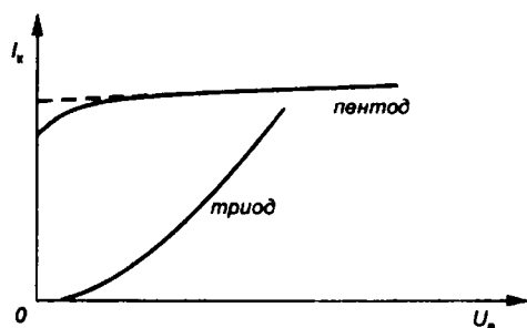
Рис. 3.24 Сравнение форм характеристик I_k = f(U_a) триода и пентода
