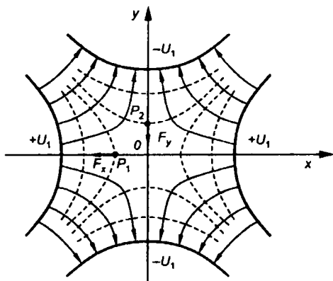
Рис. 4.33 Квадрупольная электростатическая линза
