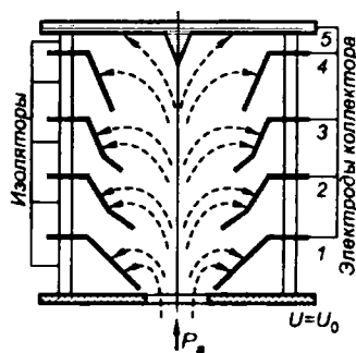
Рис. 8.17 Конструкция 5-ступенчатого коллектора-рекуператора
