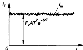
Рис. 2.13 Флуктуация эмиссионного тока термокатада
