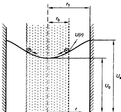
Рис. 5.36 Потенциальная яма, являющаяся ловушкой для положительных ионов
