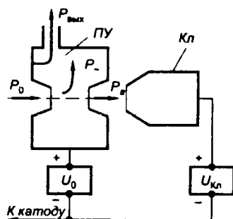
Рис. 8.15 Микроволновое преобразующее устройство с коллектором
