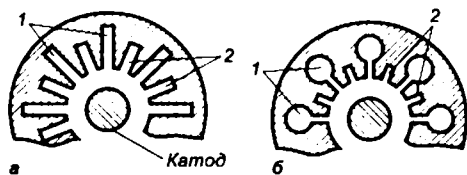
Рис. 9.27 Примеры устройства разнорезонаторных анодных блоков
