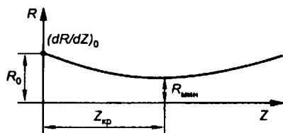
Рис. 5.29 К расчету огибающей аксиально-симметричного пучка
