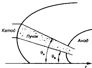
Рис. 5.17 Половина сечения пушки, формирующей полый конический пучок
