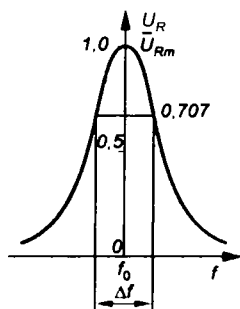
Рис. П.2 Резонансная кривая колебательного контура
