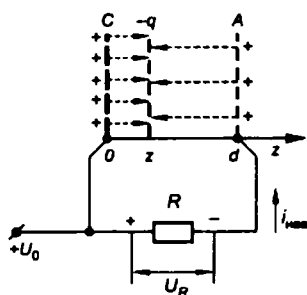
Рис. 8.2 Упрощенная схема диодного преобразующего устройства
