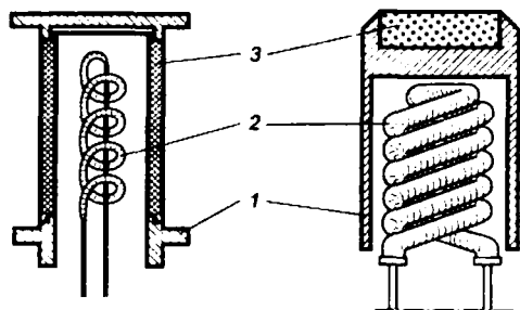
Рис. 2.19 Конструкции подогревных импрегнированных катодов
