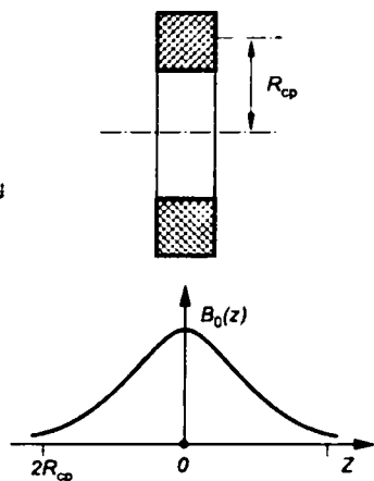
Рис. 4.19 Короткая магнитная катушка и распределение магнитной индукции на оси
