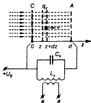
Рис. 8.1 Схема преобразующего устройства
