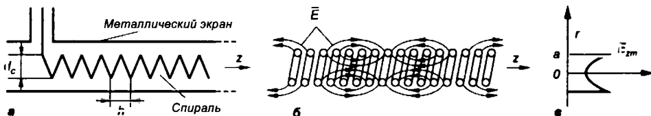
Рис. 7.40 Спиральная замедляющая линия
