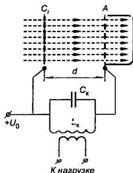
Рис. 8.7 Преобразующее устройство с камерным анодом
