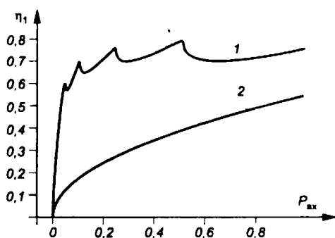
Рис. 9.6 Зависимость КПД ЛИВ от входной мощности
