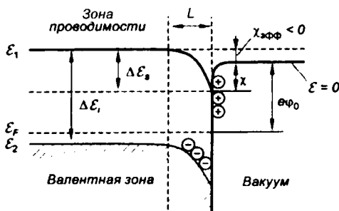
Рис. 2.29 Искривление энергетических уровней в приповерхностной области полупроводника p -типа
