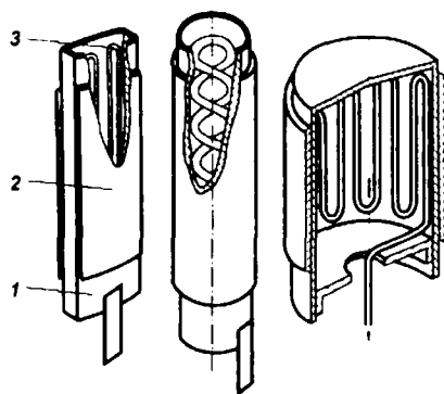
Рис. 2.22 Конструкции подогревных оксидных катодов с алундированными подогревателями
