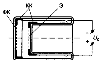
Рис. 1.11 Схема электронно-оптического преобразователя
