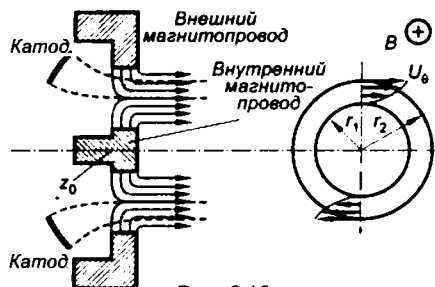
Рис. 6.12 Формирование трубчатого пучка в продольном магнитном поле
