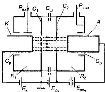
Рис. 9.1 Схема тетродного УВЧ-усилителя
