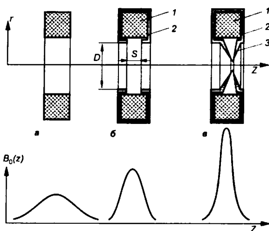
Рис. 4.21 Типы тонких магнитных линз
