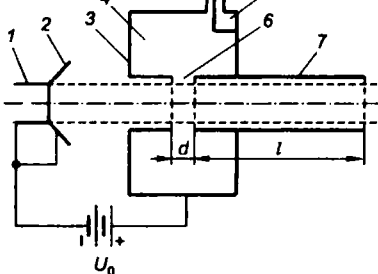
Рис. 7.24 Схема клистронного управляющего устройства
