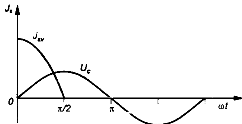
Рис. 7.17 Кривые плотности катодного тока и управляющего напряжения
