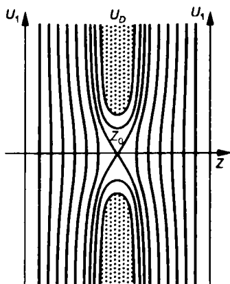
Рис. 4.5 Электрическое поле плоской диафрагмы
