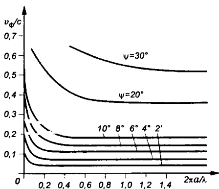
Рис. 7.41 Дисперсионные характеристики спиральной замедляющей системы при различных углах намотки спирали
