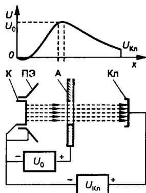
Рис. 8.13 Электронно-лучевое устройство с рекуперацией энергии электронов
