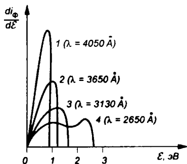
Рис. 2.27 Кривые распределения фотоэлектронов по энергиям
