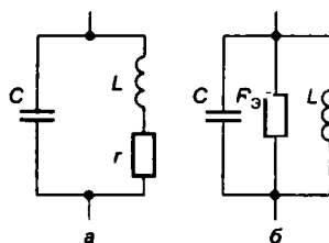
Рис. П.1 Эквивалентные схемы резонансного контура
