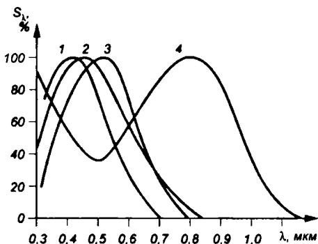
Рис. 2.30 Спектральные характеристики различных фотокатодов
