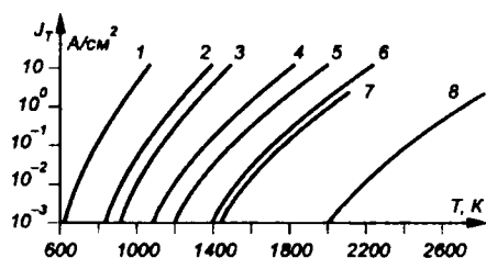
Рис. 2.20 Расчетные характеристики различных термокатодов
