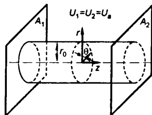
Рис. 6.22 Цилиндрический аксиально-симметричный электронный пучок
