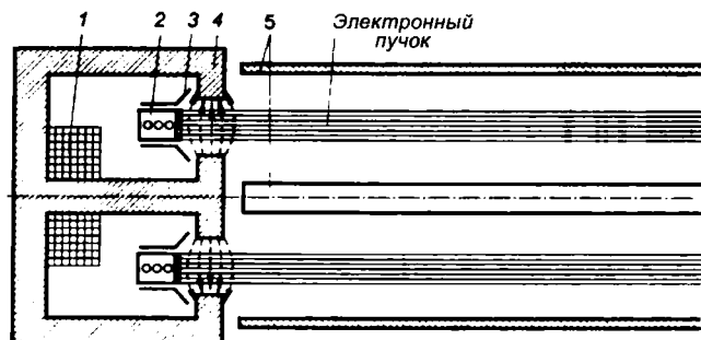
Рис. 6.33 Центробежно- электростатическая система со спиральной пушкой
