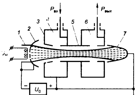
Рис. 9.7 Схема двухрезонаторного усилительного клистрона
