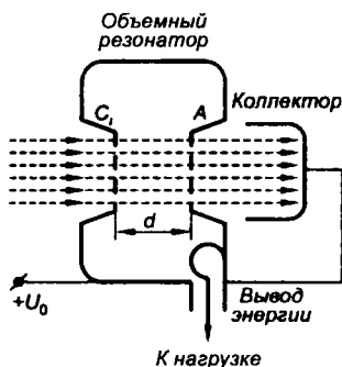
Рис. 8.8 Преобразующее устройство с объемным резонатором
