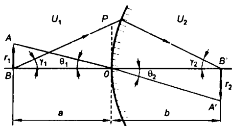
Рис. 4.4 К выводу условия Лагранжа–Гельмгольца
