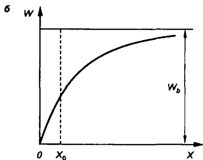
Рис. 2.4 Изменение электрических сил и потенциальной энергии электрона на границе металл-вакуум
