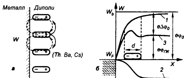
Рис. 2.12 Диполи атомов электроположительного вещества на поверхности металла и их влияние на потенциальный барьер
