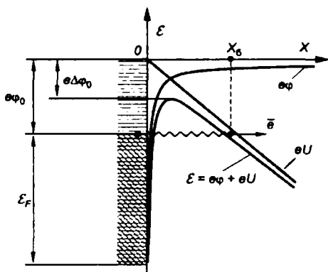
Рис. 2.24 Сужение поверхностного потенциального барьера под действием сильного электрического поля
