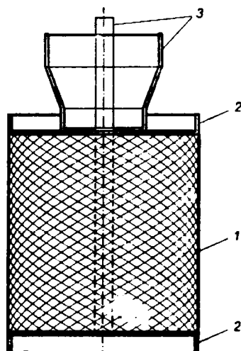
Рис. 2.16 Прямонакальный решетчатый катод
