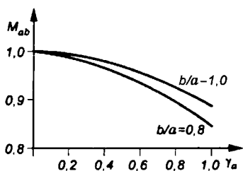
Рис. 7.27 График функции M_{ab}(\gamma a, b/a)
