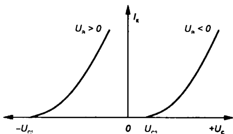
Рис. 3.20 Катодно-сеточные характеристики триода
