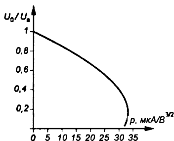
Рис. 5.35 Зависимость потенциала на оси пучка от микропереванса
