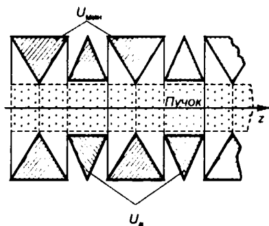
Рис. 6.24 Упрощенная форма электродов системы периодической фокусировки
