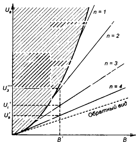
Рис. 9.29 Парабола критического режима
