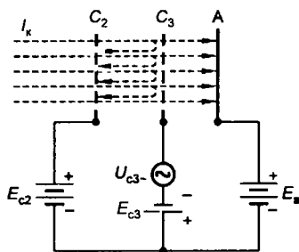
Рис. 7.13 Схема управления токопрохождением
