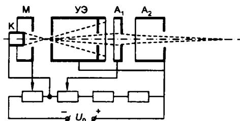
Рис. 4.42 Электронный прожектор с одиночной проекционной линзой
