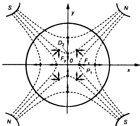
Рис. 4.35 Квадрупольная магнитная линза
