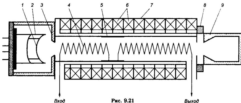
Рис. 9.21 Двухсекционная ЛБВО с МПФС
