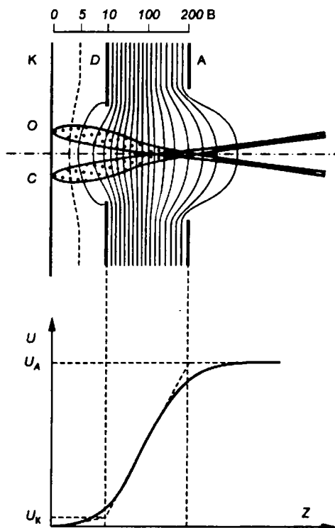
Рис. 4.17 Схема триодного иммерсионного объектива и кривая распределения потенциала на его оси
