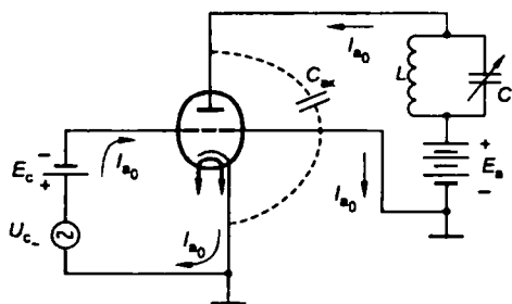
Рис. 1.9 Схема триодного усилителя с общей точкой на сетке
