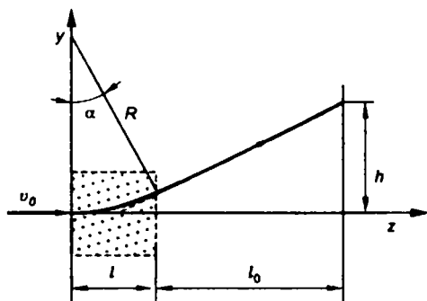
Рис. 7.23 Магнитное отклонение электронного луча
