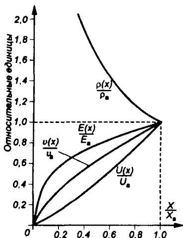
Рис. 3.7 Распределение потенциала U(x) , напряженности электрического поля E(x) , скорости электронов v(x) и плотности пространственного заряда \rho(x)
