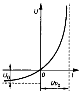
Рис. 7.35 Идеальная форма кривой модулирующего напряжения
