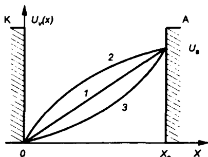
Рис. 3.2 Распределение потенциала в «холодных» диодах
