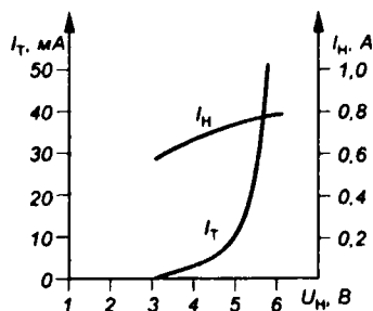
Рис. 2.14 Характеристики термокатода
