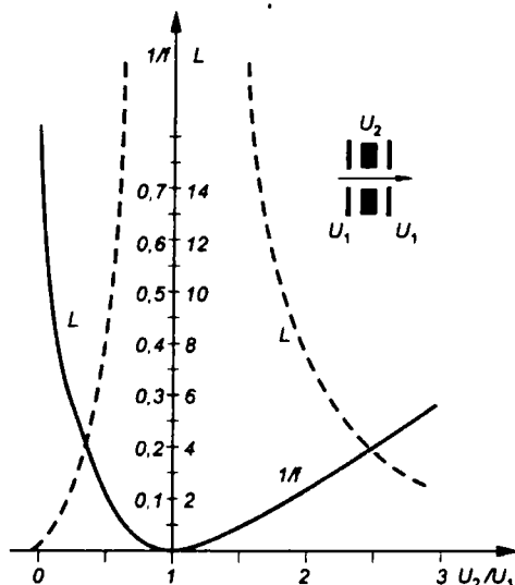
Рис. 4.11 Зависимости оптической силы и положения главного фокуса одиночной линзы от соотношения потенциалов ее электродов
