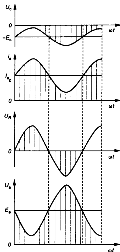
Рис. 1.4 Графики переменных величин в триодном усилителе
