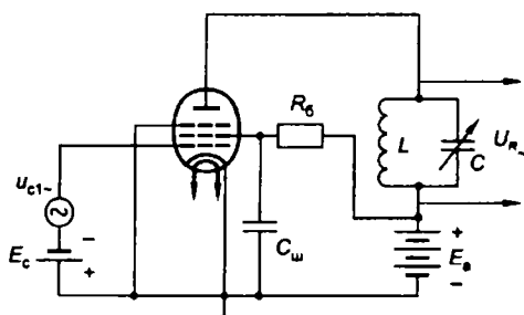
Рис. 1.8 Схема пентодного усилителя
