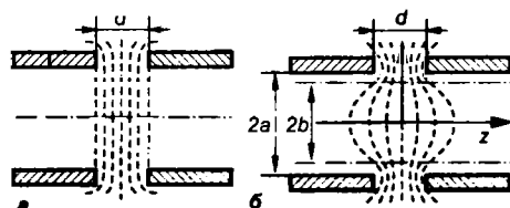
Рис. 7.25 Конструкции высокочастотных зазоров резонаторов
