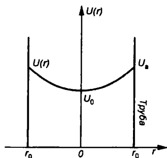
Рис. 5.33 Радиальное распределение потенциала
