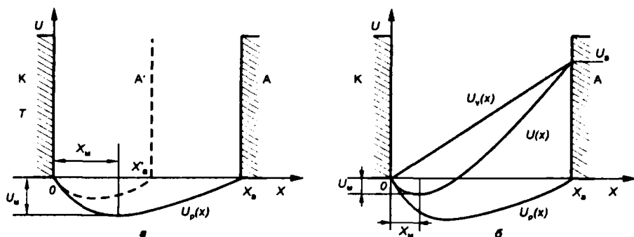
Рис. 3.3 Распределение потенциала в «горячем» плоском диode
