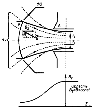
Рис. 6.2 Магнитные потоки в области пушки
