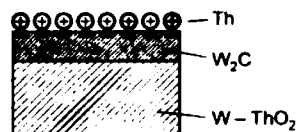
Рис. 2.15 Структура плечного торированного карбидированного вольфрамового катода
