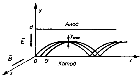
Рис. 4.37 Фокусировка электронов в скрещенных полях
