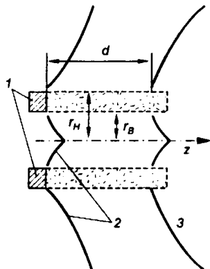
Рис. 5.16 Геометрия пушки, формирующей параллельный трубчатый электронный пучок
