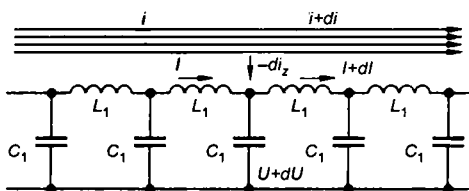
Рис. 8.11 Эквивалентная схема спиральной замедляющей системы с электронным потоком
