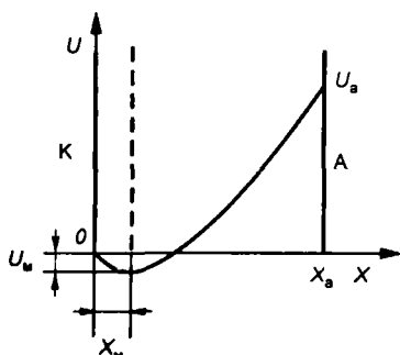
Рис. 3.8 Распределение потенциала в плоском диоде
