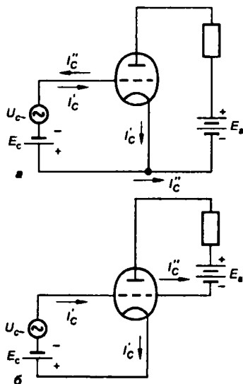
Рис. 8.5 Схемы триодных усилителей
