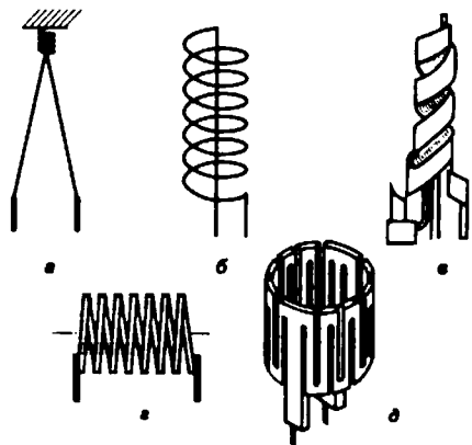
Рис. 2.21 Конструкции прямонакальных термокатодов
