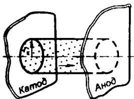
Рис. 5.6 Схема получения аксиально- симметричного пучка в плоском диоде
