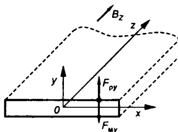
Рис. 6.3 Ленточный электронный пучок в однородном магнитном поле
