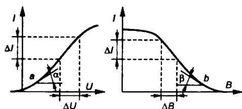
Рис. 7.4 Характеристики управления конвекционным током
