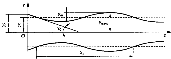
Рис. 6.11 Контур пульсирующего ленточного пучка
