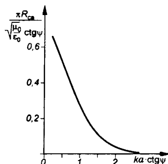
Рис. П.7 К расчету сопротивления связи спиральной замедляющей системы
