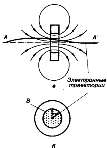
Рис. 4.20 Действие тонкой магнитной линзы
