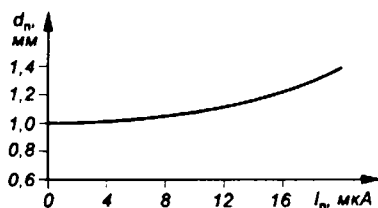
Рис. 4.31 Изменение диаметра электронного пучка в зависимости от его тока
