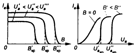
Рис. 9.28 Статические характеристики магнетрона
