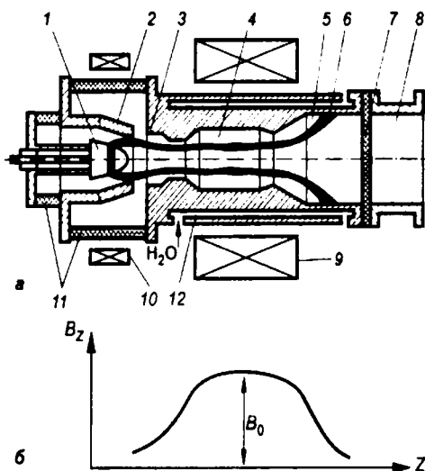
Рис. 9.34 Конструкция гиромонотрона (а) и график распределение индукции (б)
