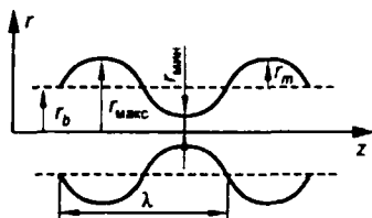
Рис. 6.6 Форма пульсирующего электронного пучка
