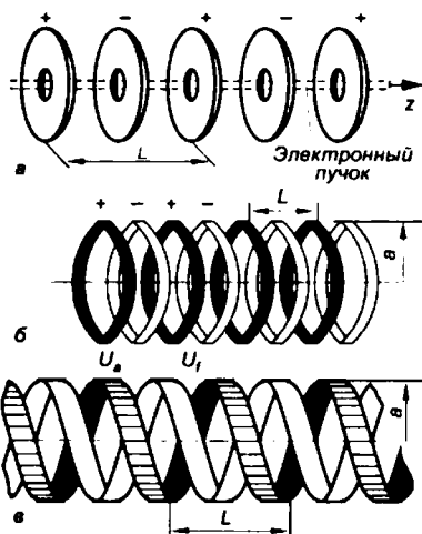
Рис. 6.25 Периодические электростатические системы
