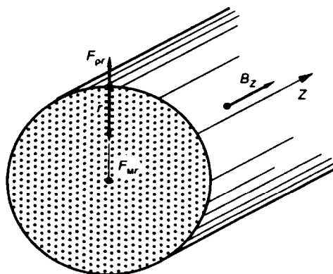
Рис. 6.1 Силы, действующие на аксиально-симметричный электронный пучок в однородном магнитном поле
