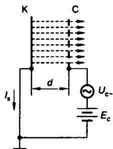
Рис. 7.6 Диодное управляющее устройство
