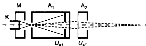
Рис. 4.41 Электронный прожектор с иммерсионной проекционной линзой
