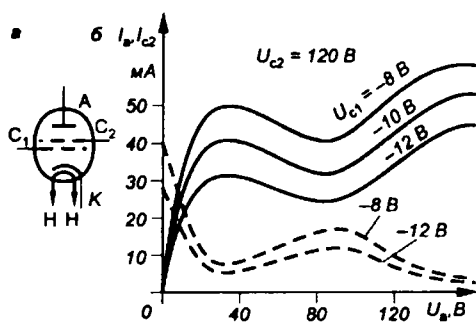
Рис. 1.5 Тетрод (а) и его статические характеристики (б)
