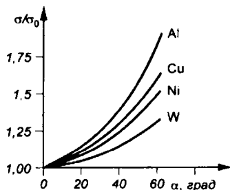
Рис. 2.33 Кривые зависимости коэффициента вторичной электронной эмиссии от угла падения пучка первичных электронов
