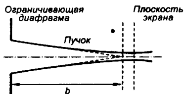
Рис. 4.30 Эффект пространственного заряда
