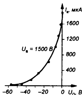
Рис. 3.30 Модуляционная характеристика триодного прожектора
