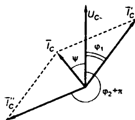
Рис. 8.6 Векторная диаграмма токов, наведенных в сеточной цепи
