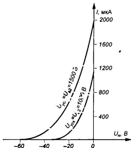
Рис. 4.43 Модуляционные характеристики электронного прожектора с одиночной проекционной линзой
