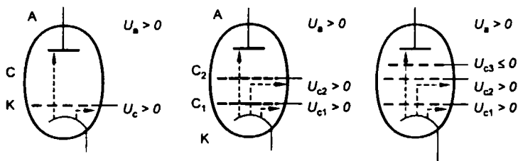
Рис. 3.31 Токораспределение в электронных лампах
