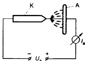
Рис. 2.25 Схема диода с острым катодом
