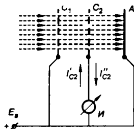
Рис. 8.4 Схема триодного преобразующего устройства
