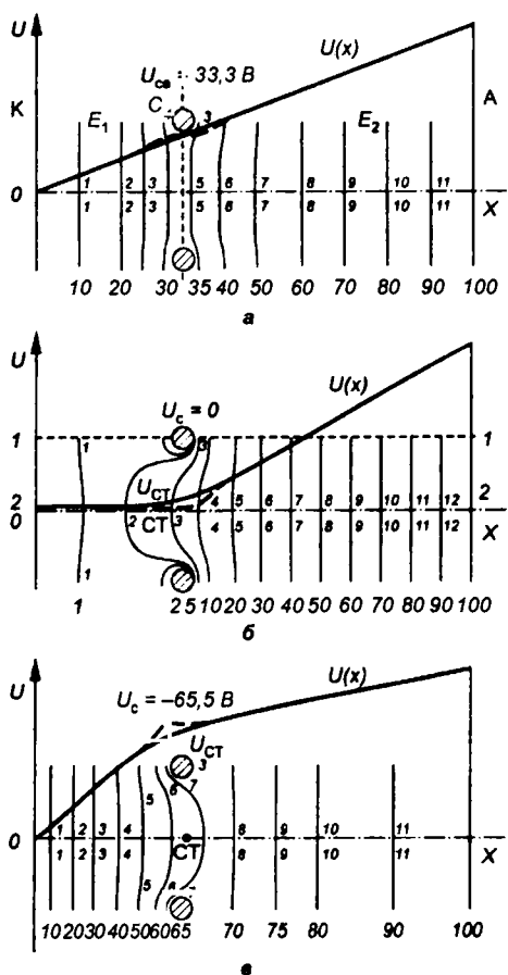
Рис. 3.15 Электростатические поля в плоском триоде
