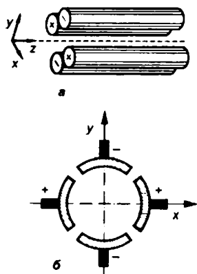
Рис. 4.34 Типы квадрупольных электростатических линз
