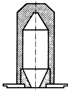
Рис. 8.14 Конструкция коллектора, снижающая выход вторичных электронов
