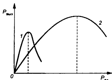
Рис. 9.10 Амплитудная характеристика многорезонаторного усилительного клистрона
