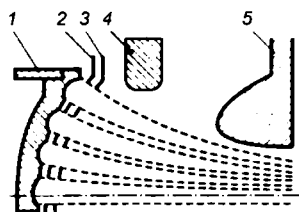
Рис. 5.26 Схема электронной пушки с тневой сеткой
