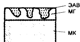
Рис. 2.18 Структура металлогубчатого катода
