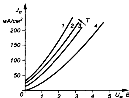
Рис. 3.13 Зависимости плотности катодного тока от анодного напряжения в плоском диоде при разных температурах катода
