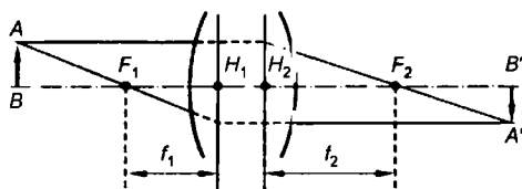
Рис. 4.3 Построение изображения в толстой линзе
