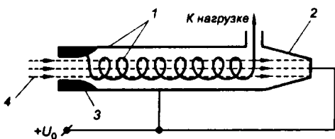
Рис. 8.10 Спиральная преобразующая система с коллектором
