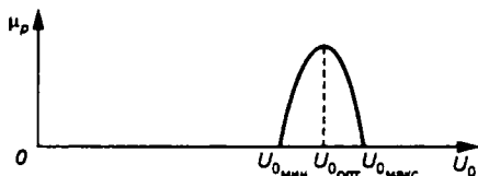
Рис. 9.16 Зависимость коэффициента усиления ЛБВО от ускоряющего напряжения
