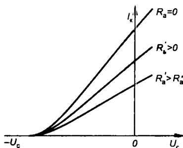
Рис. 7.10 Управляющая характеристика триодного устройства с активной анодной нагрузкой
