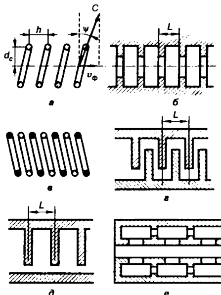
Рис. П.6 Схемы замедляющих систем электронных приборов типа О
