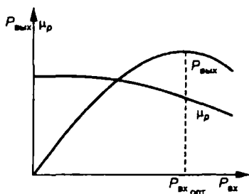
Рис. 9.8 Характеристика усилительного клистрона
