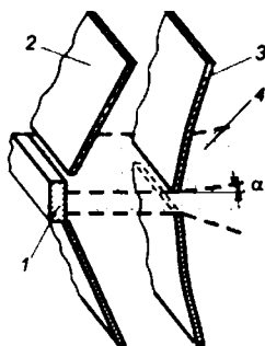
Рис. 5.3 Электронная пушка, формирующая параллельный ленточный пучок
