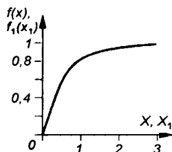
Рис. 3.28 График функций f(x) и f(x_1)
