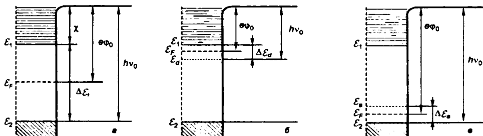
Рис. 2.28 Диаграммы, иллюстрирующие различие фотоэлектронной и термоэлектронной работ выхода в объеме полупроводника
