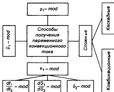
Рис. 7.3 Классификационная диаграмма способов получения переменного конвекционного тока
