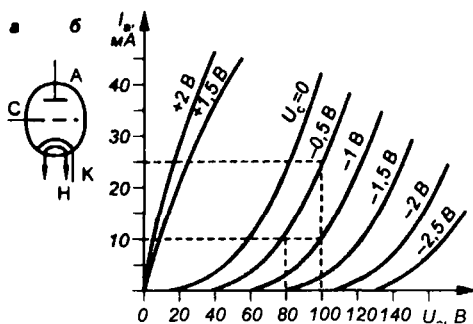
Рис. 1.2 Триод (а) и его статические анодные характеристики (б)
