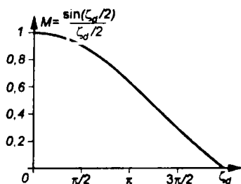
Рис. 7.26 График функции M(\zeta_d)
