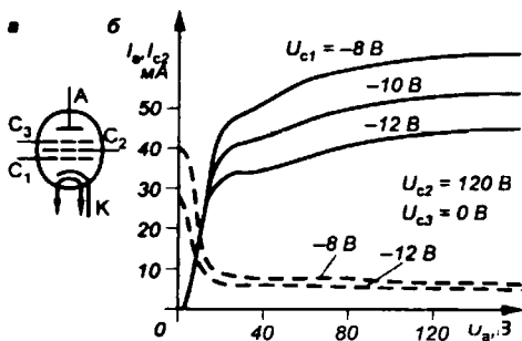
Рис. 1.7 Пентод ( а ) и его статические характеристики ( б )
