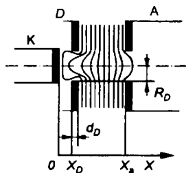
Рис. 3.27 Триодная система с управляющей диафрагмой
