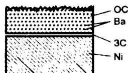
Рис. 2.17 Структура оксидного катода
