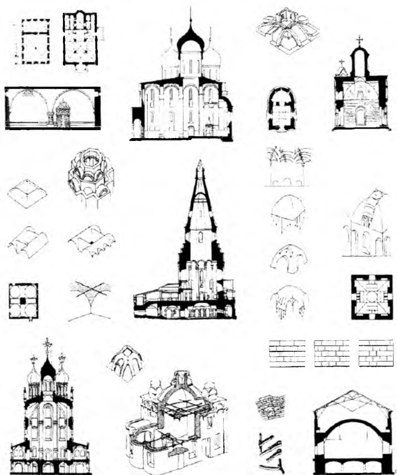
5.16 - rasm. XV–XVII asrlarda Moskva davlati arxitekturasida struktura tiplari va tosh binolar konstruksiyalari
