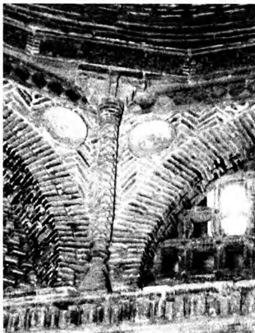
10.14-rasm. Ismoil Somoniy maqbarasining arkalar oraligʻidagi bezakdor gʻishtli konstruksiyasi (sakkiz arkali konstruksiyasining elementlari)
