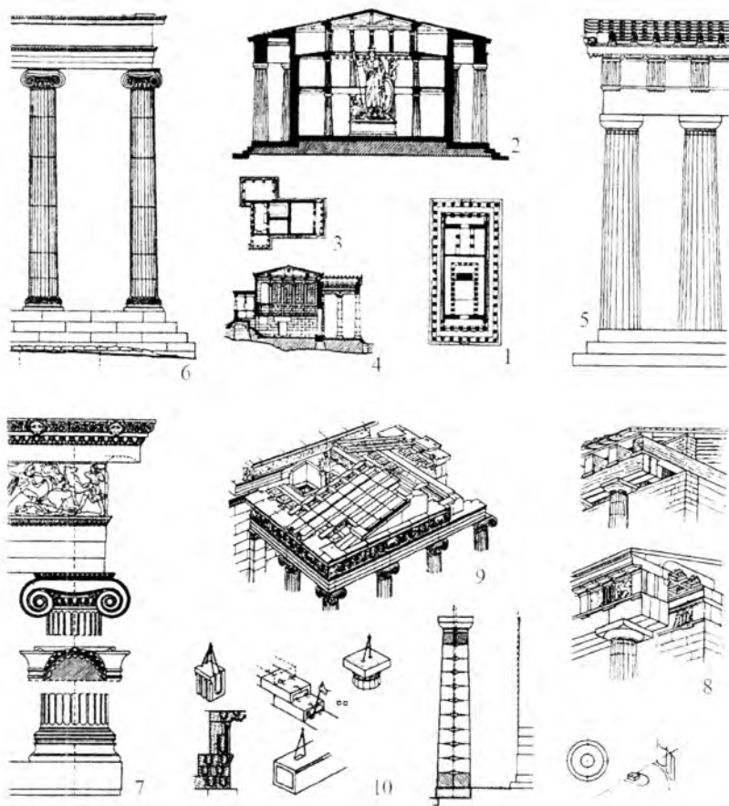
3.6 - rasm. Qadimgi Yunon arxitekturasida konstruksiya va orderlar (tartib). 1, 2 - Parfenon (qizlar uchun xona) ning rejasi va ko'ndalang qirg'imi (teramizdan oldingi 447-438 - yillar); 3, 4 - Erexteyonning rejasi va ko'ndalang qirg'imi (teramizdan oldingi 421 - 406 - yillar); 5 - Parfenonning dorik orderi; 6 - Erexteyonning ionik orderi; 7 - Niki Apteros ibodatxonasining ionik orderi detallari (teramizdan oldingi 449 - 421- yillar); 8 - dorik order va uning yog'och prototipi; 9 - Erexteyonning tom konstruksiyasi; 10 - devor, ustunlarini terish va bloklarini bir - biriga biriktirish
