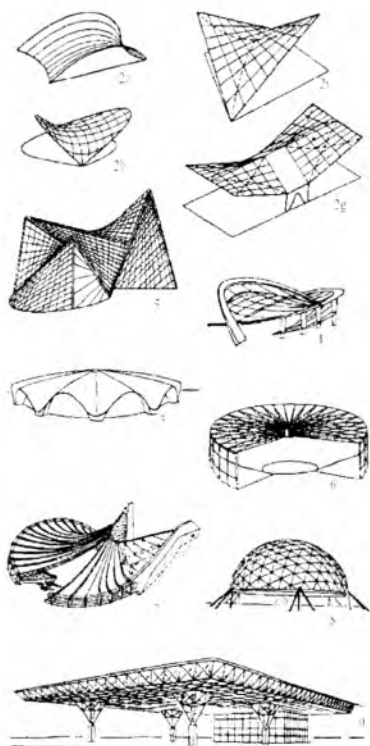
6.6 - rasm. Ikkinchi jahon urushidan so'nggi kapitalistik davlatlar arxitekturasiga misollar : 1 – Parijdagi YUNESKO binosi zalining temirbeton tom yopmasi (1958); 2 (a.b.v.g.)- giparlar asosidagi temirbeton qobiq shakllari; 3- Fransiya-dagi bozorning temirbeton tom yopmasi (1955); 4– AQSh (Rouli)dagi vintli tom yopma (1950–1952); 5- Bryusseldagi ko'rgazma paviloni tom yopmasi (1958); 6- velosiped g'ildiragi shaklidagi tom yopma; 7– Tokiodagi sport zalining vinli tom konstruksiyasi (1964); 8- AQSh ko'rgazma zalining geodezik gumbazi; 9–metall sterjenli tom yopmasi
