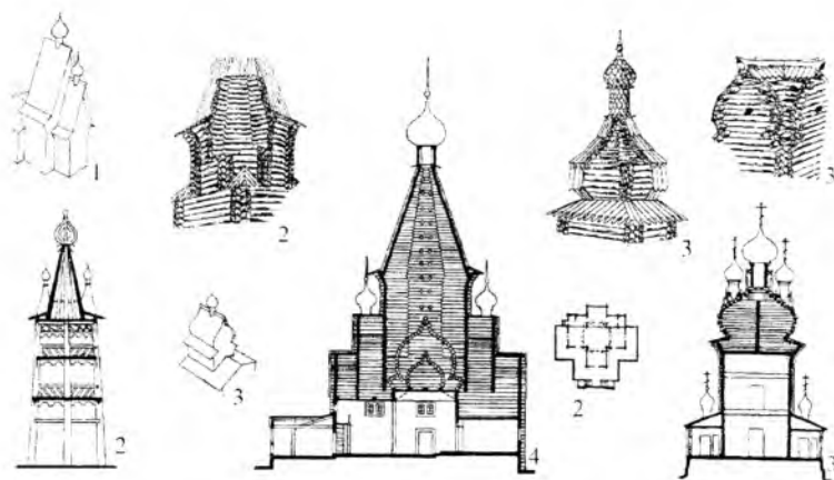
5.14-rasm. Qadimgi rus arxitekturasida yog'ochdan tayyorlangan diniy inshootlarning konstruktiv shakllari. 1-ikki qiyali oddiy cherkov binosi; 2-cherkov va qo'ng'iroq inshootlari; 3-yopma konstruksiyasi bochka va kubsimon bo'lgan cherkov inshootlari; 4-cherkov binosi qirgimi
