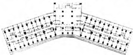
12.12-rasm. «O'zbekiston» mehmonxonasining umumiy ko'rinishi va qavat rejasi (1974-yil)
