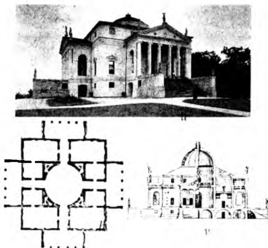
5.4-rasm. Palladio qurilishlari. Rostonda villasi, 1551-yil: umumiy koʻrinish (a), reja (b) va qirqim (v)
