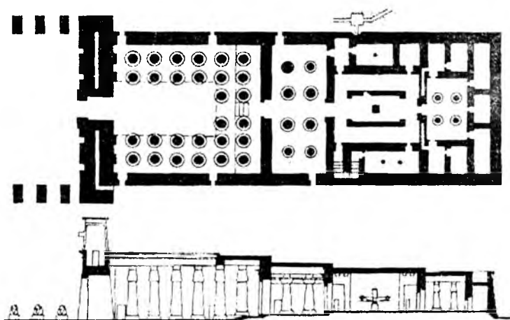
3.4 - rasim. Yangi podsholik davrida qurilgan Karnakdagi Xonsu ibodatxonasi (fasad, reja va qirqim)
