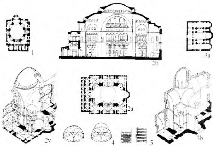
4.1 - rasim. Vizantiya arxitekturasida struktura va konstruksiya turlari.
