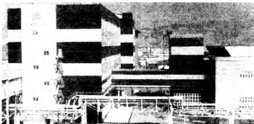
13.12-rasm. «O'zqurilishmateriallar» aksiyadorlik kompaniyasi tarkibiga kiruvchi Quvasoydagi zamonaviy kvars zavodining umumiy ko'rinishi
