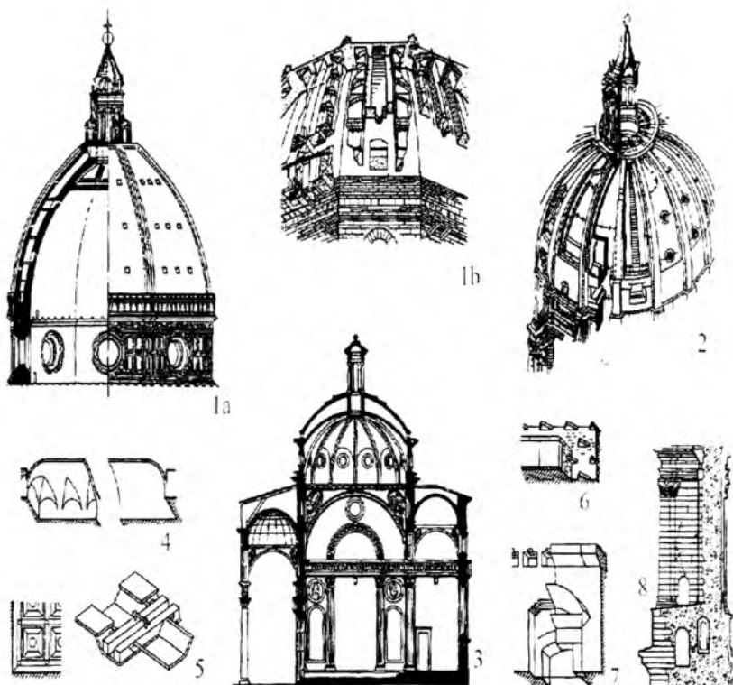
5.1-rasm. Uygʻonish davri arxitekturasiining konstruksiyalari va qurilish usullari. 1 –Florensiyadagi sobor gumbazi (Fore sobori, 1420–1471-yillar); a – qirim va fasad; b – gumbaz konstruksiyasi; 2 – Rimdagi avliyo Pyotr soborining gumbazi (XII asr ikkinchi yarmi); 3 – Florensiyadagi Paststi kapellasi; qirgim; 4 – gumbazlar; 5 – osma shift detallari; 6, 7 – devorlarni pardoiz usullari; 8 – devor boʻshliqlarini beton bilan toʻldirish (avliyo Pyotr sobori)
