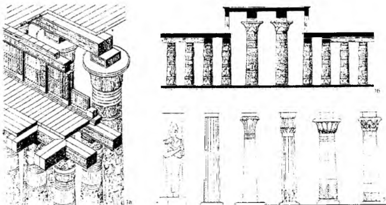
3.1 - rasm . Qadimgi Misrda ustun - to'sin konstruktiv tizimi.
