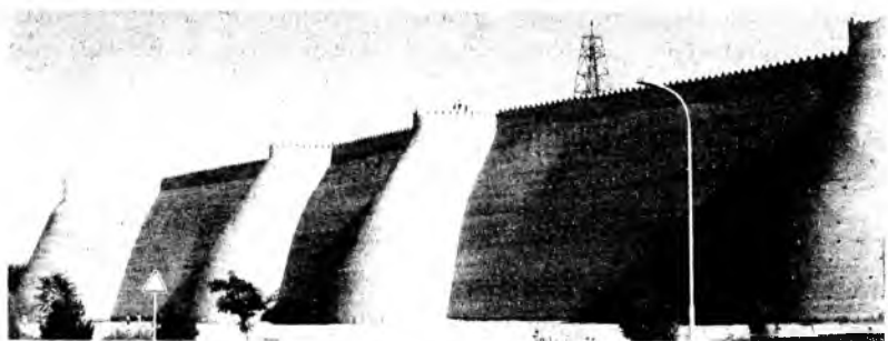
10.9-rasm. Buxoro Arkining mustaqillik davridagi ta'mirlashdan keyingi umumiy ko'rinishi (2007-yil). 1- Ark darvozaxonasi; 2 - sharq tomondagi qo'rg'on devori; 3 - janub tomondagi devor
