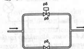
6.3-rasm. Rostlanuvchan va rostlanmaydigan klapanaga ega bo'lgan murakkab rostlovchi organ.
