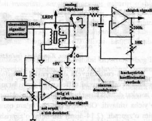
2.15-rasm. Sinusoidal signalni tekislash va shu signalni chiqishda doimiy kuchlanish ko'rinishiga olib keluvchi sinxron demodulyator sxemasi.
