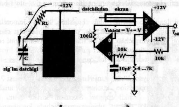
2.32-rasm. a) platada paydo bo'ladigan oqim toki u interfeysni kirish zanjirlarida, tavsifnomalarni o'zgarishiga olib keladi; b) kirish zanjirlarini aktiv ekranlash tushirish.
