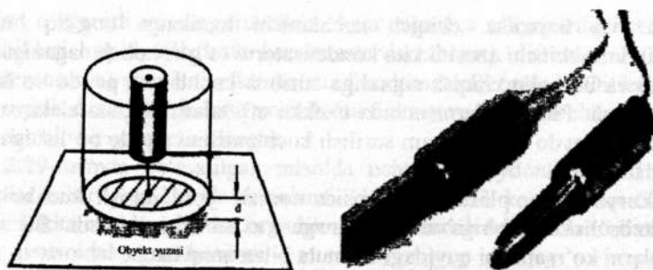
2.31 -rasm. Ekranlashtirilgan yuzaga ega bo'lgan sig'im datchigi: a – kesim yuzasi, b – tashqi ko'rinishi.
