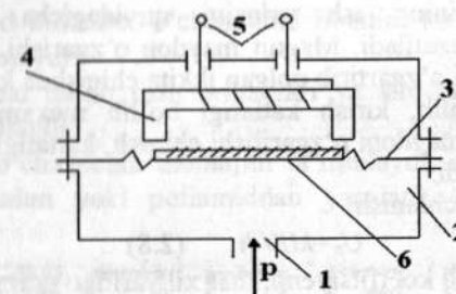
2.7-rasm. Induktiv manometrning sxemasi.
