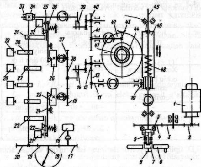
5.2- rasm. Unifikatsiyalangan elektr yuritmalar surgichlari kinematik sxemasi.
