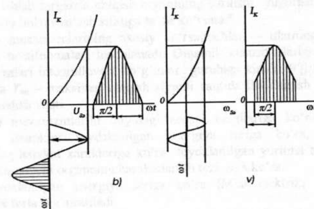
4.3-rasm. Kuchaytirgichning ish rejimlariga oid grafiklar.
