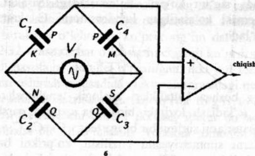
2.33-rasm. Sig'im ko'prik ko'rinishidagi datchiklarning ekvivalent sxemasi.
