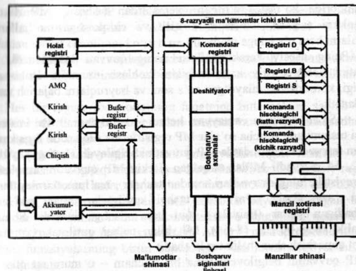
8.5 - rasm. 8-razryadli mikroprotsessorning struktura sxemasi.
