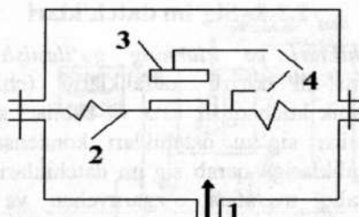
2.17-rasm. Sig'im manometrining sxemasi.
