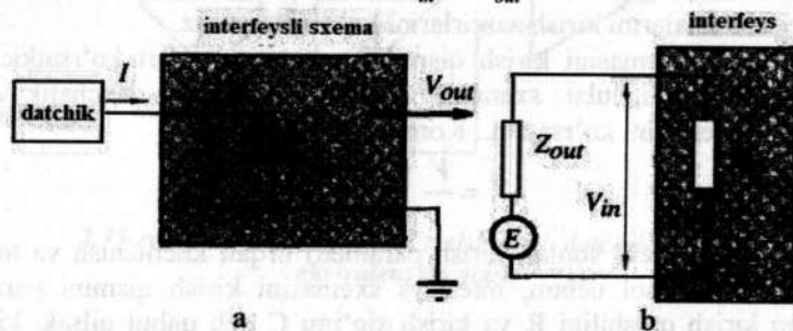
2.30-rasm, a – interfeys sxemasini kompleks kirish parametri; b – kuchlanish ko'rinishidagi chiqish signaliga ega bo'lgan datchikni ekvivalent sxemasi.
