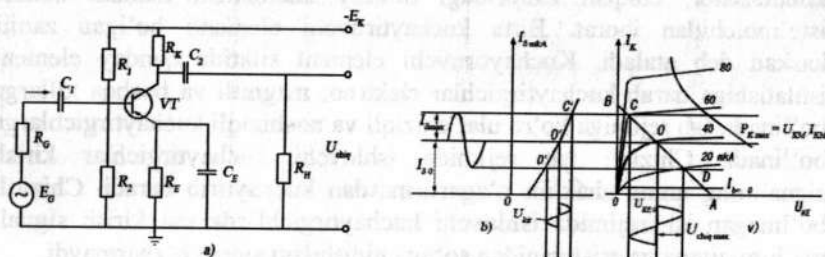
4.1-rasm. Umumiy emmitterli ( U_E ) kuchaytirish kaskadining sxemasi hamda kirish va chiqish xarakteristikalar.
