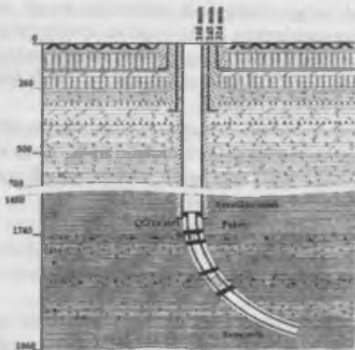
2.1-rasm. Tangensial tipdagi yo'naltirilgan quduqning vertikal proeksiyasi:
