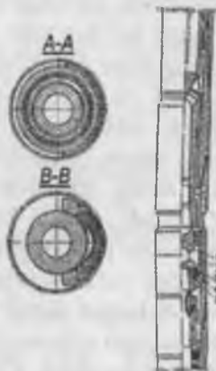
1.11-rasm. Seksiyalı turboburlar uchun og'diruvchi uskuna: 1-biriktiruvchi mufta; 2-ulama; 3-mufta venetsi; 4-po'lat shar; 5-pastki mufta.
