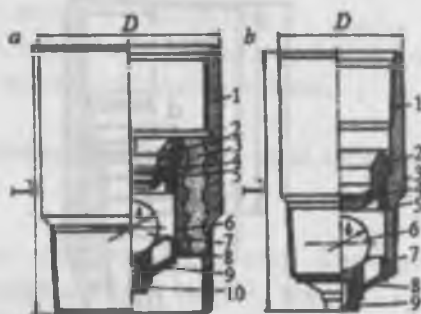
5.4-rasm. Sementlashda qo'llaniladigan drosselli teskari klapan: a) – SKOD-1: 1-korpus; 2-siquvchi halqa; 3-sement stakani; 4-qirqilgan shayba; 5-diafragma; 6-vtulka; 7-shar; 8-cheklagich; 9-membrana; 10-drossel. b) SKOD-2: 1-korpus; 2-siquvchi halqa; 3-qirqilgan shayba; 4-diafragma; 5-tayanch halqasi; 6-shar; 7-cheklagich; 8-membrana; 9-drossel.
