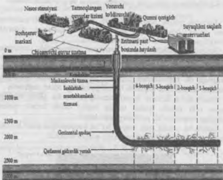
15.1-rasm. Gorizonttal uchastkani bosim ta'sirida yorishda qo'llaniladigan mashinalarni joylashuv holati
