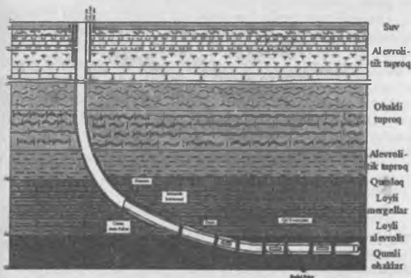
14.1-rasm. Quvurlarning orqa halqasini paklar va sementlash muftalari yordamida berkitish
