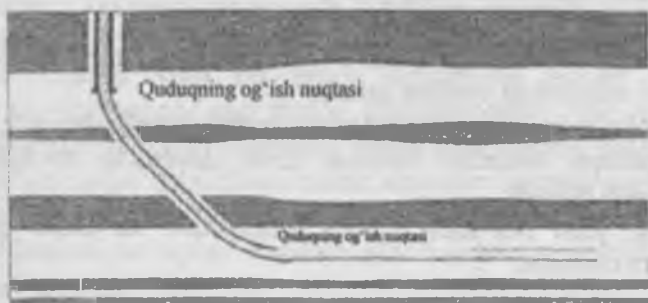
14.5-rasm. Gorizontal quduqning – uzun birikmasi sementlab mustahkamlangan
