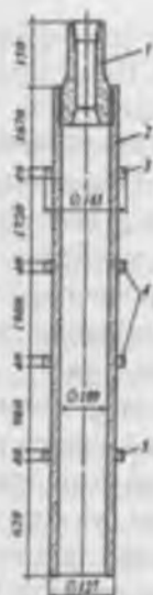
17.6-rasm. Diametri 168 mm li mustahkamlash tiznasini tekshirish uchun shablon: 1-uzatma; 2-korpus; 3-yuqori halqa; 4-oraliq halqa; 5-pastki halqa.
