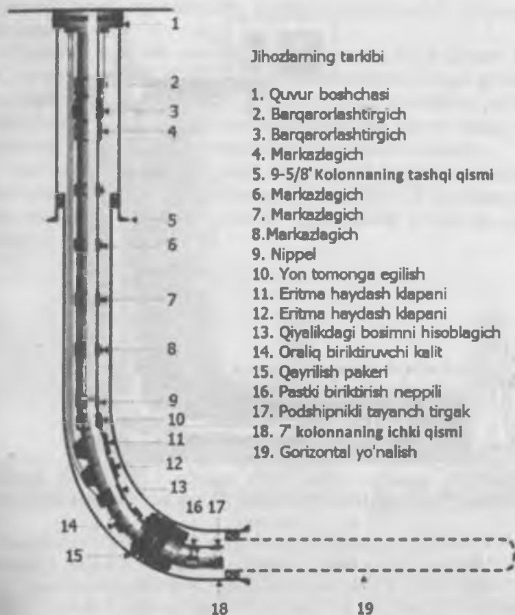
7.1-rasm. Gorizontal quduqning umumiy ko'rinishi va ichki jihozlari
