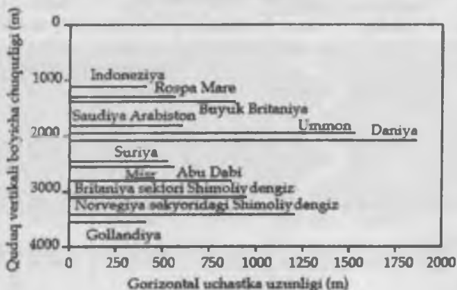
6.3-rasm. Gorizontalar quduqlarni burg'ilashni har xil mamlakatlarda kengayishi
