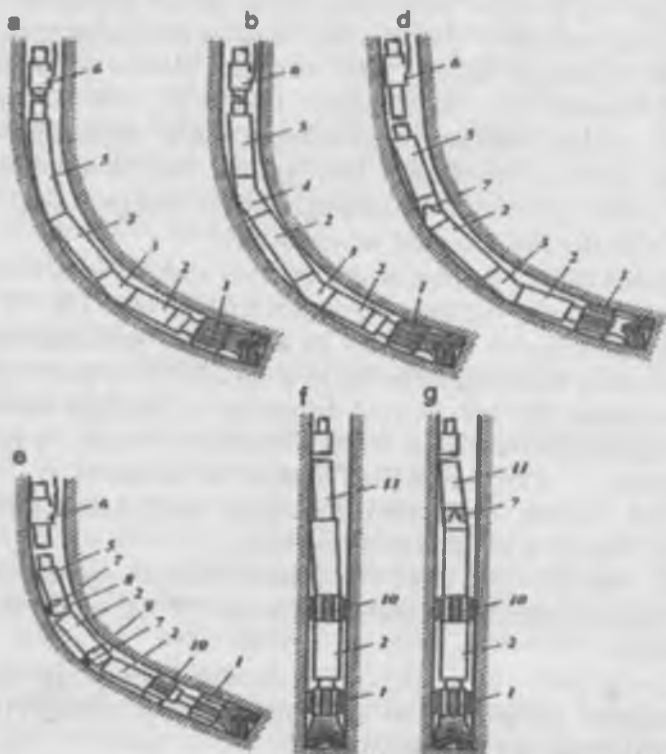
6.10-rasm. Gorizontal quduqlarni egrilantirishda qo'llaniladigan BTOJ-ni (burg'ilash tizmasini ostki jamlanmasi) sxemasi: 1-burg'i ustidagi kolibratori; 2-quduq dvigateli-og'dirgich; 3, 4-pastki va yuqori egri uzatmalar; 5-kabel kanalli aloqali telesistema; 6-yon tomondan kabel chiqarilgan uzatma; 7-egri uzatmali tirgagi; 8-sharnirli birikma; 9-sharnir korpusi; 10-quduq tubi dvigatelini markazlagichi; 11-diamagnit quvurlari.
