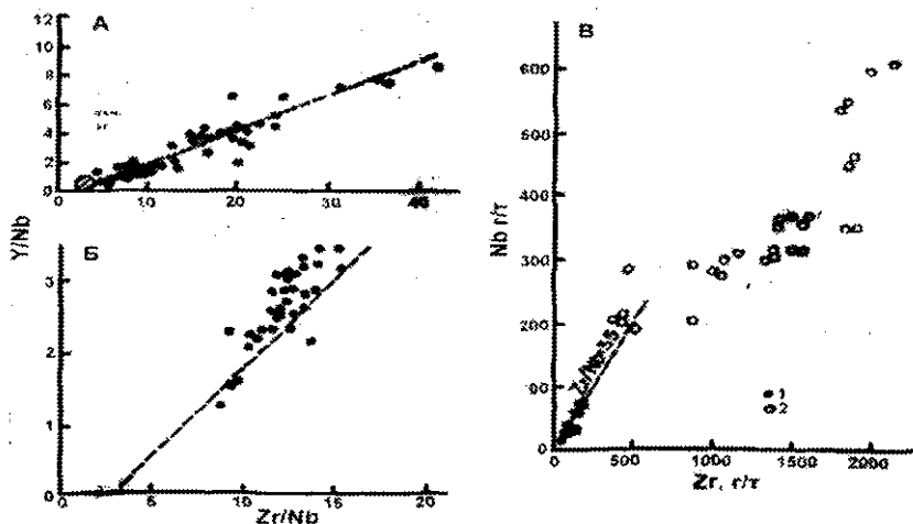
4.32- ras m. Y/Nb va Zr/Nb nisbatining bazaltlarda tarqalishi.
