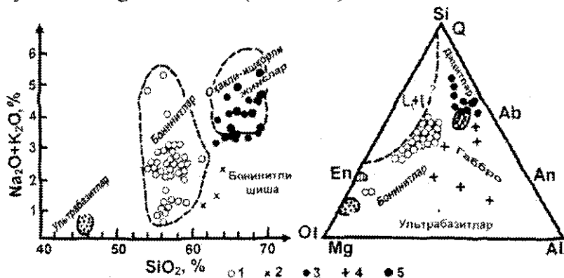
4.20-rasm. Ishqorlar va \text{SiO}_2 miqdorining boninit (1) seriyasida va ularning shishalarida (2) tarqalishi va ultrabazitlar (3), gabbrolar (4) bilan qiyoslash (L.L.Perchuk bo'yicha)
