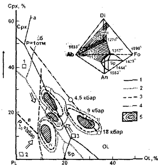
4.19- raʼsm . Bazaltlar tarkibini statistik maksimumlarini Pl-Cpx-Ol diagrammasida oʻzaro qiyoslash (T.I.Frolova boʻyicha).
