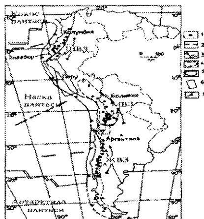
4.25-rasm. Janubiy Amerika Kordilyer-And tizmasida faol vulqon jarayonlarining taqsimlanishi (R.S.Thore, P.W.Frensis, L.Calladan).
