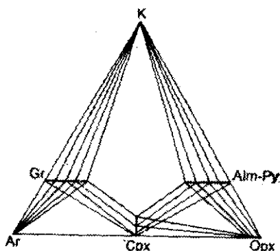
2.8-rasm. Eklogit fatsiyasining asosiy paragenezislari.
