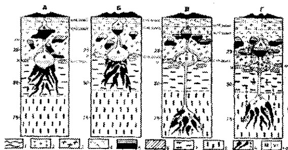
4.22-rasm. Past- (a, b) va yuqorikaliyli (v, g) vulqonlar rivojlanish modeli (Kuril-Kamchatka orollar yoyi (T.I.Frolova bo'yicha).
