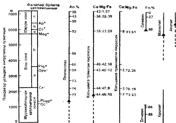
1.6-rasm. Skayergaard intruziyasining kumulat jinslardagi minerallar tarkibi. Qisqartmalar: Ol - olivin; Plag - plagioklaz; Cr - xromit; Ap - apatit; An - anortit; Fo - forsterit (L.Ueydjer, M.Braun, Xetch, bo'yicha)
