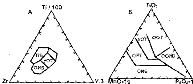
4.8-rasm. Geodinamik vaziyatlarning ba'zi bir elementlar nisbatiga qurab ajratish diagrammasi (J.A.Pearce, J.R.Carr).
