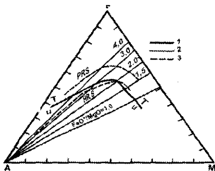
4.1-rasm. Asosiy petroximik seriyalarning AFM diagrammasidagi tutgan o'rni.
