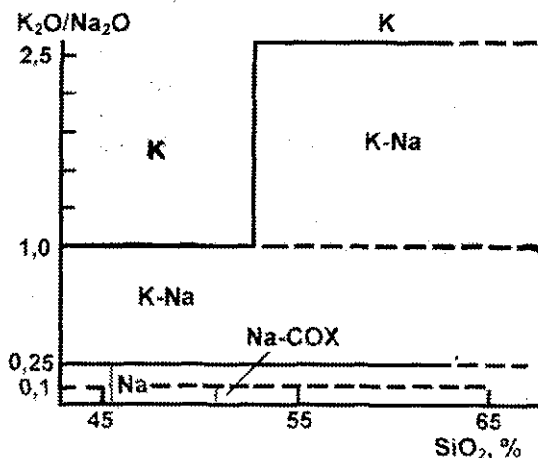
4.3-rasm. Seriyalarni K_2O/Na_2O + SiO_2 koeffitsiyenti yordamida bir-biridan ajratish sxemasi (A.Miyasiro bo'yicha).
