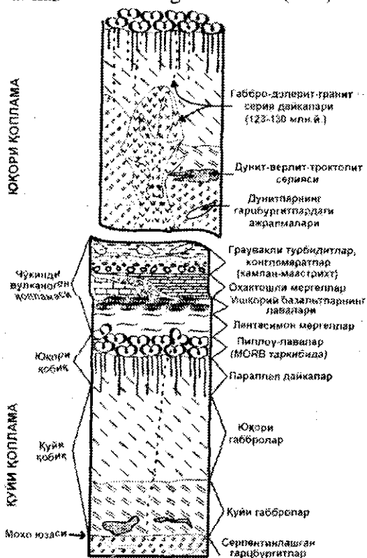
4.13-rasm. Masira orolining umumlashtirilgan litostratigrafik kesmasi (M.Kajima, bo'yicha).
