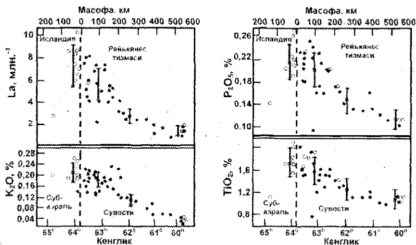
4.11- rasm. \text{La} , \text{K}_2\text{O} , \text{P}_2\text{O}_5 , \text{TiO}_2 ning toleit bazaltlarda tarqalishi.
