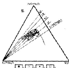
4.23-rasm. Kuril-Kamchatka orollarida vulqonitlar qo'shimchalarning tarkibi (T.E.Jrwin). A - intruziv jinslar (olivin-anortitli). Vulqonlar: 1-Zavaritskiy; 2-Mendeleyev; 3-Ksudach; 4-5,6-ularidagi qo'shimchalar; B-effuziv va gipabissal turdagi qo'shimchalar. 1-2-Bezimyanniy; 3-4-Kazimen.
