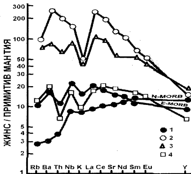
4.9-rasm. Gavayi orollaridagi vulqonik jinslarda mikroelementlarning tarqalishi. (sodda mantiya tarkibiga nishatan) (S.S.Sun bo'yicha); 1 - okean bazaltlari (N-MORB va E-MORB); 2-3 - orollar jinslari (2 - melilitli nefelinitlar, 3 - ishqorli bazaltlar); 4 - oddiy toleitlar.
