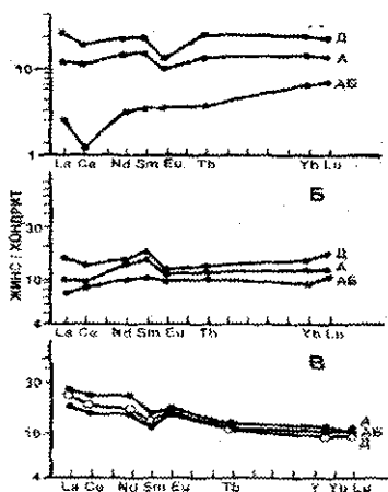
4.21-rasm. Kuril-Kamchatka orollar yoyidagi vulqonik jinslarda nodir elementlarning taqsimlanishi (xondritga nishatan).
