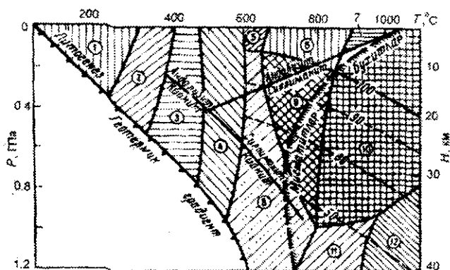
2.7-rasm. Metamorflashgan gilli jinslarning mineral fatsiyalari (A.A. Marakushen, 1988).
