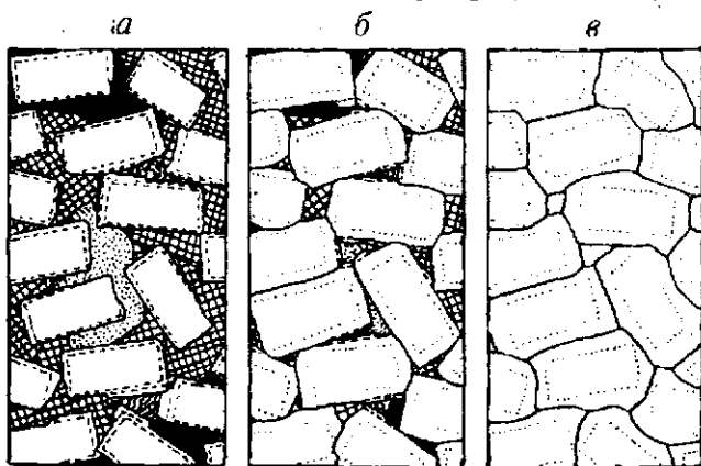
1.11-rasm. Kumulatlarining tuzilishi. a - ortokumulat; b - mezokumulat, v - adkumulat (Filbotts bo'yicha, 1880)
