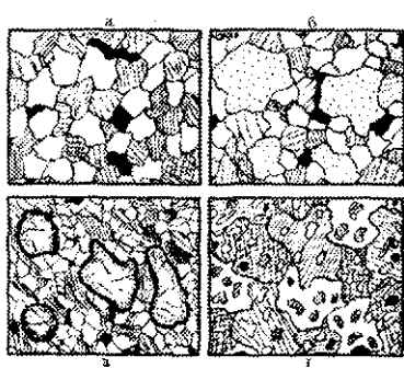
2.4-rasm. Metamorfik jinslarning tashqi ko'rinishi (teksturasi) a - slanetssimon; b - gneyssimon; v - yo'l-yo'l; g - ezilgan, to'lqinsimon
