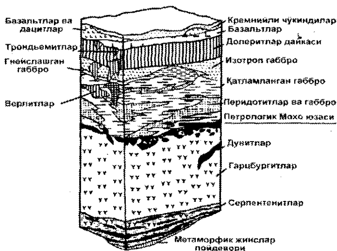
4.12-rasm. Omandagi ofiolitlarning umumlashtirilgan tasviri tasviri (D.Marquer, I.Mercolli, T.Peters)
