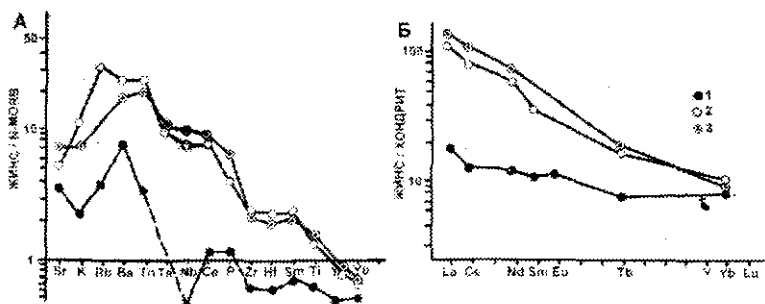
4.27-rasm. And vulqonik mintaqasidagi bazalt va andezitlarda mikroelementlarning tarqalishi.
