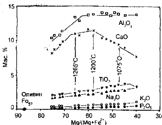
1.9-rasm. Toleitli bazaltlardagi plagioklaz (Rl) va piroksen (Rx) kristallari orasidagi magmatik eritmaning likvatsiyasi (A.R.Filpots, bo'yicha, Konnektikut, A.Sh).
