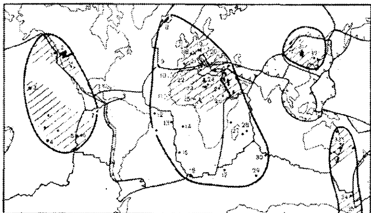
4.36-rasm. Yangi davrdagi (15 mln. y.) plitaichi magmatik jarayonlar qayd qilingan o'lkalar (L.P.Zonnenshayn, bo'yicha).
