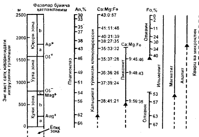
1.7-rasm. Skayergaard intruziyasidagi kumulat minerallarning o'zgaruvchanligi. Qisqartmalar: Mg - magnetit; Aug - piroksen; Ol - olivin; Ap - apatit; An - anortit; Fo - forsterit (Ch.Xeydjes, 1988)
