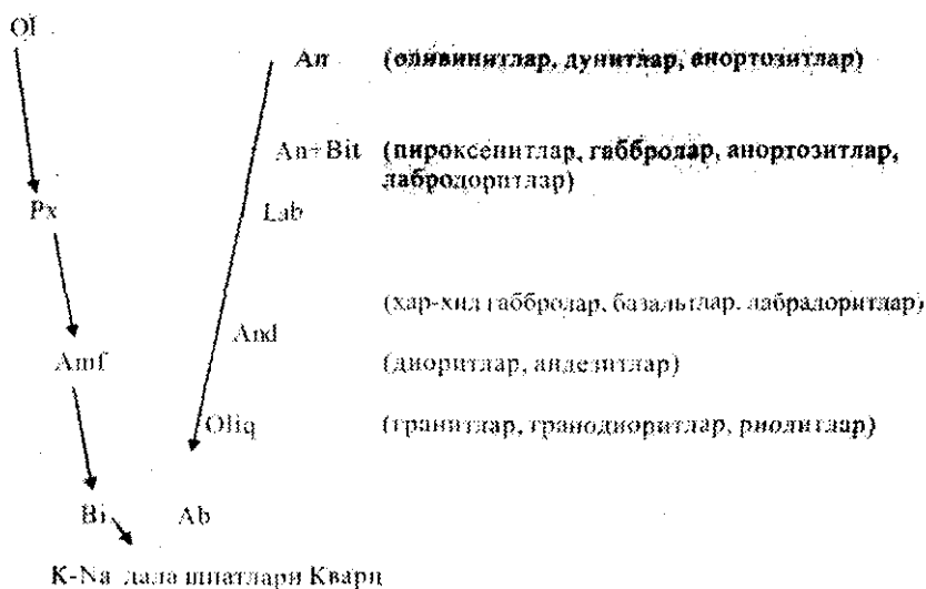
1.4-rasm. N.Bouen reaksiya qatori.
