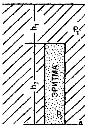
1.1-rasm. Oritqcha bosimning (DR) paydo bo'lishi. Belgilar: h_1 , h_2 -balandlik; eritmaning ( R_2 ) zichligi ( DR=R_1-R_2 ) gh (V.S.Popov bo'yicha, 2002 y)
