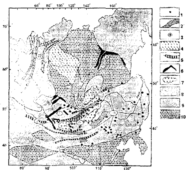
4.39-rasm. Sibir platformasida plitaiichi magmatik maydonlarining tarqalishi (V.V.Yarmolyuk, bo'yicha)
