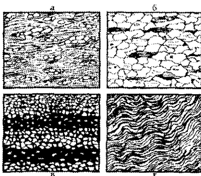
2.5-rasm. Metamorfik jinslarning dona katta-kichikligi bo'yicha tasnifi (V.S.Popov 2001 y.).
