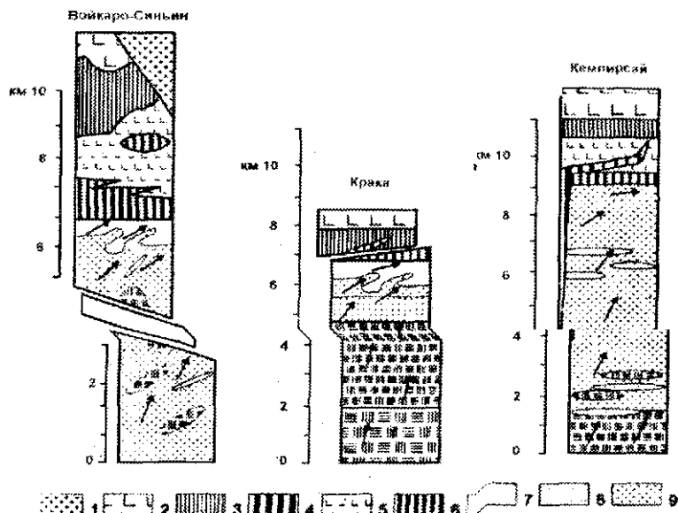
4.16-rasm. Uralofiolitlarining soddalashtirilgan kesmalari (A.A.Knipper, G.N.Savelyeva, A.Ya.Shardskin bo'yicha).
