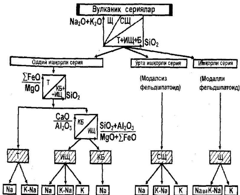
4.5-rasm. Seriyalarni tasniflash diagrammasi (T.I.Frolova bo'yicha). Seriya turlari: T - toleitli; ИЩ - ohak-ishqorli; КБ - komatiit-boninitli; СЩ - o'rta ishqorli; Щ - ishqorli; Na - natriyli; K - kaliyli.
