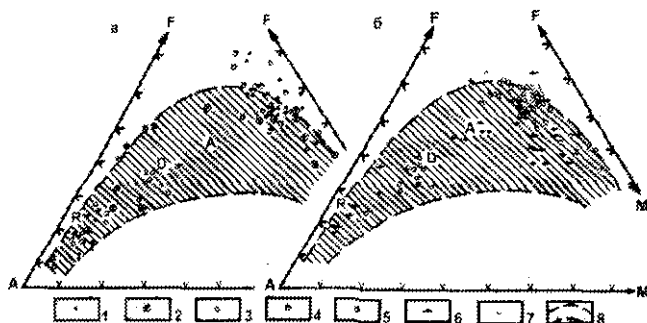
4.41-rasm. Yashiltosh mintaqalaridagi vulqon jinslarining AFM diagrammasidagi tarkibi (A.F.Grachev, bo'yicha)
