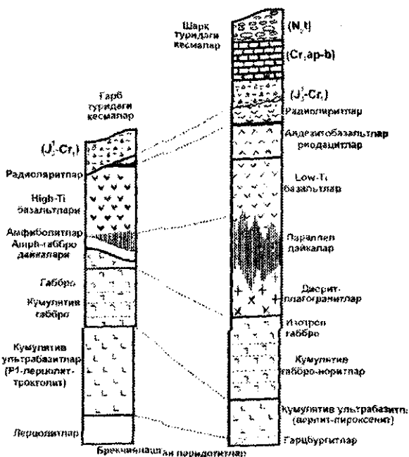
4.15-rasm. Mirdita zonasidagi (Albaniya) ikki xil ofiolitlar kesmasi. (O.G.Bagdanovskiy, G.S.Zakariadze, S.F.Karpenko, S.K.Zlobin, A.A.Savelyev, O.V.Astruxansev, A.L.Knipper, A.Ya.Sharaskin)
