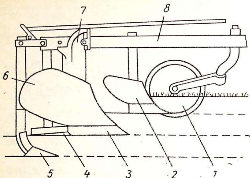
1.3- расм. Плугнинг ишчи органлари
