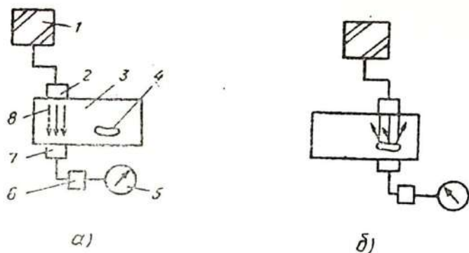
6.8- расм. Ультратовуш дефектоскопининг схемаси: 1 — ультратовуш генератори; 2 — пьезоэлектрик нурантиргич; 3 — деталь; 4 — нуқсон; 5 — индикатор; 6 — купайтиргич; 7 — — ультратовушнинг қабул қилувчи датчик; 8 — ультратовуш тўлқини
