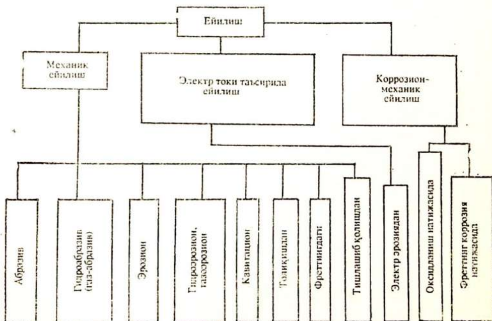
5.4- расм. Ейилиш турларининг ГОСТ 23. 002— 78 бўйича таснифи
