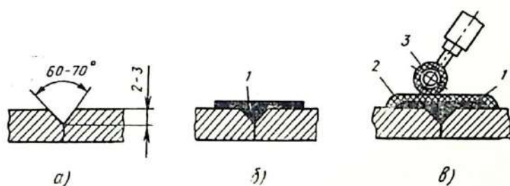
7.33-расм. Дарзларни беркитиш схемаси:
