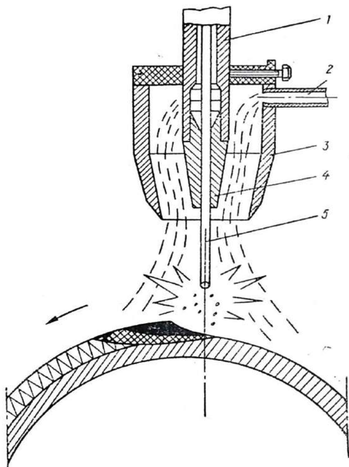
7.23- расм. Цилиндрсимон деталларни карбонат анг. дрид гази муҳитида автоматик суюқлантириб қоплаш схемаси:
