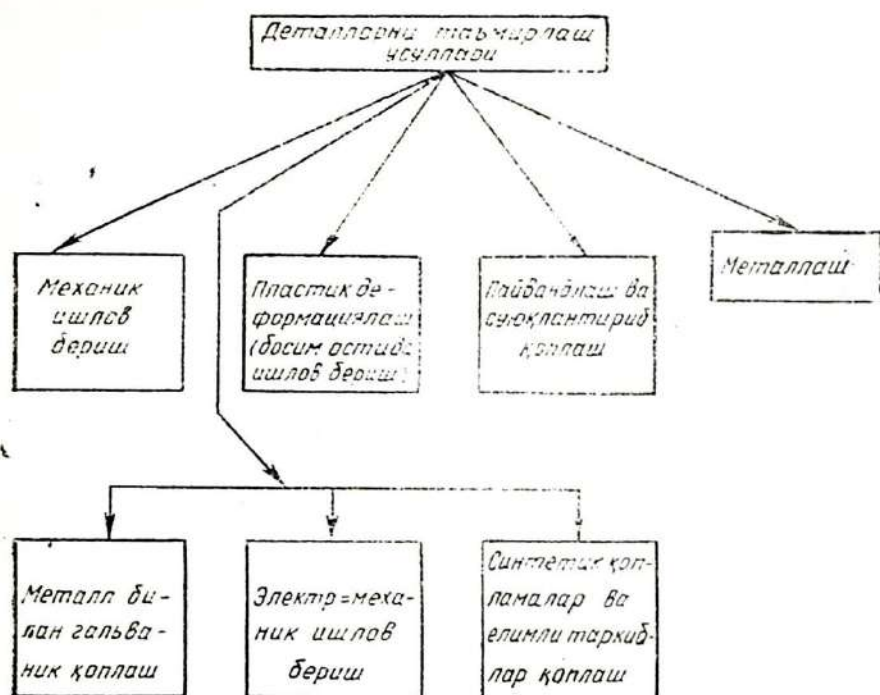
7.1- расм. Деталларни таъмирлаш усуллариининг таснифи
