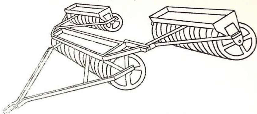
1.6- расм. Халқа-тирпоқли ғалтакмола
