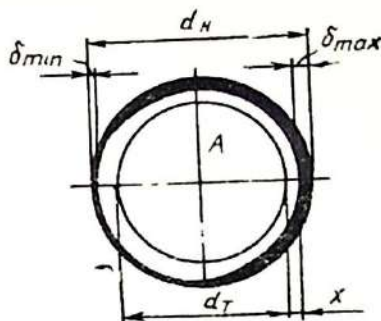
7.2-расм. Валнинг таъмирлаш ўлчамини ҳисоблаш схемаси
