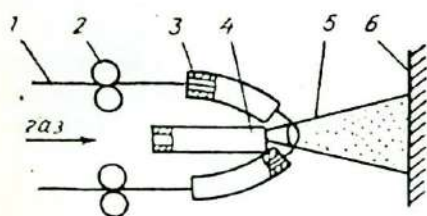
7.28- расм. Электр ёйи воситасида металл шемаси:
