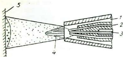
7.27- расм. Газ алангаси воситасида металллада ишлатиладиган металлатор пуркаш каллагининг схемаси:
