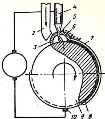
7.18- расм. Флюс қатлами остида пайвандлаш схемаси:
