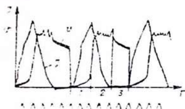
7.22- расм. Ток кучи ва кучланишнинг ўзгариш осциллограммалари
