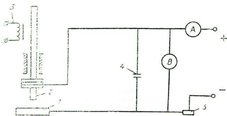
7.26- расм. Электр учқуни билан ишлов бериш схемаси:
