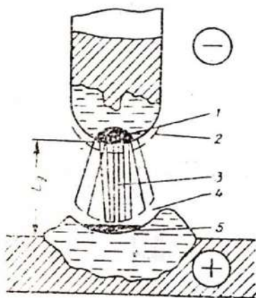
7.17- расм. Пайвандлашдаги электр ёйининг тузилиш схемаси:
