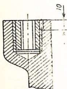
7.43- расм. Деталларни янги (қўшимча) деталь ўрнатиш усули билан таъмирлаш
