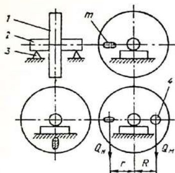
6.9- расм. Деталларни статик мувозанатлаш схемаси:
