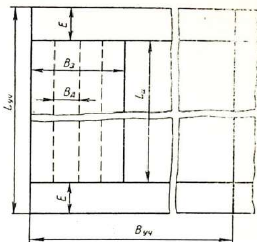
3.1-расм. Трактор агрегатининг иш участкаси схемаси
