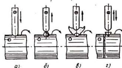
7.21- расм. Тебранма ёй воситасида сууюқлантириб қоплашда электрод материалнинг эриши ва унинг ҳаракат цикл схемаси:
