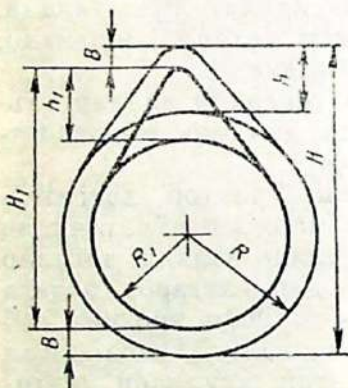
7.39- расм. Кулачокни жилвирлаш йўли билан таъмирлаш схемаси
