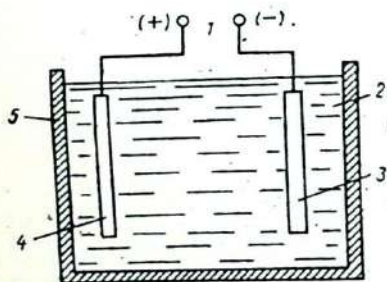
7.30- расм. Электролиз жараёни схемаси:
