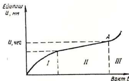
5.5- расм. Ейилишнинг намунавий эгри чизиги:
