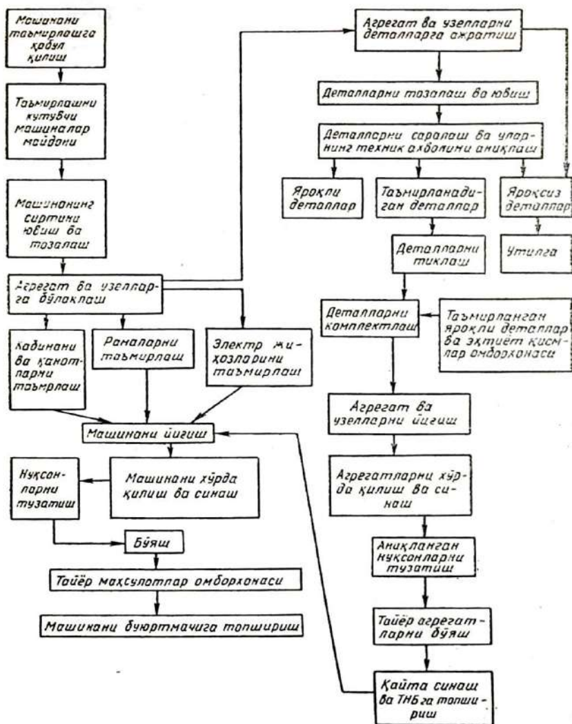
6.1- расм. Тракторни капитал таъмирлаш жараёнининг схемаси
