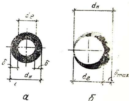
7.3-расм. Валнинг ейилиш схемаси: а — текис ейилиш; б — бир томонлама ейилиш
