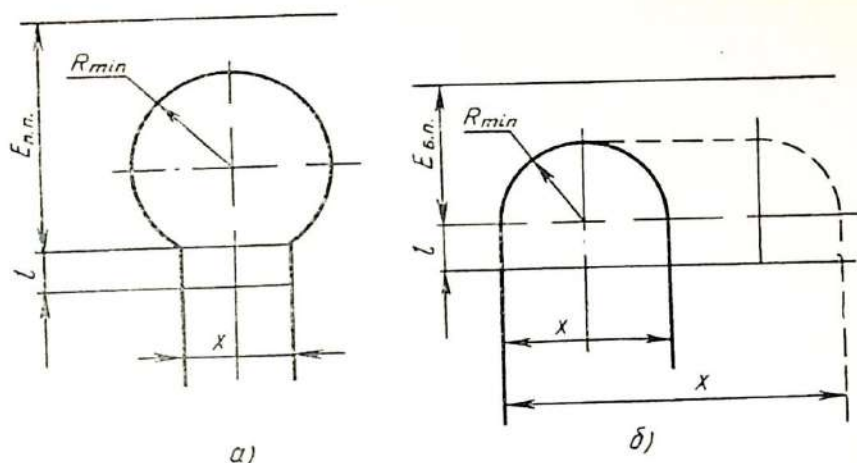
3.3- расм. Бурилиш турлари:
