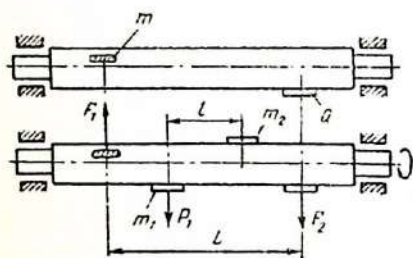
6.10- расм. Деталларни динамик мувозанатлаш схемаси
