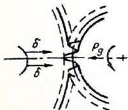
7.12- расм. Накаткалаш схемаси
