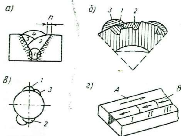
7.25- расм. Пайвандлашнинг махсус усуллари:
