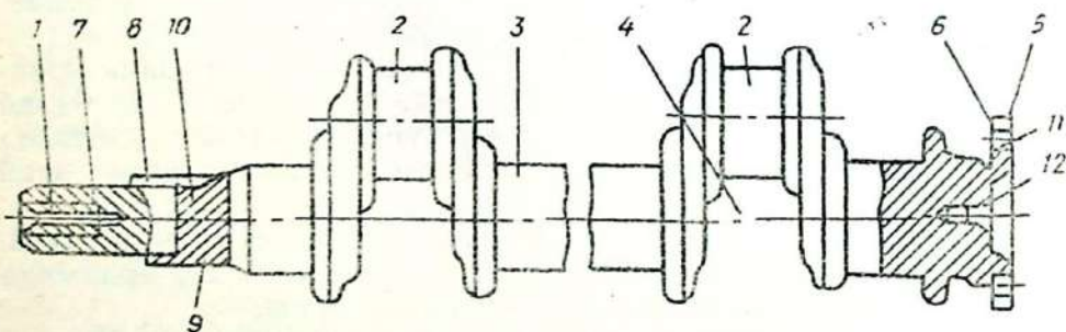
7.37- расм. СМД- 14 двигателининг тирсакли валидаги нуқсонлар учрайдиган жойлар схемаси
