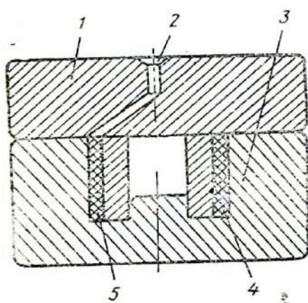
7.34- расм. Ёйилган деталь юзасини bosим остида капрон билан қоплаш схемаси;
