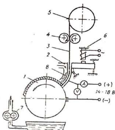
7.20- расм. Тебранма ёй воситасида сууюқлантириб қоплаш қурилмасининг схемаси:
