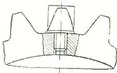
7.41- расм. Ғилдирак тишларнинг шпилька қўйиш ёрдамида таъмирлаш
