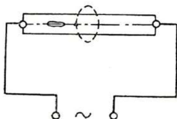
6.5- расм. Ташқи юзадаги бўйлама дарзларни аниқлашдаги циркуляр магнитланиш схемаси
