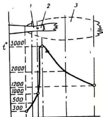
7.14- рasm. Ацетилен-кислород алангаси ёрдамида пайвандлашда аланганинг тузилиши ва температурасининг ўзгариш схемаси:
