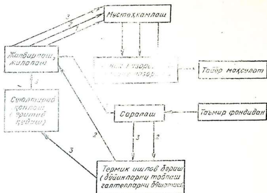
7.38- расм. Тирсакли вал бўйинларини йўналиш (маршрут) лар бўйича таъмирлаш технологик жараёнининг схемаси
