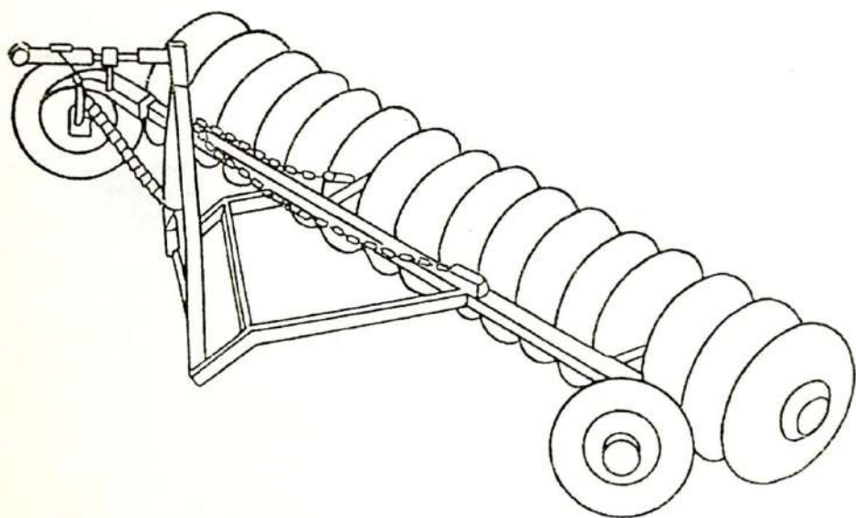
1. 1- расм. Дискли осма юза юмшаткич (лушчи́льник)
