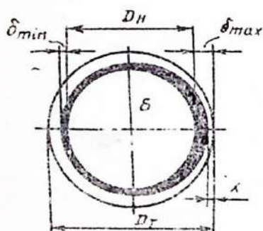
7.4- расм. Тешикнинг таъмирлаш ўлчамини аниқлаш схемаси
