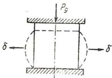
7.5-расм. Деталларни чўктириш усулида таъмирлаш схемаси
