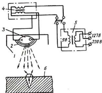
6.7-расм. Флуоресцент дефектоскопнинг схемаси:
