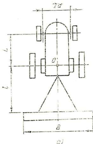
3.2-расм. Трактор агрегатининг ҳаракатланиши ва бурилиш схемаси:
