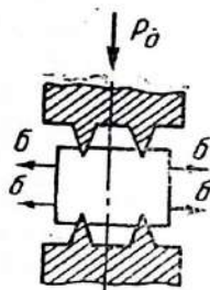
7.7 расм. Деталларни ботириш усулида таъмирлаш схемаси
