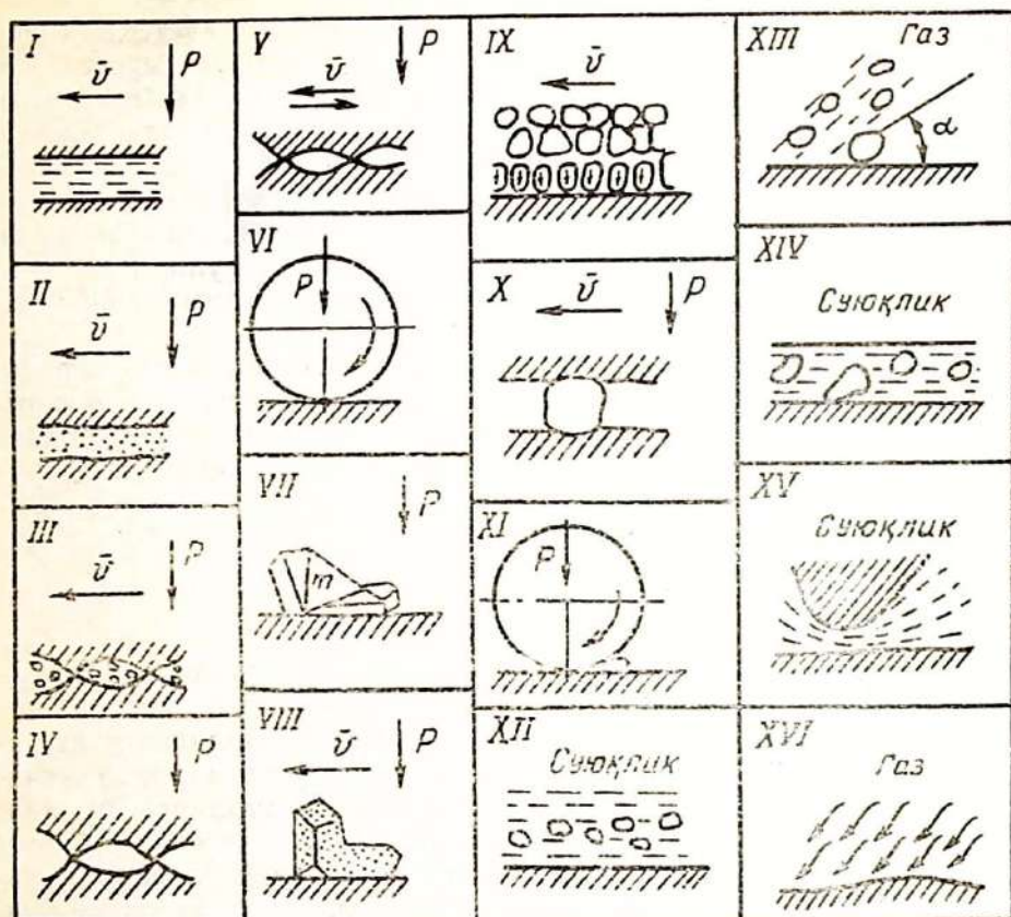
5.3- расм. Ейилиш жараёнининг М. М. Тененбаум таснифи
