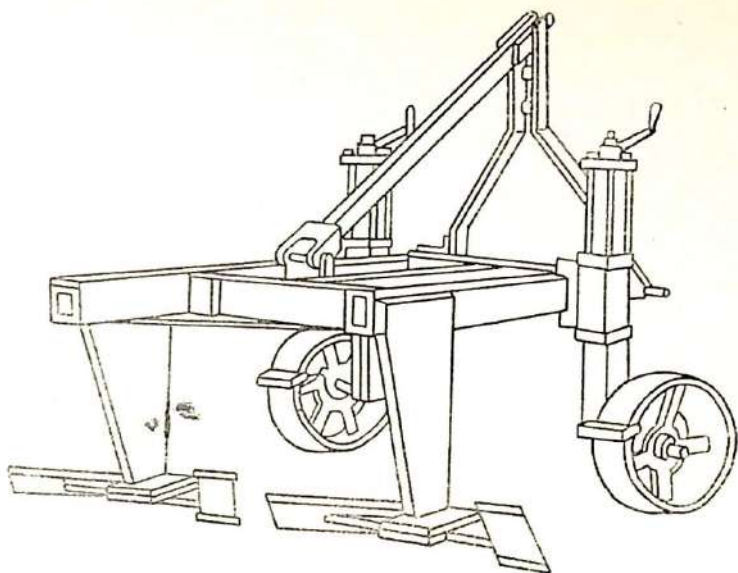
1.4- расм. ҚПГ- 250 маркали ётиқ кесувчи ва чуқур юмшатувчи культиватор
