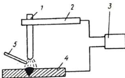
7.15- расм. Н. Н. Бенардос усулида пайвандлаш схемаси:
