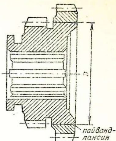
7.42- расм. Шестерня блокнинг тишли чамбаракларнинг алмаштириш йўли билан таъмирлаш
