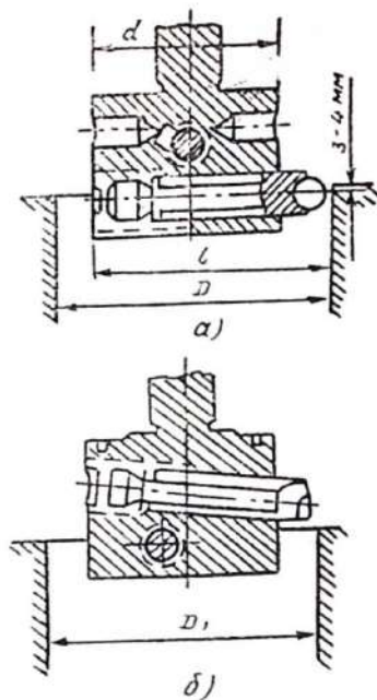
7.36- расм. Цилиндрни марказлаштириш (а) ва кескични ўрниатиш (б)
