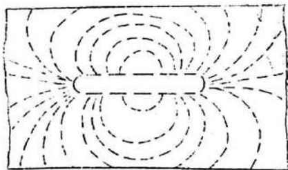
6.3- расм. Ферромагнит темир оксиди кукунининг магнит майдони таъсирида жойлашиш схемаси
