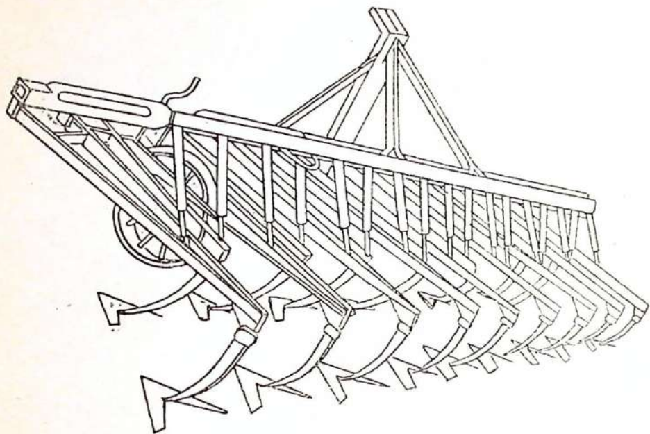
1.5- расм. Тупроққа ёппасига ишлов берувчи культиватор
