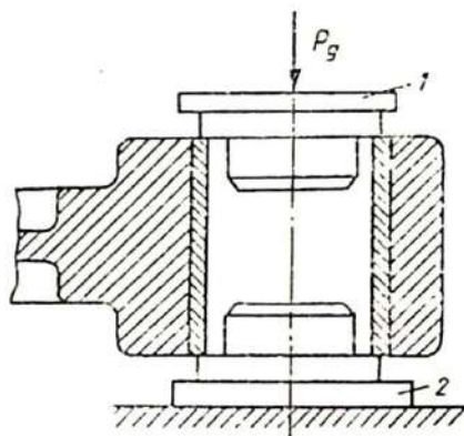
7.6-расм. Шатуннинг юқори каллагидagi бронза втулкани чўктириш схемаси
