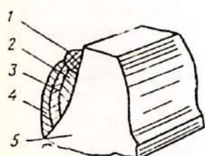
7.40- расм. Тишли ғилдираклар тишини суюқлантириб қоплаш усули билан таъмирлаш схемаси
