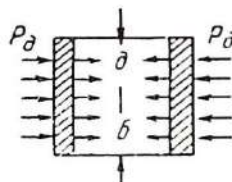
7.9- расм. Втулкани торайтириш схемаси
