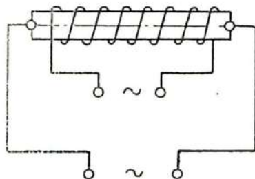
6.6- расм. Ташқи юзадаги дарзларни аниқлашдаги аралаш магнитлаш схемаси
