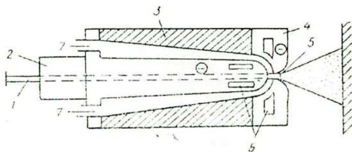
7.29- расм. Плазма-ёй металлизатори каллагининг схемаси:
