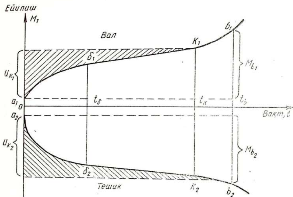
5.6- расм. Вал — тешик бирикмасидаги тирқишнинг катталашуви
