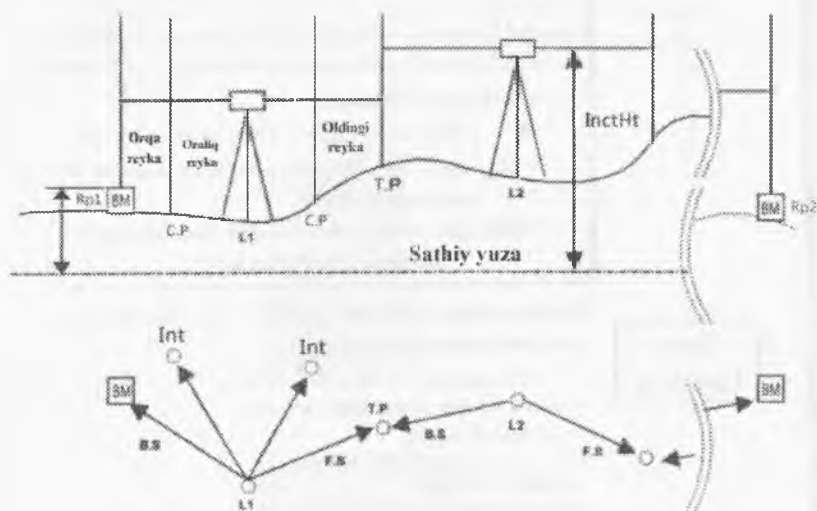
2.20-rasm.DL-102C TOPCON raqamli nivelirda nivelir yo'lni o'tkazish:
