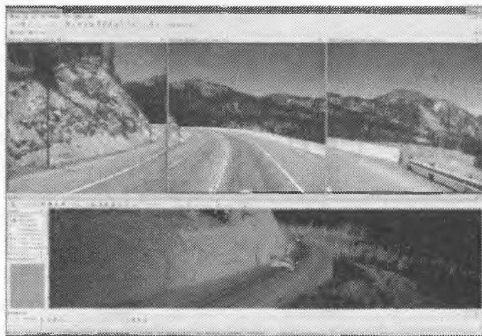
3.13-rasm. Trident Analyst yordamida ishlab chiqilgan mobil fotosyomka va lazer skanerlash natijalari
